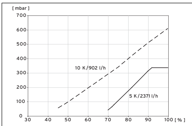
Abb. 9.8 Diagramm Leistungsoptimierung Heizkreispumpe VWW 101/3
