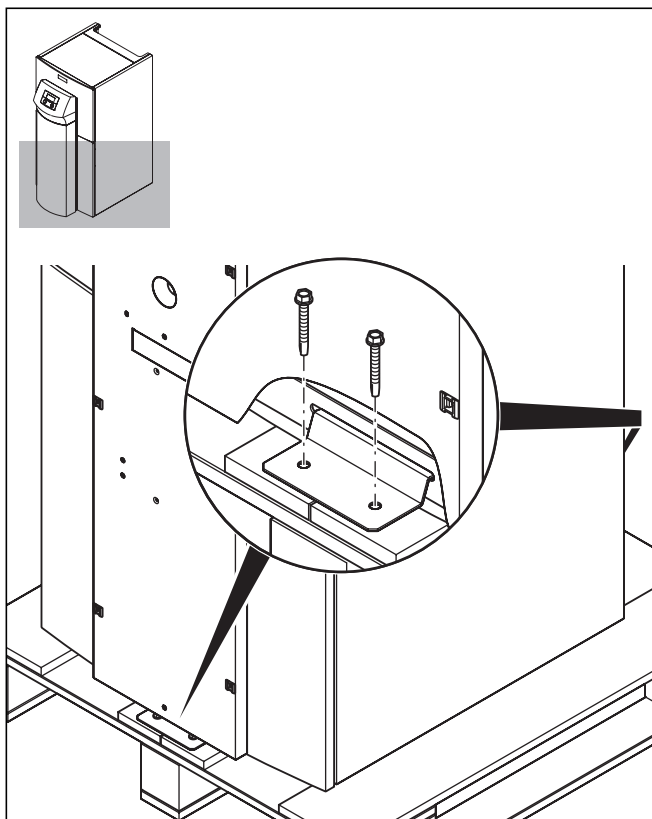
Abb. 4.4 Transportsicherungen entfernen
