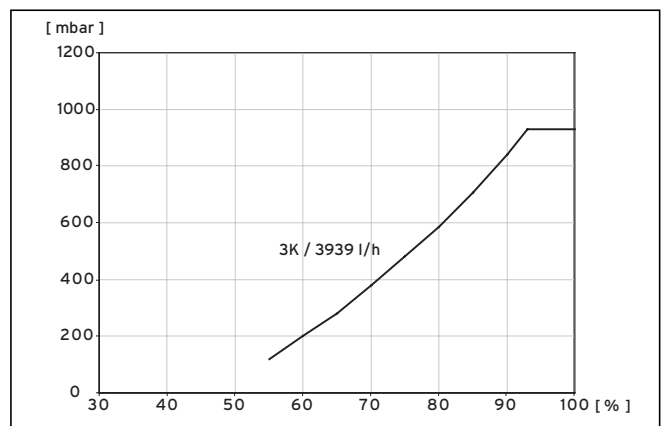
Abb. 9.5 Diagramm Leistungsoptimierung Solepumpe VWS 171/3
