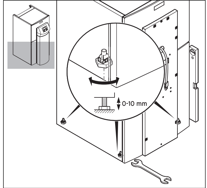
Abb. 4.6 Stellfüße einstellen
