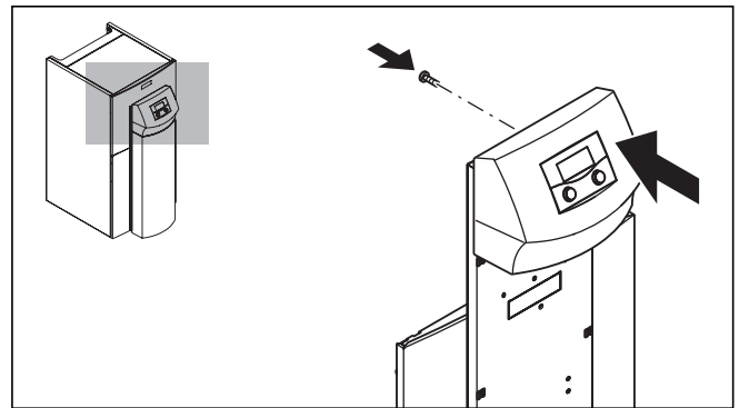
Abb. 7.17 Bedienkonsole montieren
