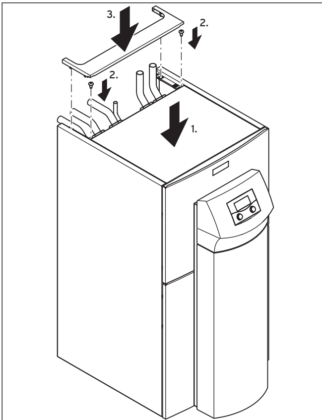
Abb. 7.21 Obere Verkleidungsteile montieren
