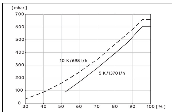
Abb. 9.7 Diagramm Leistungsoptimierung Heizkreispumpe VWS 81/3
