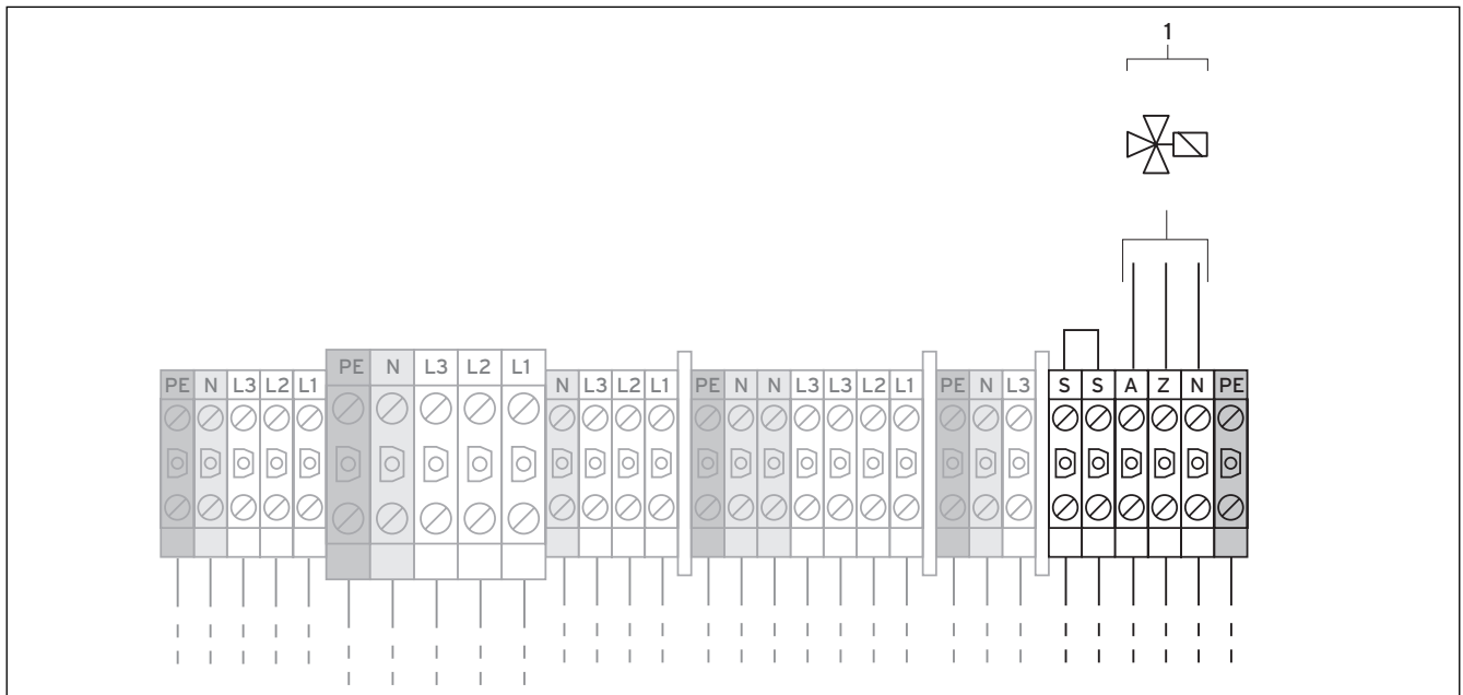
Abb. 7.7 Externes 3-Wege-Ventil für Pufferspeicher anschließen
