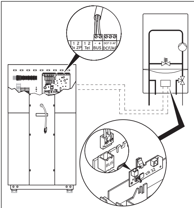
Abb. 7.14 Heizgerät mit eBUS-Schnittstelle anschließen
