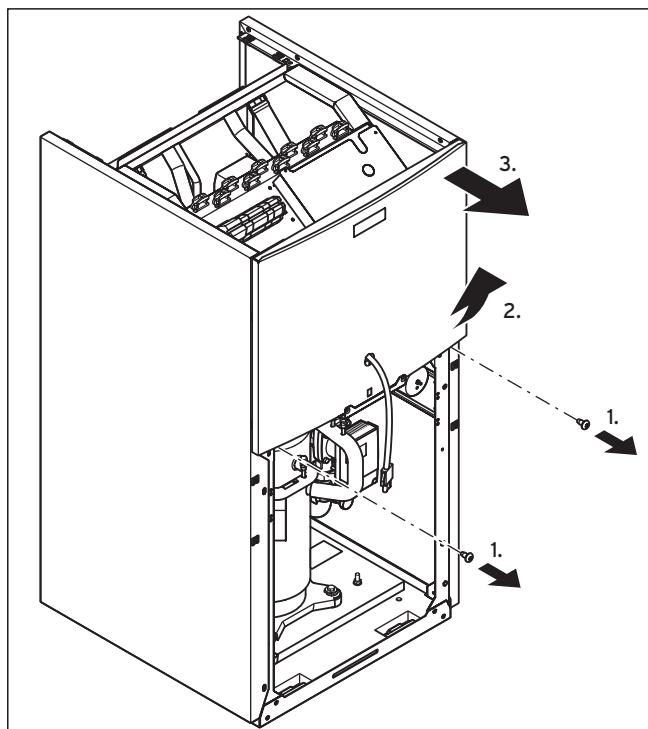
Abb. 4.9 Oberteil der Frontverkleidung abnehmen
