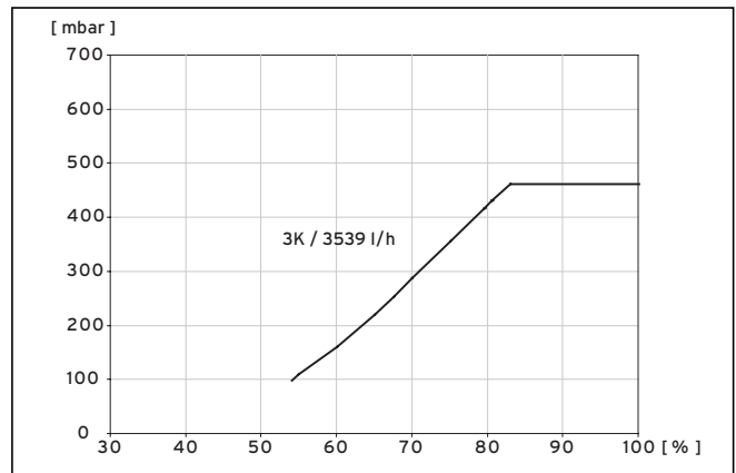
Abb. 9.4 Diagramm Leistungsoptimierung Solepumpe VWS 141/3
