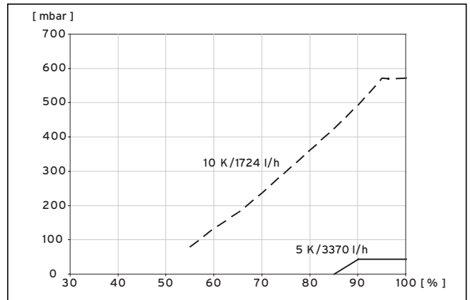
Abb. 9.9 Diagramm Leistungsoptimierung Heizkreispumpe VWW 141/3
