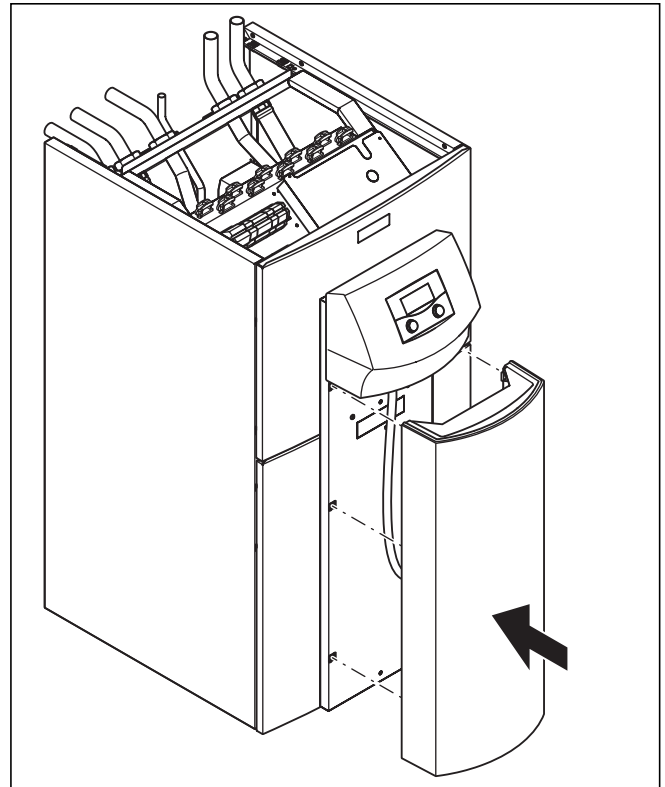
Abb. 7.20 Abdecksäule der Bedienkonsole montieren
