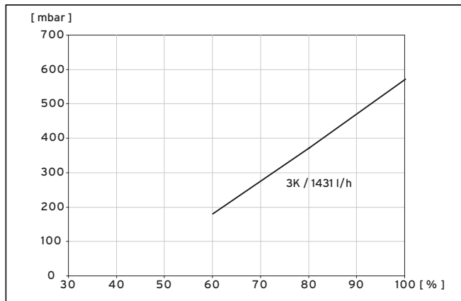
Abb. 9.1 Diagramm Leistungsoptimierung Solepumpe VWS 61/3
