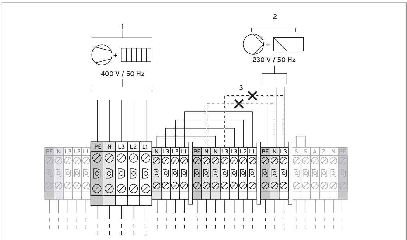
Abb. 7.4 Zweikreis-Einspeisung Sondertarif
