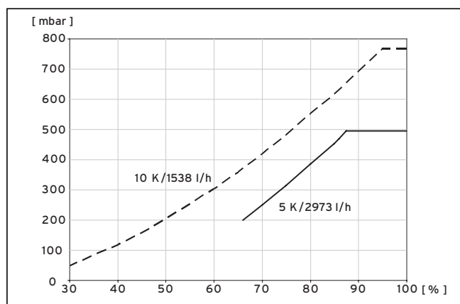
Abb. 9.10 Diagramm Leistungsoptimierung Heizkreispumpe VWS 171/3
