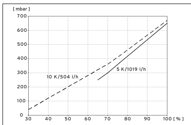
Abb. 9.6 Diagramm Leistungsoptimierung Heizkreispumpe VWS 61/3
