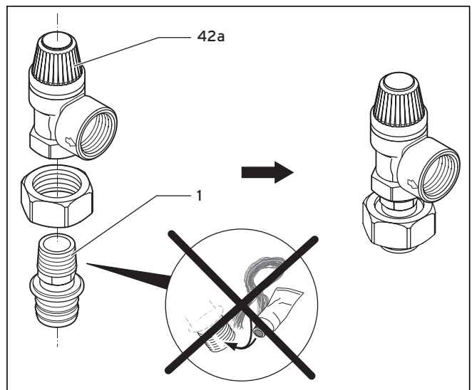
Abb. 5.9 Sicherheitsventil montieren
