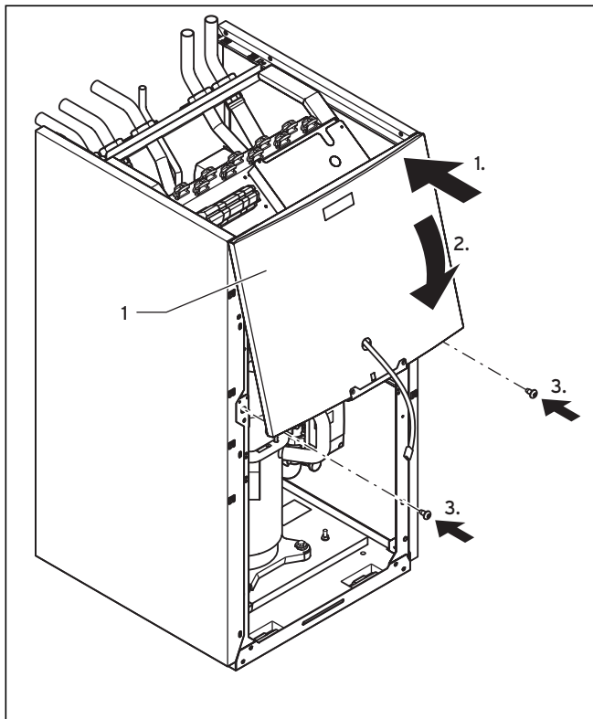
Abb. 7.16 Oberteil der Frontverkleidung montieren
