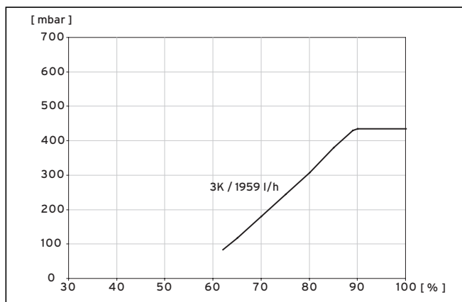
Abb. 9.2 Diagramm Leistungsoptimierung Solepumpe VWS 81/3
