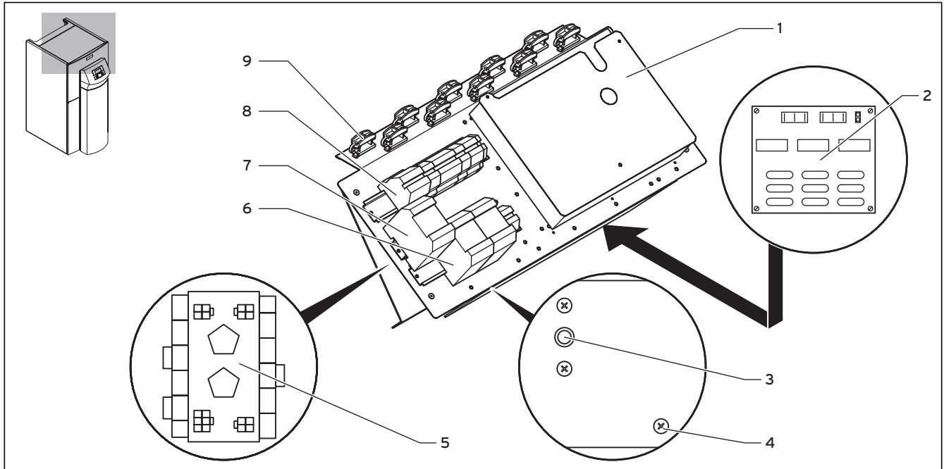
Abb. 7.1 Elektro-Schaltkasten (VWW)
