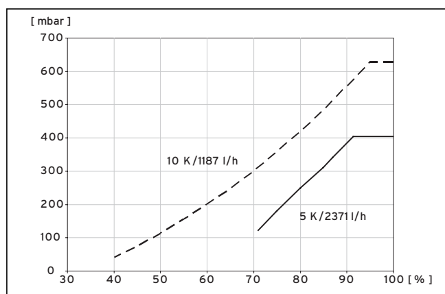
Abb. 9.9 Diagramm Leistungsoptimierung Heizkreispumpe VWS 141/3
