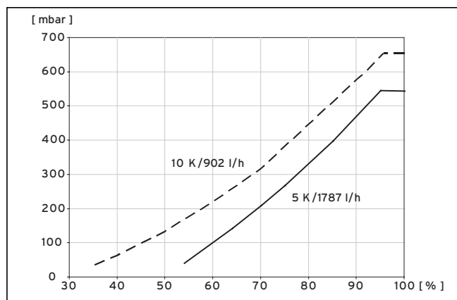
Abb. 9.8 Diagramm Leistungsoptimierung Heizkreispumpe VWS 101/3
