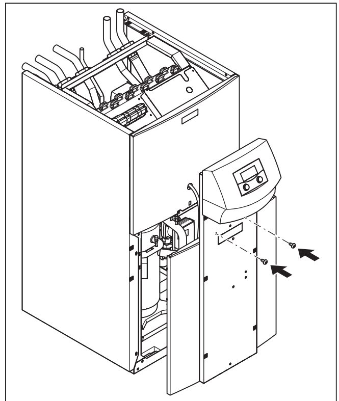
Abb. 7.18 Unterteil der Frontverkleidung montieren
