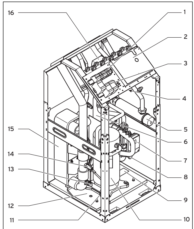
Abb. 3.6 Vorderansicht geöffnet (VWW)
