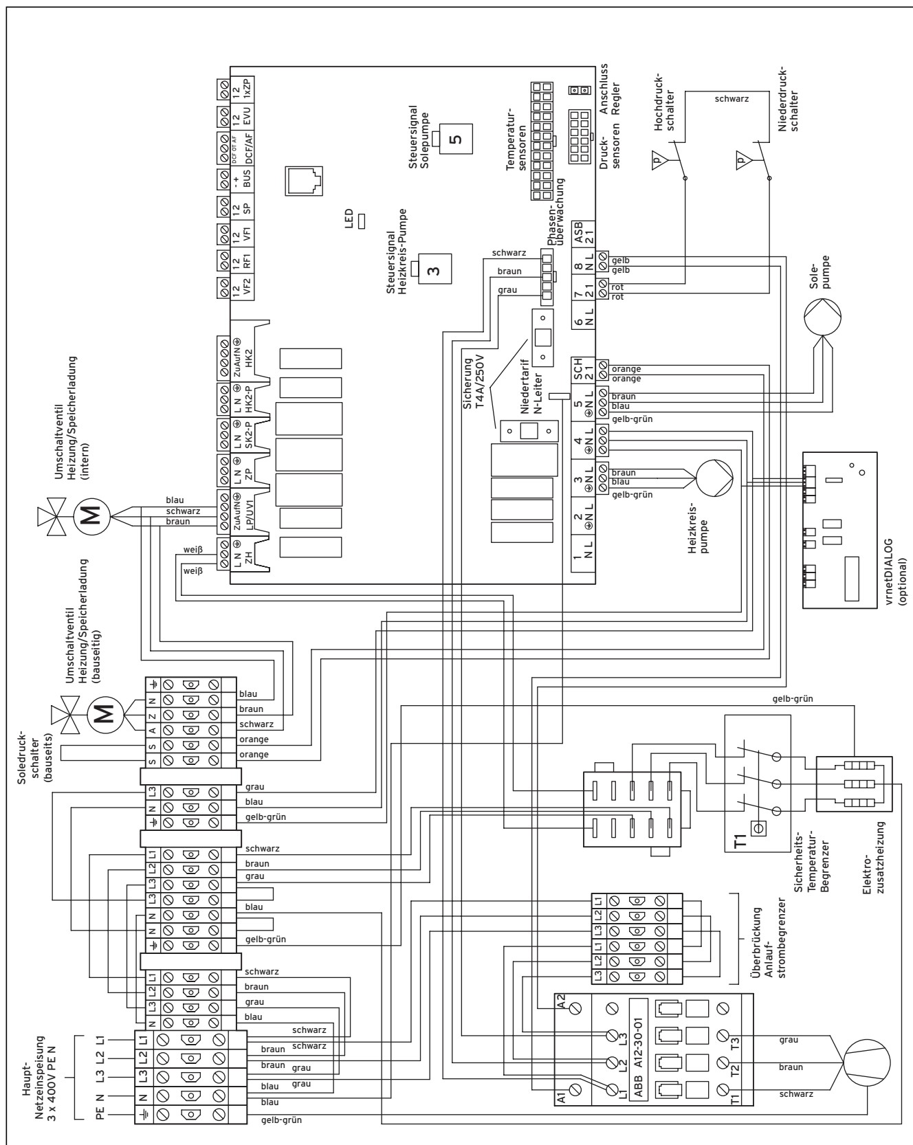
Abb. 3, Anhang, Stromlaufplan VWS 61/3 - VWS 141/3
