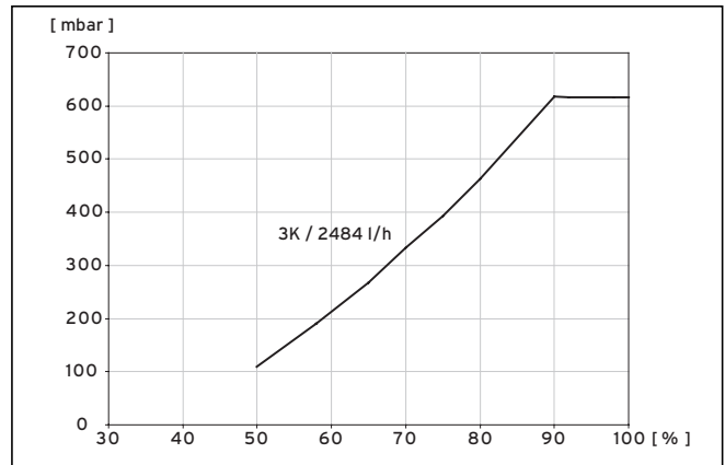
Abb. 9.3 Diagramm Leistungsoptimierung Solepumpe VWS 101/3
