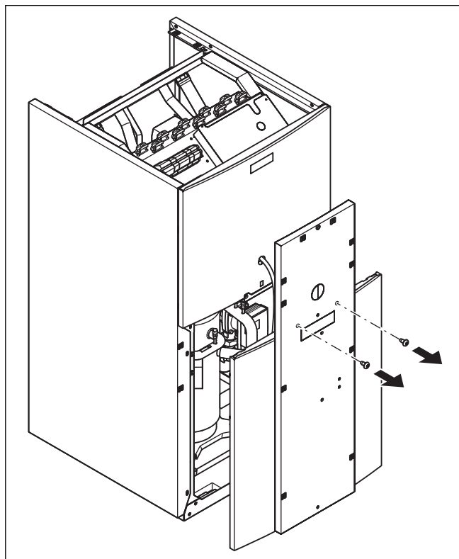
Abb. 4.8 Unterteil der Frontverkleidung abnehmen
