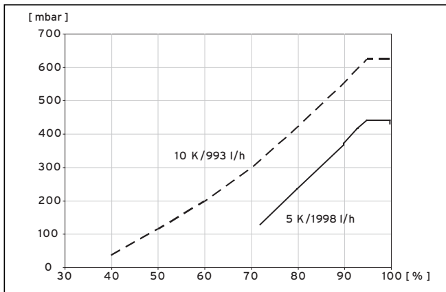
Abb. 9.7 Diagramm Leistungsoptimierung Heizkreispumpe VWW 81/3
