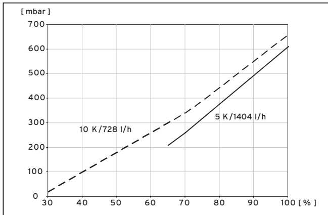
Abb. 9.6 Diagramm Leistungsoptimierung Heizkreispumpe VWW 61/3
