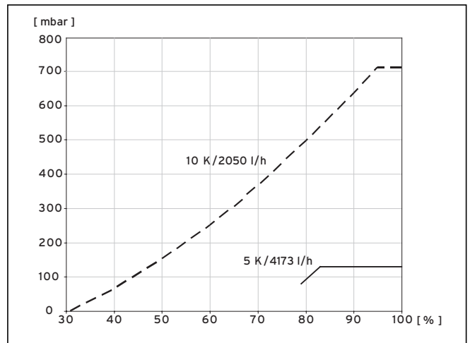
Abb. 9.10 Diagramm Leistungsoptimierung Heizkreispumpe VWW 171/3
