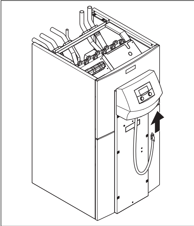
Abb. 7.19 eBUS-Leitung der Bedienkonsole anschließen
