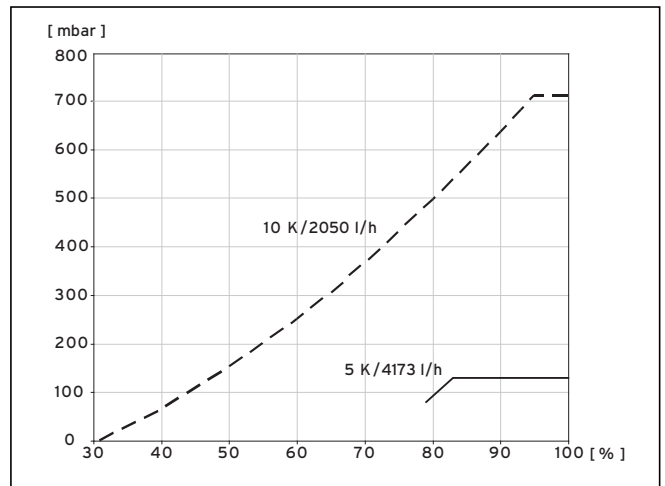
Abb. 9.10 Diagramm Drehzahloptimierung Heizkreispumpe VWW 171/3
