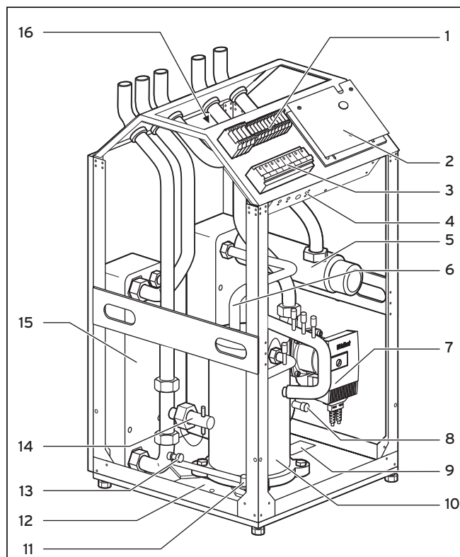
Abb. 3.6 Vorderansicht geöffnet (VWW)
