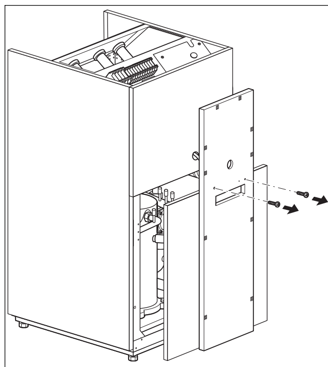
Abb. 4.8 Unterteil der Frontverkleidung abnehmen
