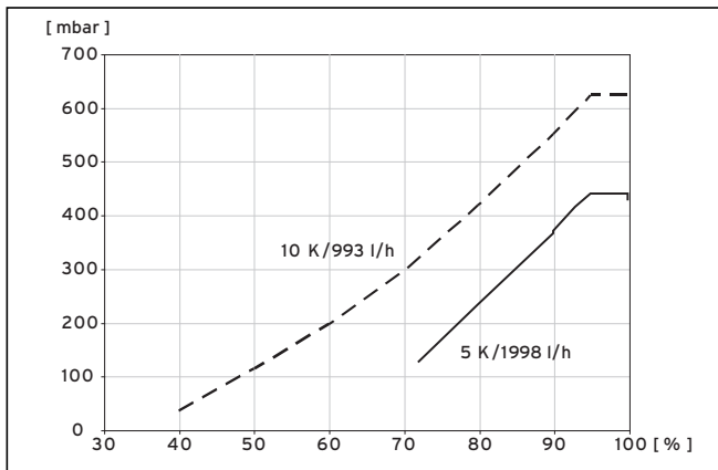
Abb. 9.7 Diagramm Drehzahloptimierung Heizkreispumpe VWW 81/3
