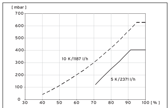
Abb. 9.9 Diagramm Drehzahloptimierung Heizkreispumpe VWS 141/3
