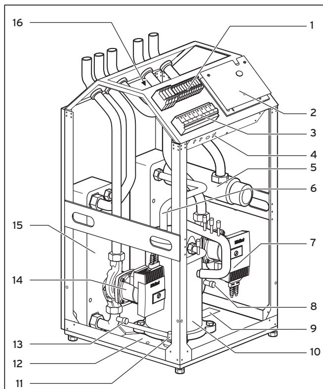
Abb. 3.5 Vorderansicht geöffnet (VWS)
