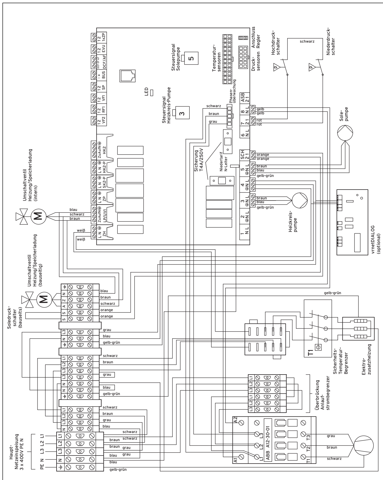
Abb. 3, Anhang, Stromlaufplan VWS ..1/3
