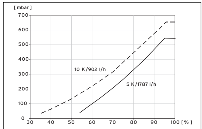
Abb. 9.8 Diagramm Drehzahloptimierung Heizkreispumpe VWS 101/3
