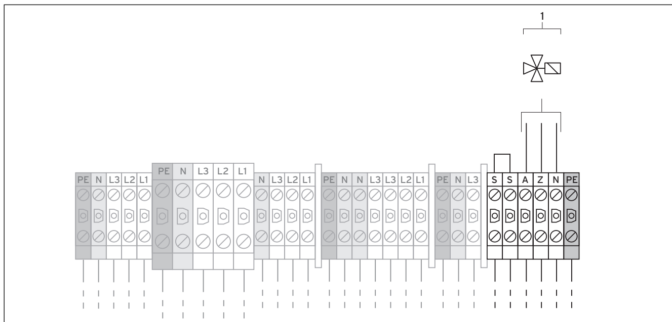
Abb. 7.7 Externes Umschaltventil für Pufferspeicher anschließen
