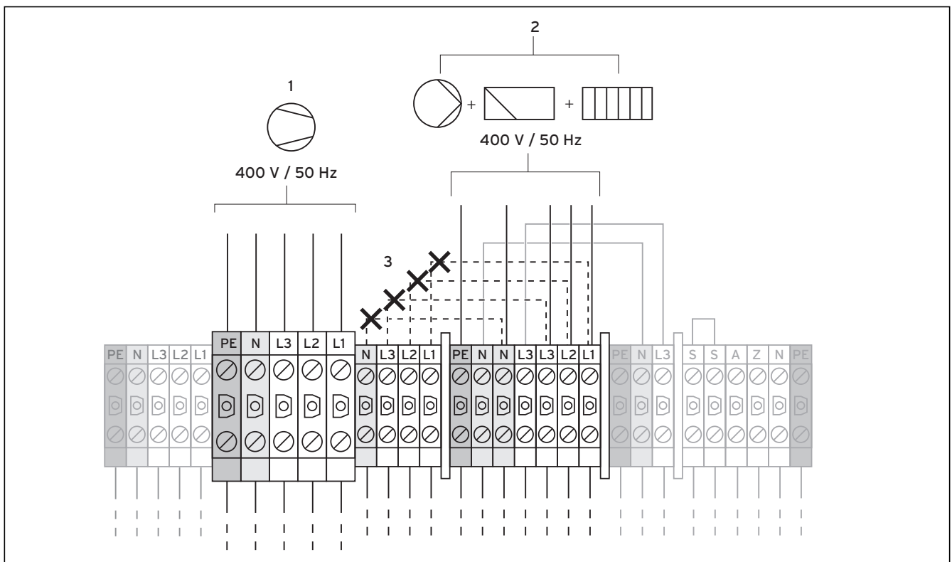
Abb. 7.3 Zweikreis-Einspeisung Wärmepumpen-Tarif
