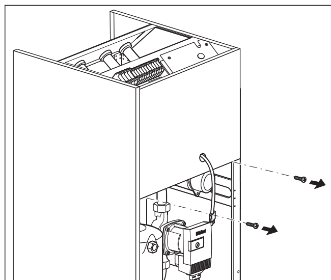
Abb. 4.9 Oberteil der Frontverkleidung abnehmen
