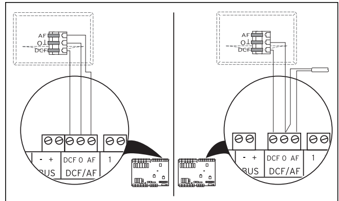
Abb. 7.11 VRC DCF-Empfänger anschließen
