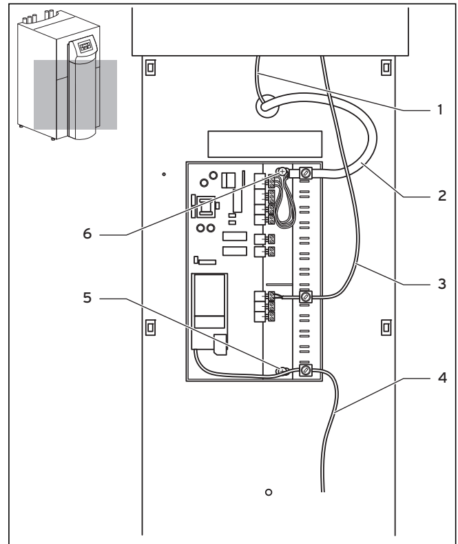
Abb. 7.22 vrnetDIALOG installieren
