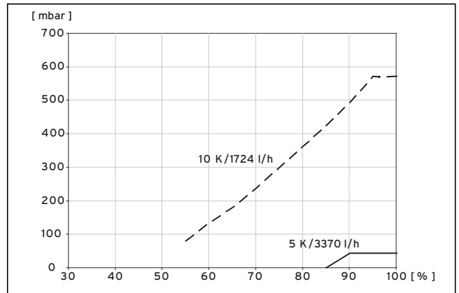
Abb. 9.9 Diagramm Drehzahloptimierung Heizkreispumpe VWW 141/3
