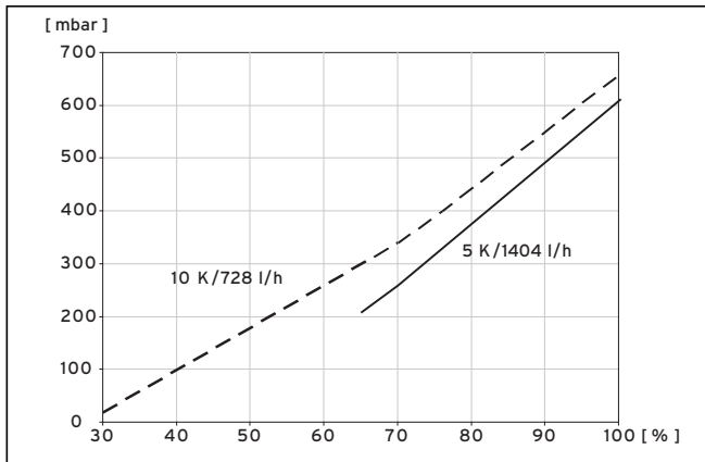
Abb. 9.6 Diagramm Drehzahloptimierung Heizkreispumpe VWW 61/3
