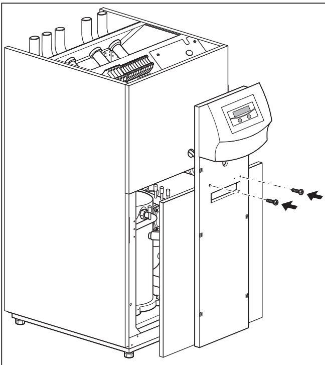
Abb. 7.18 Unterteil der Frontverkleidung montieren
