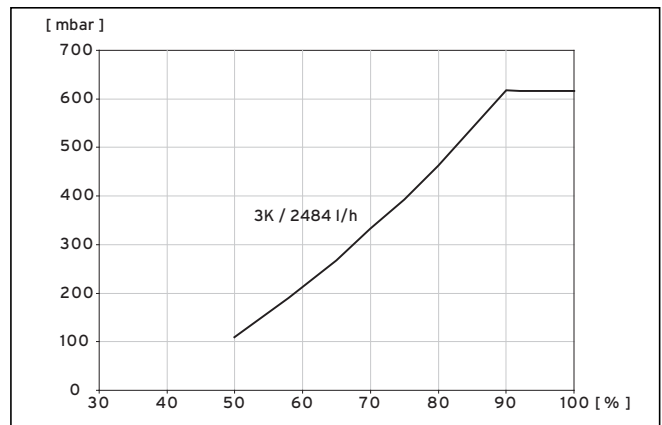
Abb. 9.3 Diagramm Drehzahloptimierung Solepumpe VWS 101/3
