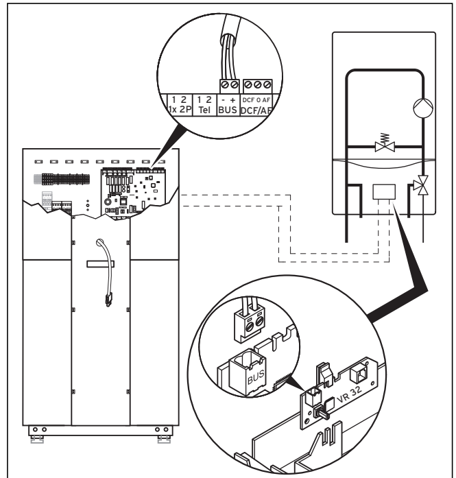
Abb. 7.14 Heizgerät mit eBUS-Schnittstelle anschließen
