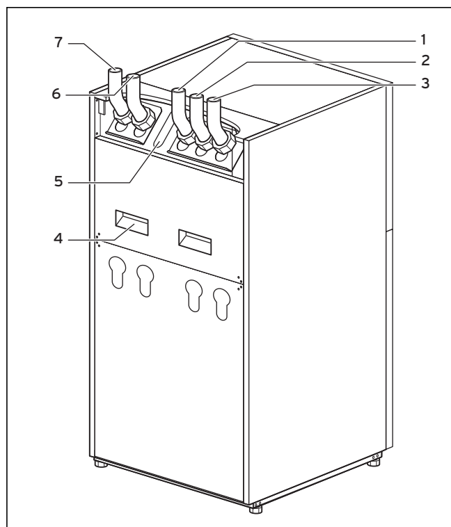
Abb. 3.4 Rückansicht
