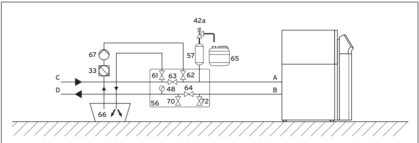
Abb. 6.6 Gesamten Solekreis in einem Arbeitsgang befüllen und entlüften
