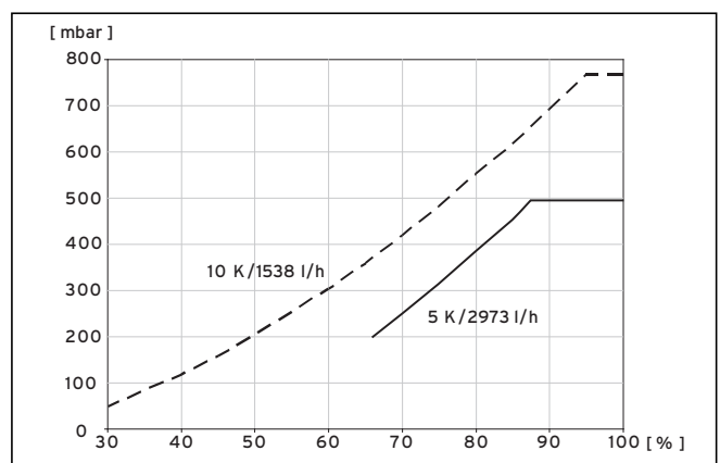
Abb. 9.10 Diagramm Drehzahloptimierung Heizkreispumpe VWS 171/3
