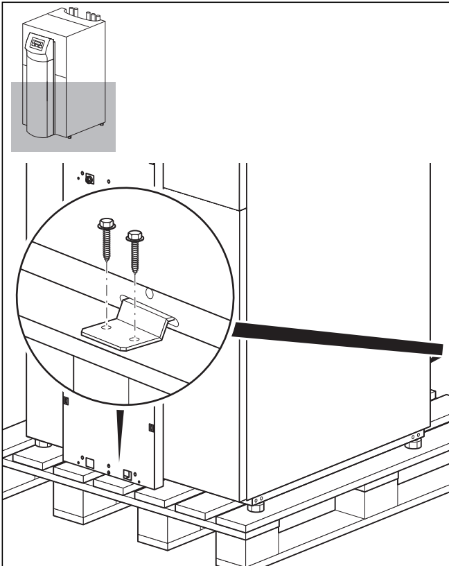
Abb. 4.4 Transportsicherungen entfernen
