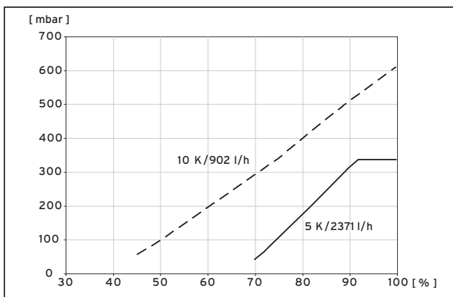
Abb. 9.8 Diagramm Drehzahloptimierung Heizkreispumpe VWW 101/3
