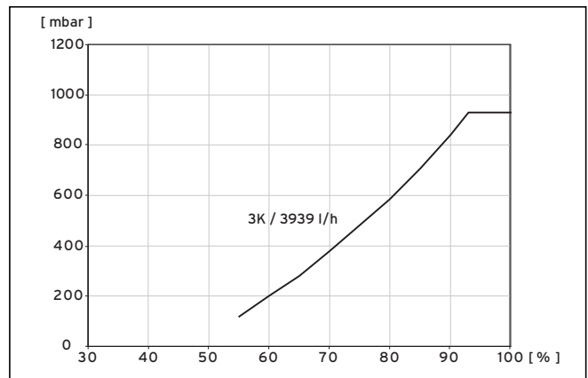
Abb. 9.5 Diagramm Drehzahloptimierung Solepumpe VWS 171/3
