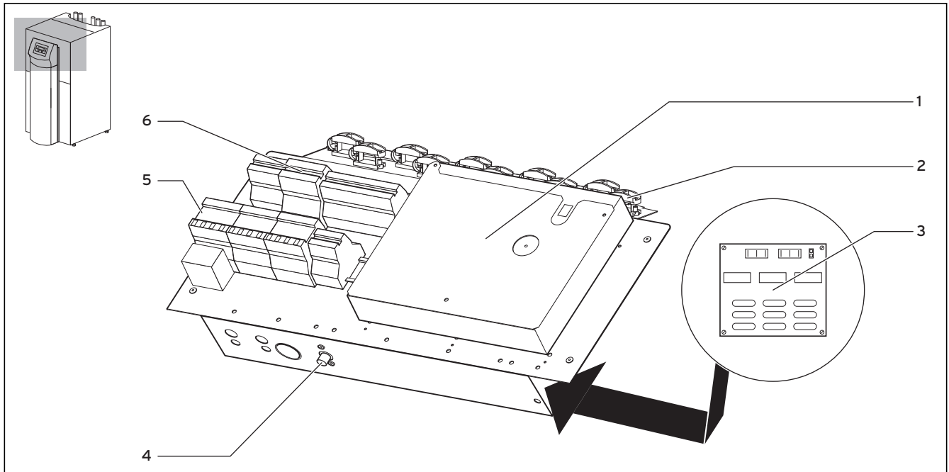
Abb. 7.1 Elektro-Schaltkasten
