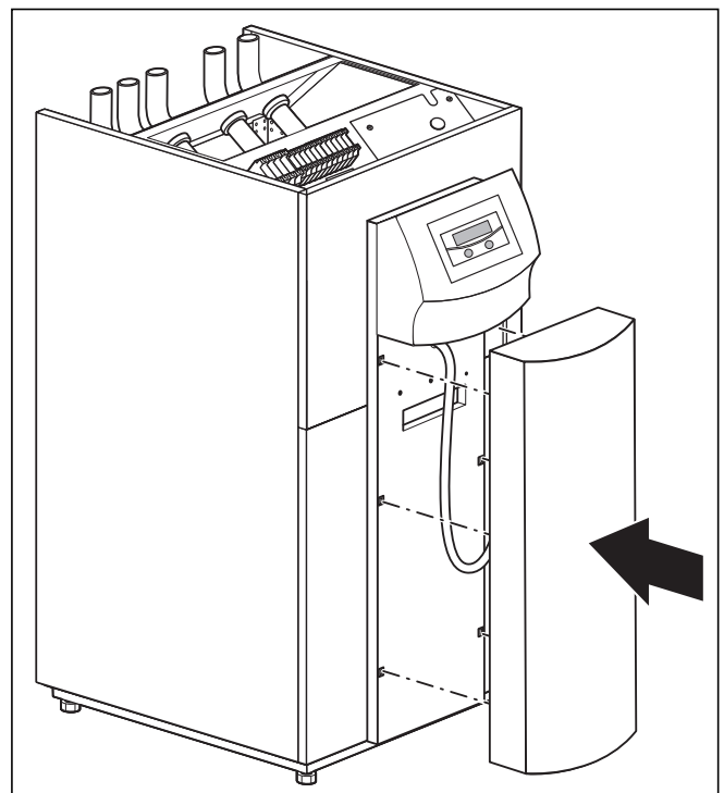
Abb. 7.20 Abdecksäule der Bedienkonsole montieren
