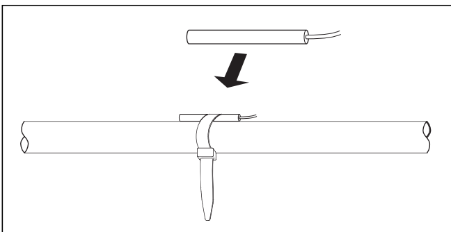
Abb. 7.10 Standardfühler VR 10 als Anlegefühler installieren
