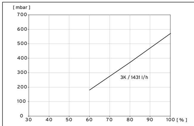
Abb. 9.1 Diagramm Drehzahloptimierung Solepumpe VWS 61/3
