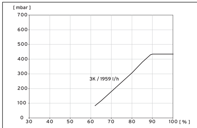
Abb. 9.2 Diagramm Drehzahloptimierung Solepumpe VWS 81/3
