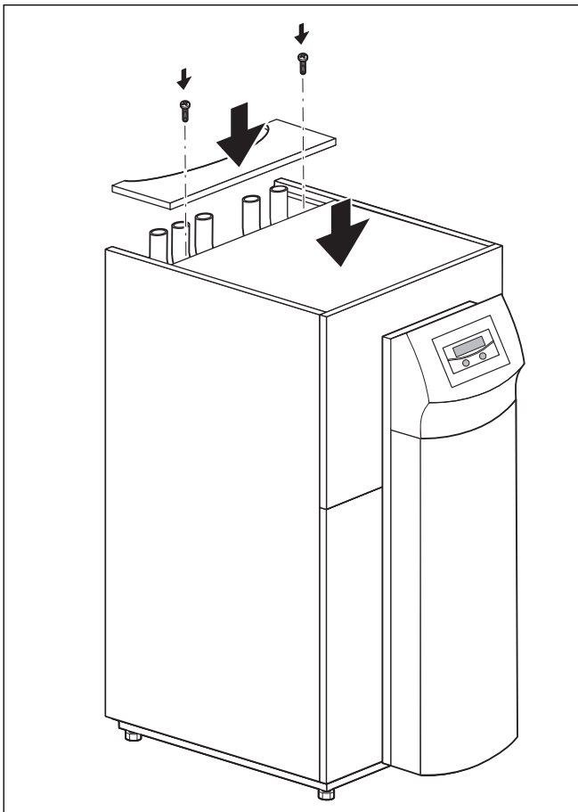
Abb. 7.21 Obere Verkleidungsteile montieren
