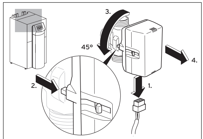
Abb. 6.3 Motorgehäuse des Umschaltventils abnehmen
