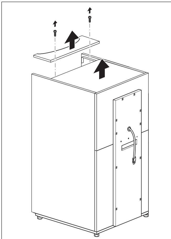
Abb. 4.7 Obere Abdeckungen abnehmen
