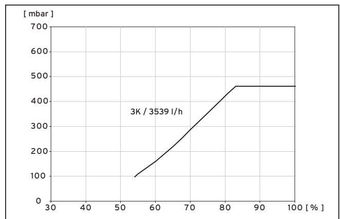
Abb. 9.4 Diagramm Drehzahloptimierung Solepumpe VWS 141/3
