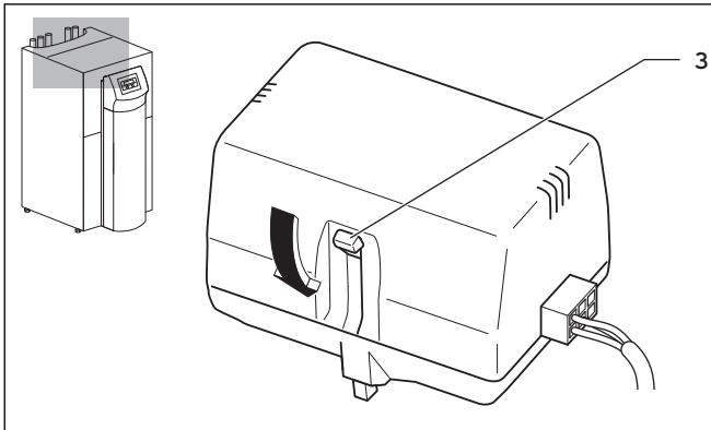
Abb. 6.2 Umschaltventil in Mittelstellung bringen
