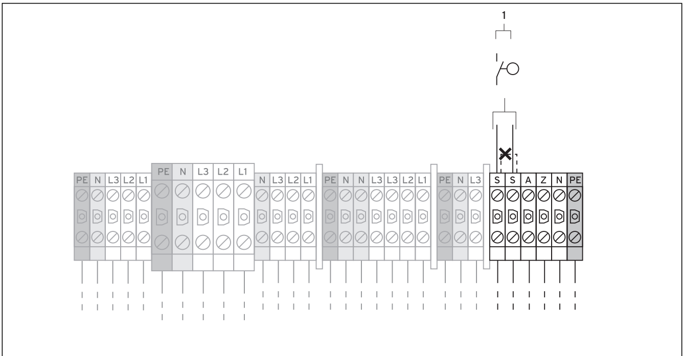
Abb. 7.6 Externen Soledruckschalter (nur VWS) und Maximalthermostaten anschließen
