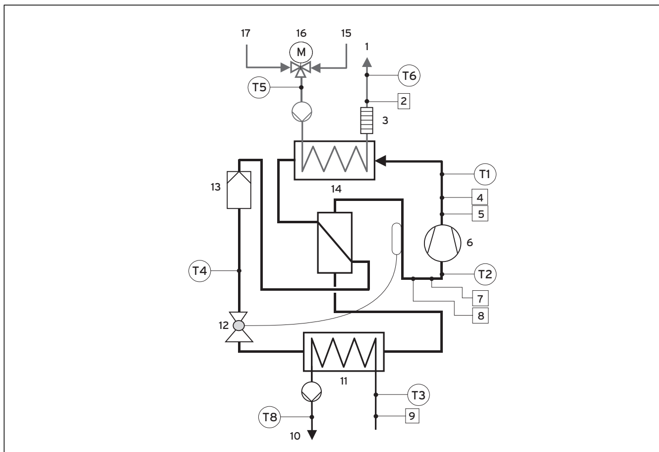
Abb. 1, Anhang, Wärmepumpenschema VWS ..1/3
