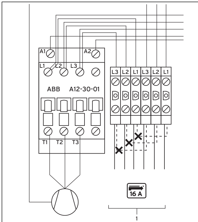
Abb. 7.8 Anlaufstrombegrenzer (Zubehör) anschließen
