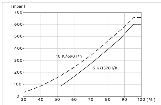
Abb. 9.7 Diagramm Drehzahloptimierung Heizkreispumpe VWS 81/3
