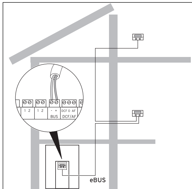
Abb. 7.12 Fernbediengeräte installieren
