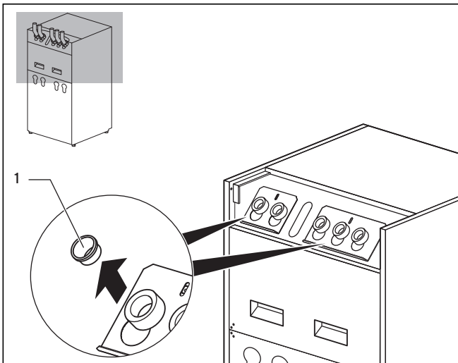
Abb. 5.5 Blindstopfen entfernen
