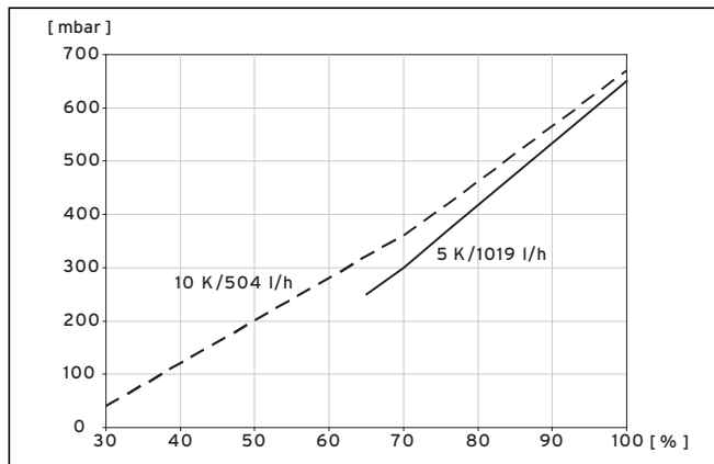
Abb. 9.6 Diagramm Drehzahloptimierung Heizkreispumpe VWS 61/3
