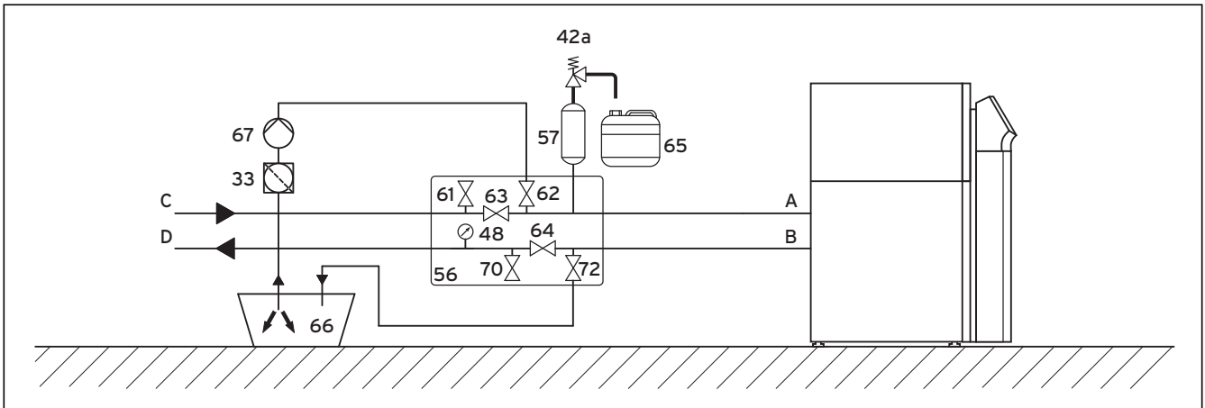
Abb. 6.5 Inneren Teil des Solekreises befüllen und entlüften
