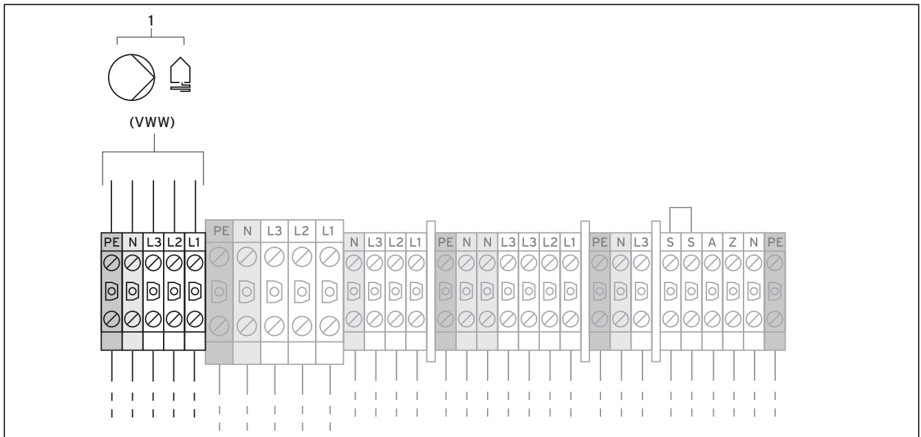
Abb. 7.5 Externen Brunnenpumpe anschließen (nur VWW)
