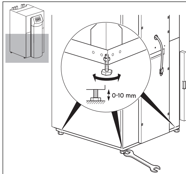
Abb. 4.6 Stellfüße einstellen
