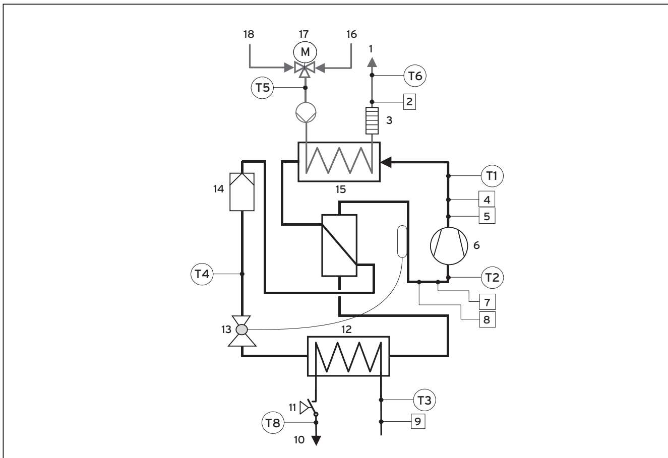
Abb. 2, Anhang, Wärmepumpenschema VWW ..1/3
