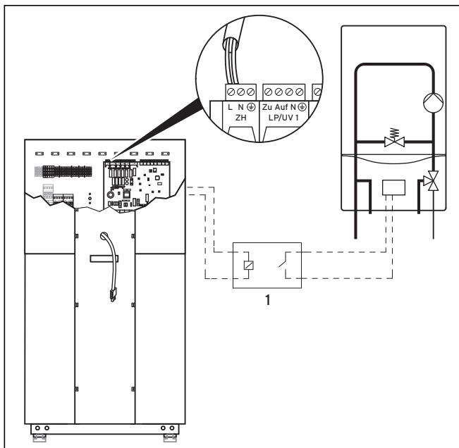
Abb. 7.15 Heizgerät ohne eBUS-Schnittstelle anschließen
