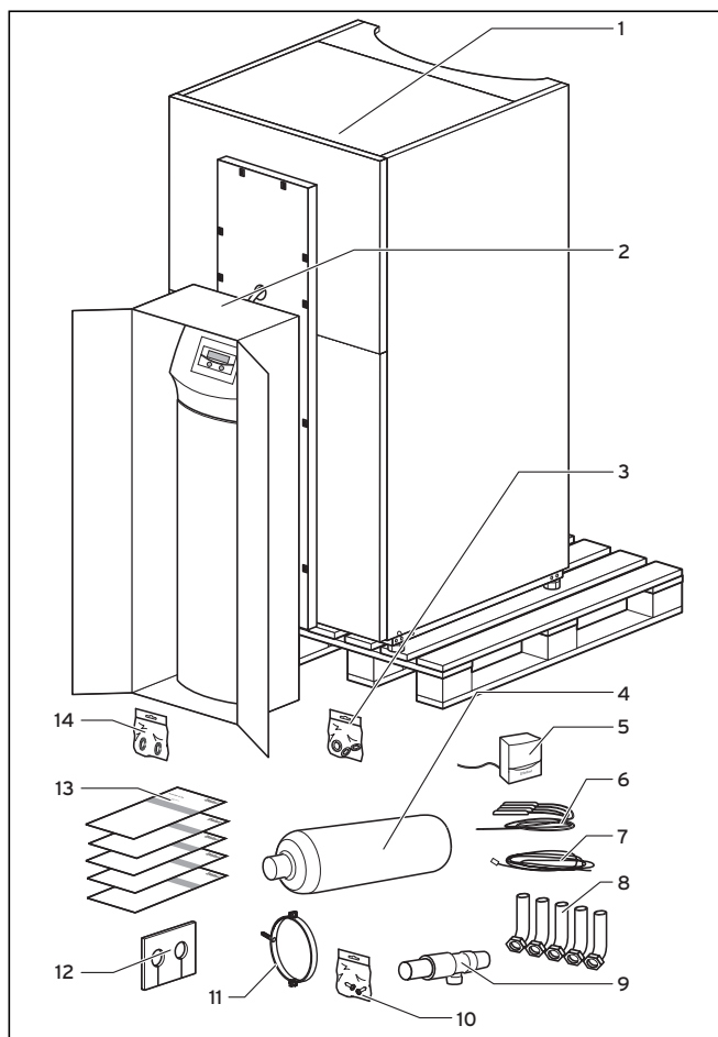
Abb. 4.3 Lieferumfang prüfen
