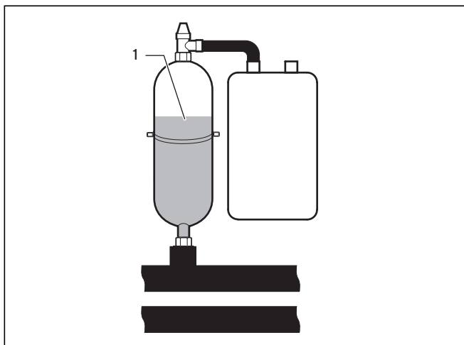
Abb. 6.7 Füllstand des Sole-Ausgleichsbehälters prüfen
