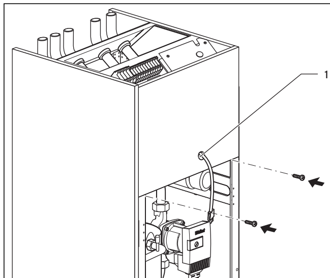
Abb. 7.16 Oberteil der Frontverkleidung montieren
