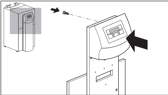
Abb. 7.17 Bedienkonsole montieren
