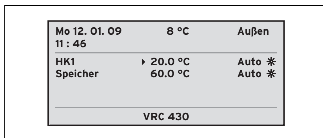
Abb. 6.5 Grundanzeige
