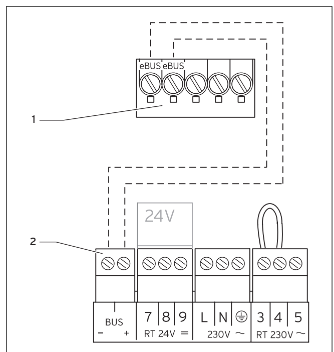
Abb. 5.3 Regler anschließen
