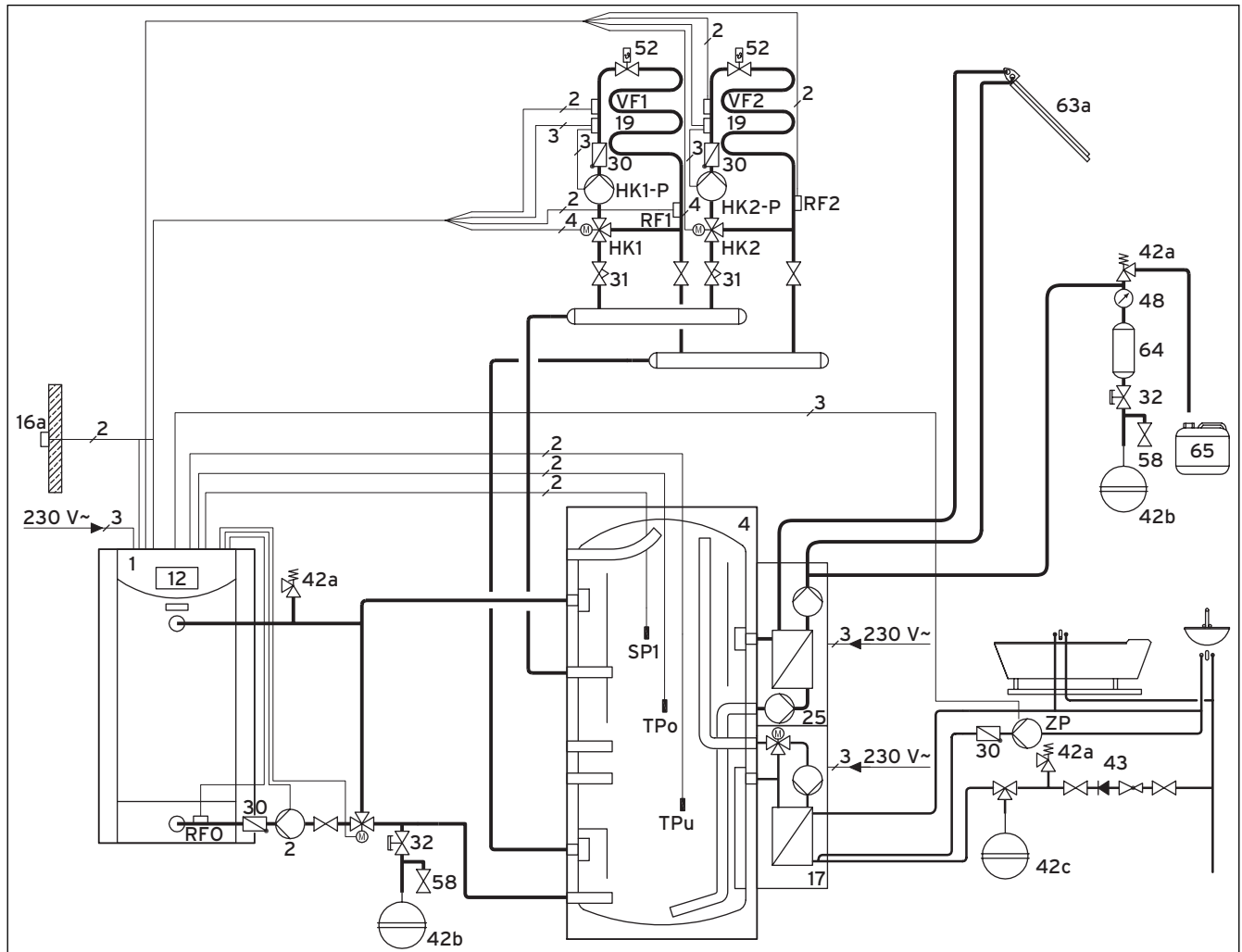
Abb. 6.21 Hydraulikplan 4
