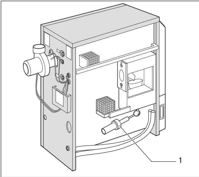
Abb. 9.14 Zündgebläse ausbauen
