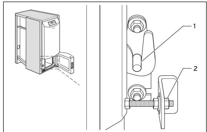
Abb. 9.13 Verschluss kontrollieren
