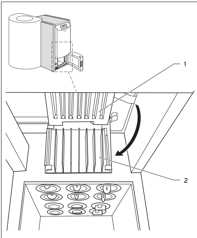
Abb. 9.12 Brennerrost reinigen
