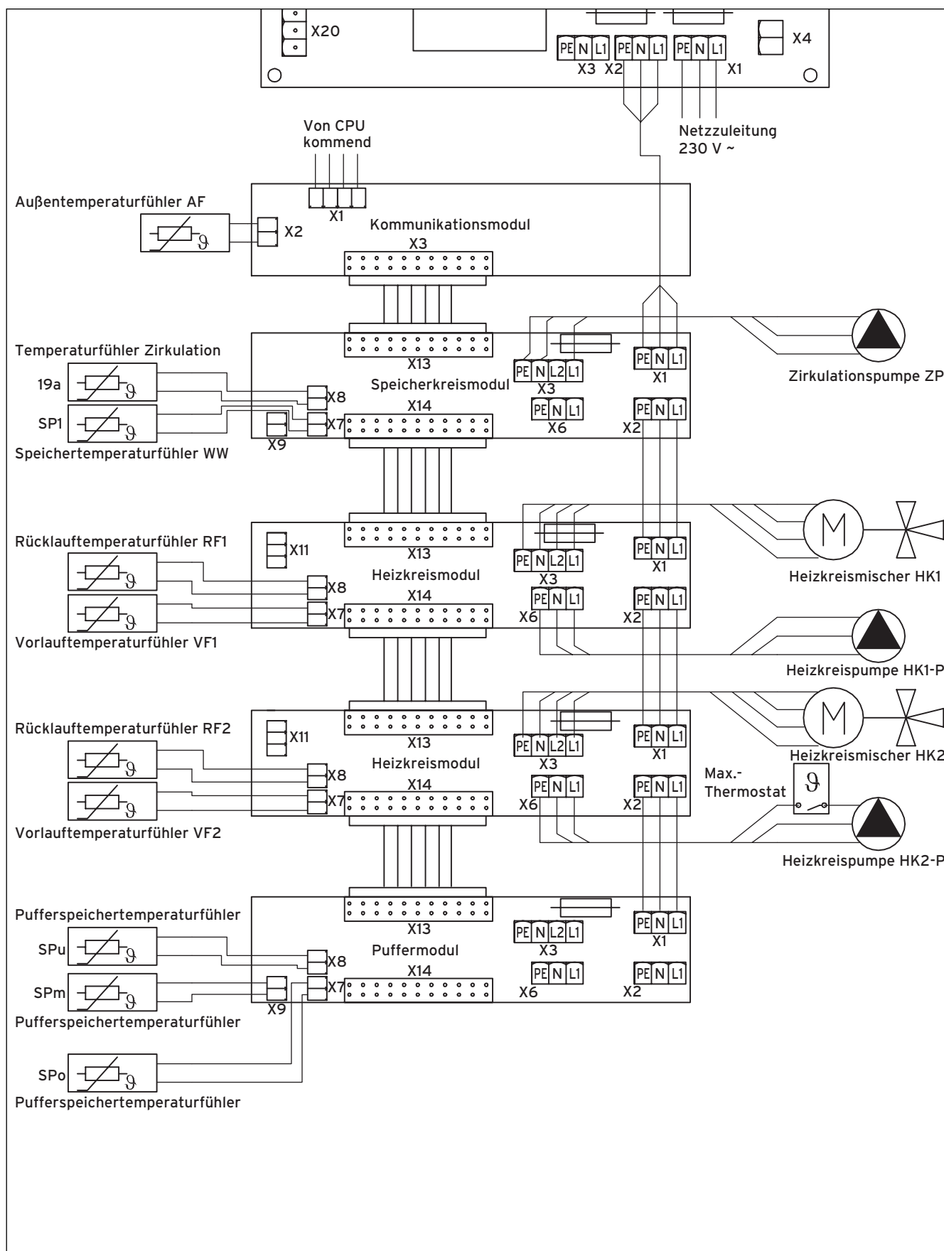
Abb. 6.24 Verdrahtungsplan 5
