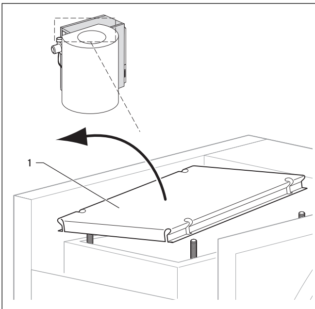
Abb. 9.2 Wärmetauscherdeckel (1) abheben
