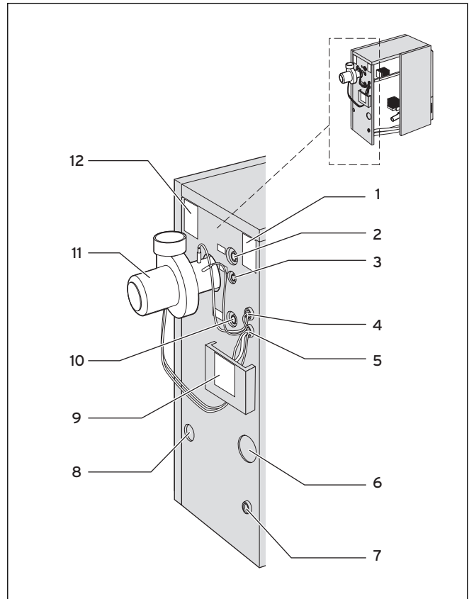
Abb. 5.1 Anschlüsse Rückseite
