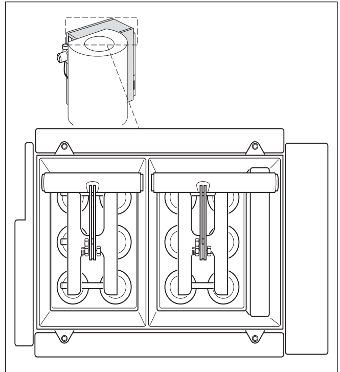
Abb. 9.3 Wärmetauscher
