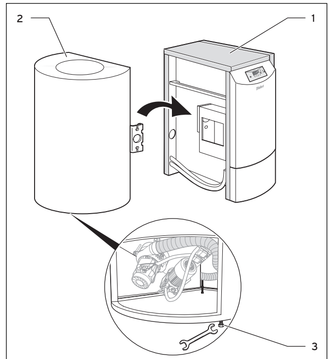
Abb. 4.12 Vorratsbehälter an Pellet-Heizkessel renerVIT montieren (hier Saugaustragung)
