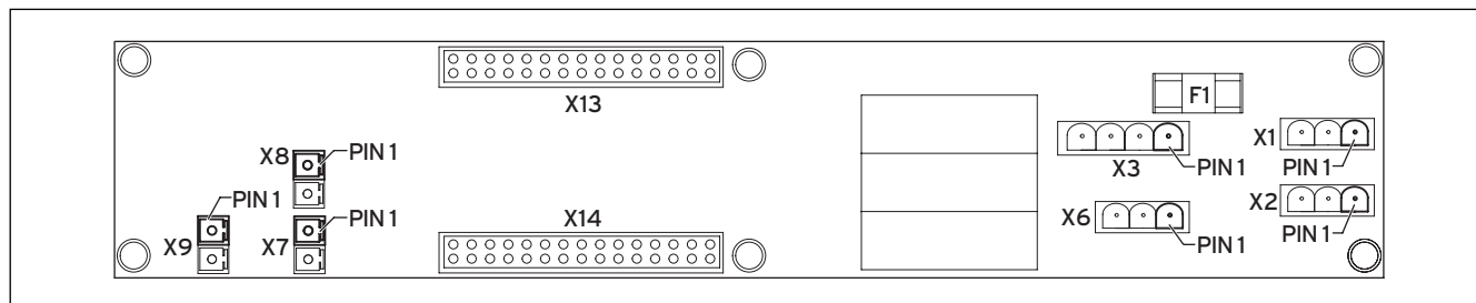
Abb. 6.14 Pufferspeichermodul
