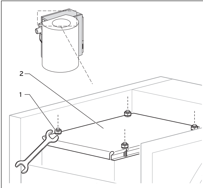
Abb. 9.1 Wärmetauscherdeckel aufschrauben
