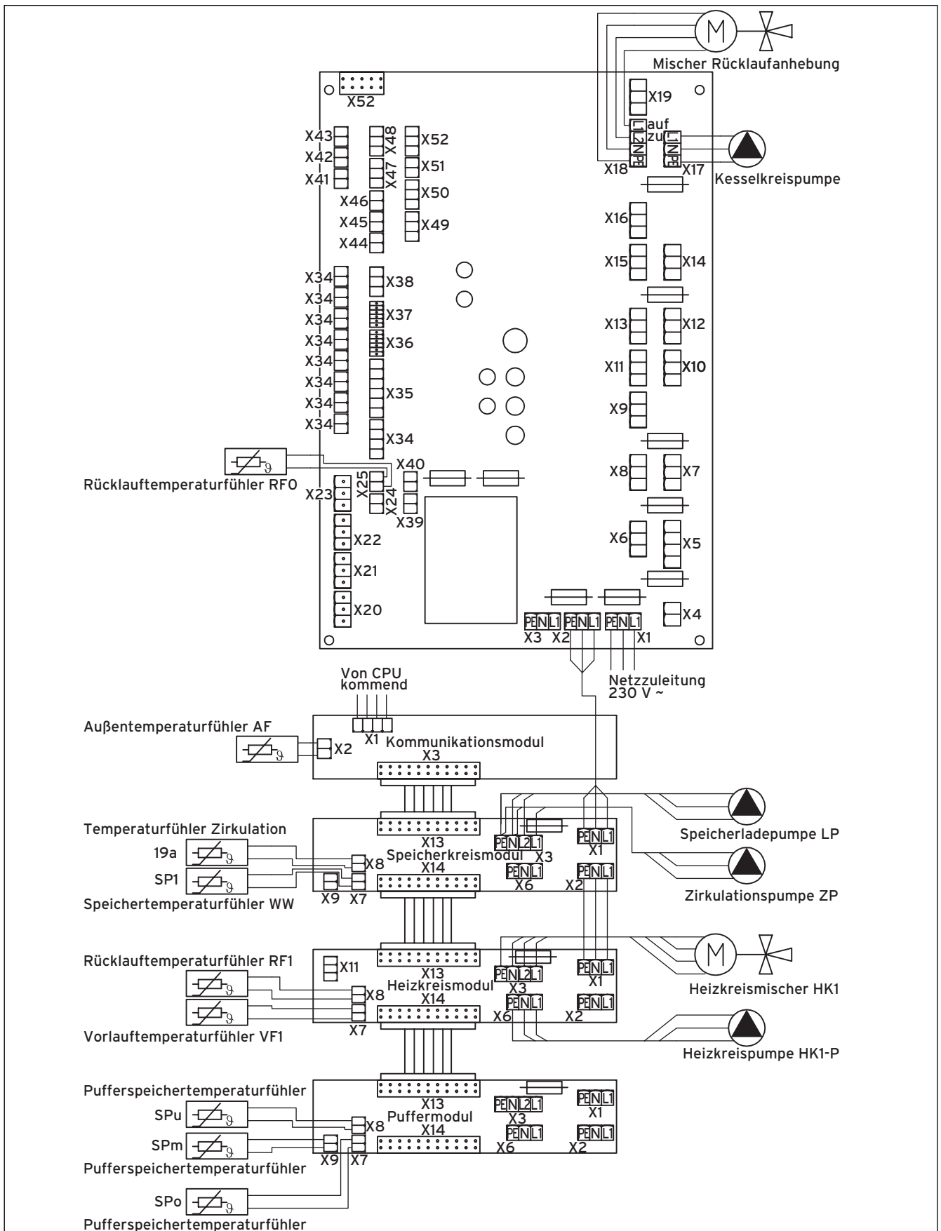
Abb. 6.16 Verdrahtungsplan 1
