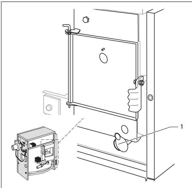
Abb. 9.17 Primärluftöffnung prüfen
