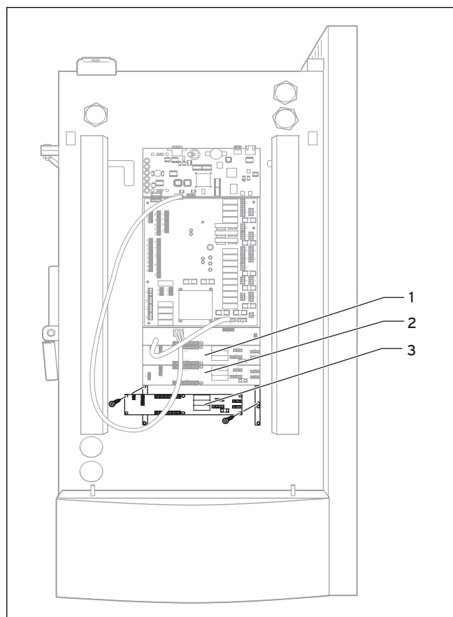
Abb. 6.13 Zubehörmodul anschließen
