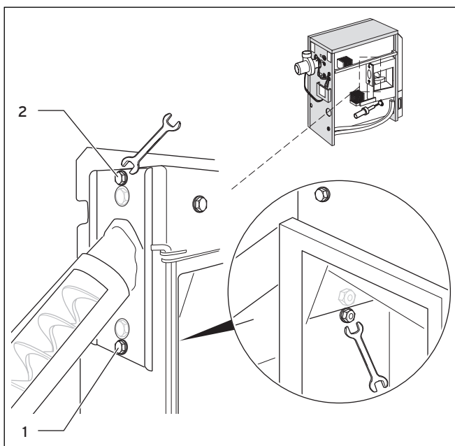
Abb. 4.13 Schrauben am Einschubflansch
