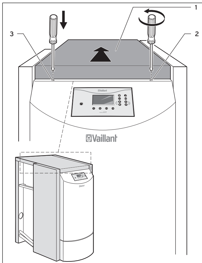
Abb. 10.1 Sicherheitstemperaturbegrenzer entriegeln
