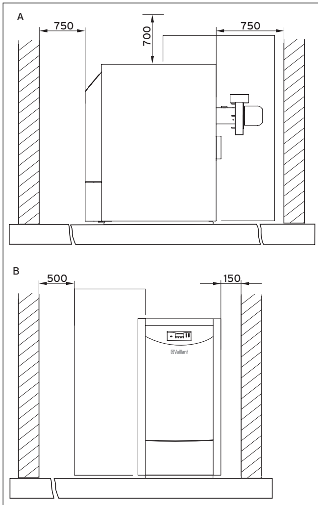
Abb. 4.3 Abmessungen des Pellet-Heizkessels renerVIT (in mm)
