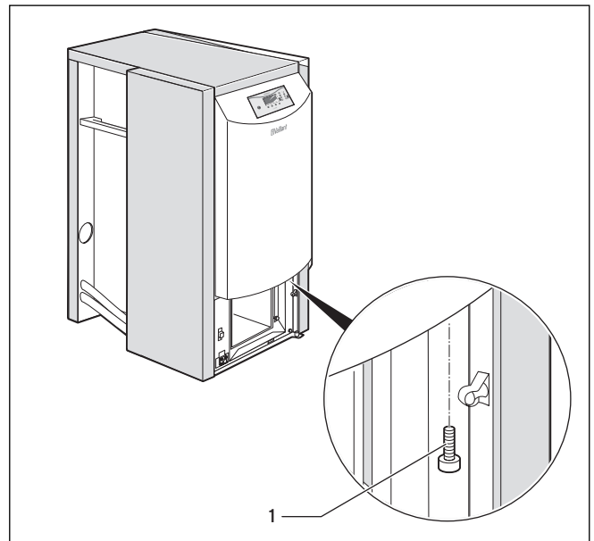
Abb. 4.4 Befestigungsschraube herausnehmen
