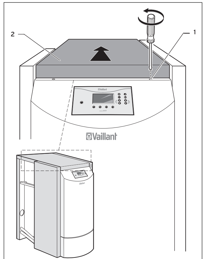
Abb. 4.8 Obere Verkleidung abnehmen
