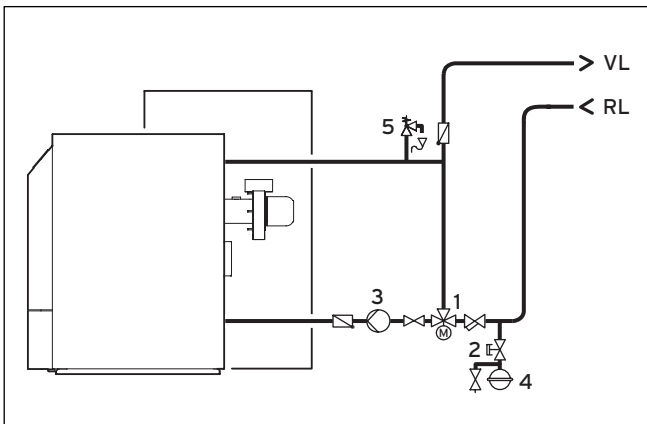
Abb. 5.2 Heizungsseitiges Anschlusschema
