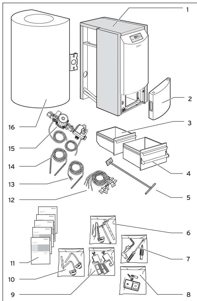
Abb. 4.2 Lieferumfang Pellet-Heizkessel
