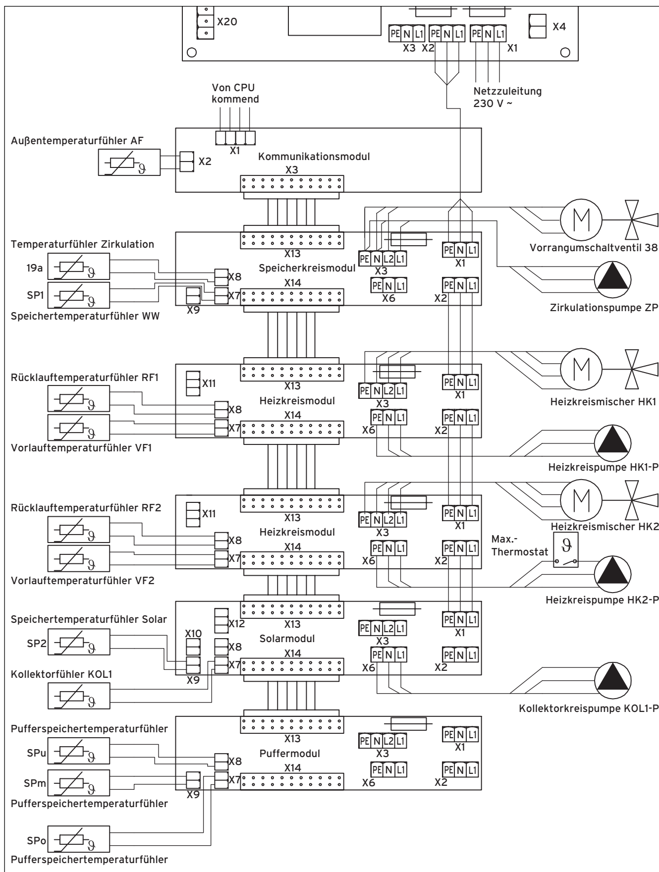
Abb. 6.20 Verdrahtungsplan 3
