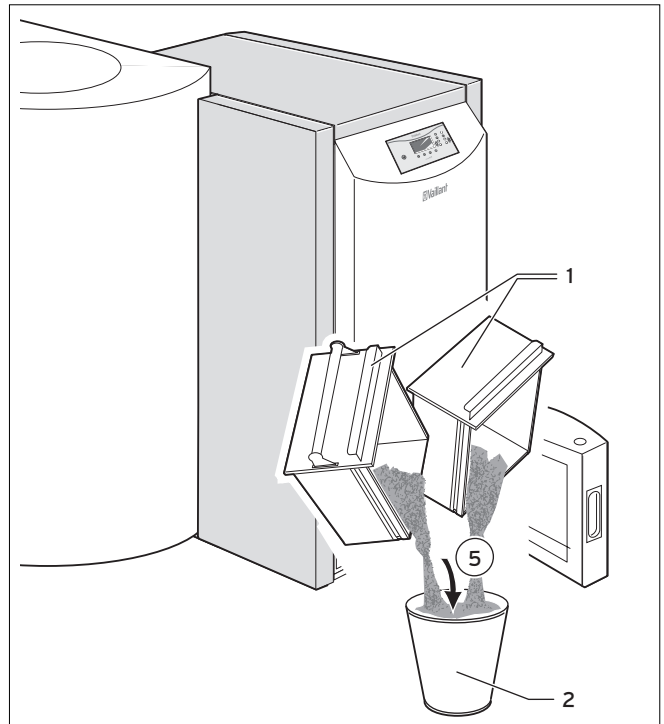
Abb. 9.11 Aschebehälter leeren
