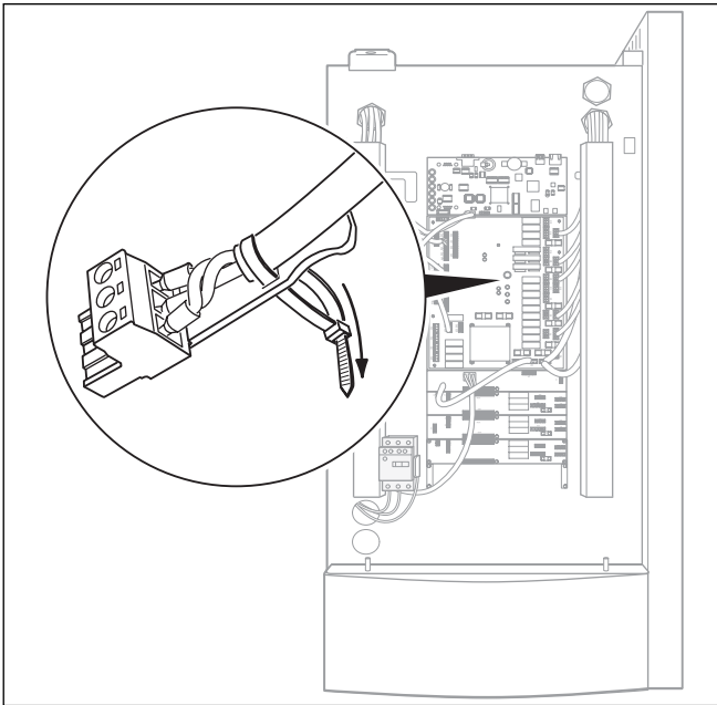
Abb. 6.6 Kabel an Zugentlastung mit Kabelbinder befestigen
