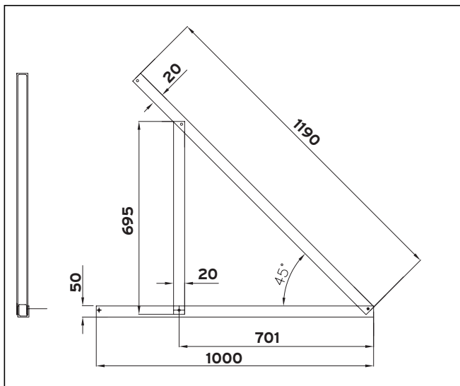
Abb. 7.5 Winkelträgeraufbau
