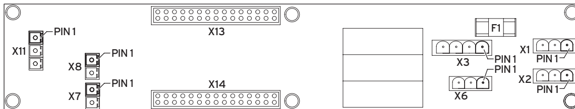
Abb. 6.12 Heizkreismodul
