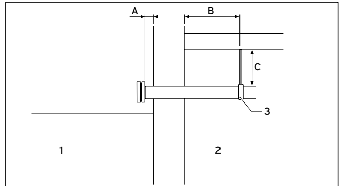
Abb. 7.4 Abstand zwischen Stützen und Unterkante Decke
