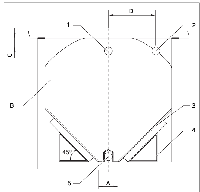
Abb. 7.1 Nutzbares Raumvolumen
