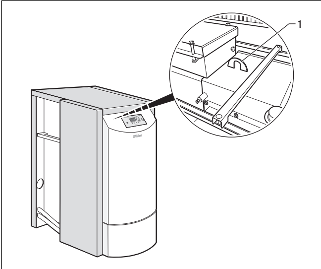
Abb. 4.7 Kranöse
