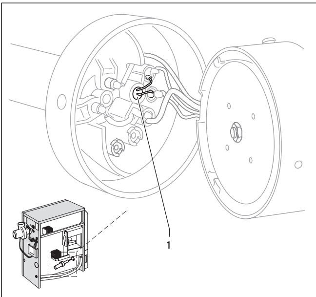
Abb. 9.15 Fotozelle reinigen
