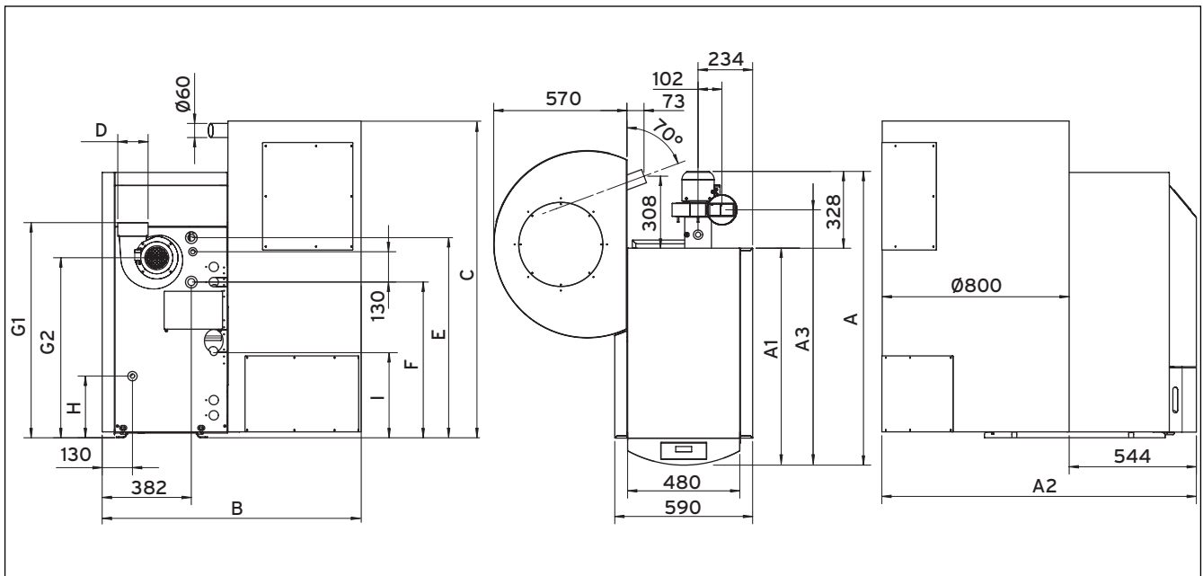
Abb.13.1 Abmessungen renerVIT
