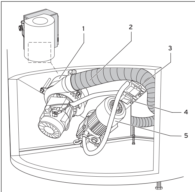
Abb. 6.2 Stromversorgung im Vorratsbehälter (hier Saugaustragung)
