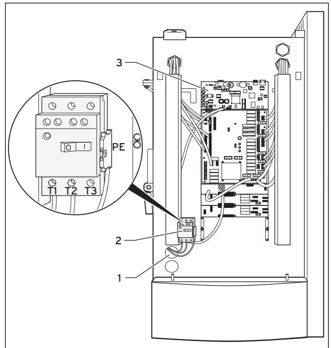
Abb. 6.3 Elektrischer Anschluss am Motorschutz für den Austragschneckenmotor (nur Saugaustragung)
