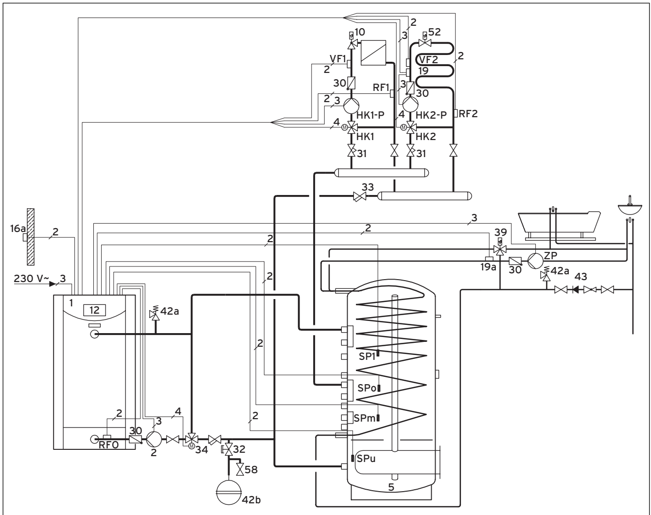
Abb. 6.23 Hydraulikplan 5
