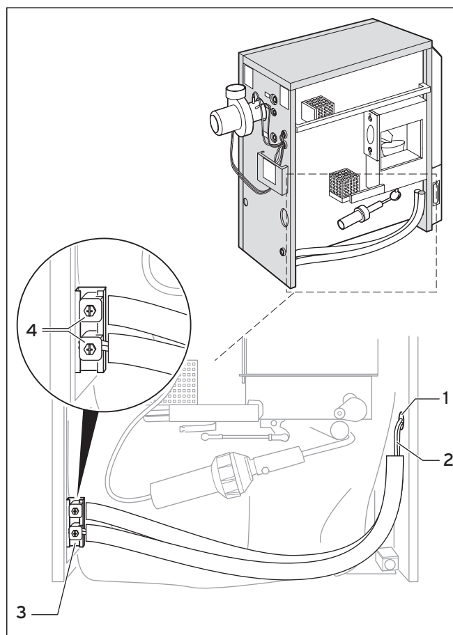
Abb. 6.1 Kabel verlegen
