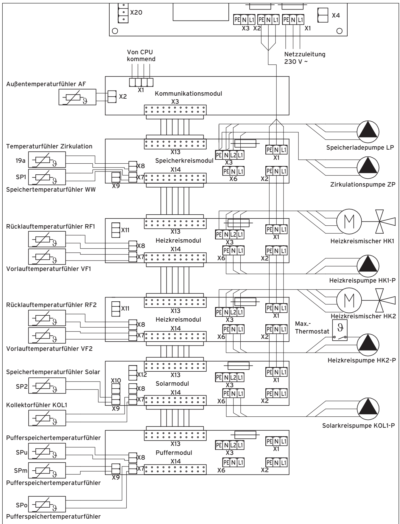
Abb. 6.18 Verdrahtungsplan 2
