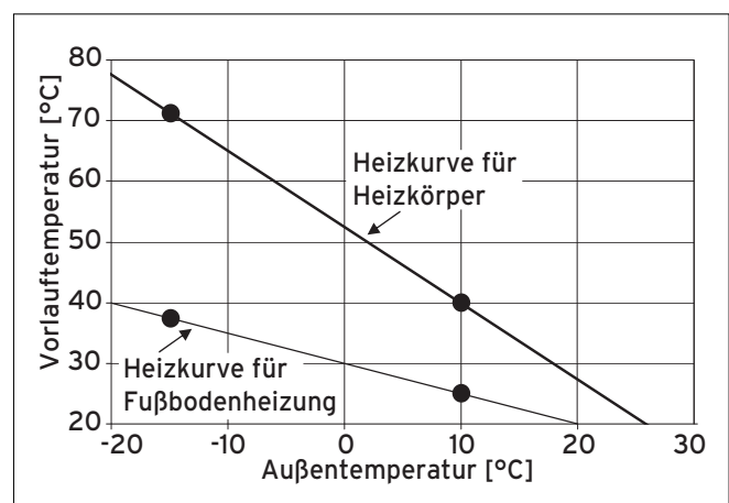
Abb. 8.3 Heizkurve (Beispiel)
