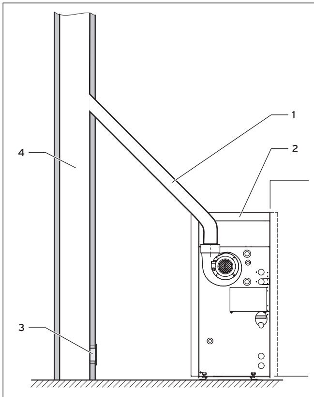
Abb. 5.4 Abgasführung (Beispiel)
