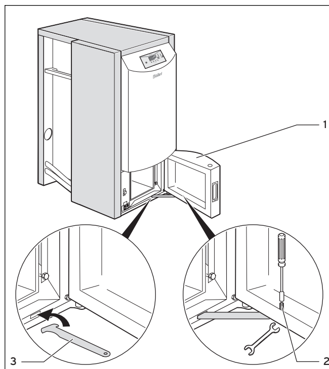
Abb. 4.6 Türstopper montieren
