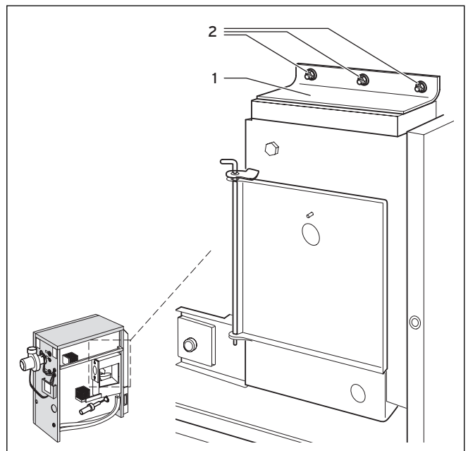
Abb. 9.16 Befestigungsschrauben festziehen
