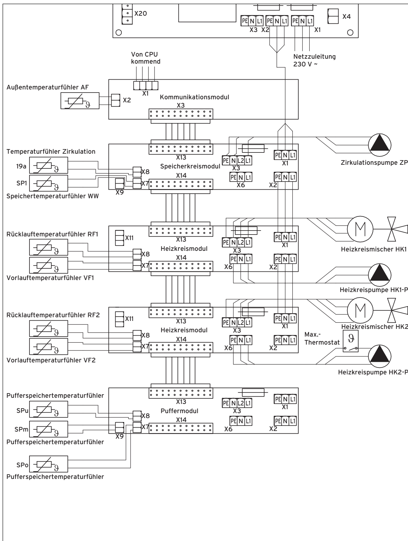
Abb. 6.22 Verdrahtungsplan 4
