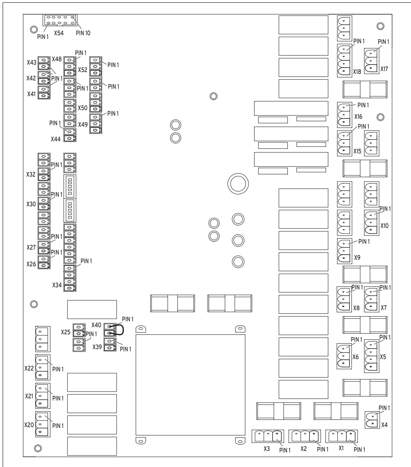
Abb. 6.9 Leiterplatte - Leistungsteil
