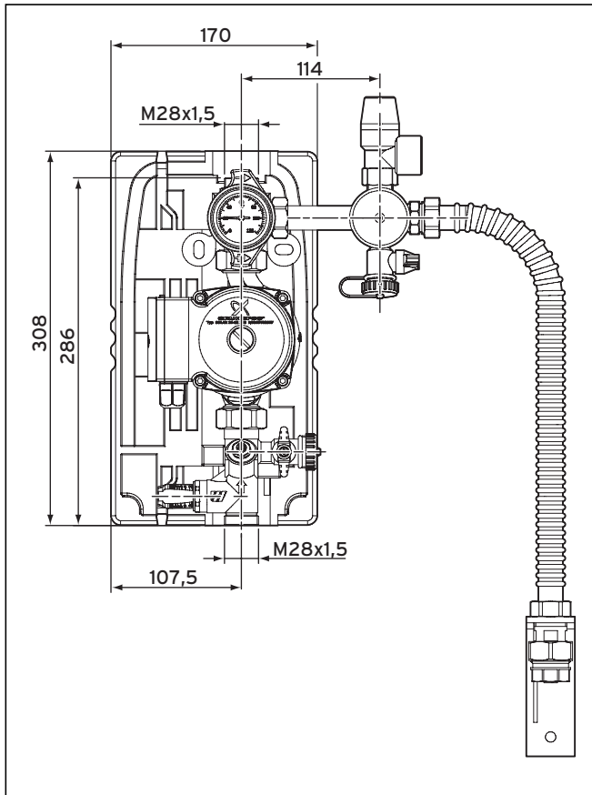
Abb. 10.1 Maße Einstrang-Solarstation
