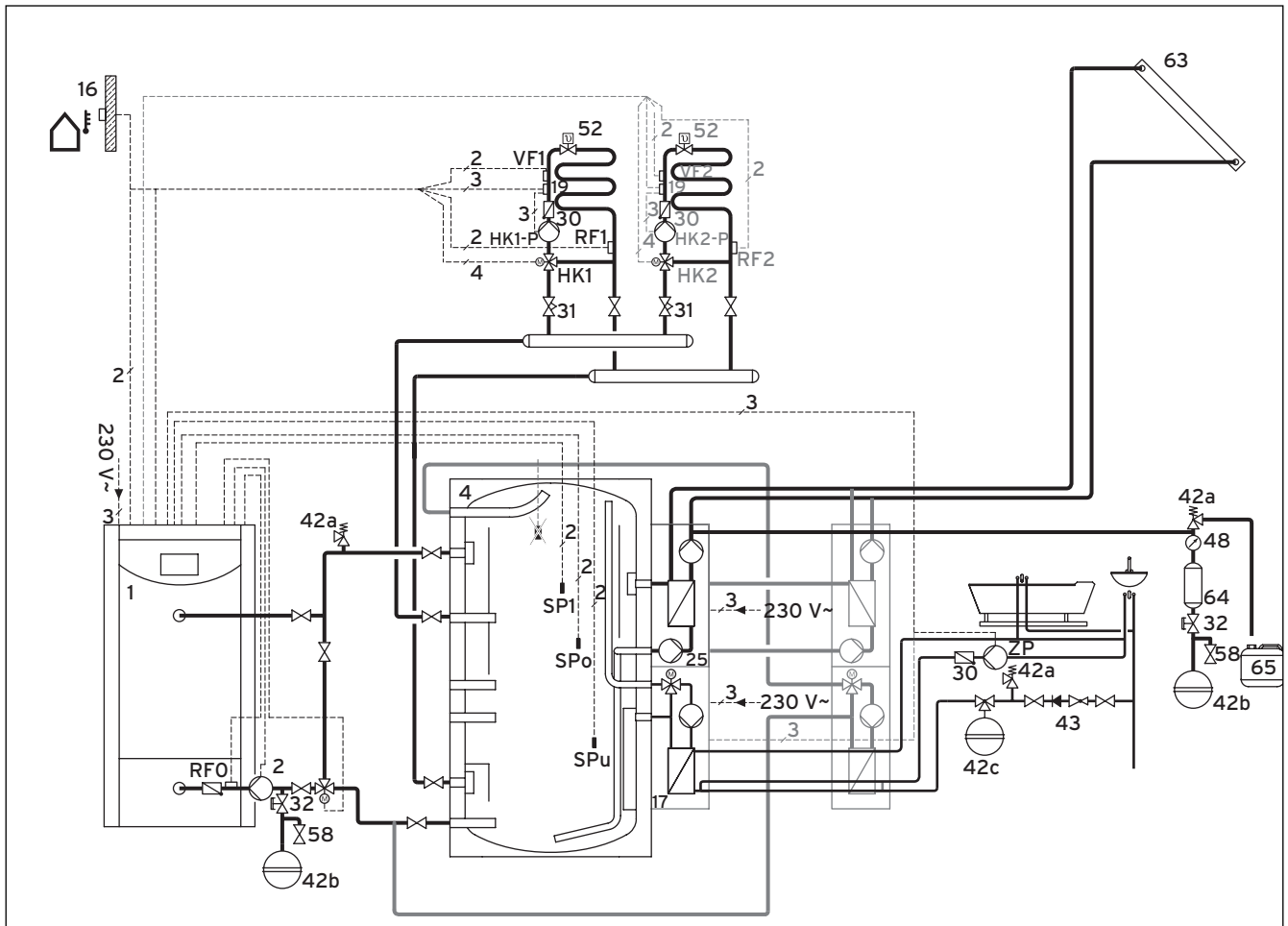
Abb. 3.10 Anschlussschema Pellet-Heizkessel
