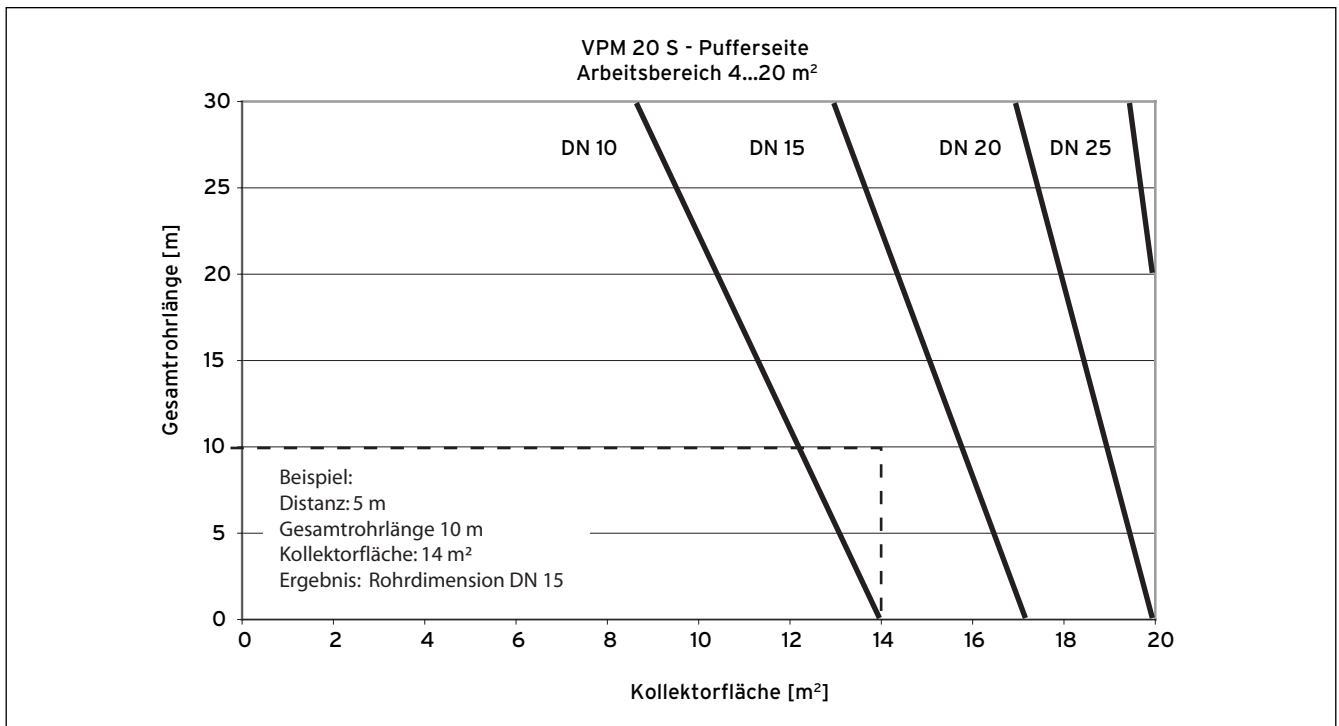
Abb. 3.16 Bestimmung Nenndurchmesser DN - VPM 20 S Pufferspeicherseite
