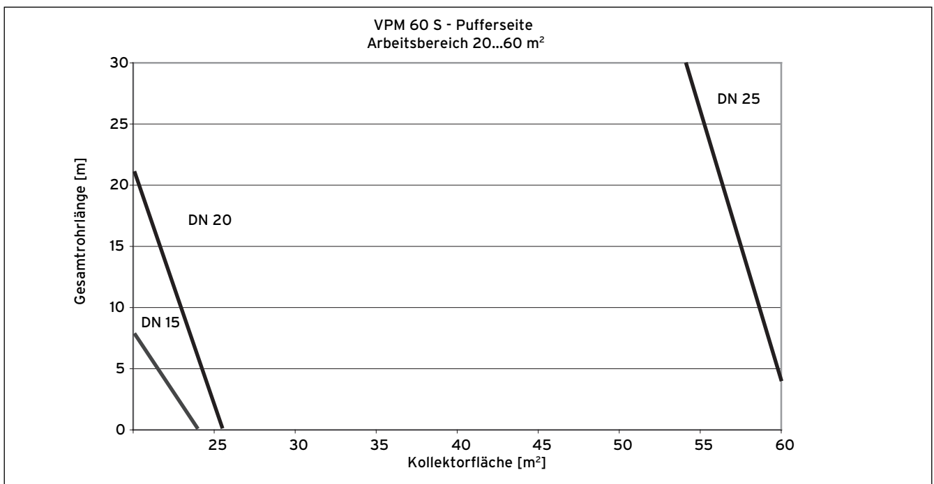
Abb. 3.17 Bestimmung Nenndurchmesser DN - VPM 60 S Pufferspeicherseite
