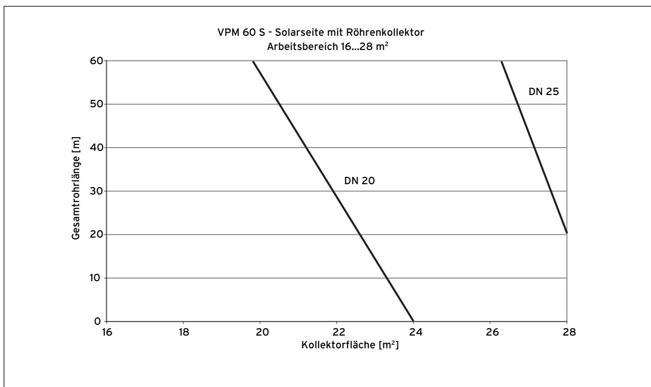
Abb. 3.19 Bestimmung Nenndurchmesser DN - VPM 60 S Solarseite mit Röhrenkollektoren
