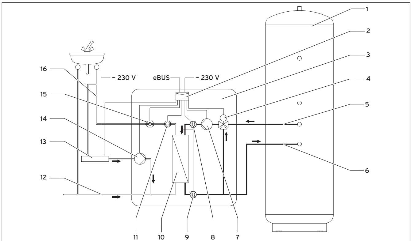
Abb. 3.5 Hydraulische Einbindung der Trinkwasserstation, Montage am Pufferspeicher VPS/2
