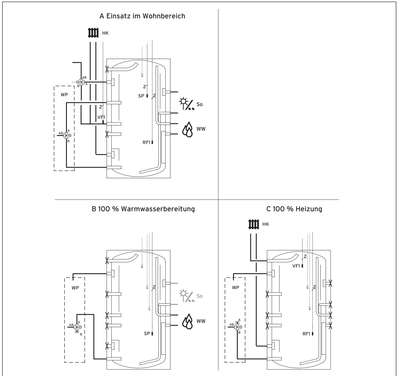
Abb. 3.13 Anwendungsbeispiele geoTHERM
