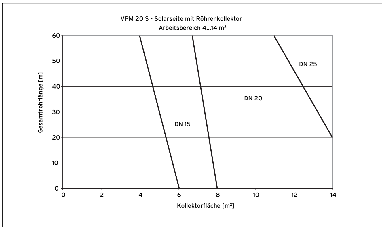
Abb. 3.18 Bestimmung Nenndurchmesser DN - VPM 20 S Solarseite mit Röhrenkollektoren
