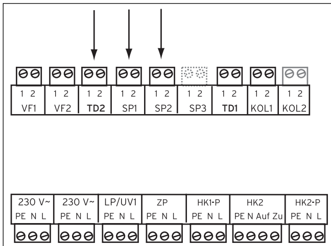
Abb. 4.3 Verdrahtung Solarsystemregler
