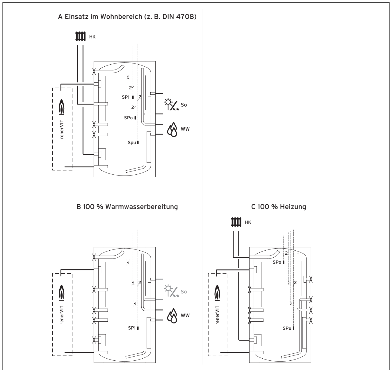
Abb. 3.12 Anwendungsbeispiel renerVIT
