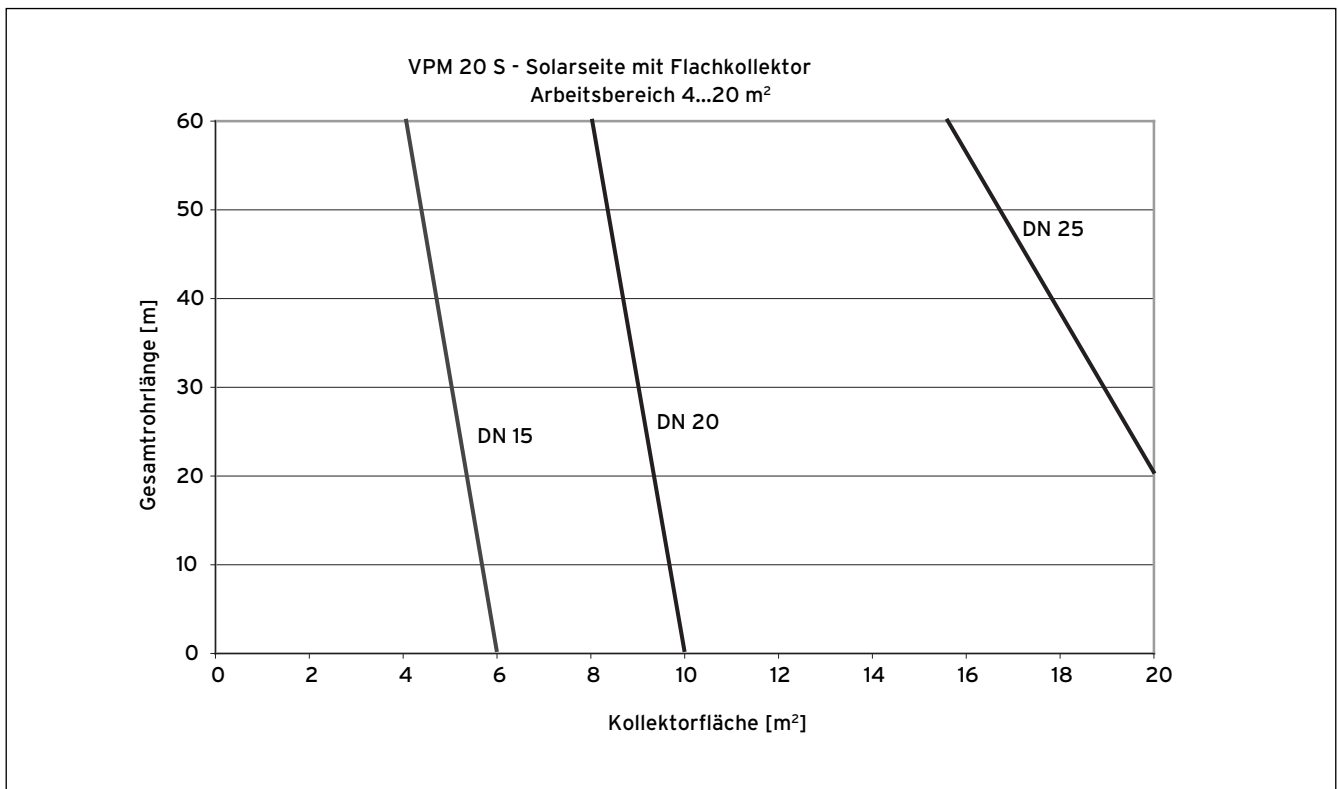
Abb. 3.20 Bestimmung Nenndurchmesser DN - VPM 20 S Solarseite mit Flachkollektoren
