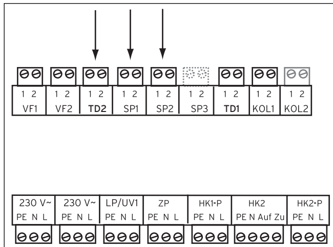
Abb. 4.3 Verdrahtung Solarsystemregler
