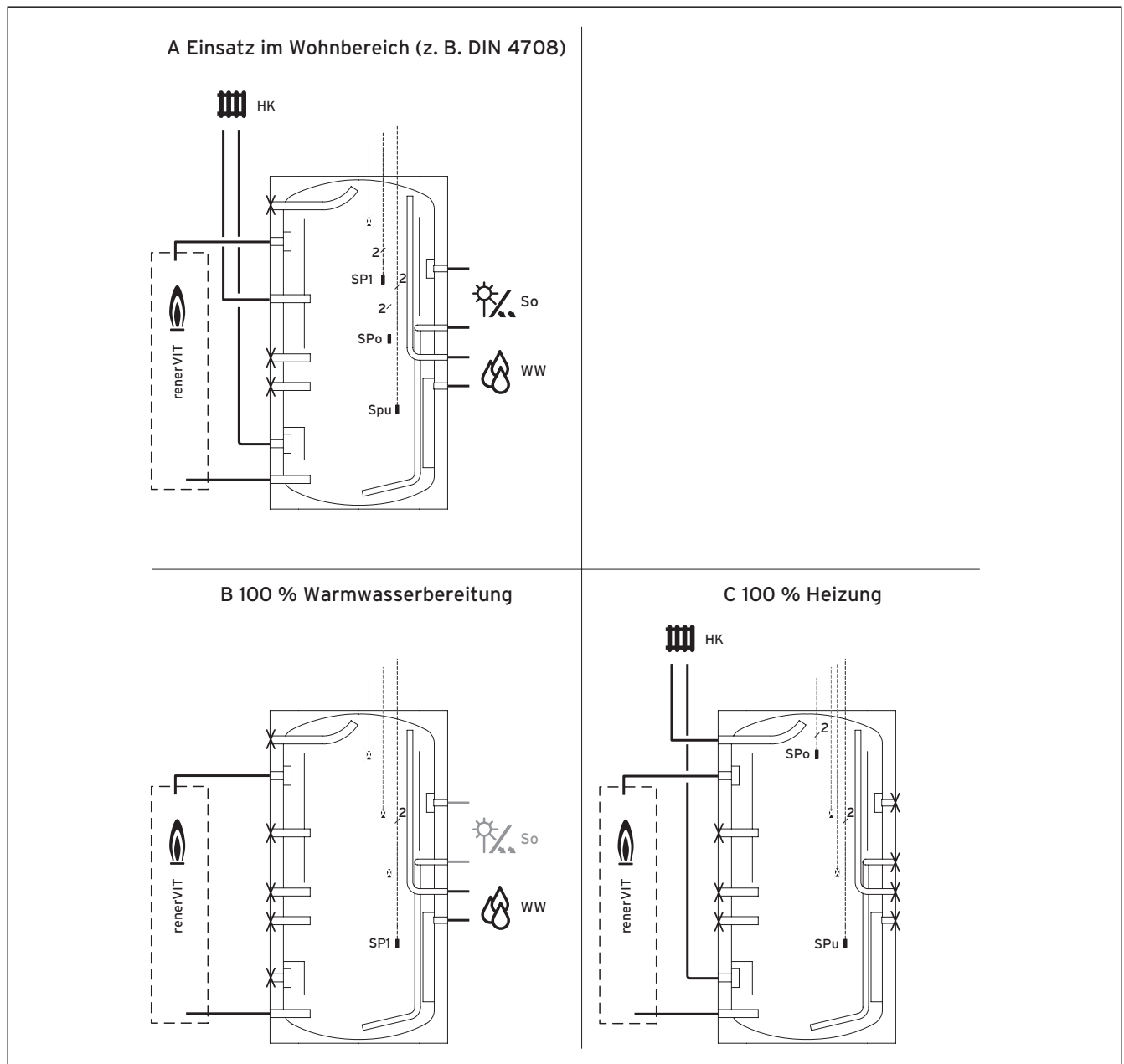
Abb. 3.12 Anwendungsbeispiel renerVIT
