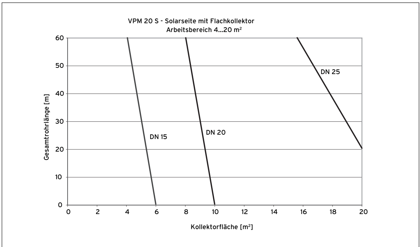
Abb. 3.20 Bestimmung Nenndurchmesser - VPM 20 S Solarseite mit Flachkollektoren
