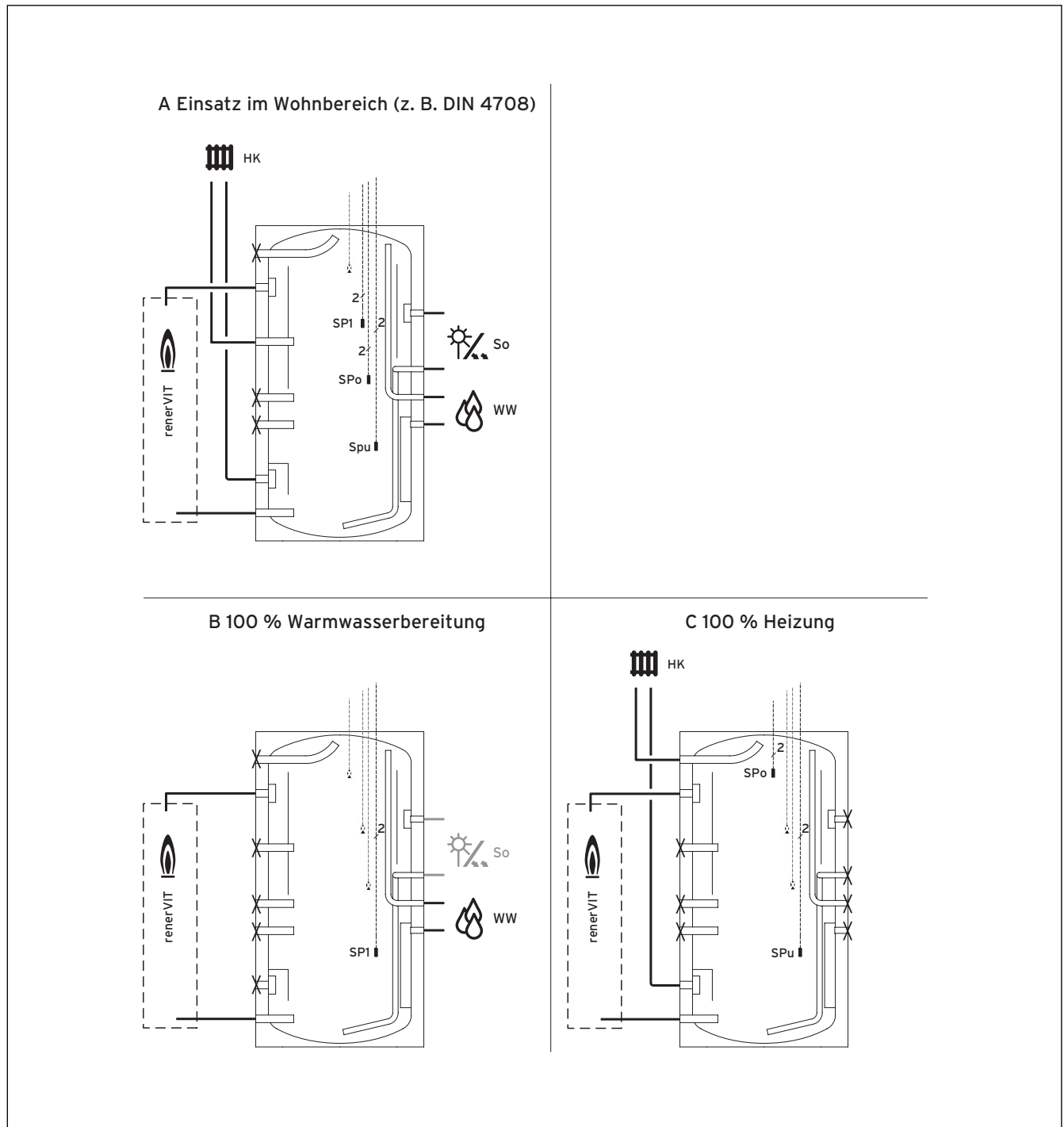
Abb. 3.12 Anwendungsbeispiel renerVIT
