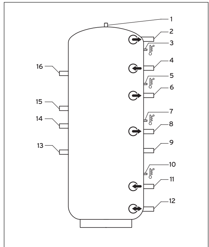
Abb 3.1 Anschlussschema Pufferspeicher VPS/2
