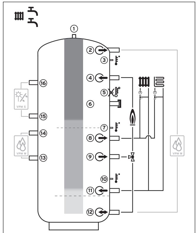
Abb. 3.3 Pufferspeicher VPS/2: Beispiel für Sportanwendung
