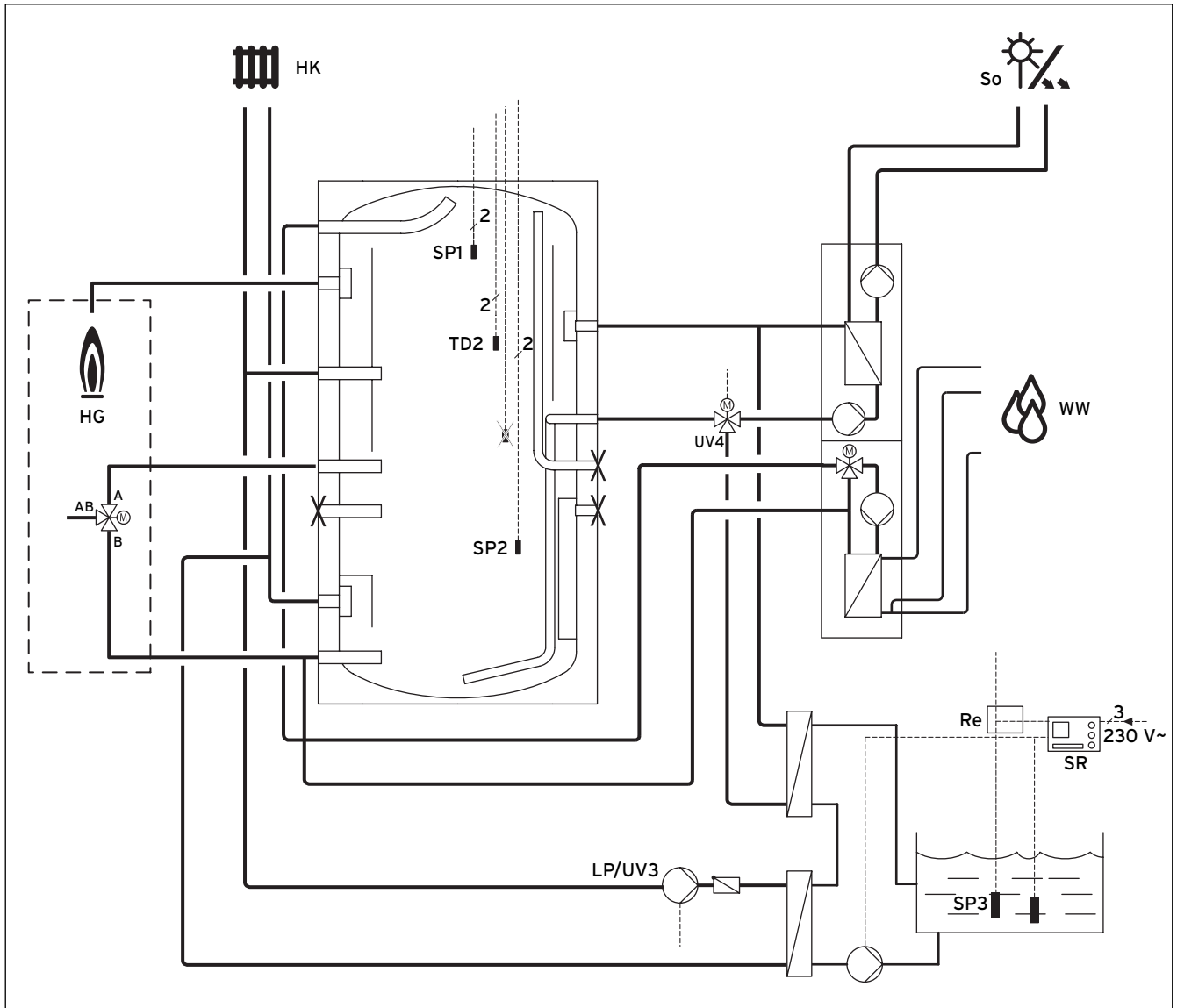
Abb. 3.14 Detail-Plan Schwimmbadbeheizung
