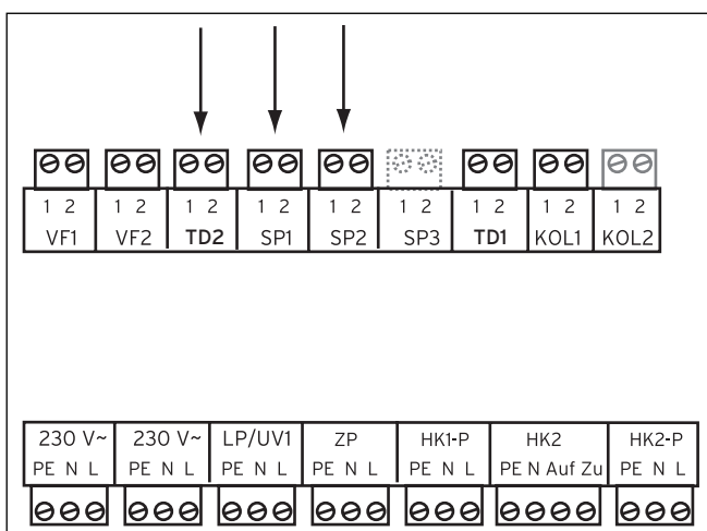
Abb. 4.3 Verdrahtung Solarsystemregler
