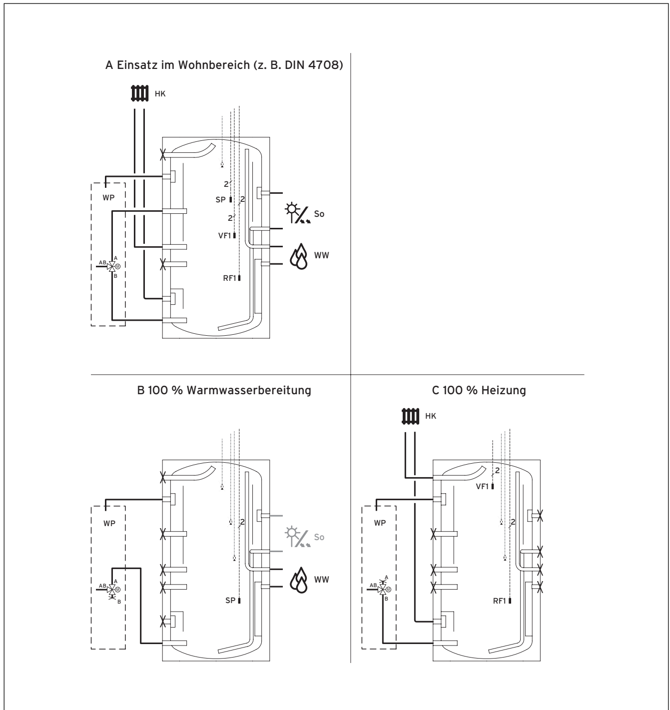
Abb. 3.13 Anwendungsbeispiele geoTHERM
