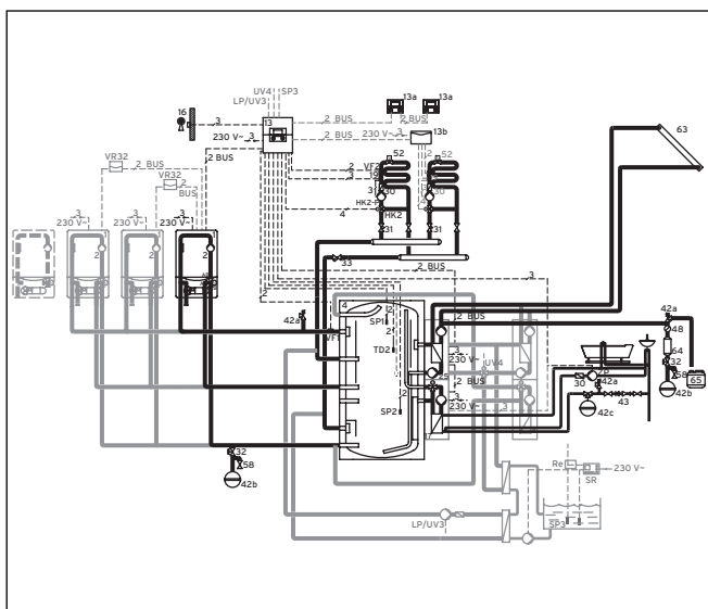
Abb. 4.1 Anschlusschema mit Wandheizgerät
