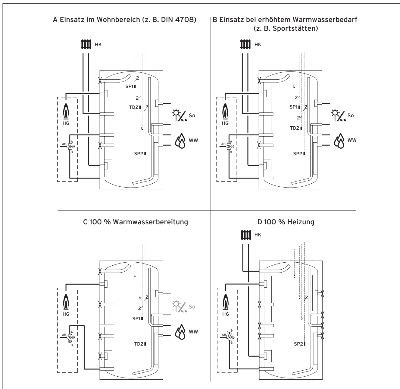
Abb. 3.11 Anwendungsbeispiel mit Solarsystem-regler VRS 620/3
