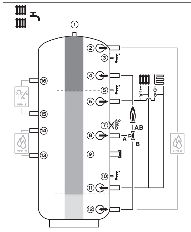
Abb. 4.2 Anschlusschema Wohnanwendung
