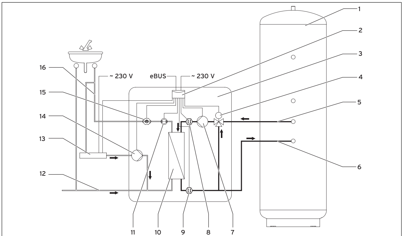
Abb. 3.5 Hydraulische Einbindung der Frischwasserstation, Montage am Pufferspeicher VPS/2
