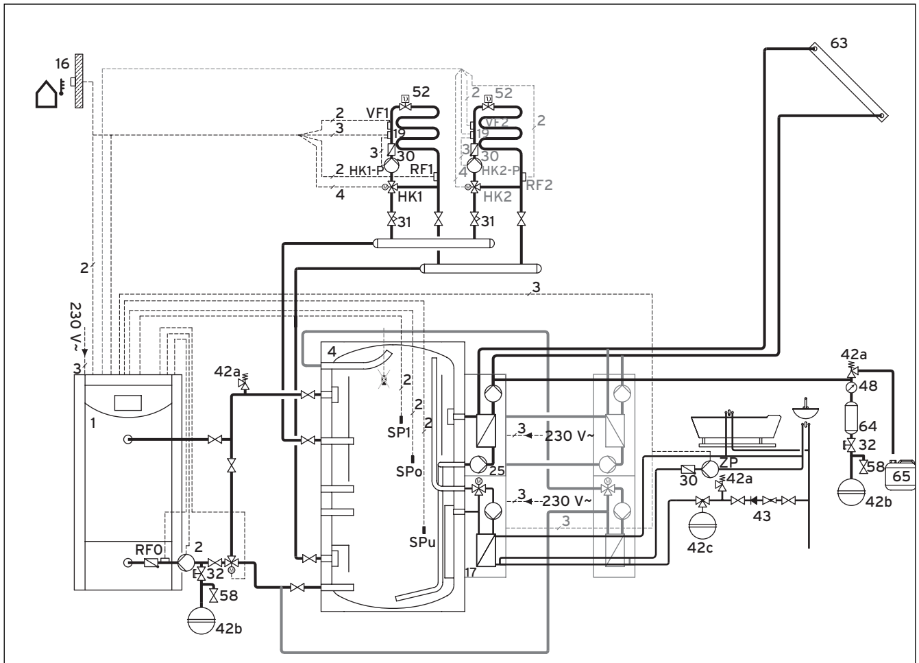
Abb. 3.10 Anschlussschema Pellet-Heizkessel
