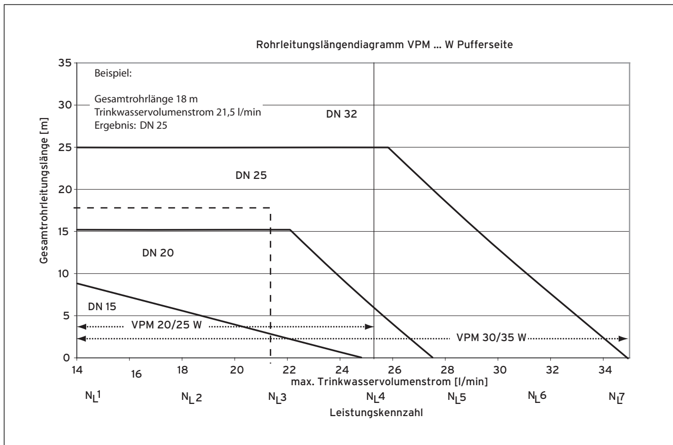
Abb. 3.22 Rohrleitungsdiagramm Frischwasserstation
