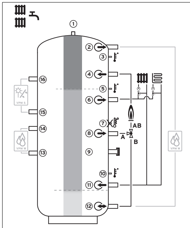
Abb. 3.2 Pufferspeicher VPS/2: Beispiel für Anschluss Wohnbereich
