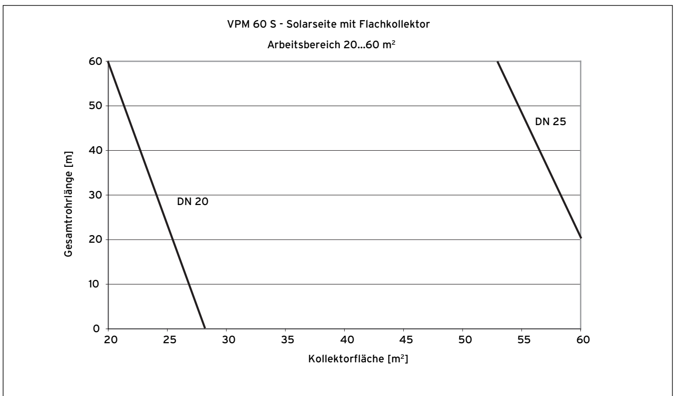
Abb. 3.21 Bestimmung Nenndurchmesser - VPM 60 S Solarseite mit Flachkollektoren
