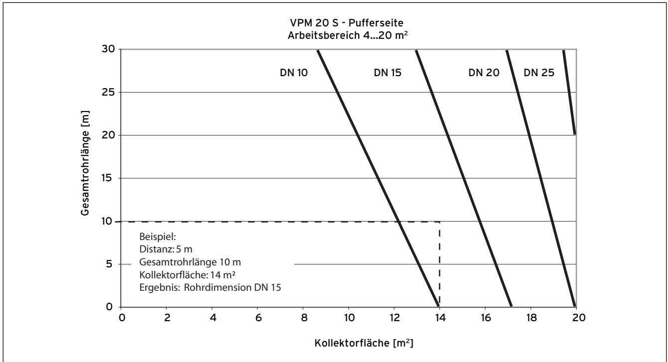
Abb. 3.16 Bestimmung Nenndurchmesser - VPM 20 S Pufferspeicherseite
