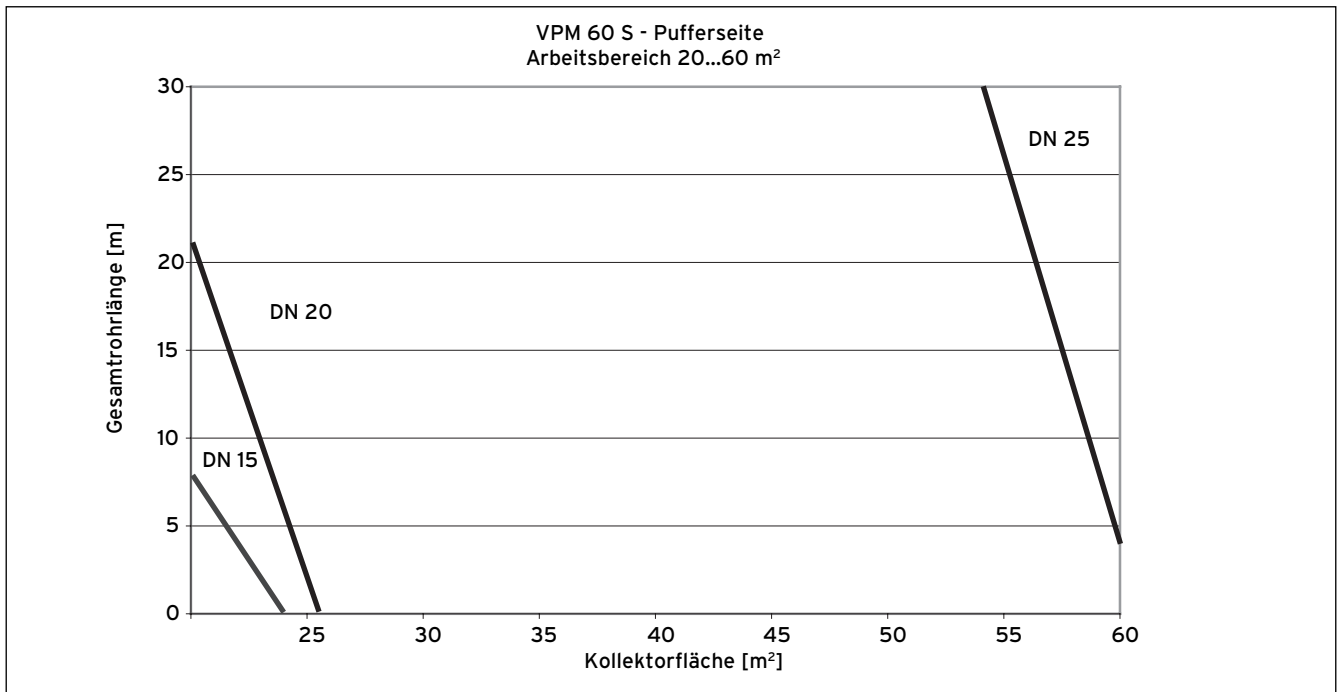
Abb. 3.17 Bestimmung Nenndurchmesser - VPM 60 S Pufferspeicherseite
