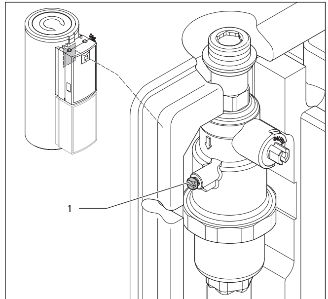
Abb. 5.9 Entlüfterschraube
