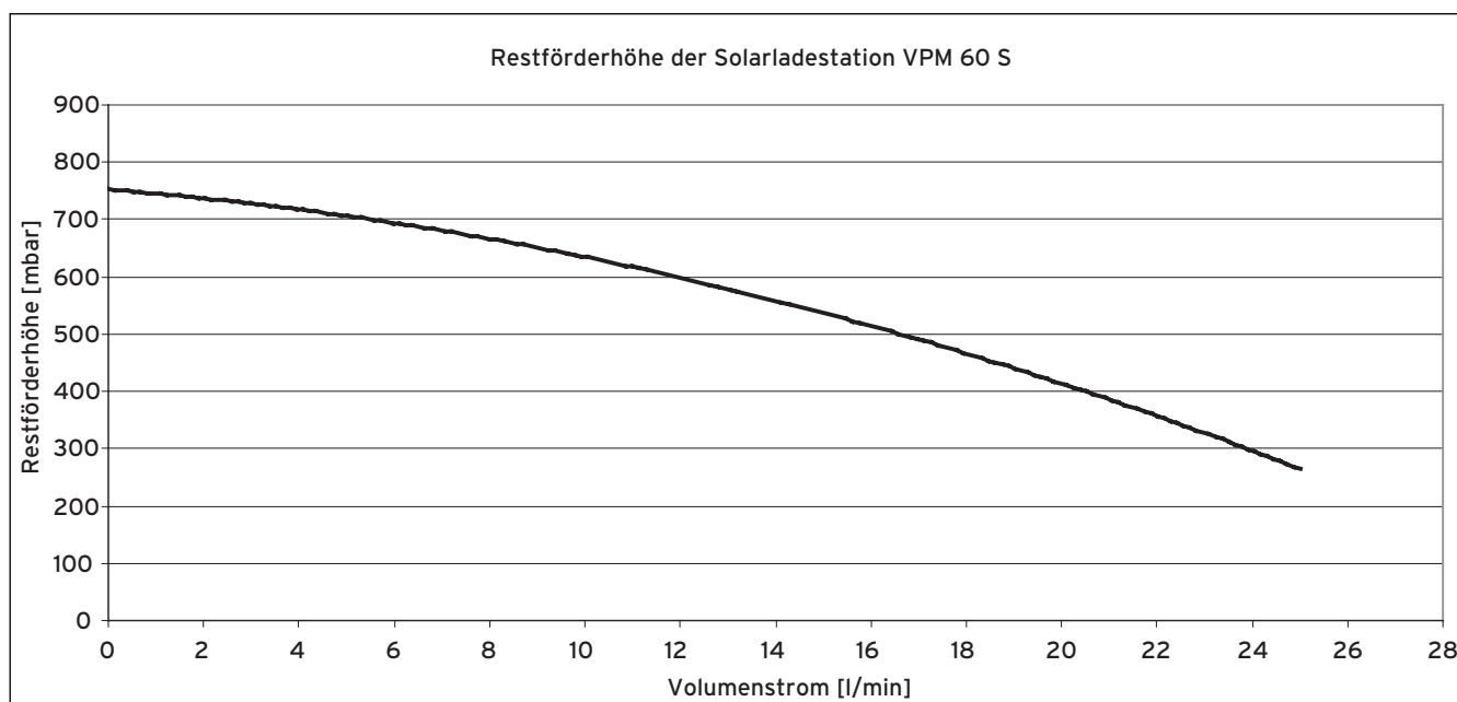
Abb. 12.3 Restförderhöhe Solarladestation VPM 60 S im Solar- kreis
