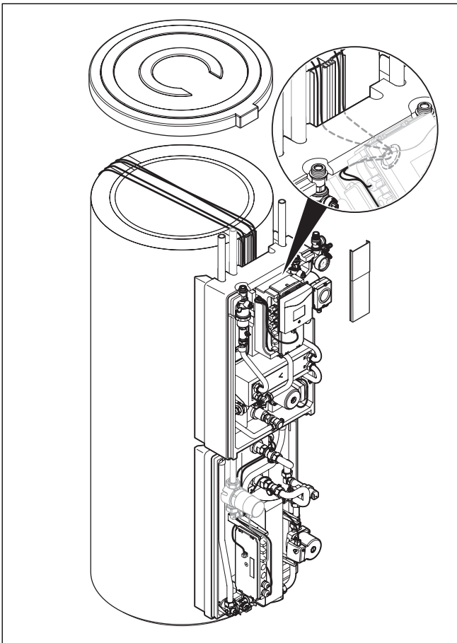
Abb. 5.13 Verlegung der Leitungen im Kabelkanal des Pufferspeichers im System mit Frischwasserstation.
