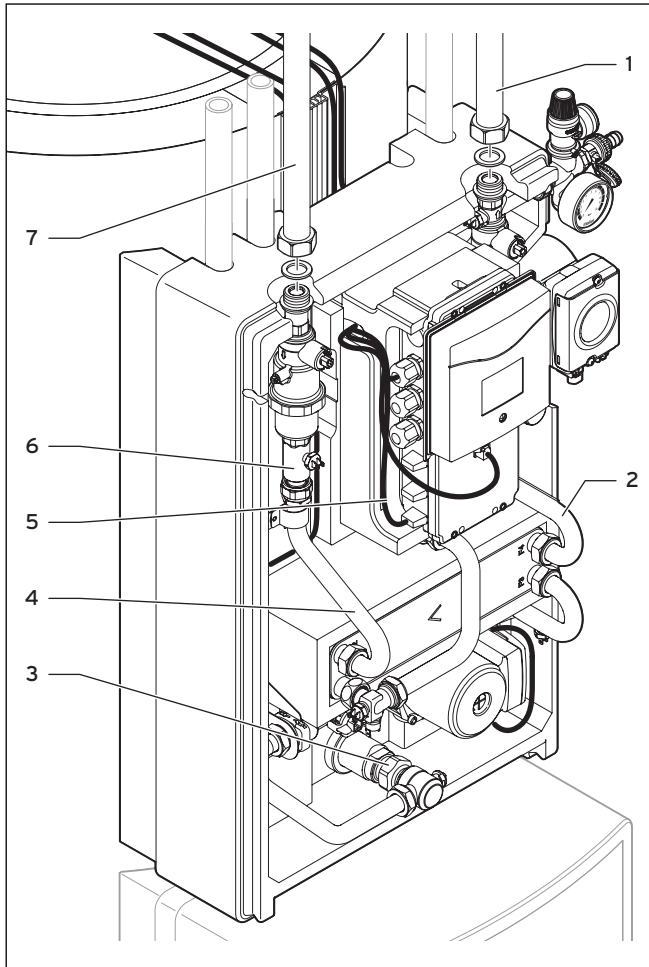
Abb. 5.6 Anschlussverrohrung - hydraulische Montage an das Kollektorfeld
