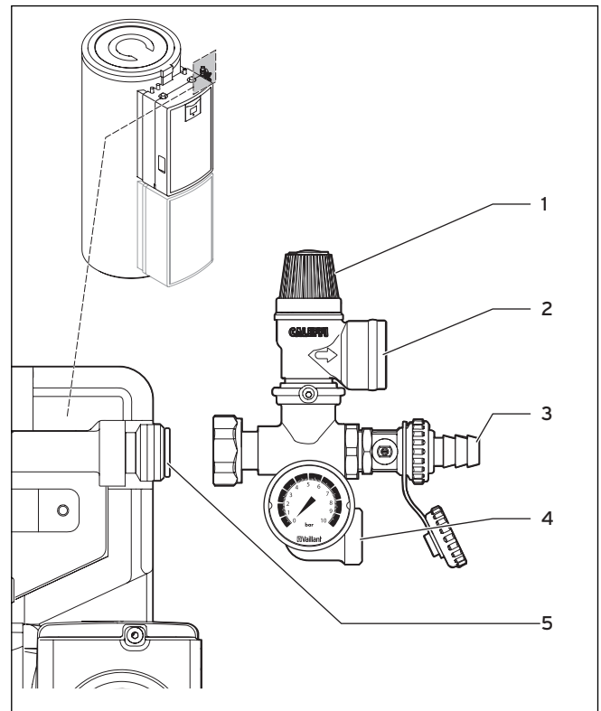
Abb. 5.5 Sicherheitsgruppe an Solarladestation anschließen
