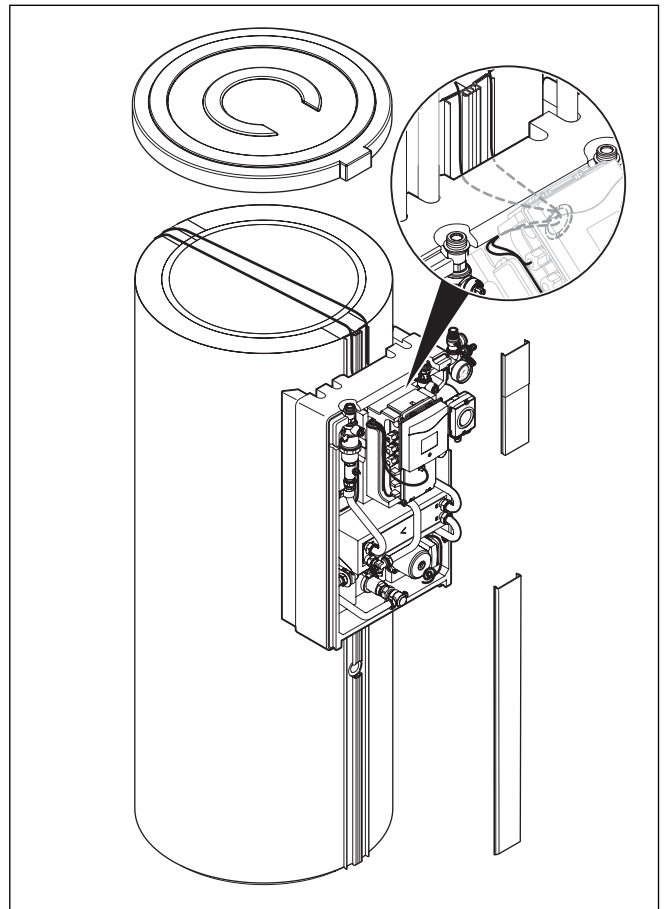
Abb. 5.12 Verlegung der Leitungen im Kabelkanal des Pufferspeichers ohne Frischwasserstation
