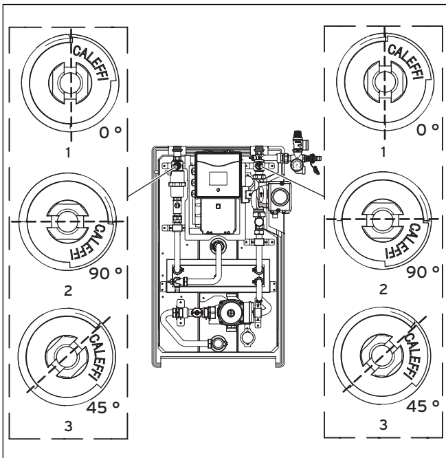
Abb. 5.8 Ventilstellungen in der Solarladestation
