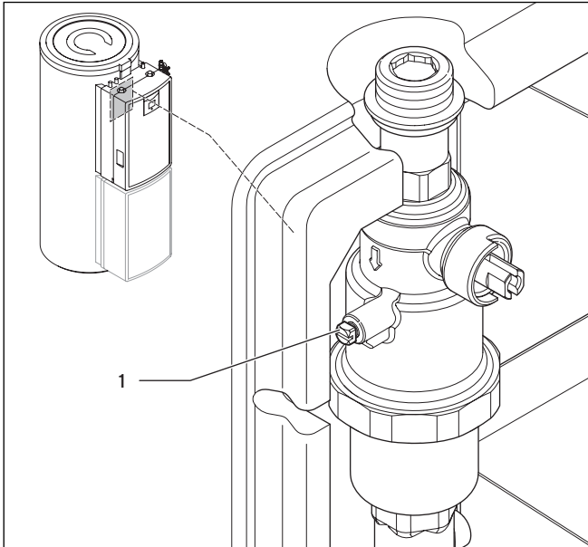
Abb. 5.9 Entlüfterschraube
