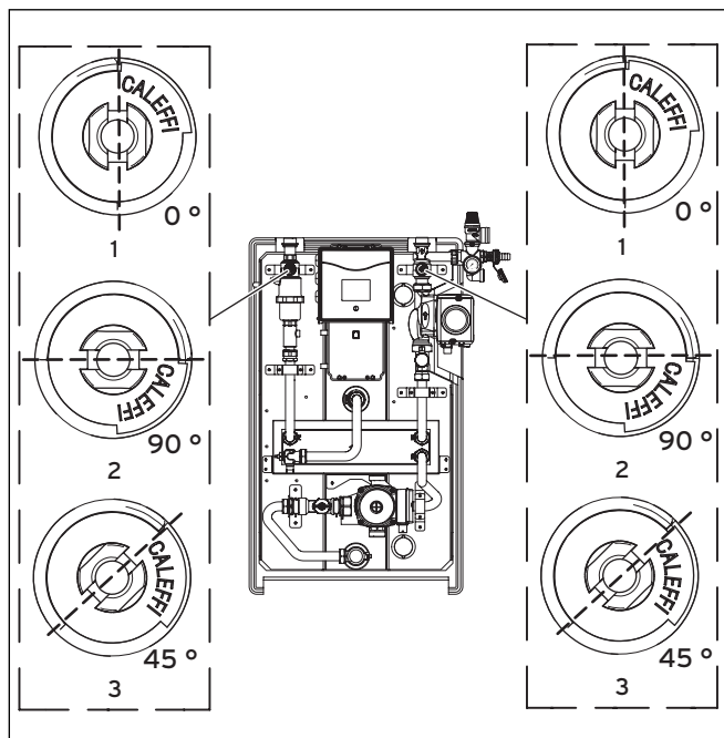
Abb.10.1 Ventilstellungen in der Solarladestation
