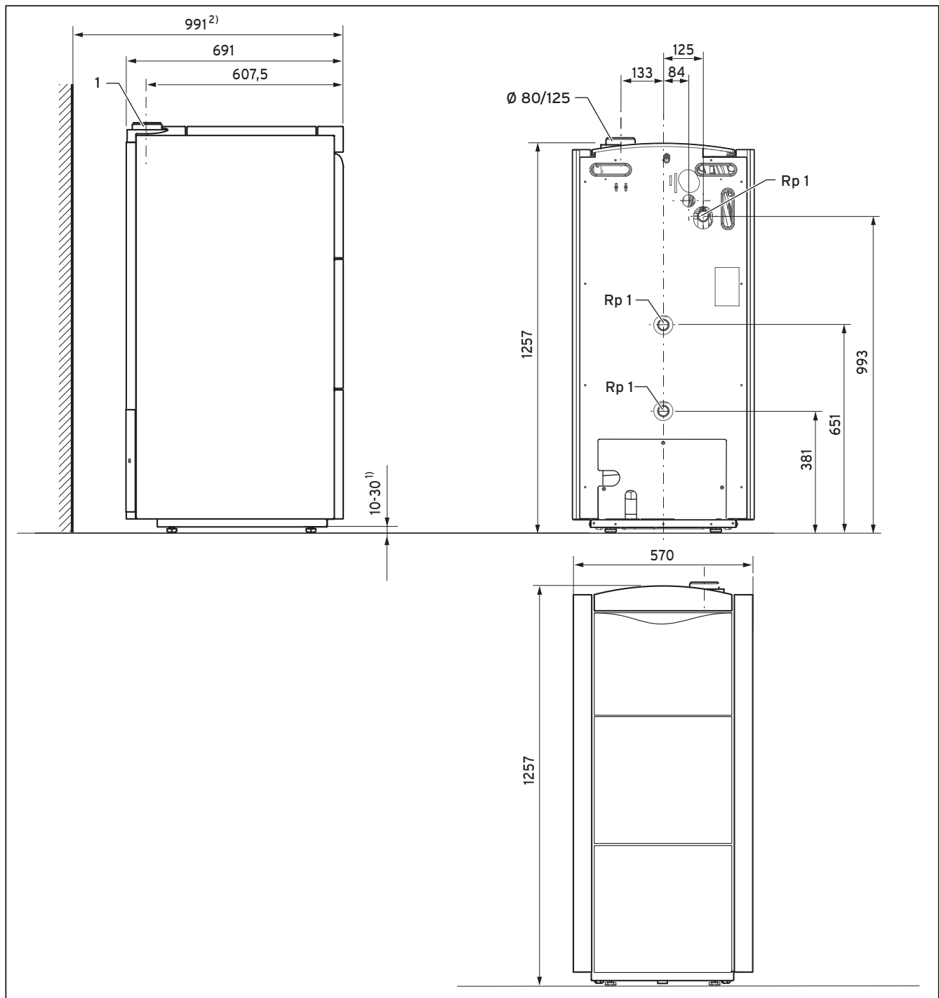
Abb. 4.2 Abmessungen
