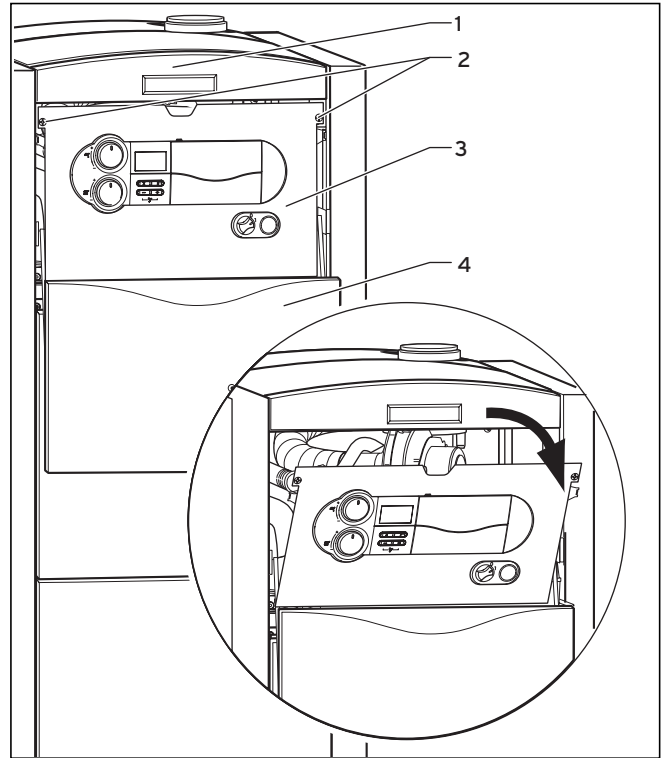
Abb. 5.1 Schaltschrank abklappen
