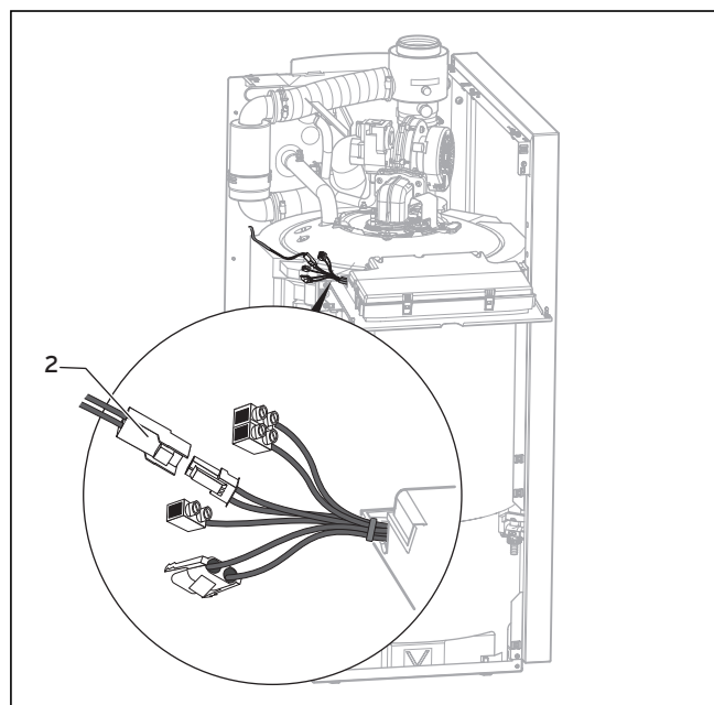
Abb. 5.6 Speichertemperaturfühler anschließen
