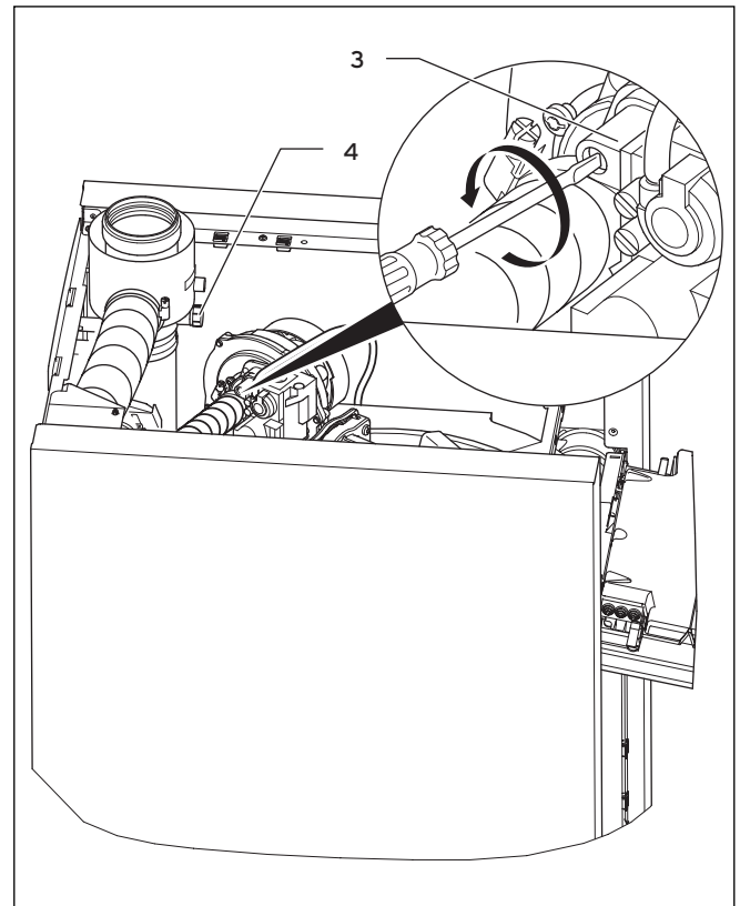
Abb. 6.4 CO 2 -Prüfung
