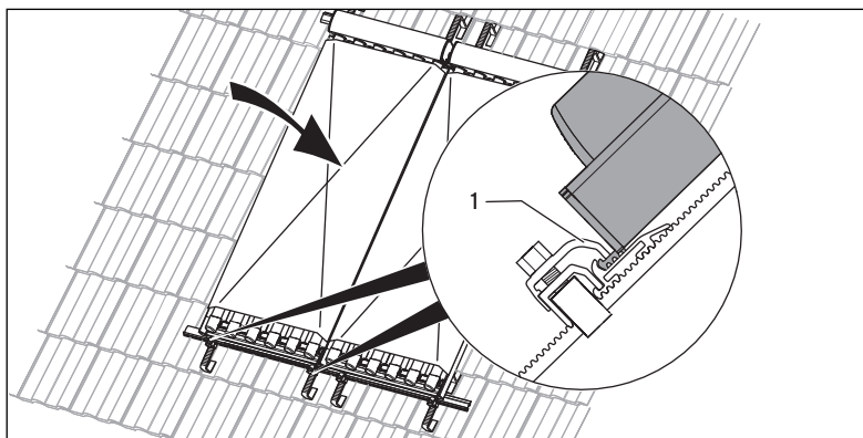
Abb. 5.27 Weitere Röhrenkollektoren montieren
