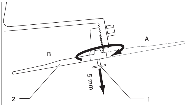
Abb. 5.12 Unterteil drehen
