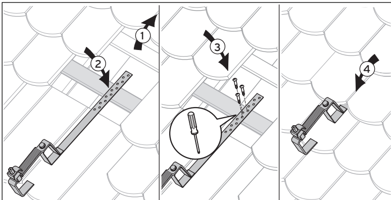
Abb. 5.17 Dachanker Typ S befestigen (hier: Befestigen an der Dachlatte)
