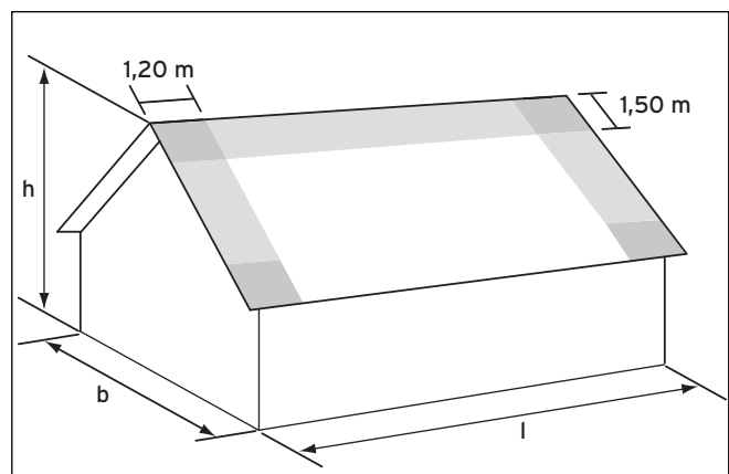
Abb. 5.7 Beispiel Einfamilienhaus, 12 m x 15 m x 8 m (Breite/Länge/Höhe)
