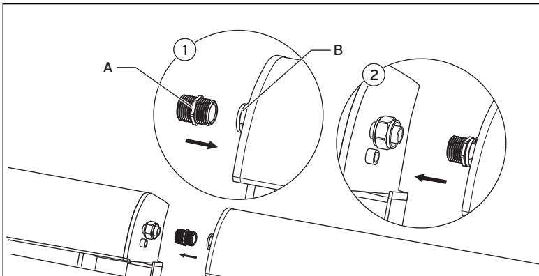
Abb. 6.15 Röhrenkollektoren verbinden
