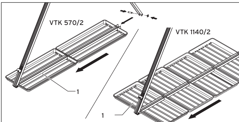
Abb. 6.4 Kieswannen montieren
