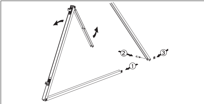
Abb. 6.3 Gestelle vorbereiten
