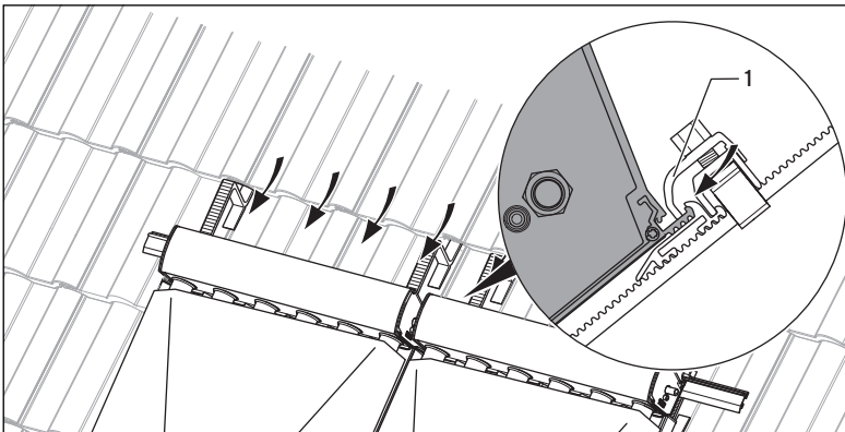
Abb. 5.30 Obere Montageschiene positionieren
