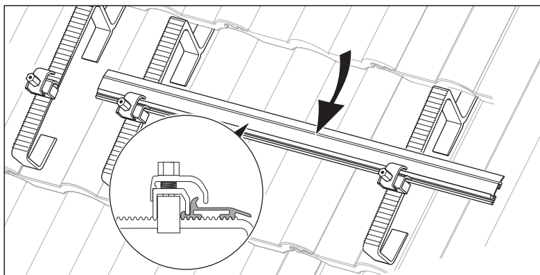
Abb. 5.21 Montageschienen montieren
