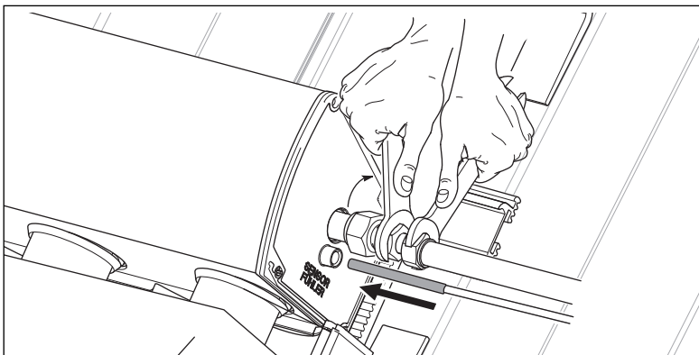
Abb. 5.33 Hydraulische Anschlüsse montieren
