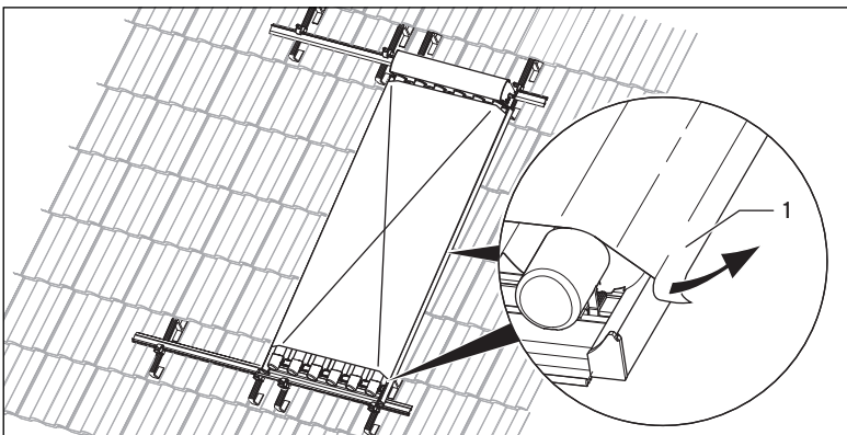
Abb. 5.25 Sonnenschutzfolie von Kollektorrändern ziehen
