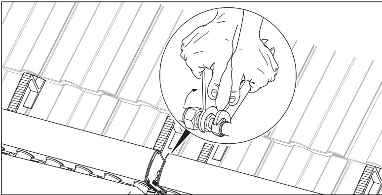
Abb. 5.29 Klemmringverbindung festziehen
