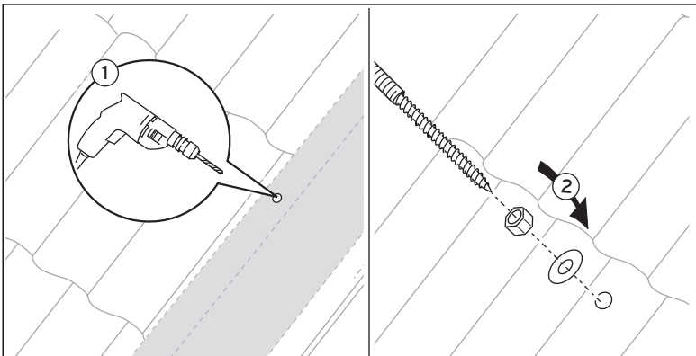
Abb. 5.19 Position des Dachankers auf dem Dachsparren festlegen
