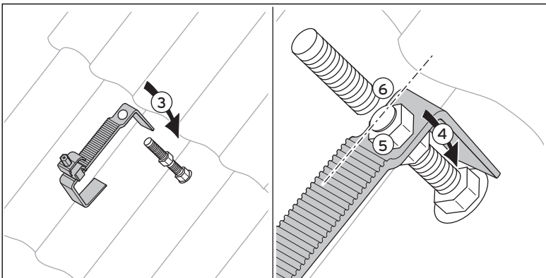
Abb. 5.20 Dachanker auf dem Dachsparren befestigen
