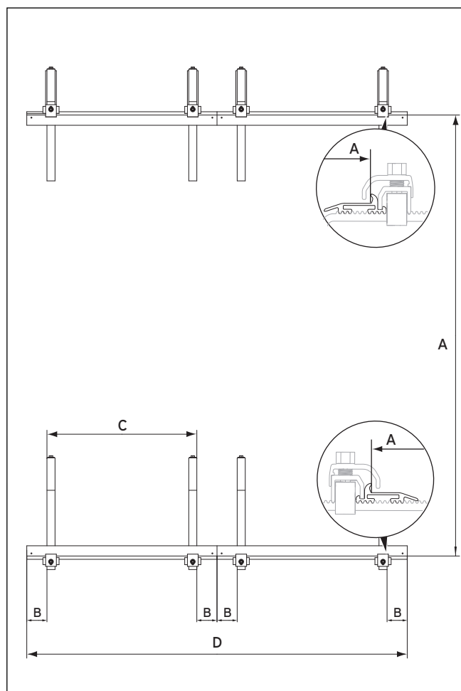
Abb. 5.8 Abstände bei Kollektoranordnung nebeneinander
