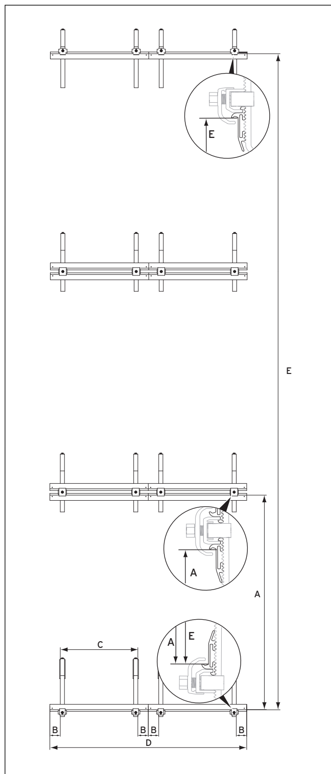
Abb. 5.10 Abstände bei 3-reihiger Kollektormontage
