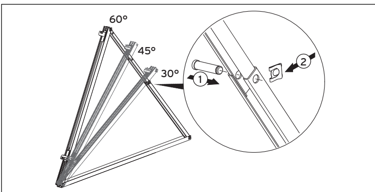
Abb. 6.5 Gestelle montieren
