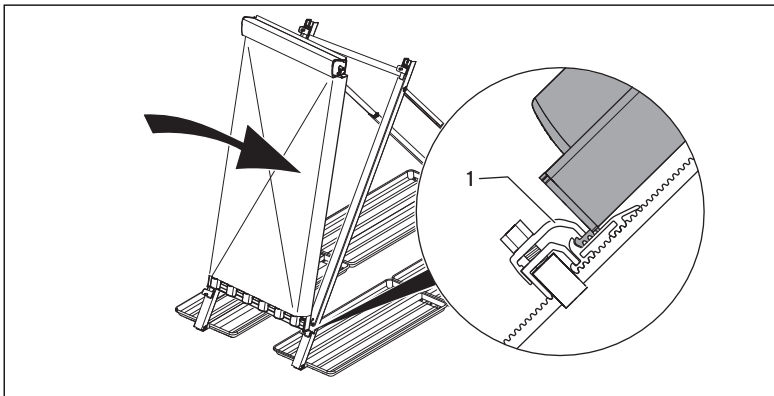
Abb. 6.11 Röhrenkollektor einhängen
