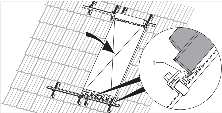
Abb. 5.24 Röhrenkollektor einhaken
