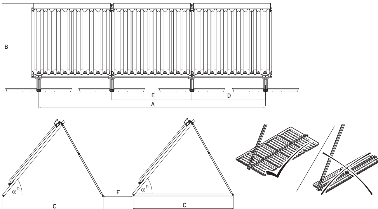
VTK 1140/2 (Abstände in mm)
