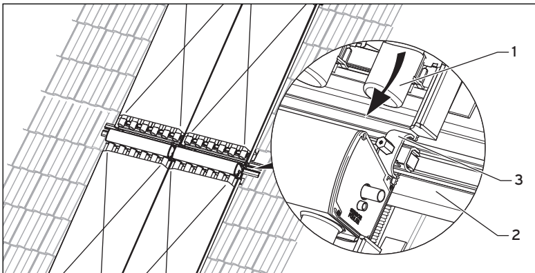
Abb. 5.32 Mittlere Montageschiene bei 2 oder 3 Kollektorreihen
