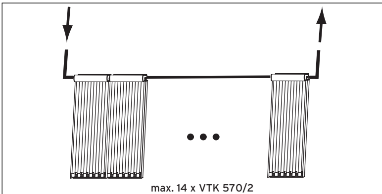
Abb. 4.2 Reihenschaltung VTK 570/2
