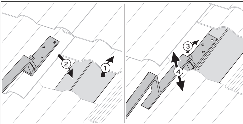
Abb. 5.13 Position des Dachankers Typ P auf dem Dachsparren festlegen
