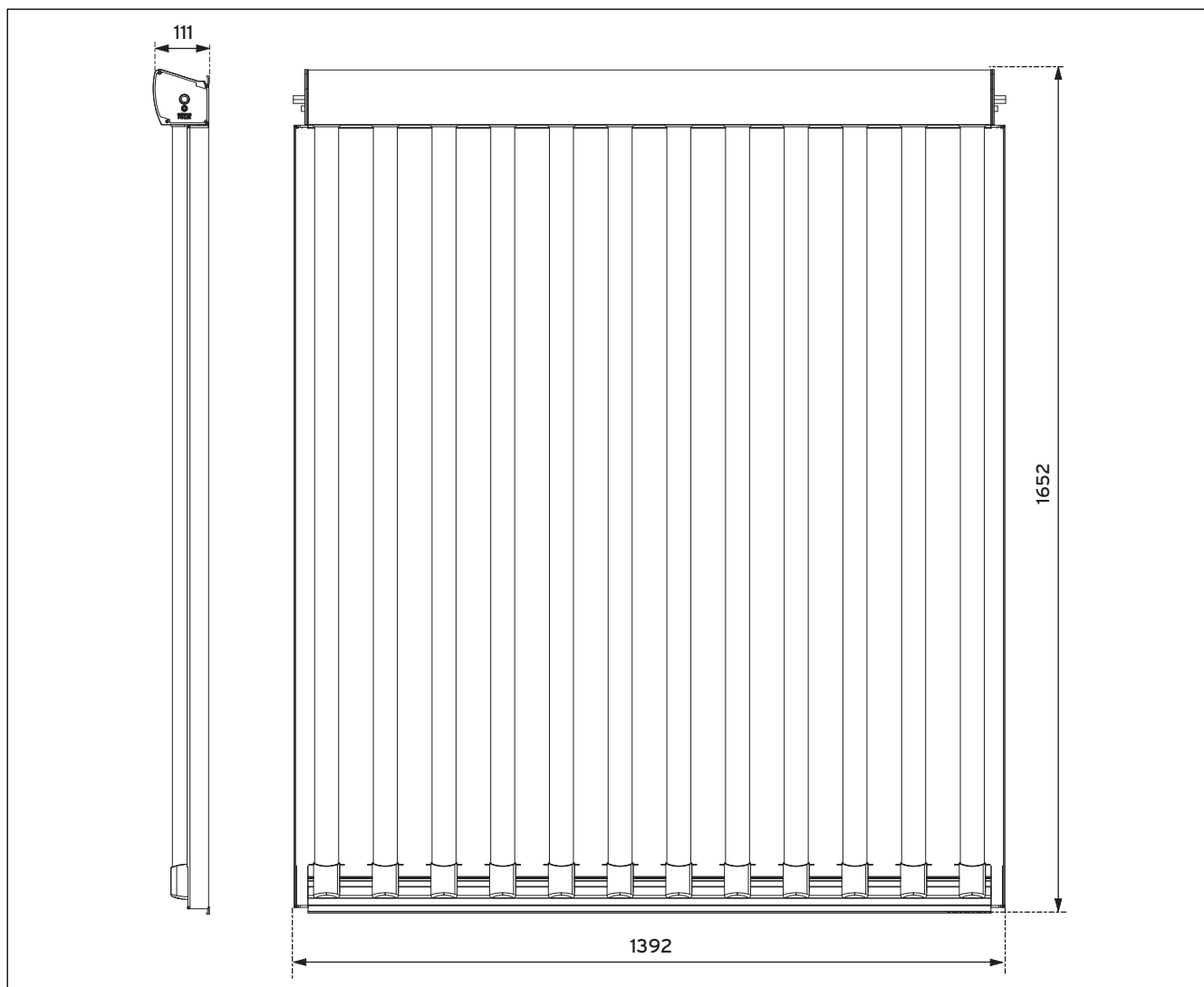
Abb. 14.2 Maßzeichnung VTK 1140/2
