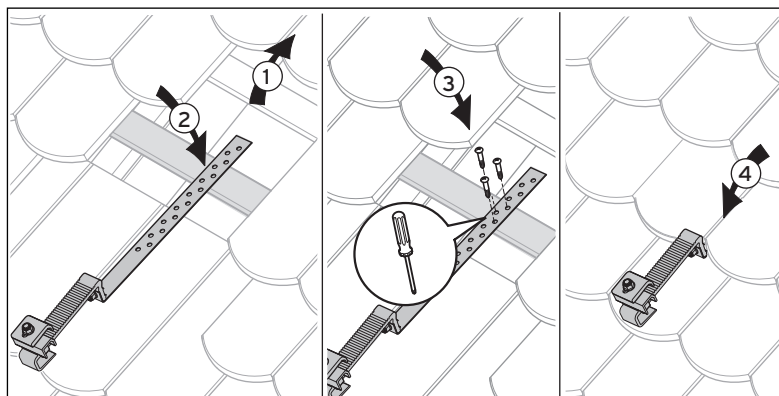
Abb. 5.18 Dachanker Typ S flach befestigen (hier: Befestigen an der Dachlatte)
