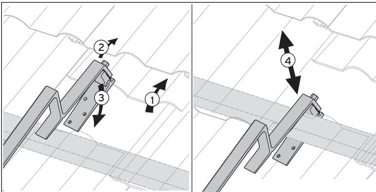
Abb. 5.15 Position des Dachankers Typ P auf der Dachlatte festlegen
