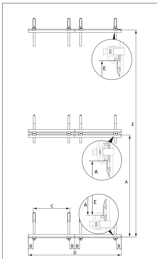
Abb. 5.9 Abstände bei 2-reihiger Kollektormontage
