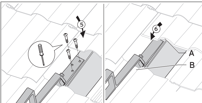
Abb. 5.14 Dachanker Typ P auf dem Dachsparren befestigen
