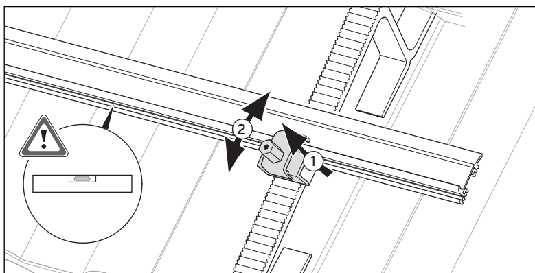
Abb. 5.23 Montageschienen austarieren
