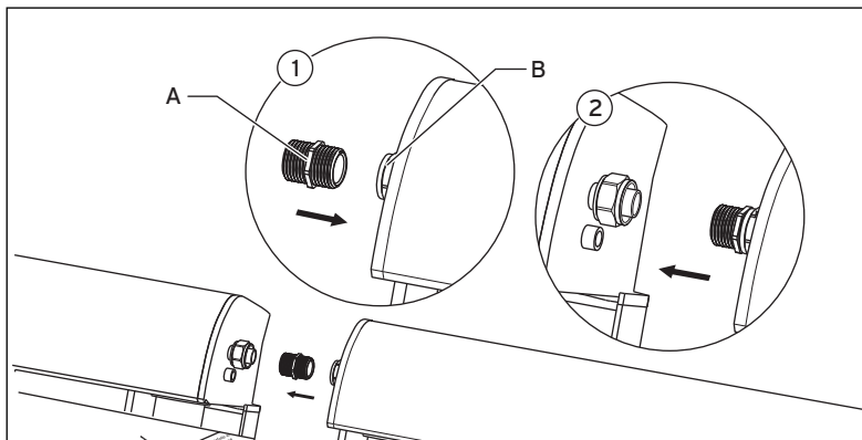
Abb. 5.28 Röhrenkollektoren verbinden
