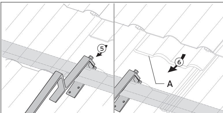
Abb. 5.16 Dachanker Typ P an der Dachlatte befestigen
