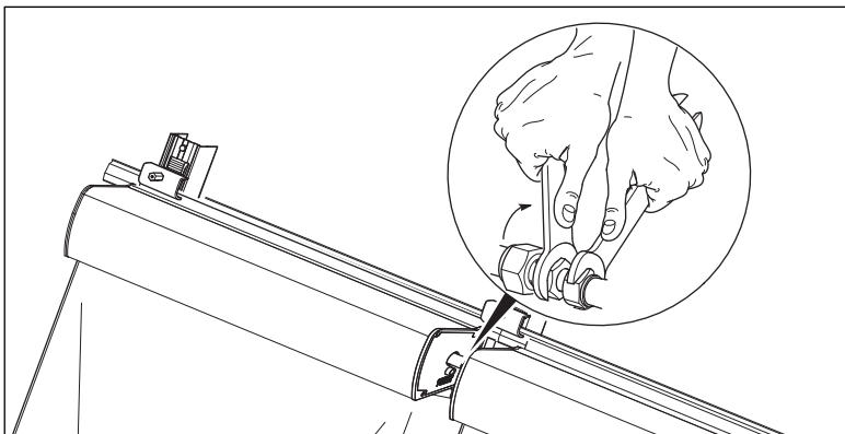
Abb. 6.16 Klemmringverbindung festziehen
