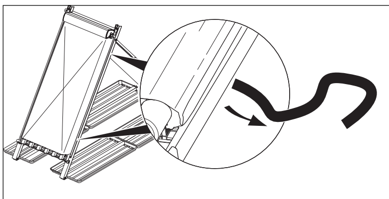
Abb. 6.13 Tragegurte entfernen
