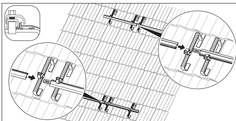
Abb. 5.22 Montageschienen verbinden
