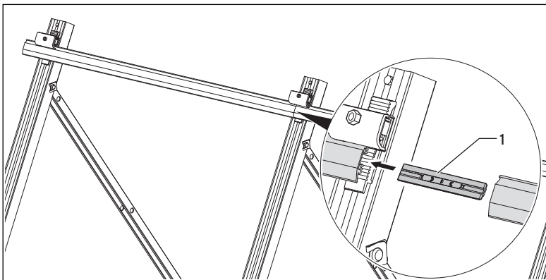
Abb. 6.10 Montageschienen verbinden
