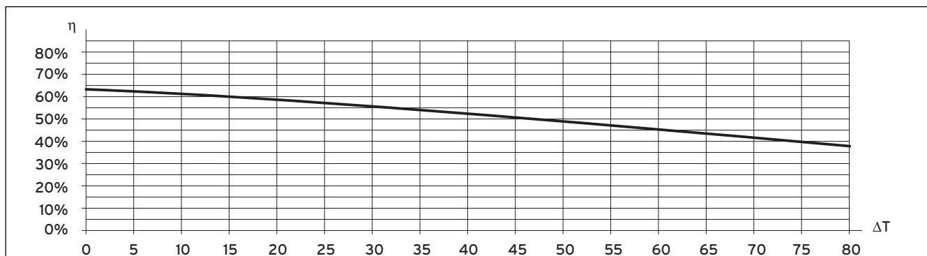
Abb. 14.3 Wirkungsgrad des VTK 570/2 und des VTK 1140/2 bei einer Einstrahlung EG von 300 W/m²
