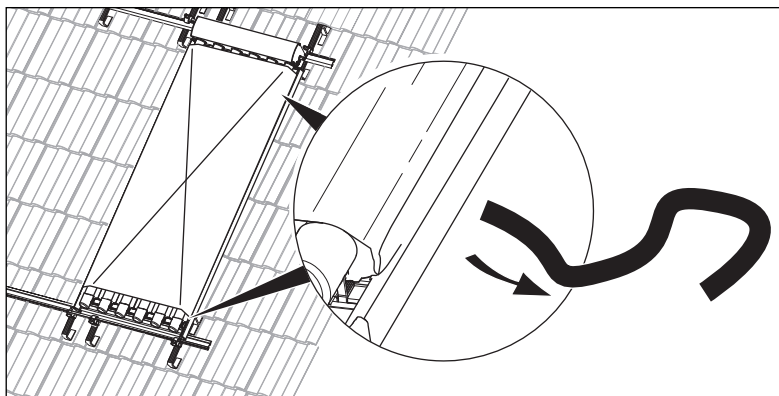
Abb. 5.26 Tragegurte entfernen
