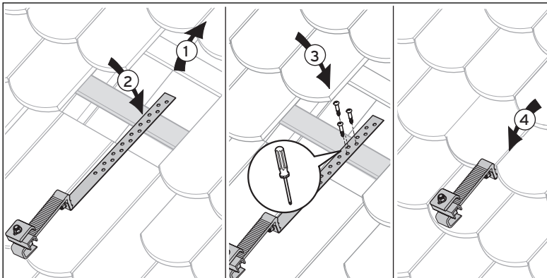
Abb. 5.17 Dachanker Typ S flach befestigen (hier: Befestigen an der Dachlatte)
