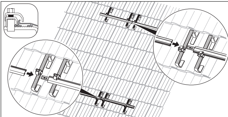
Abb. 5.21 Montageschienen verbinden
