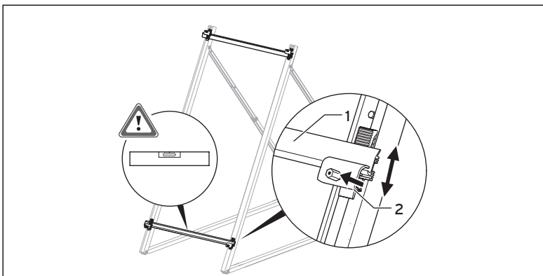
Abb. 6.8 Montageschienen befestigen und arretieren
