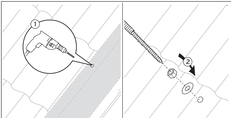
Abb. 5.18 Position des Dachankers auf dem Dachsparren festlegen
