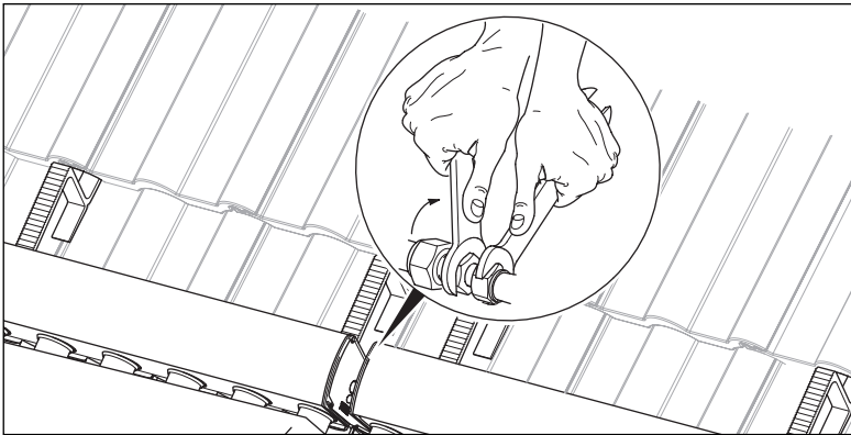
Abb. 5.28 Klemmringverbindung festziehen
