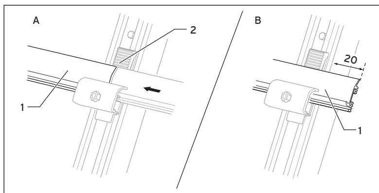
Abb. 6.9 Positionierung der Montageschienen
