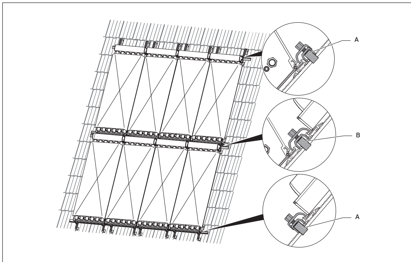
Abb. 5.5 Einbau-Set Aufdachmontage 2-reihig (hier: VTK 570/2)
