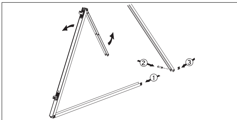
Abb. 6.3 Gestelle vorbereiten
