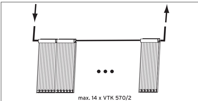
Abb. 4.2 Reihenschaltung VTK 570/2
