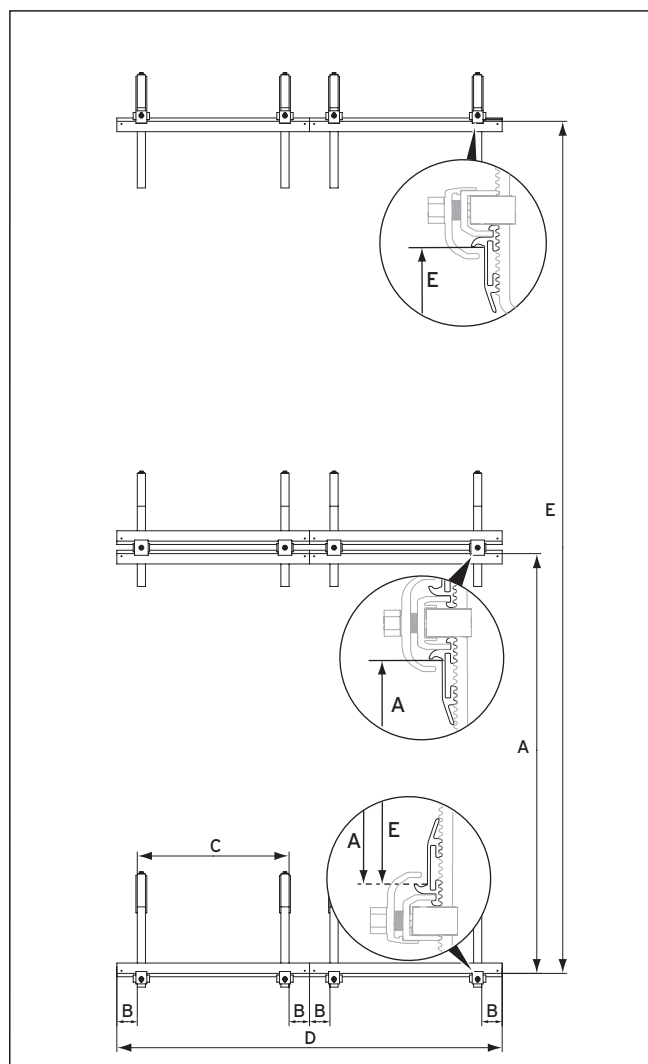
Abb. 5.8 Abstände bei 2-reihiger Kollektormontage
