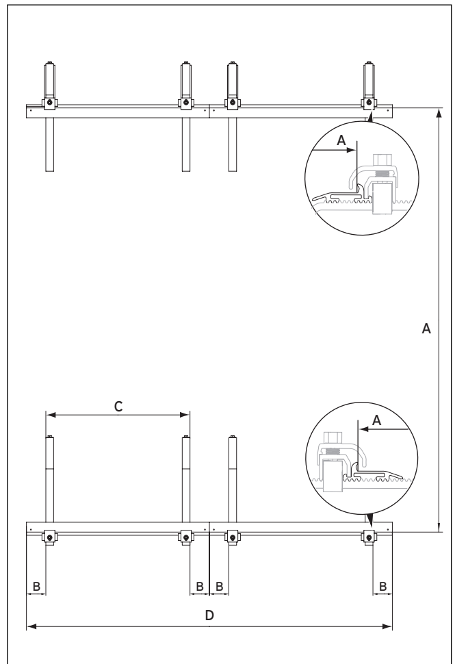
Abb. 5.7 Abstände bei Kollektoranordnung nebeneinander
