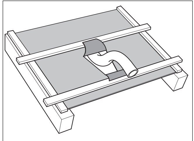
Abb. 5.1 Rohr durch Unterspannbahn oder Dachpappe führen
