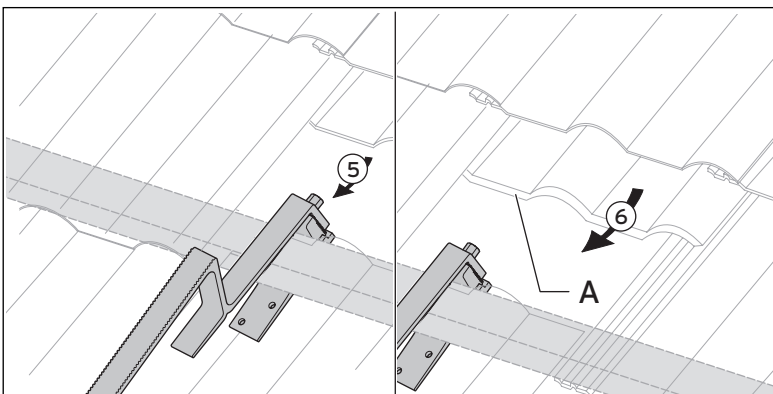
Abb. 5.15 Dachanker Typ P an der Dachlatte befestigen
