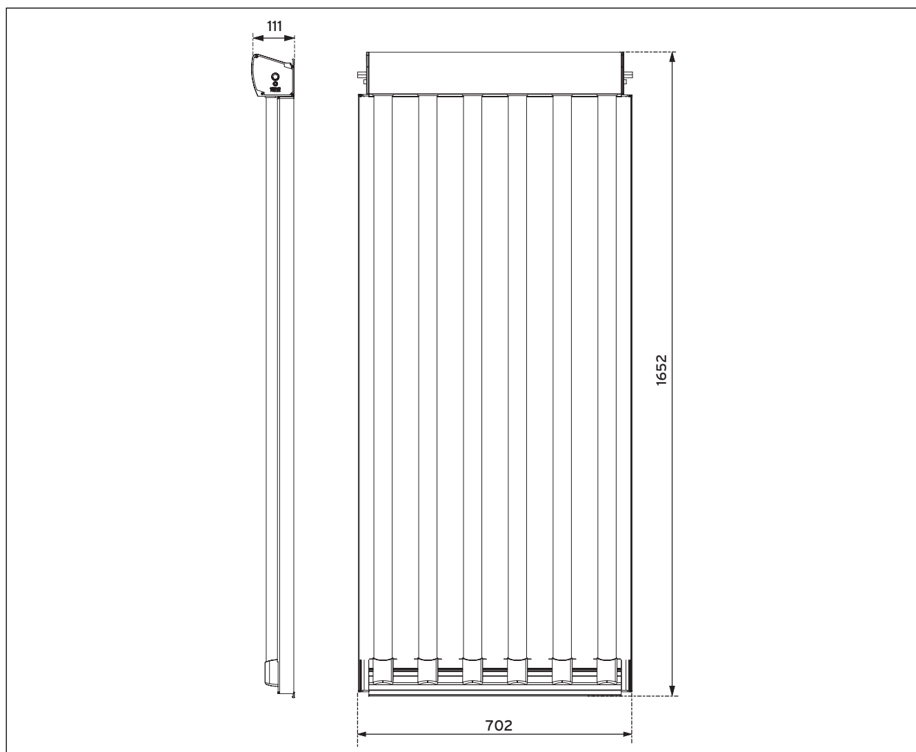
Abb. 14.1 Maßzeichnung VTK 570/2
