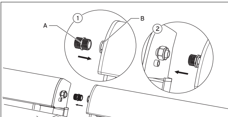
Abb. 5.27 Röhrenkollektoren verbinden
