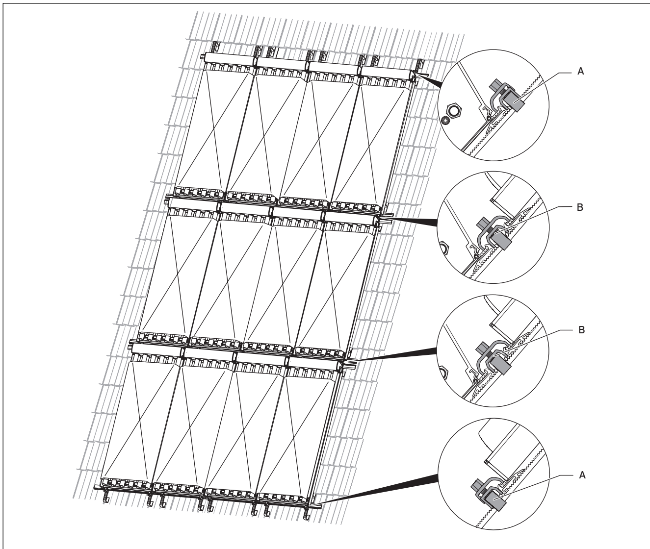
Abb. 5.6 Einbau-Set Aufdachmontage 3-reihig (hier: VTK 570/2)
