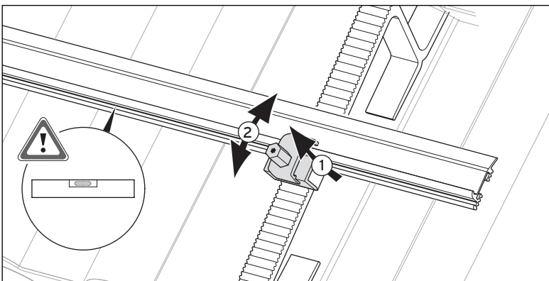
Abb. 5.22 Montageschienen austarieren
