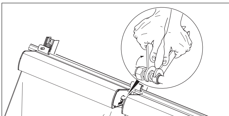
Abb. 6.16 Klemmringverbindung festziehen
