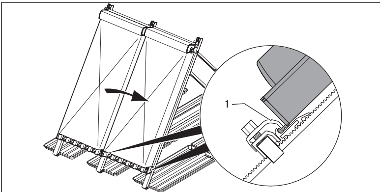
Abb. 6.14 Weitere Röhrenkollektoren montieren
