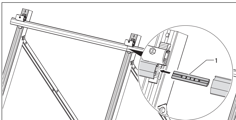
Abb. 6.10 Montageschienen verbinden
