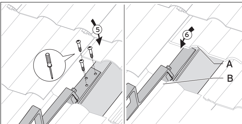
Abb. 5.13 Dachanker Typ P auf dem Dachsparren befestigen
