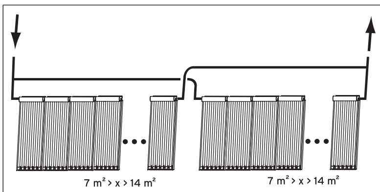
Abb. 4.5 Parallelverschaltung (hier abgebildet: VTK 570/2)
