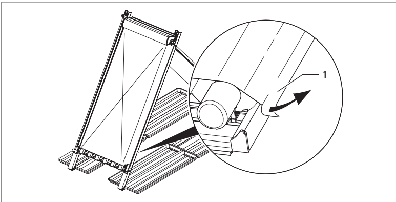
Abb. 6.12 Sonnenschutzfolie von Kollektorrändern ziehen
