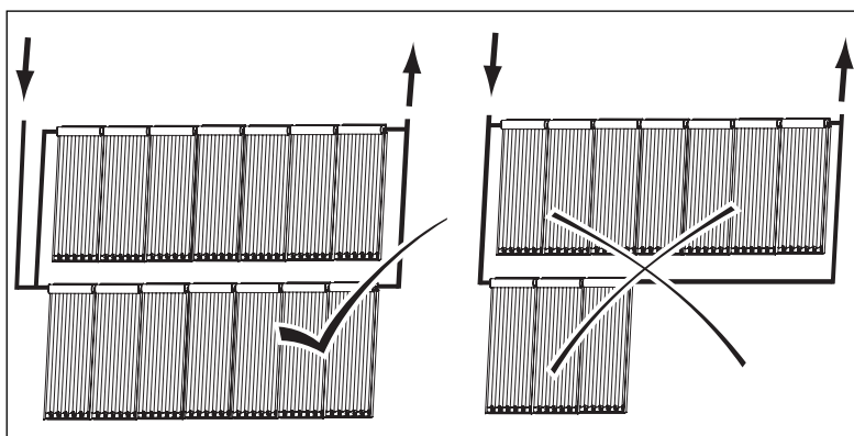
Abb. 4.6 Größe der Einzelreihen (hier abgebildet: VTK 570/2)
