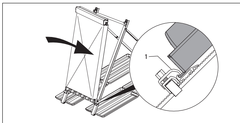
Abb. 6.11 Röhrenkollektor einhängen
