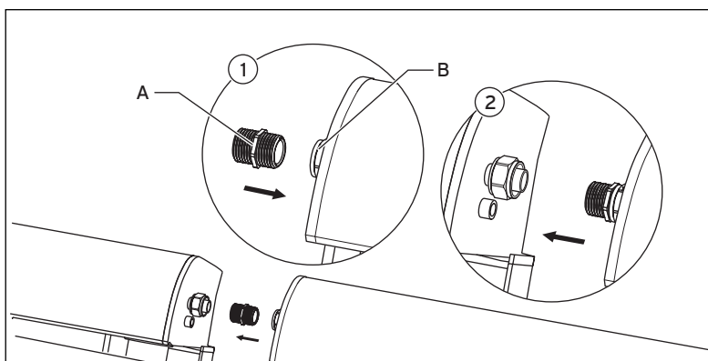
Abb. 6.15 Röhrenkollektoren verbinden
