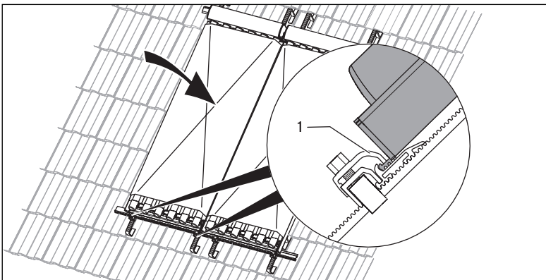
Abb. 5.26 Weitere Röhrenkollektoren montieren
