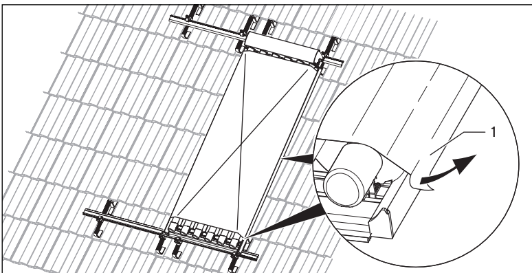
Abb. 5.24 Sonnenschutzfolie von Kollektorrändern ziehen
