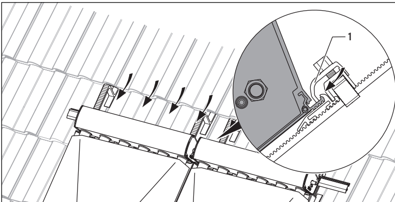
Abb. 5.29 Obere Montageschiene positionieren
