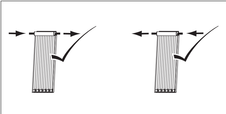
Abb. 4.1 Durchströmungsrichtung (hier abgebildet: VTK 570/2)
