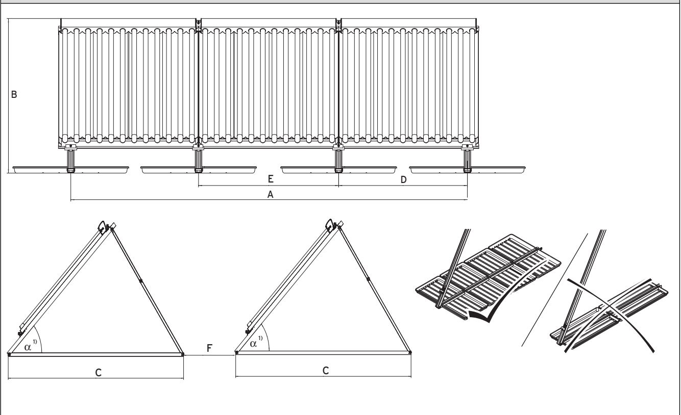
VTK 1140/2 (Abstände in mm)
