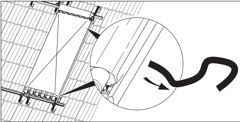
Abb. 5.25 Tragegurte entfernen
