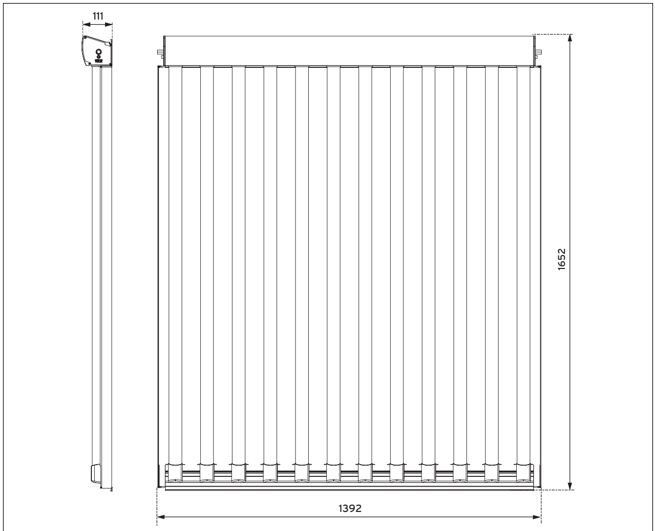
Abb. 14.2 Maßzeichnung VTK 1140/2
