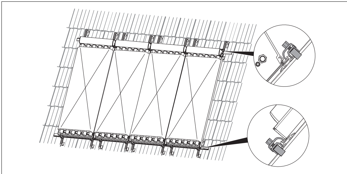
Abb. 5.4 Einbau-Set Aufdachmontage 1-reihig (hier: VTK 570/2)
