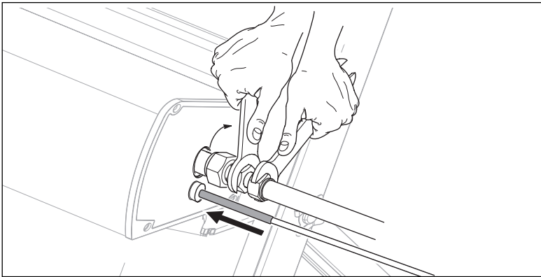
Abb. 6.18 Hydraulische Anschlüsse montieren
