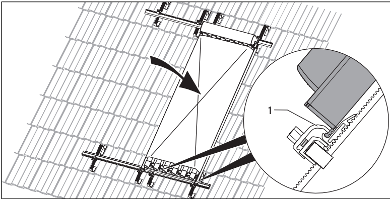
Abb. 5.23 Röhrenkollektor einhaken
