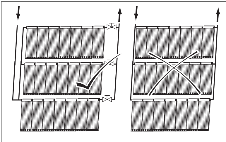
Abb. 4.7 Absperrventil in Kollektorvorlauf (hier abgebildet: VTK 570/2)
