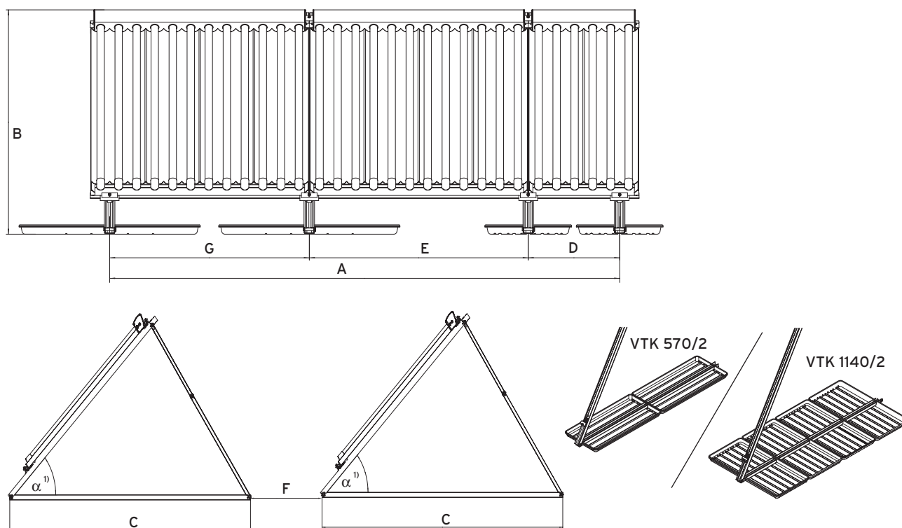
VTK 1140/2 und VTK 570/2 in Kombination (Abstände in mm)
