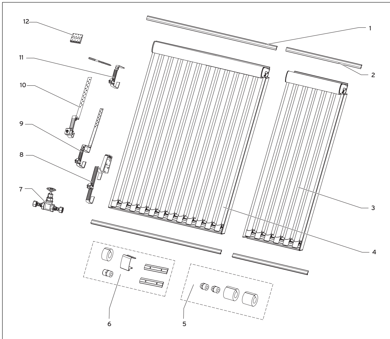
Abb. 5.3 Einbau-Set Aufdachmontage
