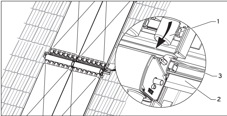
Abb. 5.31 Mittlere Montageschiene bei 2 oder 3 Kollektorreihen
