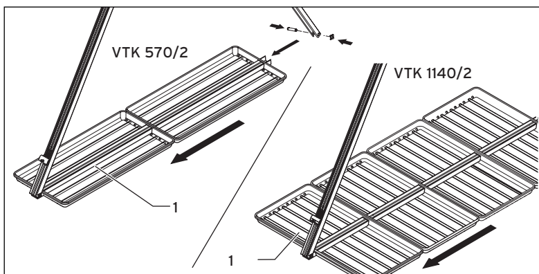
Abb. 6.4 Kieswannen montieren
