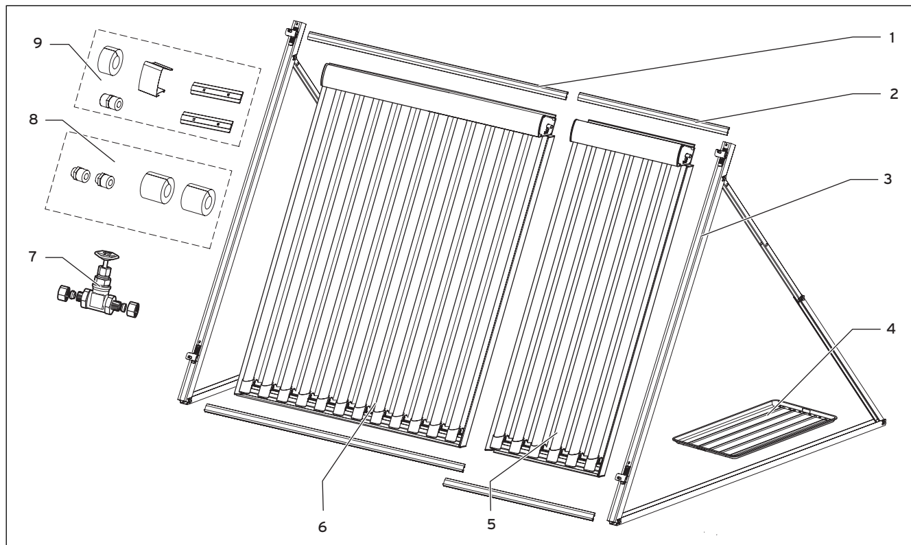
Abb. 6.2 Einbau-Set Flachdachmontage
