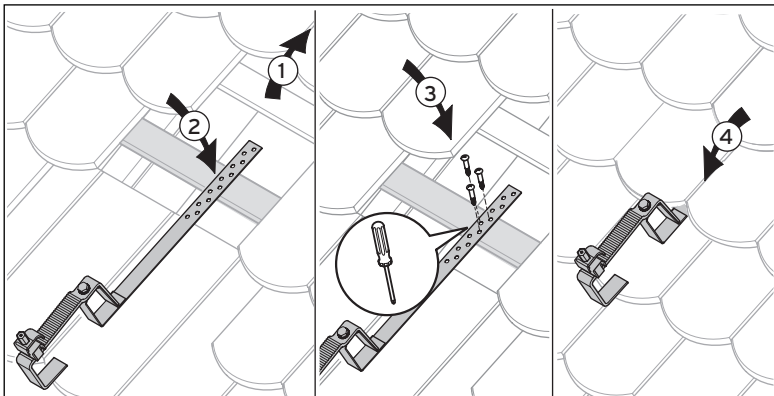
Abb. 5.16 Dachanker Typ S befestigen (hier: Befestigen an der Dachlatte)
