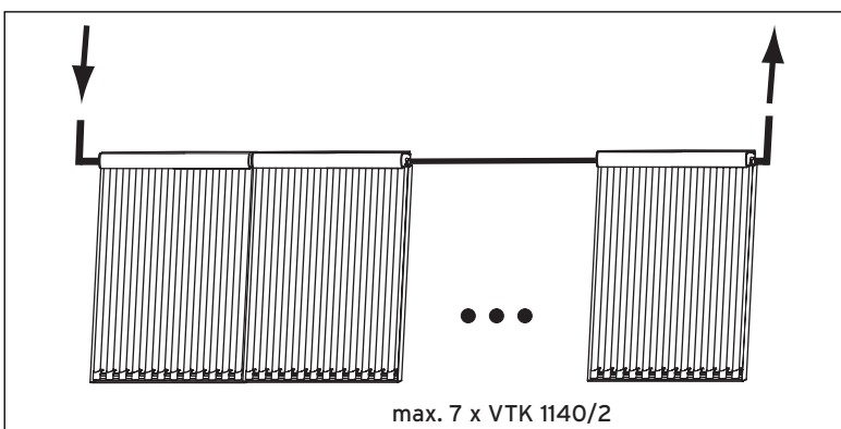
Abb. 4.3 Reihenschaltung VTK 1140/2
