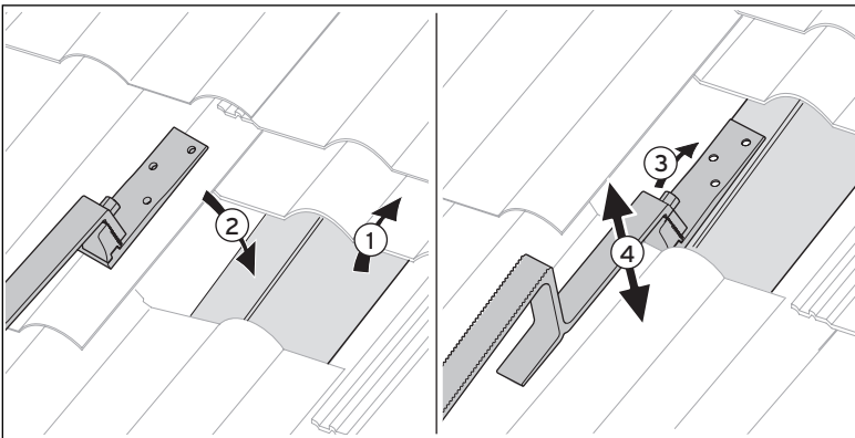
Abb. 5.12 Position des Dachankers Typ P auf dem Dachsparren festlegen
