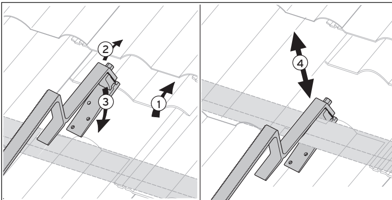
Abb. 5.14 Position des Dachankers Typ P auf der Dachlatte festlegen
