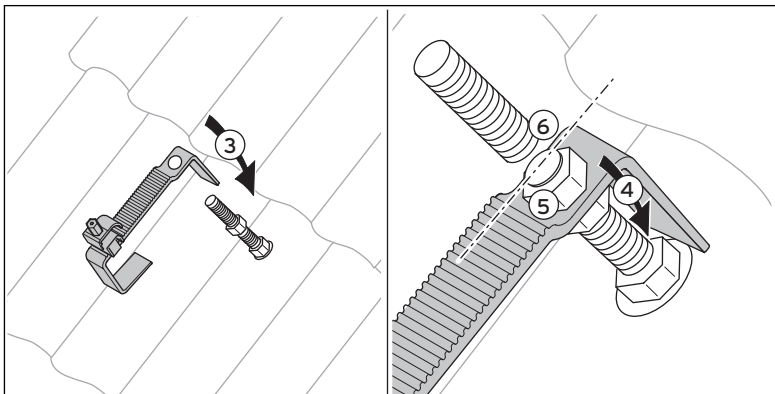
Abb. 5.19 Dachanker auf dem Dachsparren befestigen
