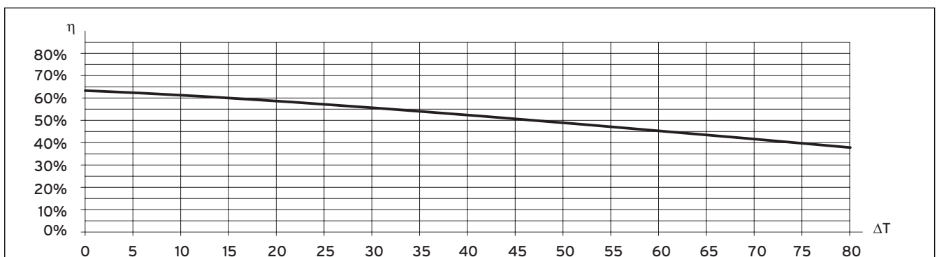
Abb. 14.3 Wirkungsgrad des VTK 570/2 und des VTK 1140/2 bei einer Einstrahlung EG von 300 W/m 2
