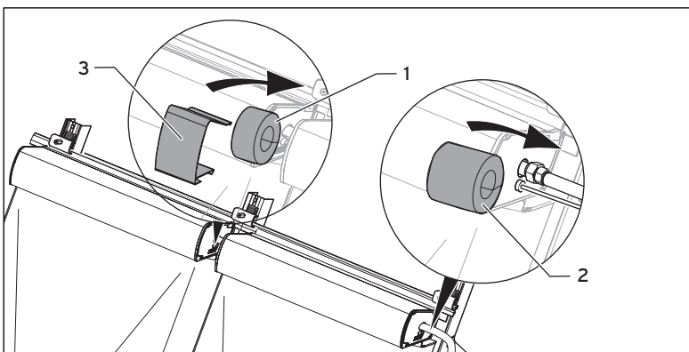
Abb. 6.19 Hydraulische Anschlüsse isolieren
