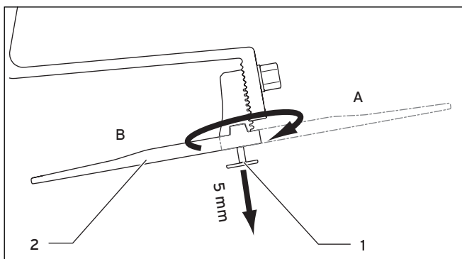
Abb. 5.11 Unterteil drehen
