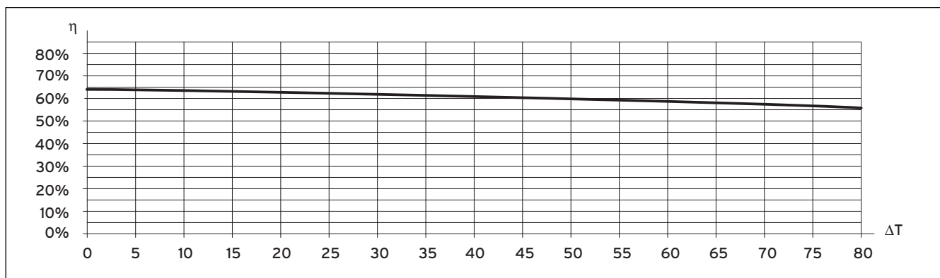
Abb. 14.4 Wirkungsgrad des VTK 570/2 und des VTK 1140/2 bei einer Einstrahlung EG von 800 W/m 2
