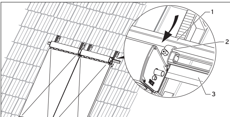
Abb. 5.30 Mittlere Montageschiene bei 2 oder 3 Kollektorreihen
