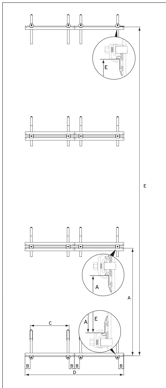
Abb. 5.9 Abstände bei 3-reihiger Kollektormontage
