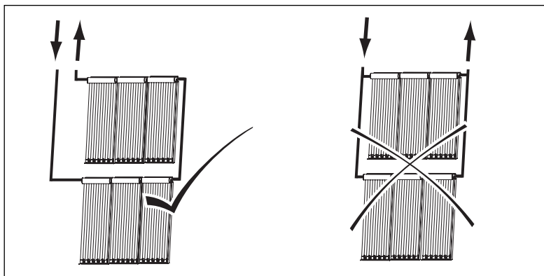
Abb. 4.4 Parallelverschaltung (hier abgebildet: VTK 570/2)
