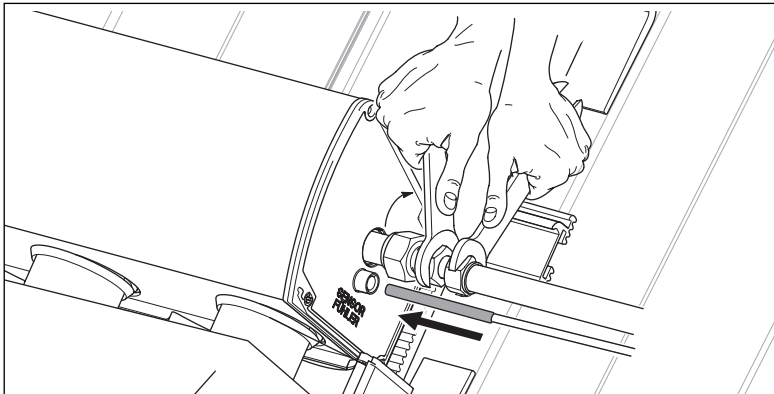
Abb. 5.32 Hydraulische Anschlüsse montieren
