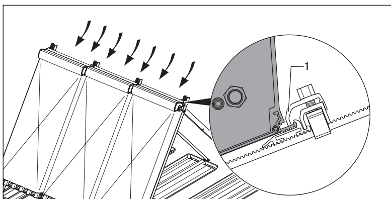
Abb. 6.17 Obere Montageschiene positionieren
