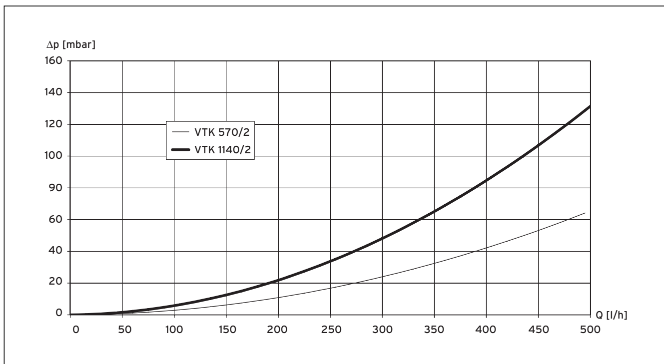
Abb. 14.5 Druckverlustrdiagramm
