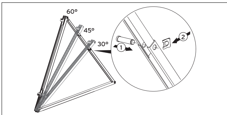
Abb. 6.5 Gestelle montieren
