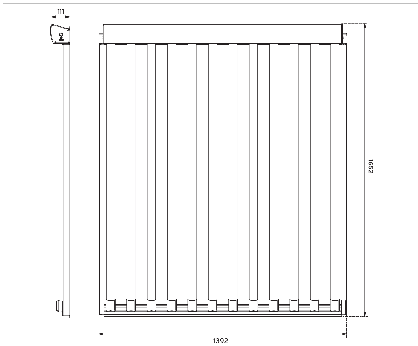
Abb. 10.2 Maßzeichnung VTK 1140/2
