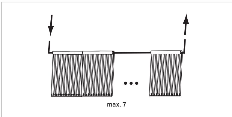
Abb. 4.7 Reihenschaltung VTK 1140/2
