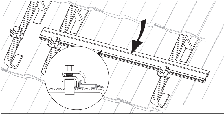
Abb. 5.9 Montageschienen montieren
