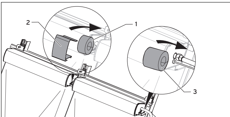
Abb. 6.17 Hydraulische Anschlüsse isolieren
