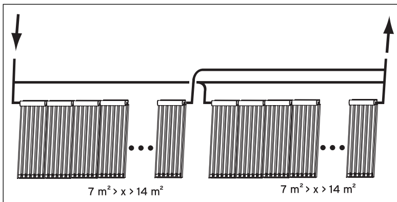
Abb. 4.8 Parallelverschaltung (hier VTK 570/2)
