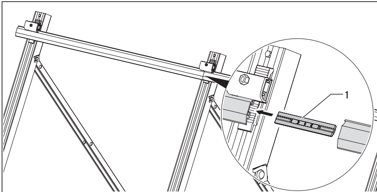
Abb. 6.8 Montageschienen verbinden
