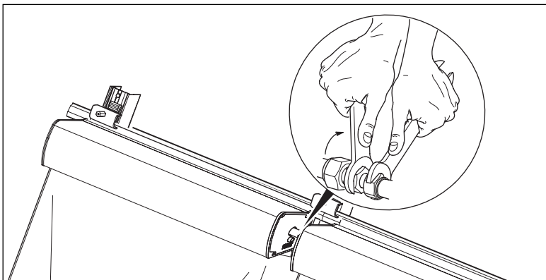
Abb. 6.14 Klemmringverbindung festziehen
