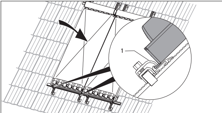
Abb. 5.15 Weitere Kollektoren montieren
