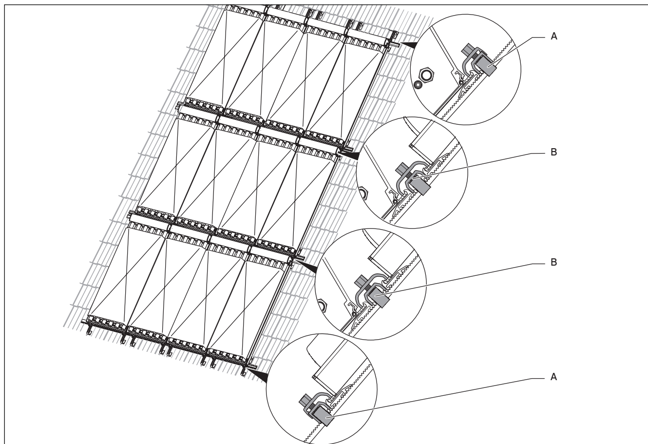
Abb. 4.5 Einbauset Aufdachmontage 3-reihig (hier: VTK 570/2)
