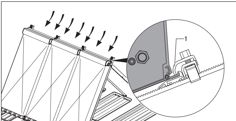
Abb. 6.15 Obere Montageschiene positionieren
