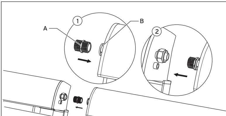
Abb. 6.13 Kollektoren verbinden
