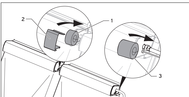
Abb. 5.22 Hydraulische Anschlüsse isolieren
