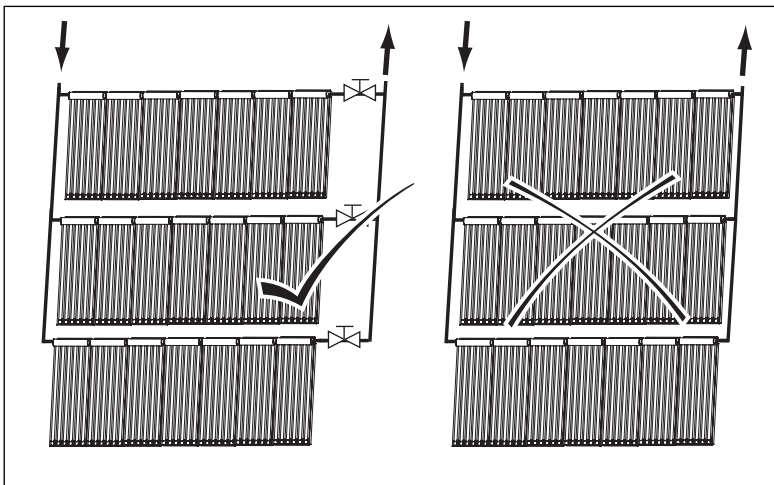
Abb. 4.10 Absperrventil in Kollektorvorlauf
