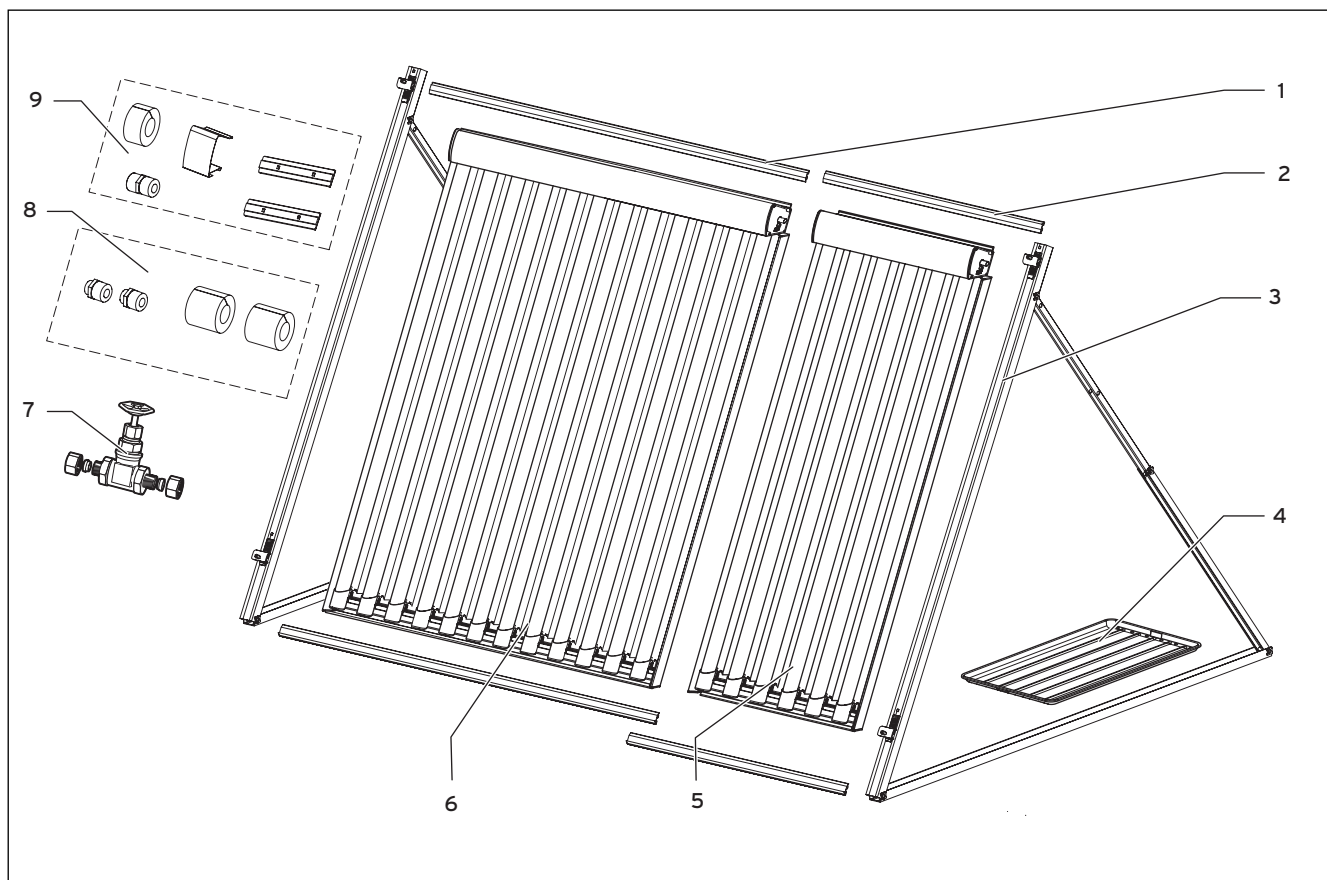
Abb. 4.2 Einbauset Flachdachmontage
