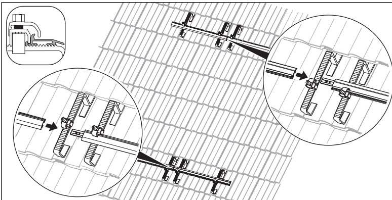
Abb. 5.10 Montageschienen verbinden
