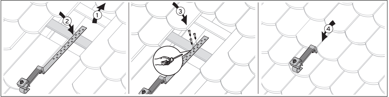
Abb. 5.7 Befestigung Dachanker Typ S flach
