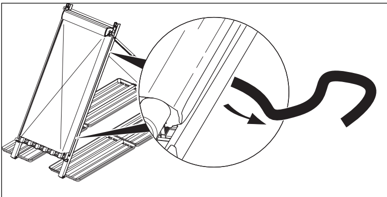
Abb. 6.11 Tragegurte entfernen
