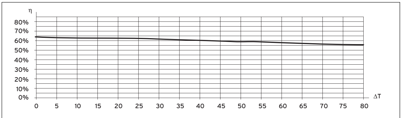
Abb. 10.4 Wirkungsgrad des VTK 570/2 und des VTK 1140/2 bei einer Einstrahlung EG von 800 W/m 2
