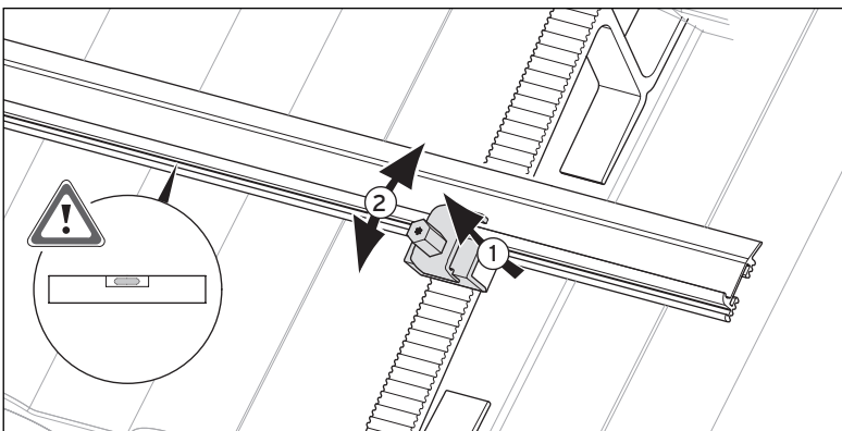
Abb. 5.11 Montageschienen austarieren
