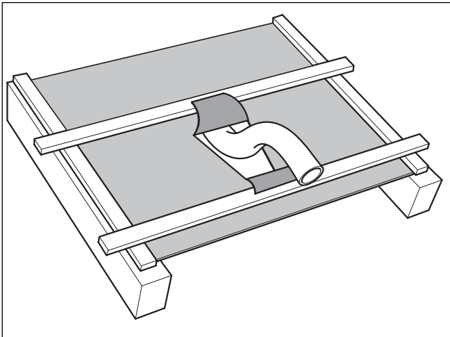
Abb 4.11 Rohr durch Unterspannbahn führen
