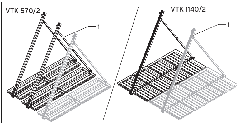
Abb. 6.4 Gestelle mit Kieswannen
