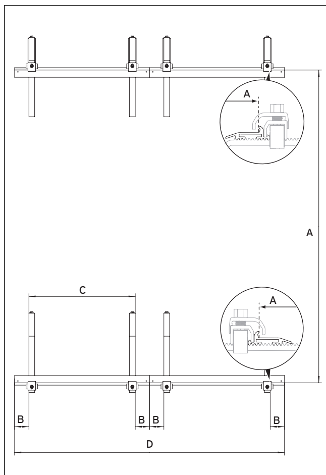
Abb. 5.1 Abstände bei Kollektoranordnung nebeneinander
