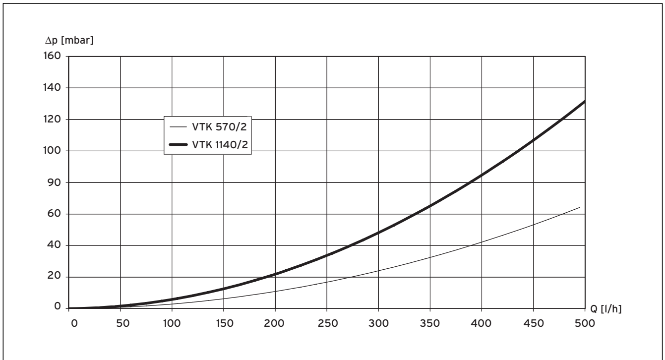
Abb. 10.5 Druckverlustdiagramm
