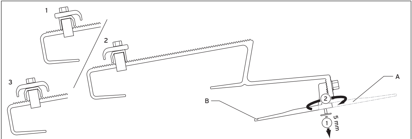
Abb. 5.3 Dachanker Typ P
