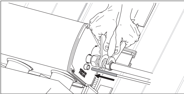
Abb. 5.21 Hydraulische Anschlüsse montieren
