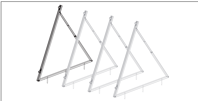
Abb. 6.5 Direktverschraubung
