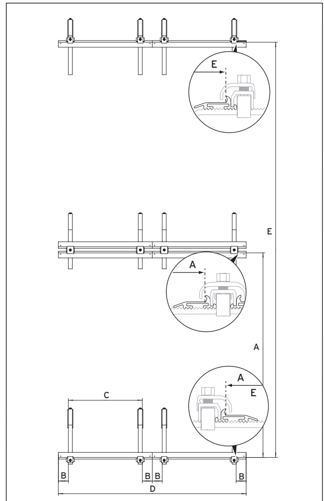
Abb. 5.2 Abstände bei Kollektoranordnung übereinander
