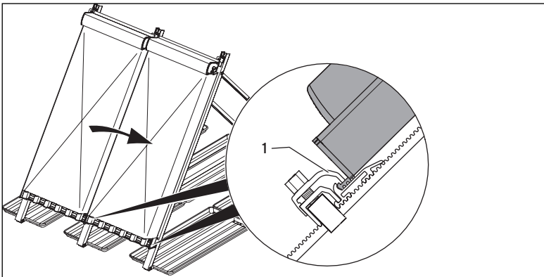
Abb. 6.12 Weitere Kollektoren montieren
