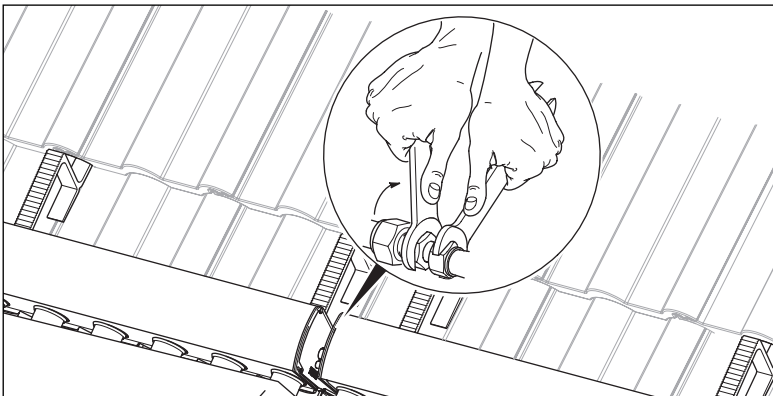
Abb. 5.17 Klemmringverbindung festziehen
