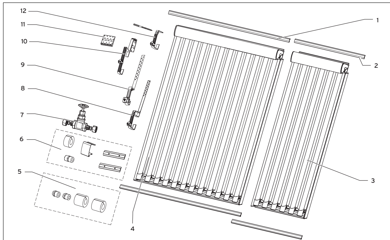
Abb. 4.1 Einbauset Aufdachmontage
