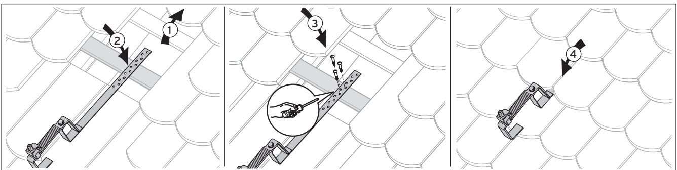
Abb. 5.6 Befestigung Dachanker Typ S
