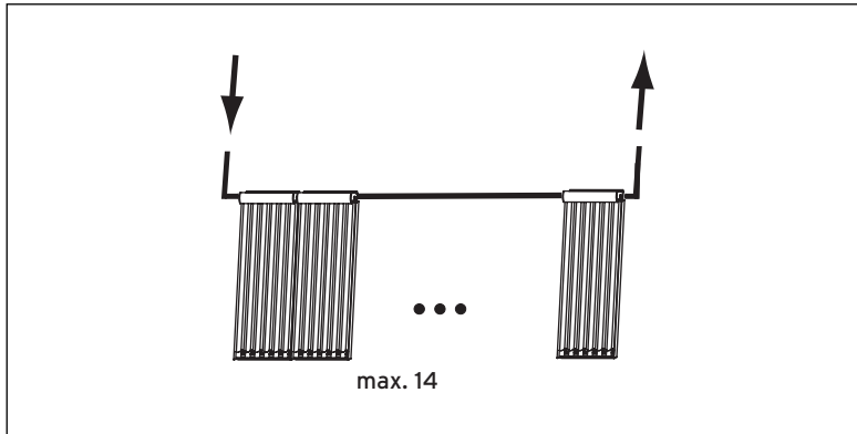
Abb. 4.6 Reihenschaltung VTK 570/2
