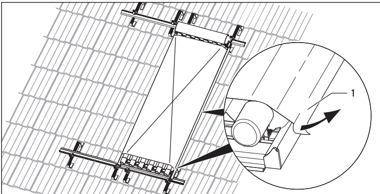
Abb. 5.13 Folie von Kollektorrändern ziehen
