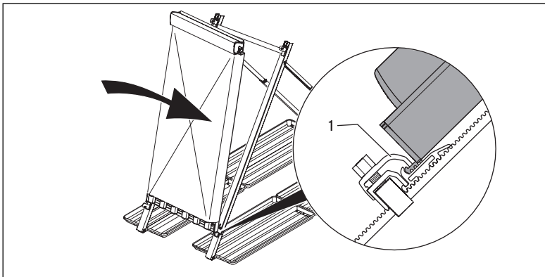
Abb. 6.9 Kollektor einhängen
