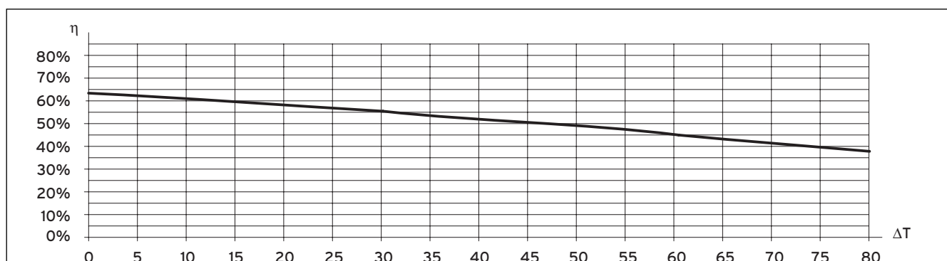
Abb. 10.3 Wirkungsgrad des VTK 570/2 und des VTK 1140/2 bei einer Einstrahlung EG von 300 W/m 2
