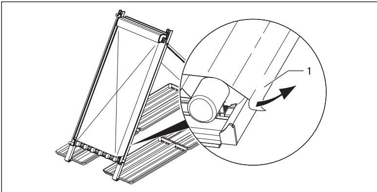
Abb. 6.10 Folie von Kollektorrändern ziehen
