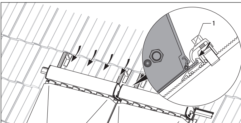
Abb. 5.18 Obere Montageschiene positionieren
