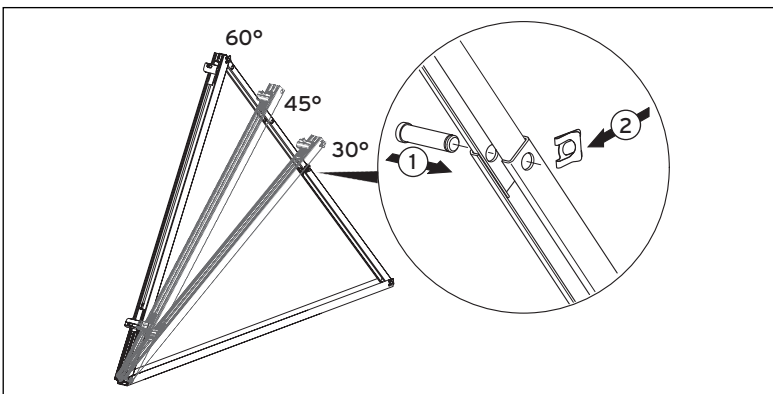
Abb. 6.3 Gestelle montieren
