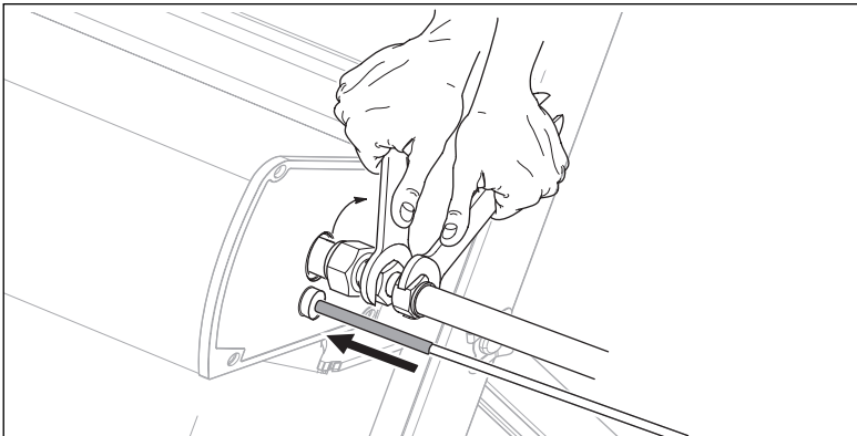
Abb. 6.16 Hydraulische Anschlüsse montieren
