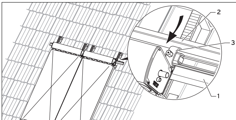
Abb. 5.19 Mittlere Montageschiene bei 2 oder 3 Kollektorreihen
