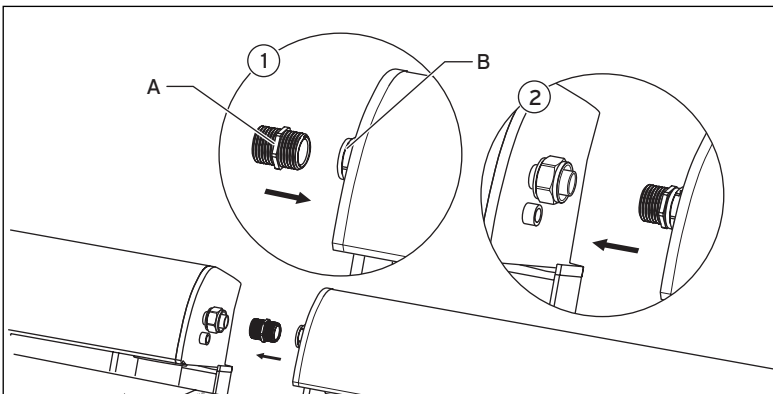
Abb. 5.16 Kollektoren verbinden
