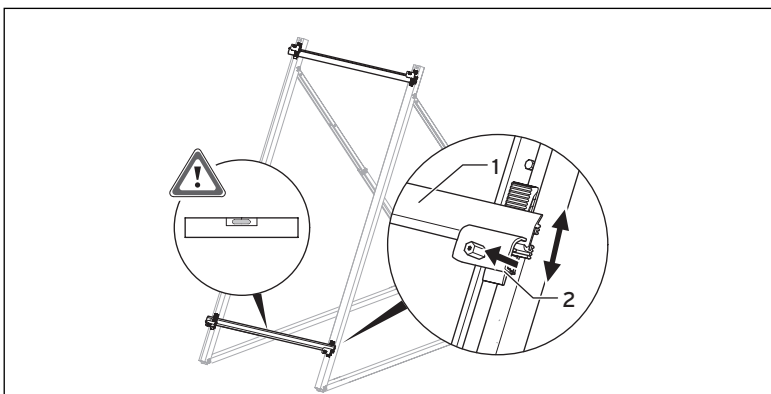
Abb. 6.6 Montageschienen befestigen und arretieren
