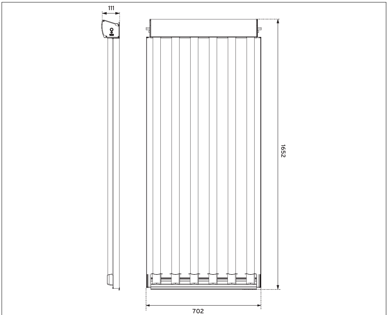
Abb. 10.1 Maßzeichnung VTK 570/2
