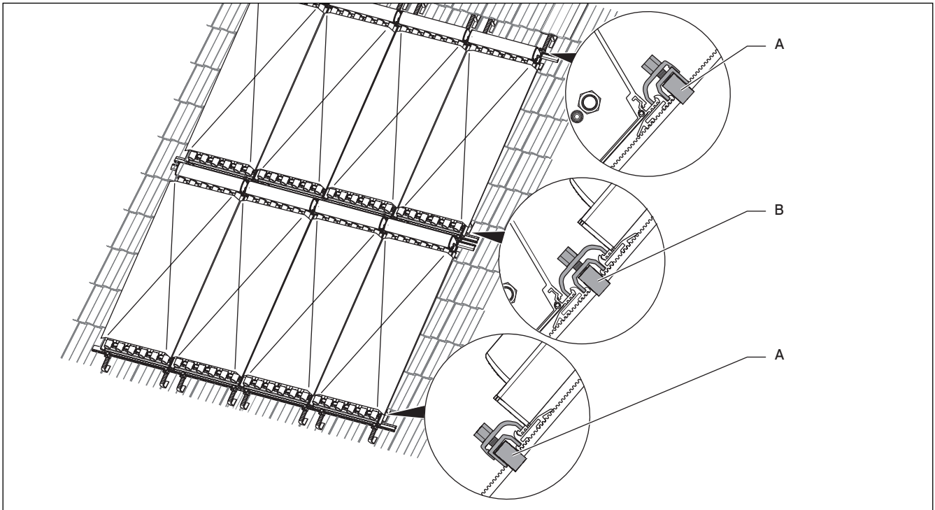
Abb. 4.4 Einbauset Aufdachmontage 2-reihig (hier: VTK 570/2)
