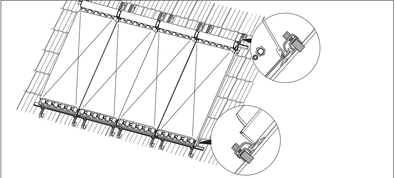
Abb. 4.3 Einbauset Aufdachmontage 1-reihig (hier: VTK 570/2)
