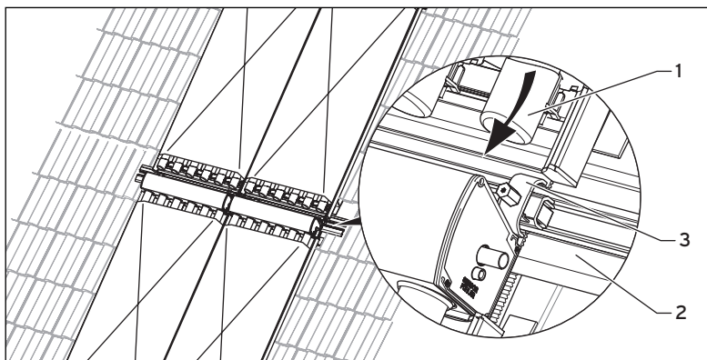
Abb. 5.20 Mittlere Montageschiene bei 2 oder 3 Kollektorreihen
