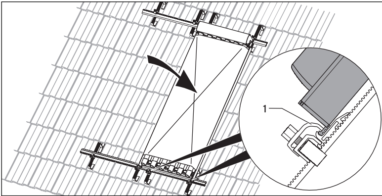
Abb. 5.12 Kollektor einhaken
