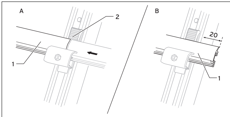
Abb. 6.7 Positionierung der Montageschienen
