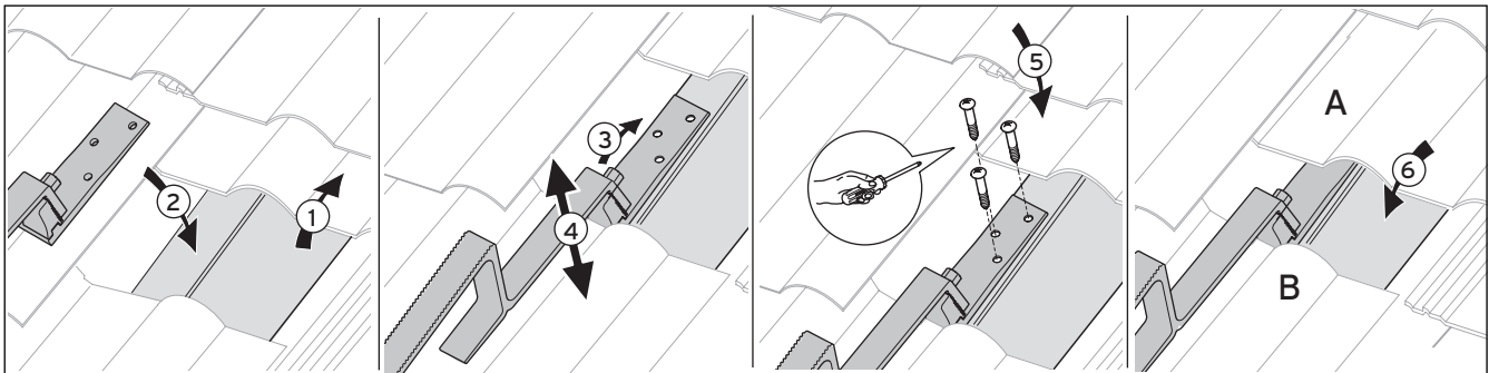
Abb. 5.4 Befestigung am Dachsparren
