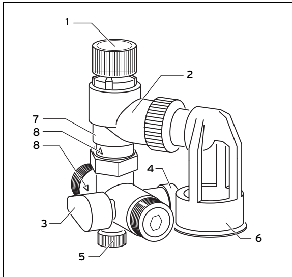
Abb. 3.1 Sicherheitsgruppe
