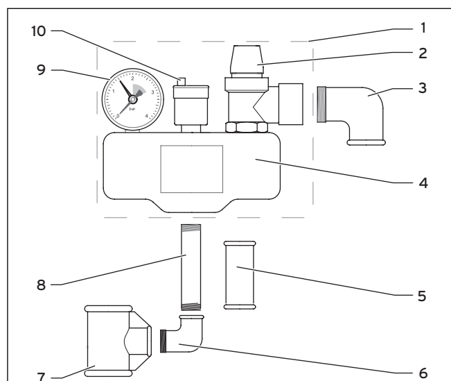
Afb. 3.1 Veiligheidsgroep
