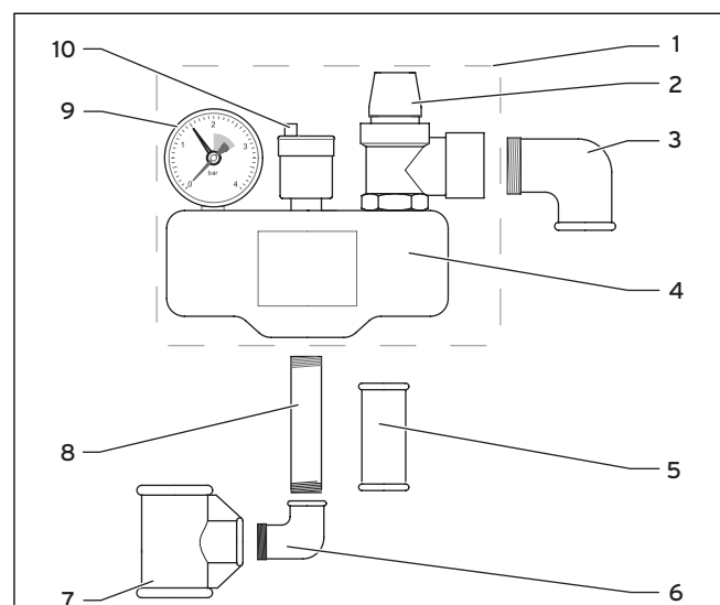
Abb. 3.1 Sicherheitsgruppe
