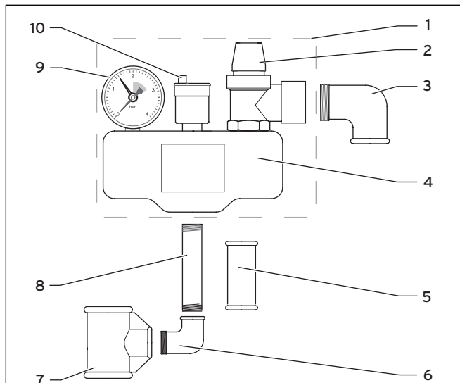
Rys. 3.1 Grupa bezpieczeństwa
