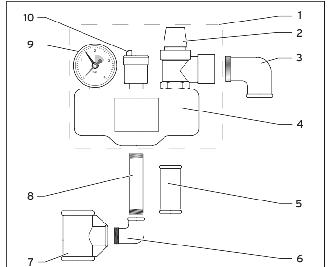
Şekil 3.1 Emniyet grubu
