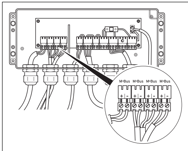
Fig. 5.11L Collegamento dei componenti bus M
