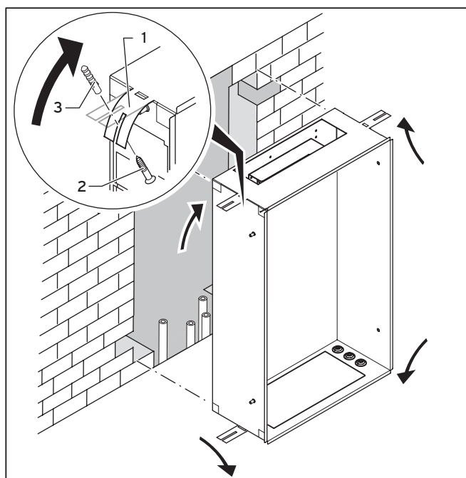
Fig. 4.6 Montaggio della cassetta da parete, uniSAT VSW 15-35 I
