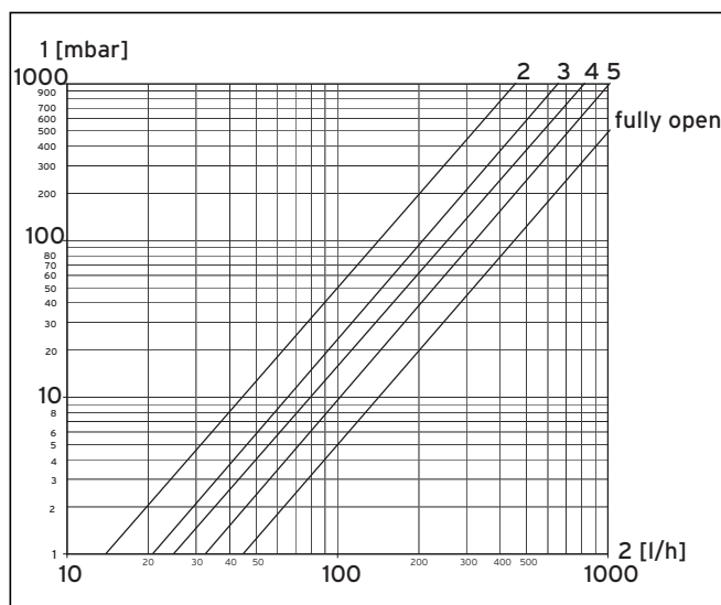
Fig. 7.1 Curve di perdita della pressione con regolazione della valvola di zona senza regolatore a temperatura differenziale
