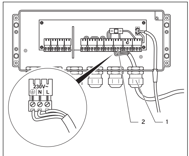
Abb. 5.13 Anschluss der Netzzuleitung
