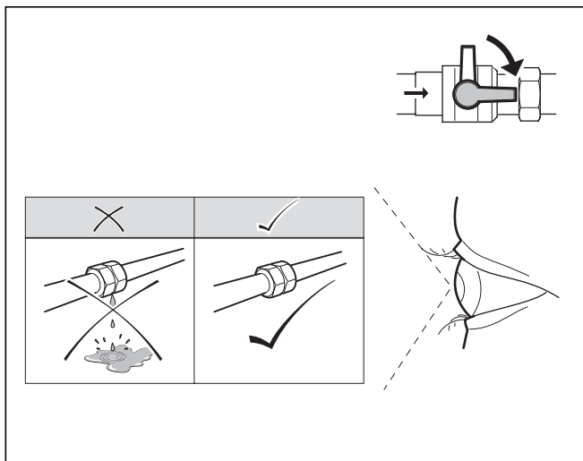
Abb. 6.1 Funktionsprüfung
