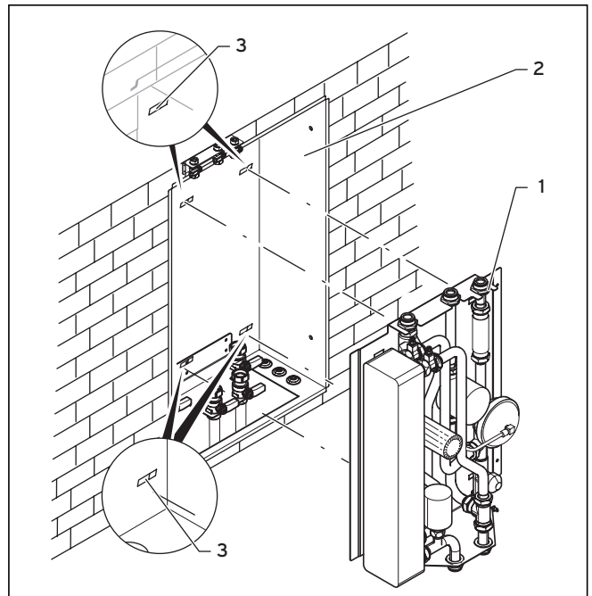
Abb. 4.10 Hydraulikmodul einsetzen uniSAT VSW 15-35 I
