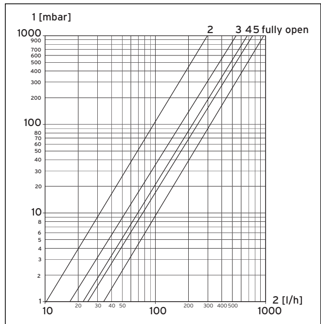
Abb. 7.2 Druckverlustkurven bei Einstellung des Zonenventils mit Differenzdruckregler
