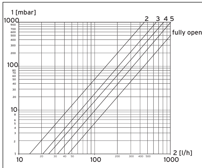
Abb. 7.1 Druckverlustkurven bei Einstellung des Zonenventils ohne Differenzdruckregler
