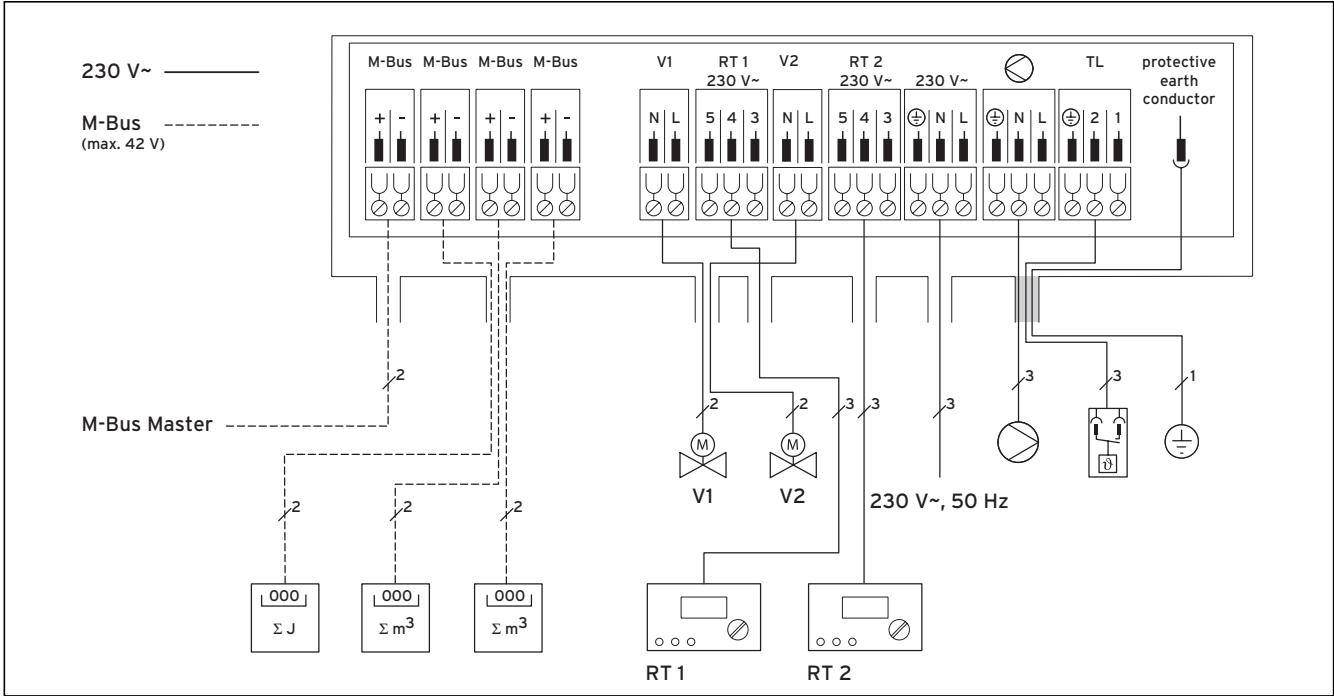
Fig. 5.7 Schema allacciamenti
