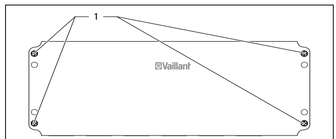
Abb. 5.5 Verdrahtungsbox öffnen
