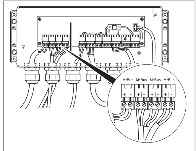
Abb. 5.14 Anschluss der M-BUS-Komponenten
