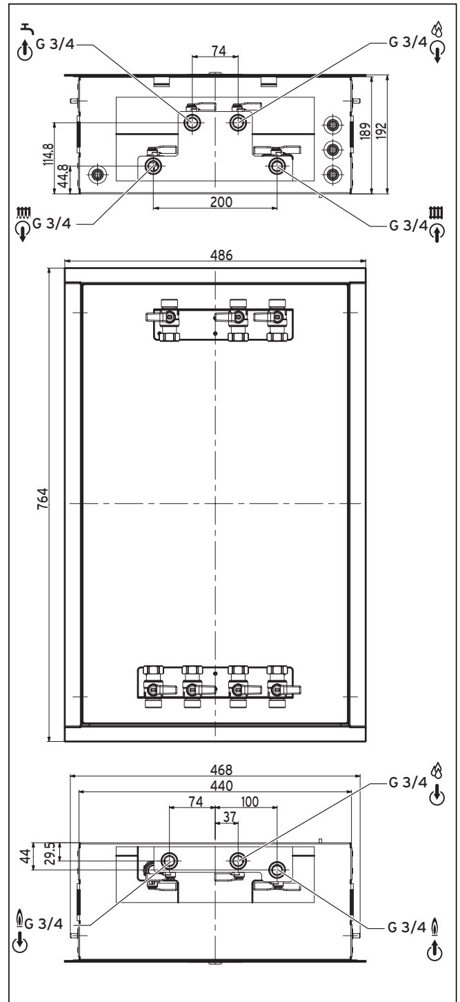
Abb. 4.4 Anschlussmaße uniSAT VSW 15-35 I (in mm)
