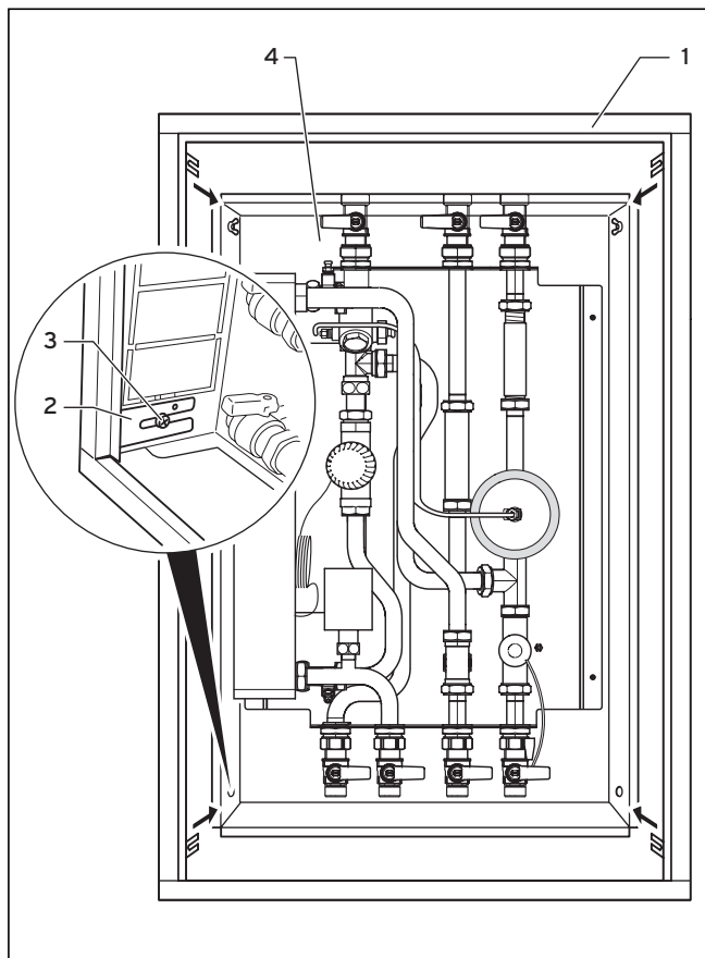
Fig. 4.8 Montaggio dell'intelaiatura, uniSAT VSW 15-35 I
