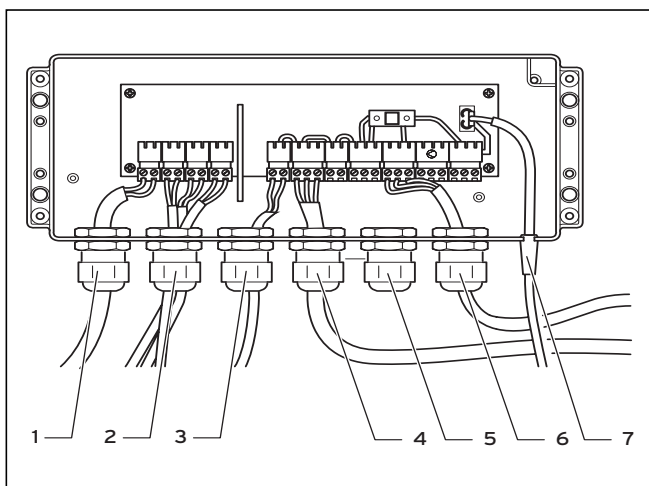
Abb. 5.11 Belegung Verdrahtungsbox
