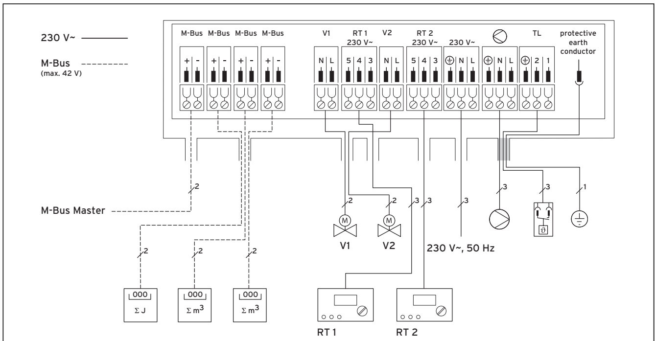
Abb. 5.10 Anschlussplan
