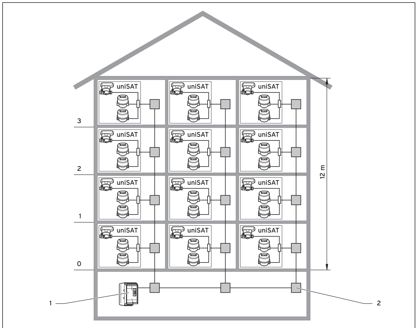
Fig. 5.12 Installazione bus M: condotto cavi a fascio
