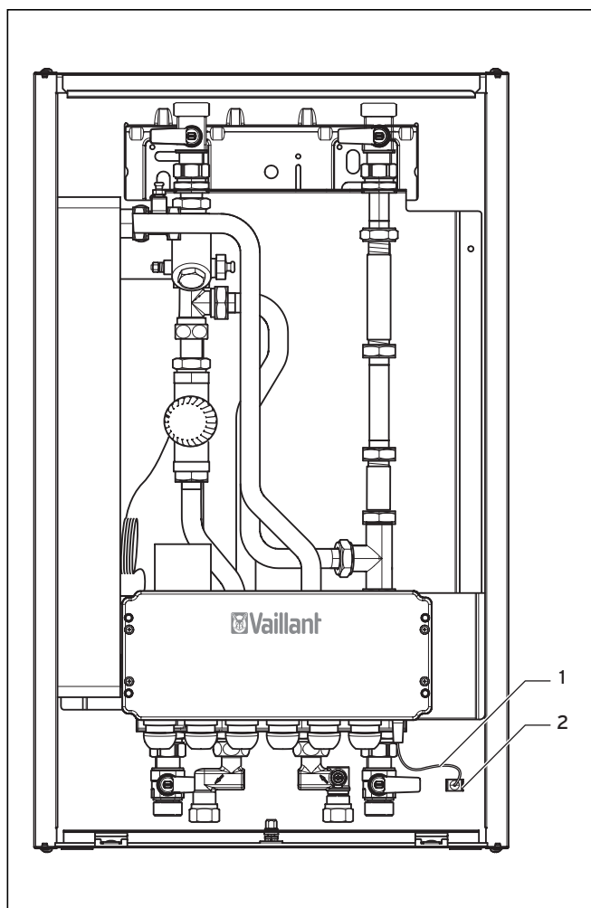
Fig. 5.5 Collegamento del cavo di guardia tra la scatola di cablaggio e l'alloggiamento dell'uniSAT
