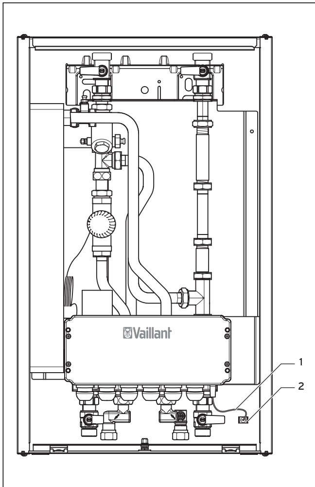
Abb. 5.8 Schutzleiterverbindung zwischen Verdrahtungsbox und Gehäuse des uniSAT
