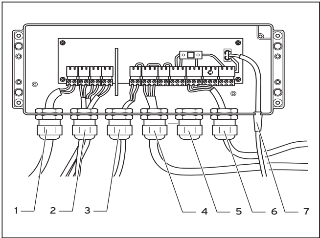
Fig. 5.8 Impiego dei cavi nella scatola
