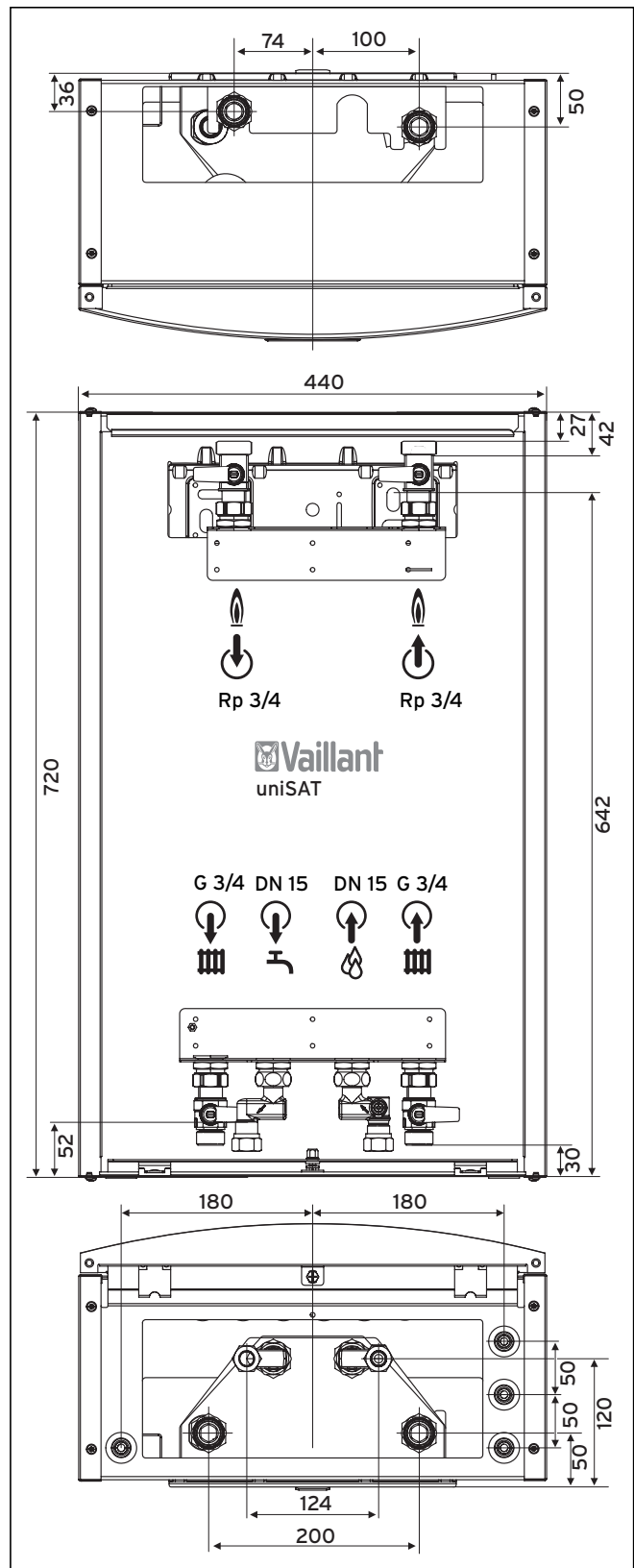
Abb. 4.12 Montageschablone/Montagefreiräume
