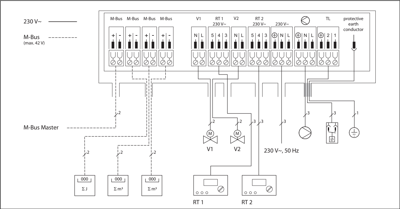
Fig. 5.6 Schema allacciamenti
