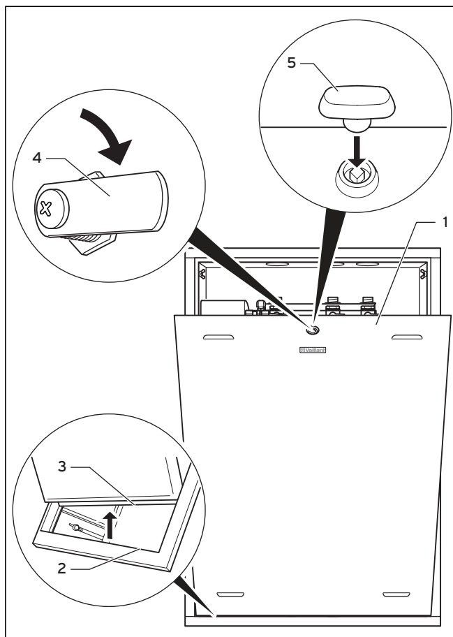
Abb. 4.8 Verkleidungstr ffnen uniSAT VSW 15-35 I
