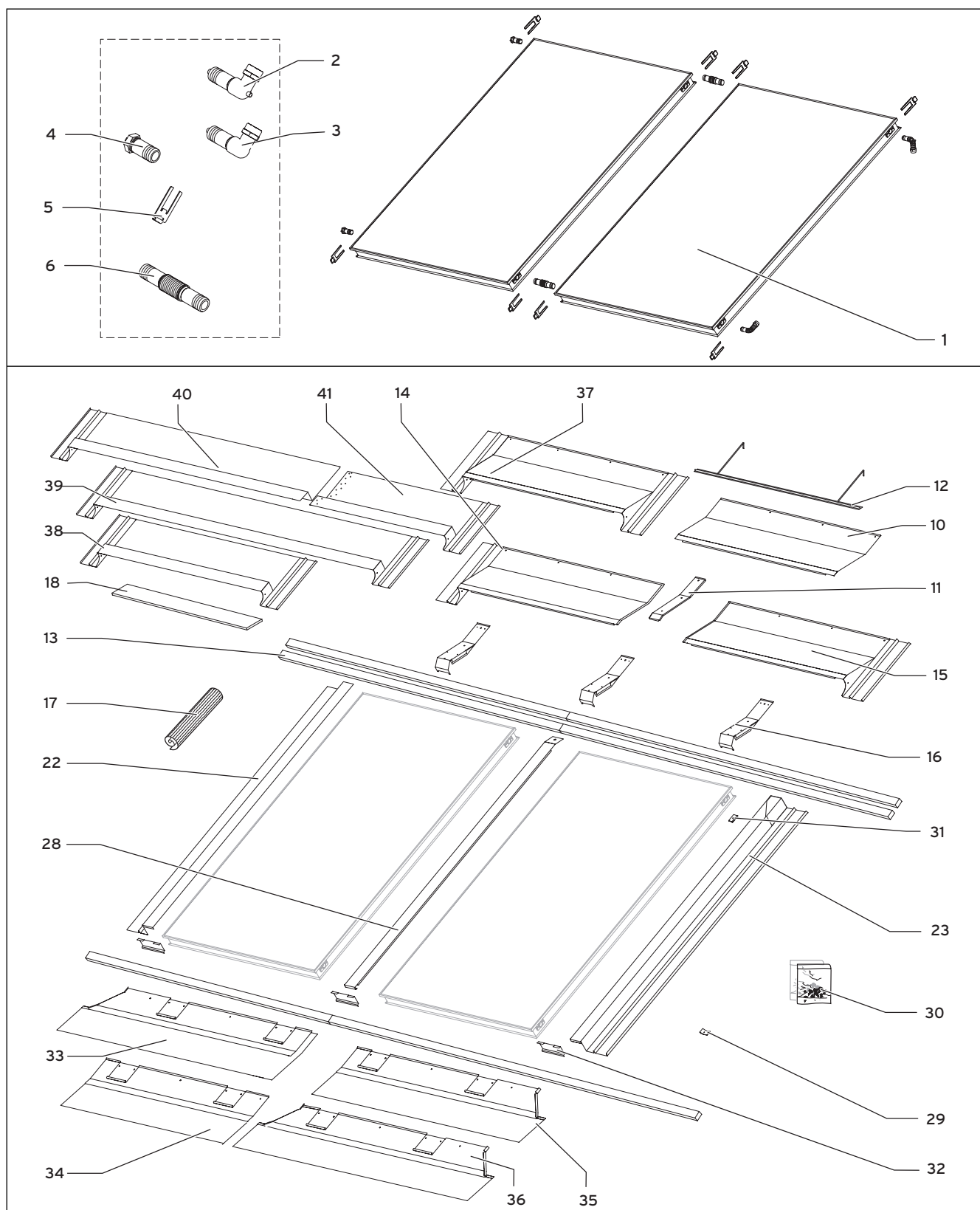
Abb. 5.3 Einbauset vertikaler Kollektor (VFK 145/150 V)
