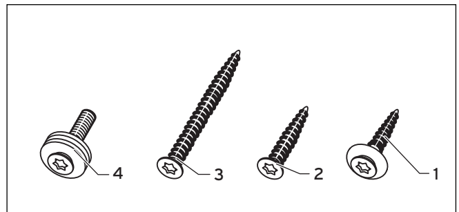
Abb. 5.6 Lieferumfang Schraubenset
