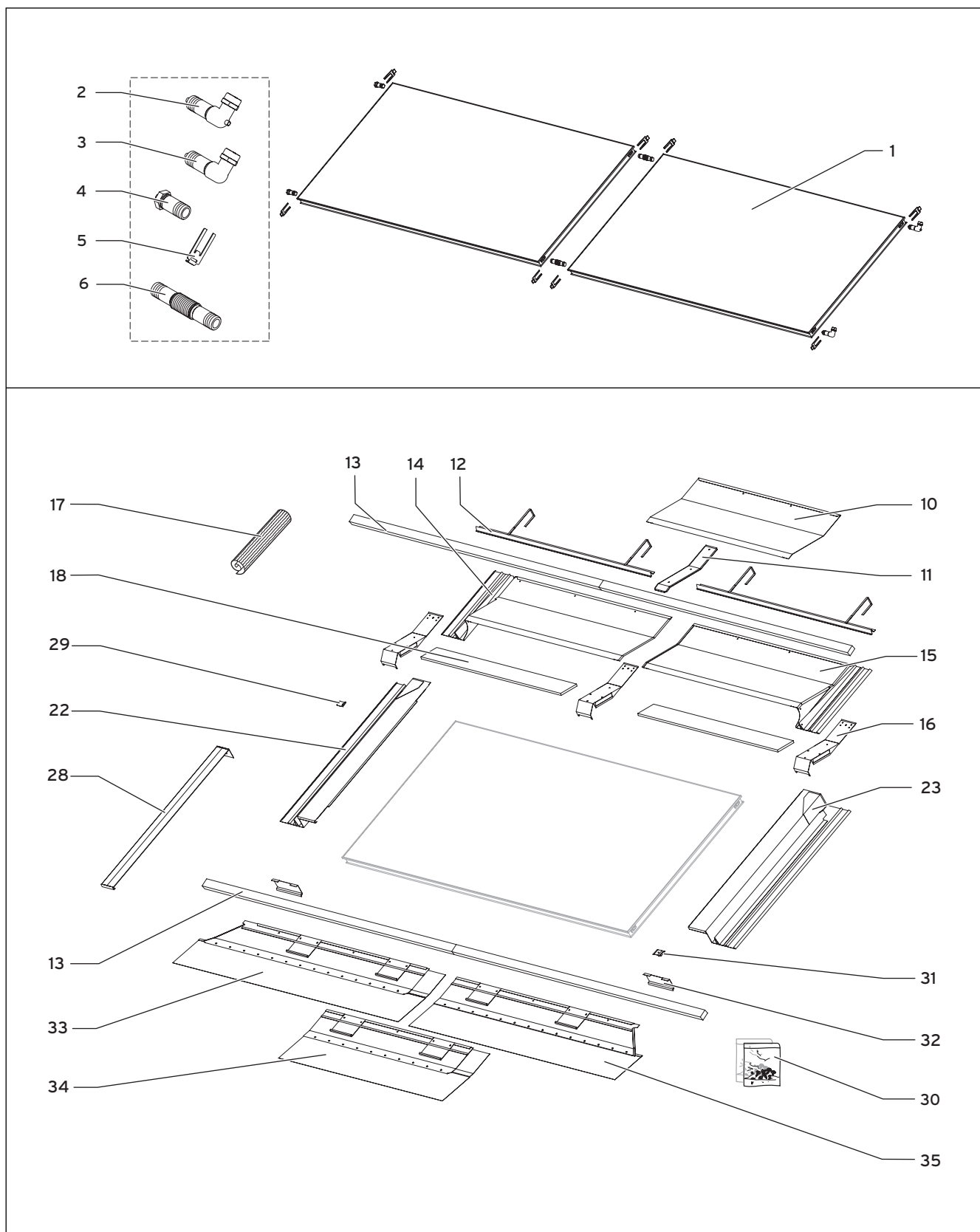
Abb. 5.5 Einbauset horizontaler Kollektor (VFK 145/150 H)
