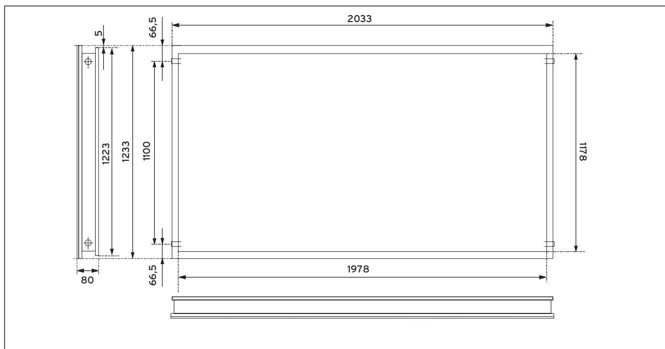
Abb. 9.1 Maßzeichnung VFK 145 H, VFK 150 H
