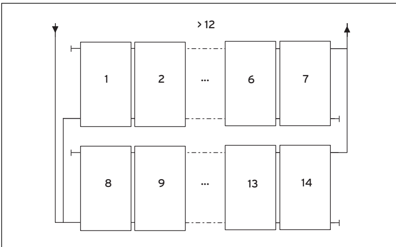
Abb. 4.4 Parallelverschaltung (hier dargestellt: 145V / 150V)
