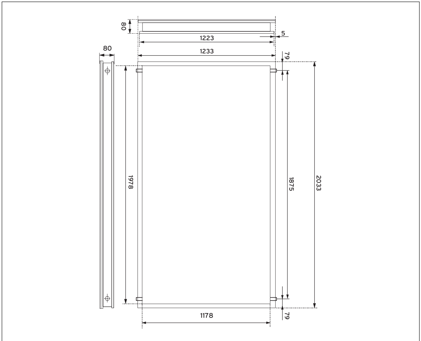
Abb. 9.2 Maßzeichnung VFK 145 V, VFK 150 V
