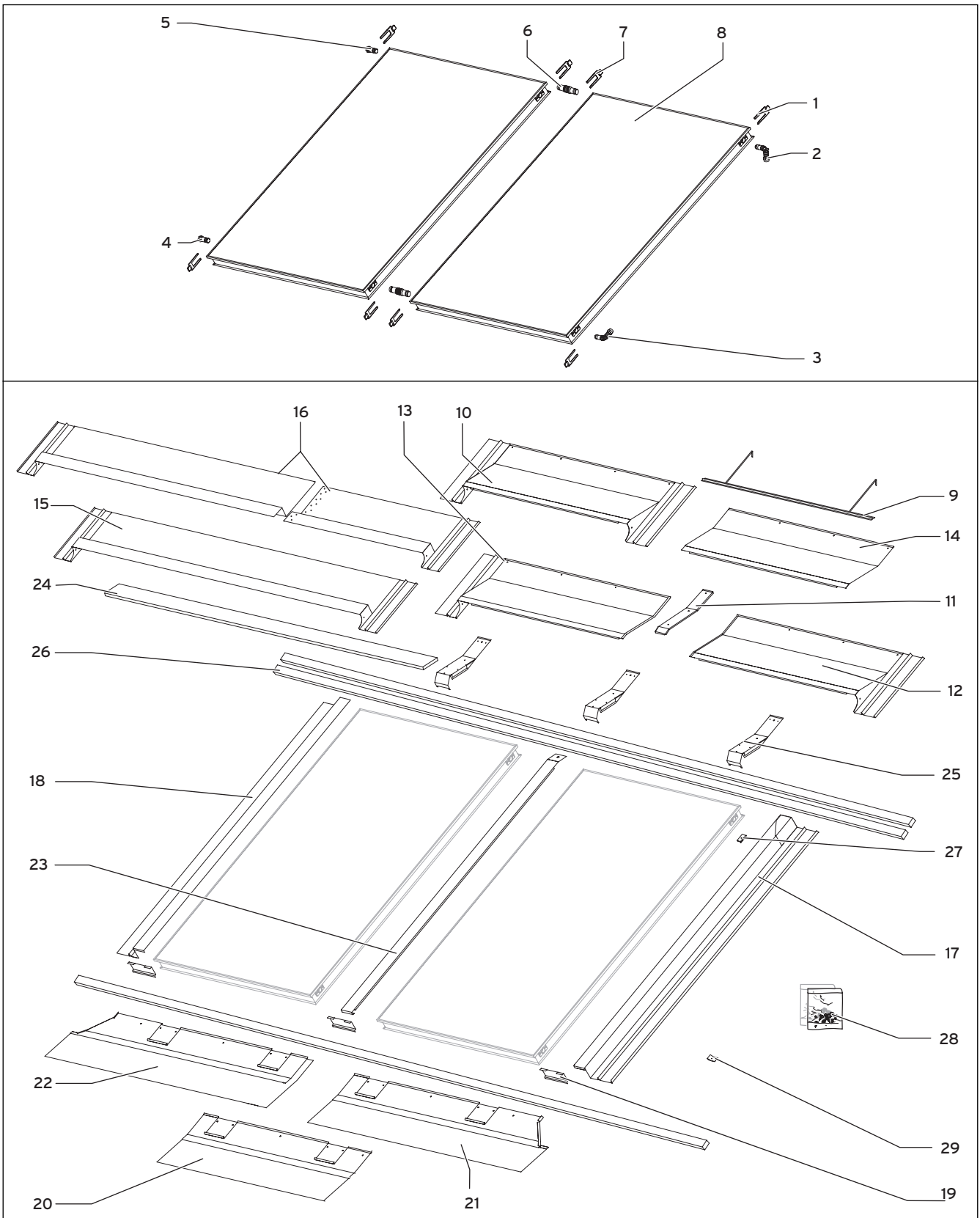
Abb. 4.1 Einbauset vertikaler Kollektor
