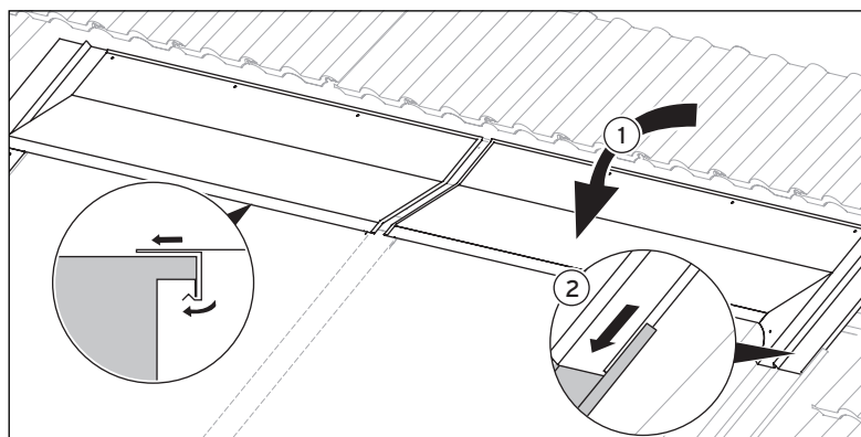
Abb. 4.35 Firstbleche anbringen
