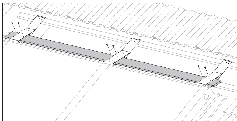
Abb. 4.34 Stützbretter anbringen
