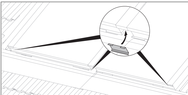
Abb. 4.39 Profilabschlüsse abdecken
