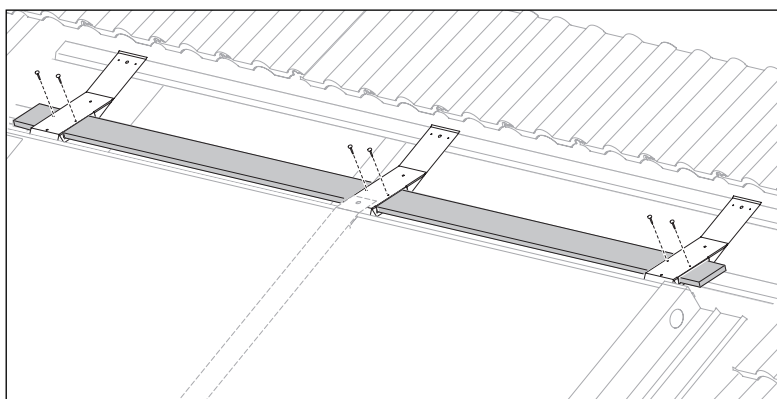
Abb. 4.34 Stützbretter anbringen
