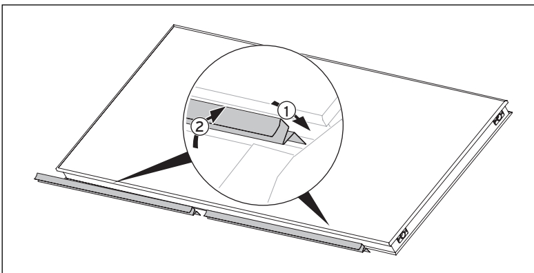
Abb. 4.16 Kollektor vorbereiten
