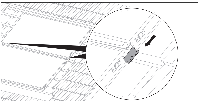
Abb. 4.17 Kollektor anordnen
