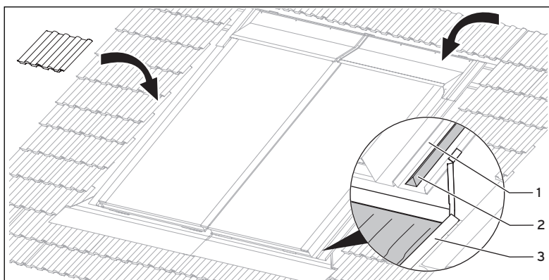
Abb. 4.43 Dach decken
