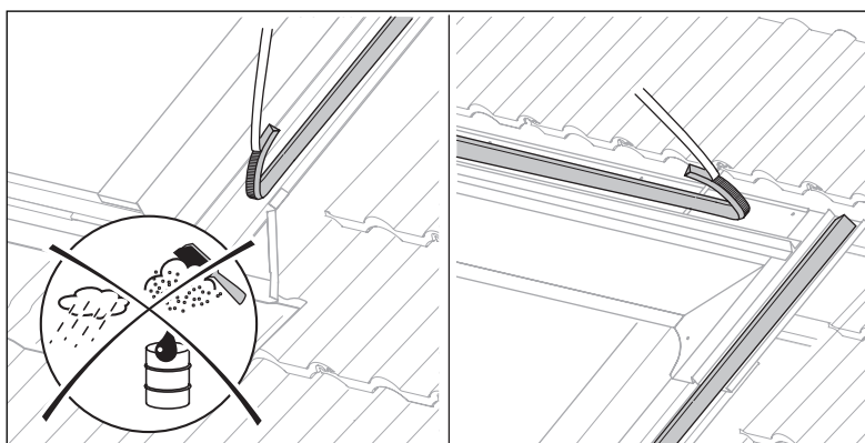
Abb. 4.42 Schaumstoffdichtkeil anbringen
