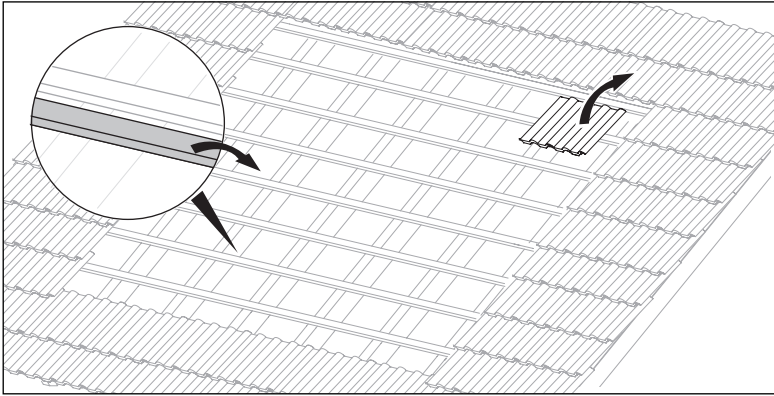
Abb. 4.10 Einbaufeld festlegen
