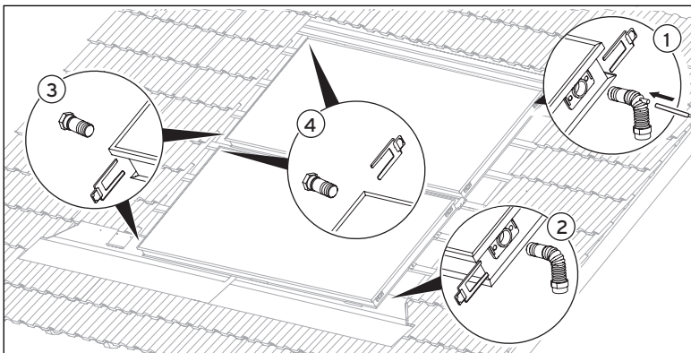
Abb. 4.19 Hydraulische Anschlüsse VFK 145/150
