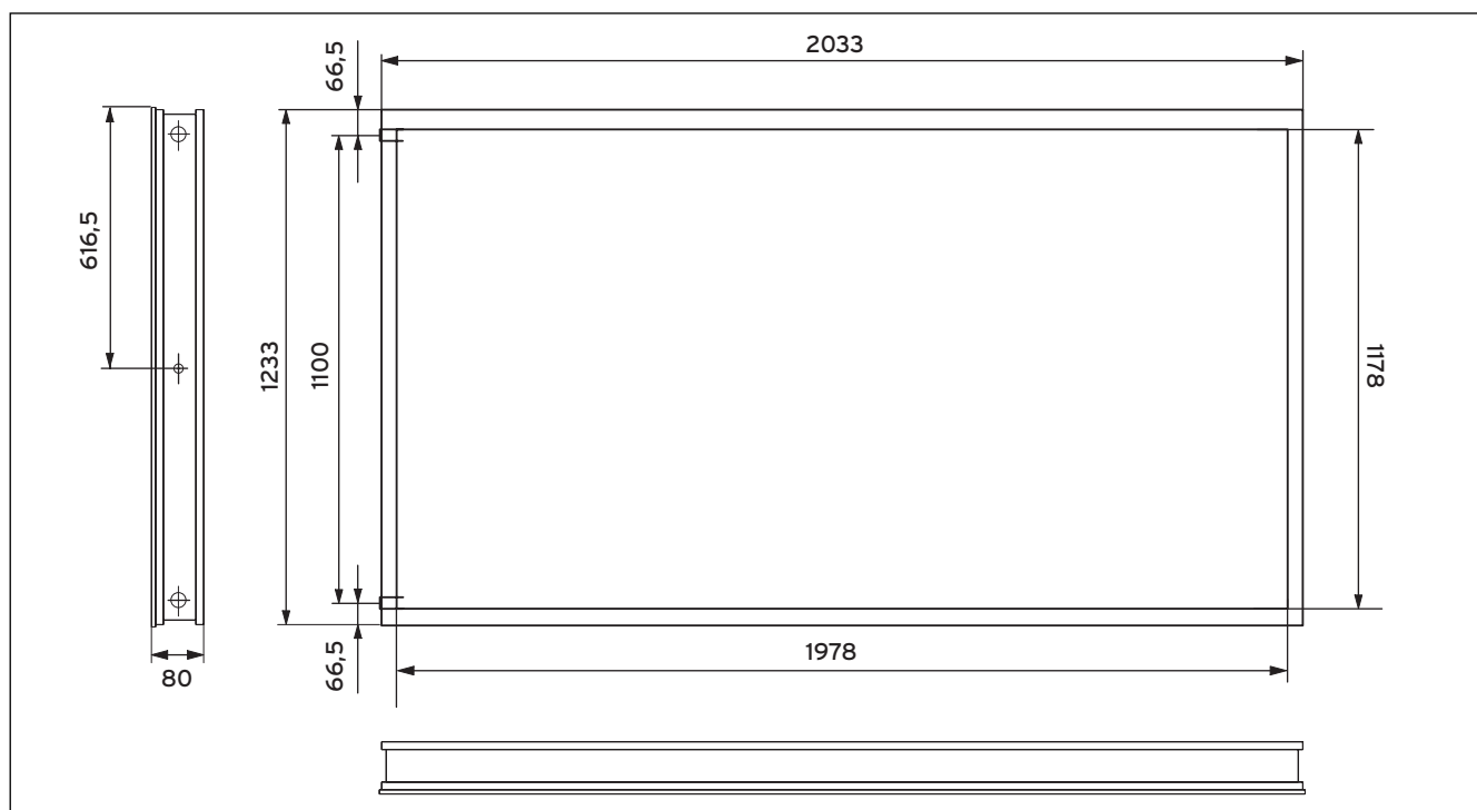
Abb. 7.2 Maßzeichnung VFK 135 D
