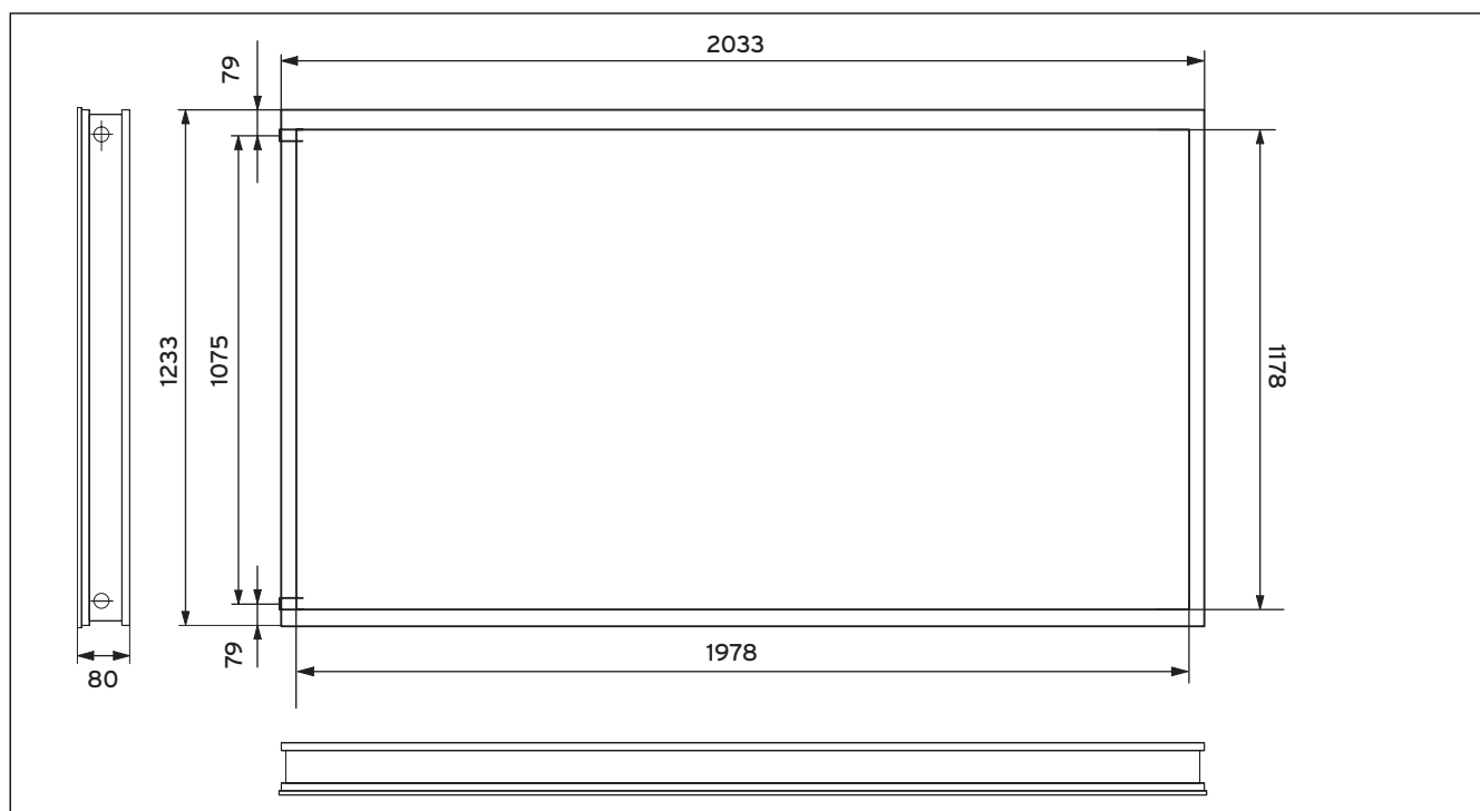
Abb. 7.1 Maßzeichnung VFK 145 H, VFK 150 H
