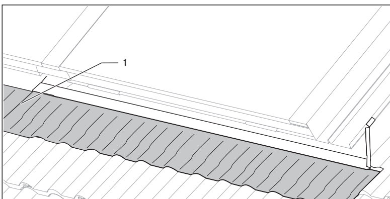
Abb. 4.39 Bleischürze anpassen
