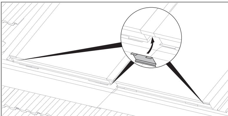
Abb. 4.38 Profilabschlüsse abdecken
