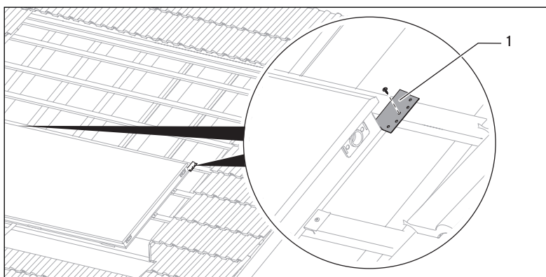
Abb. 4.15 Platzhalter anschrauben
