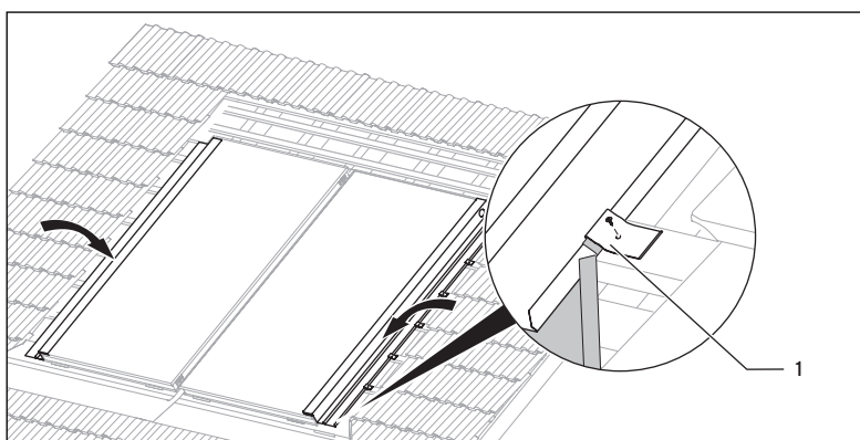
Abb. 4.28 Seitenteile festschrauben
