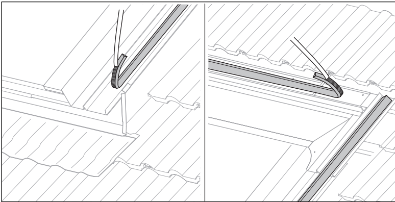
Abb. 4.40 Schaumstoffdichtkeil anbringen
