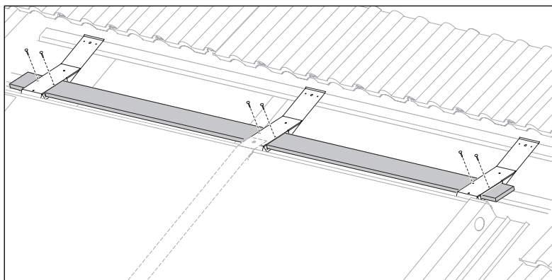
Abb. 4.33 Stützbretter anbringen
