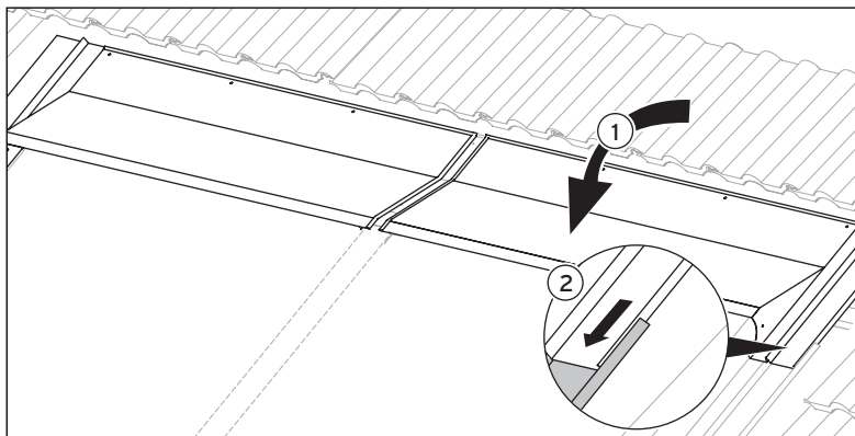
Abb. 4.34 Firstbleche anbringen
