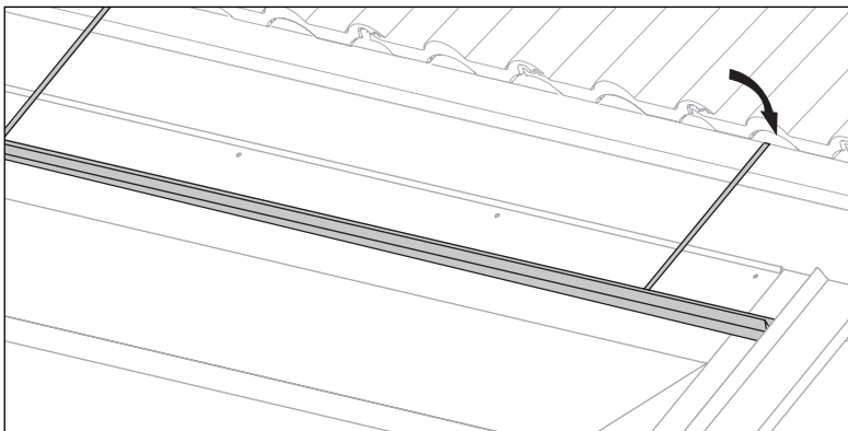
Abb. 4.37 Profilabschlüsse abdecken
