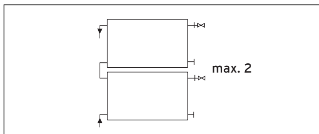
Abb 4.5 Feldanordnung übereinander
