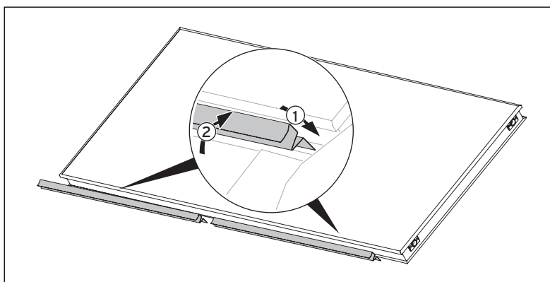
Abb. 4.16 Kollektor vorbereiten
