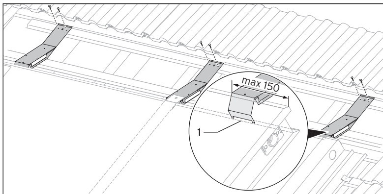
Abb. 4.32 Stützbleche anbringen
