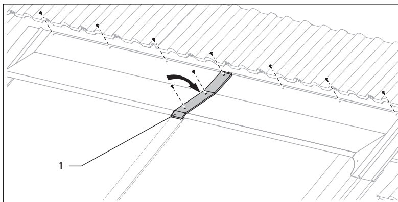
Abb. 4.35 Firstblechverbinder
