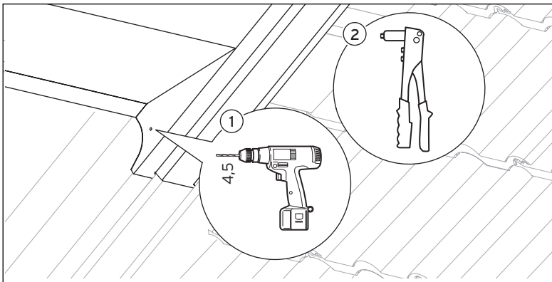
Abb. 4.36 Rahmen vernieten
