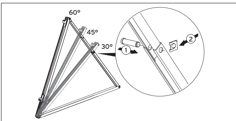
Abb. 5.4 Gestelle montieren
