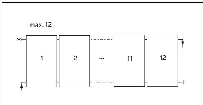
Abb. 4.4 Feldanordnung nebeneinander für 6 - 12 Kollektoren
