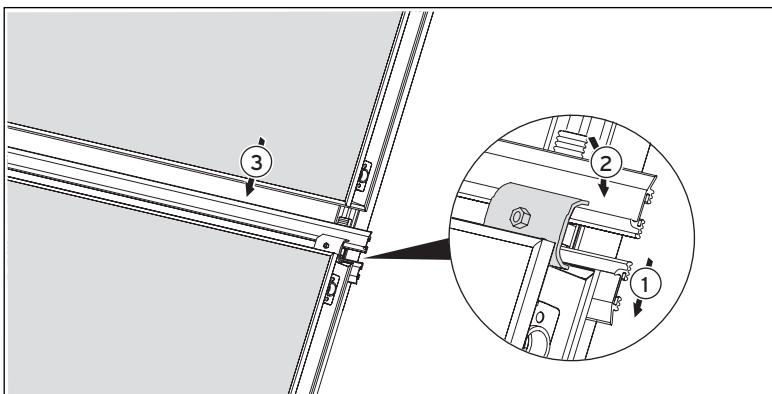
Abb. 5.16 Mittlere Montageschiene
