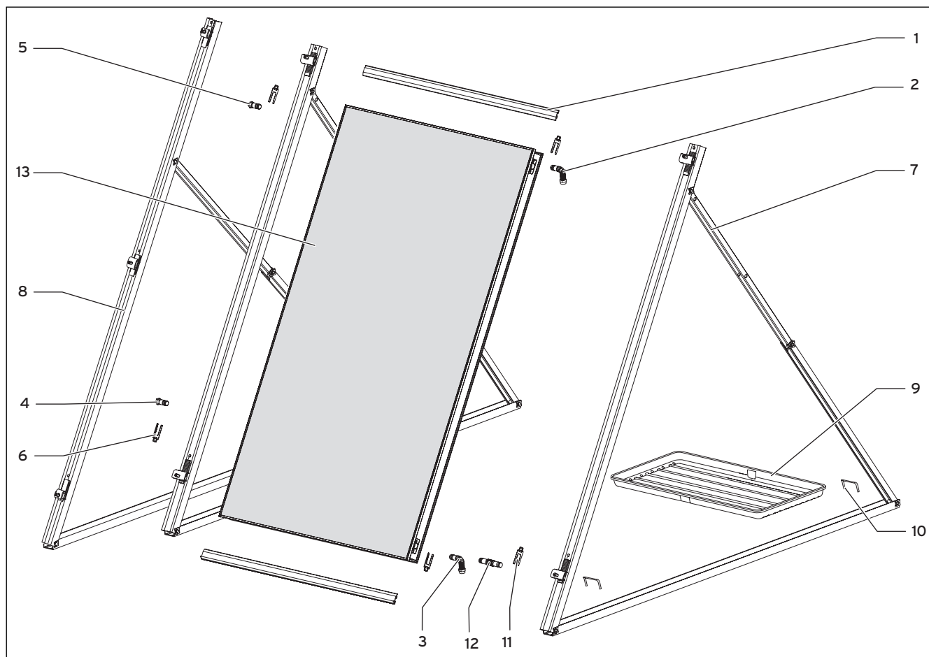
Abb. 4.2 Einbauset für vertikale und horizontale Flachdachmontage (hier: Vertikaler Kollektor)
