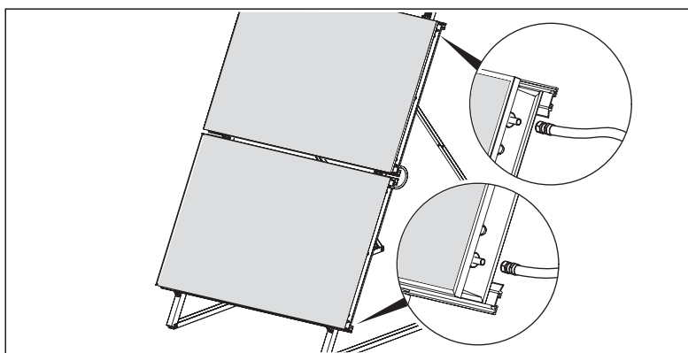
Abb. 5.19 Hydraulischer Anschluss bei Drainback-Kollektoren
