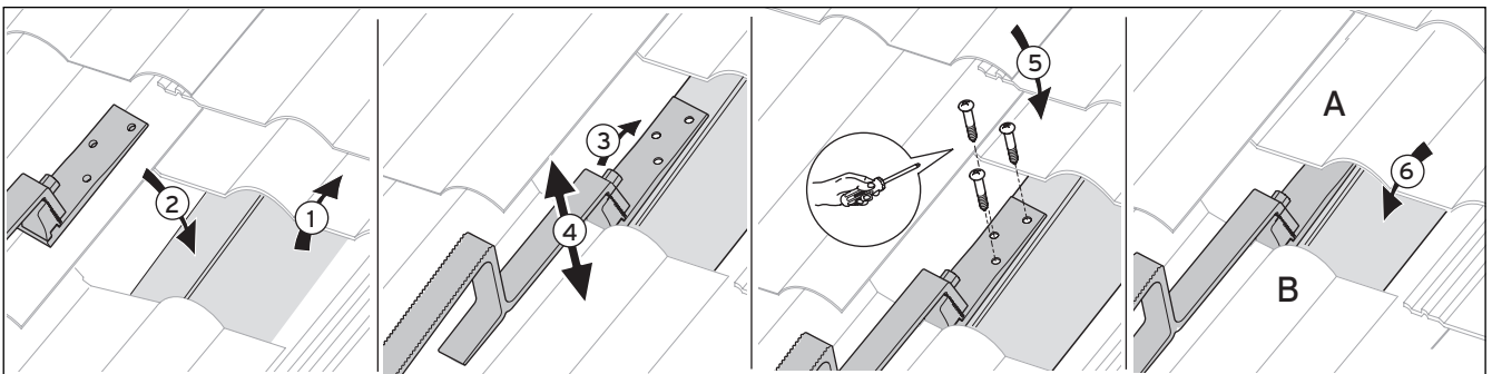
Abb. 6.4 Befestigung am Dachsparren
