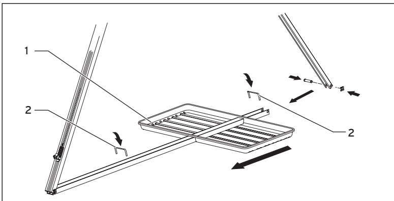
Abb. 5.3 Kieswannen montieren
