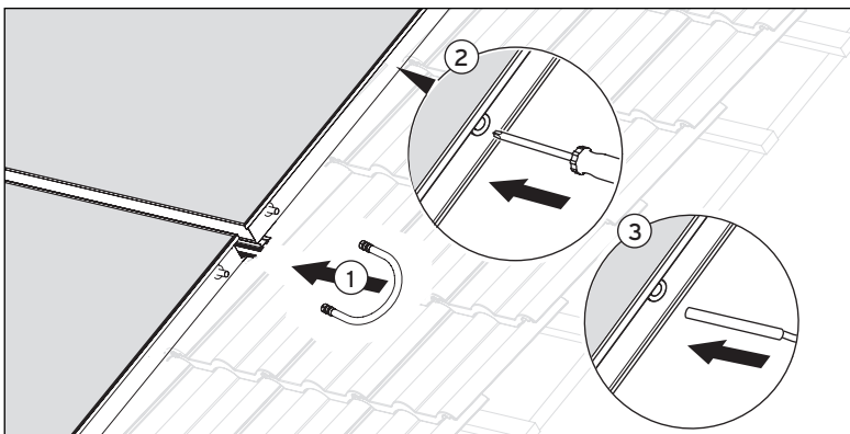
Abb. 6.20 Anschluss der Drainback-Kollektoren untereinander
