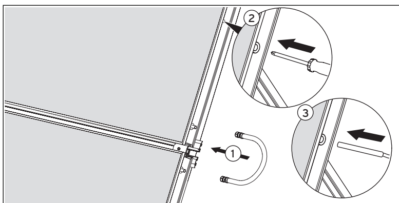
Abb. 5.18 Anschluss der Drainback-Kollektoren untereinander
