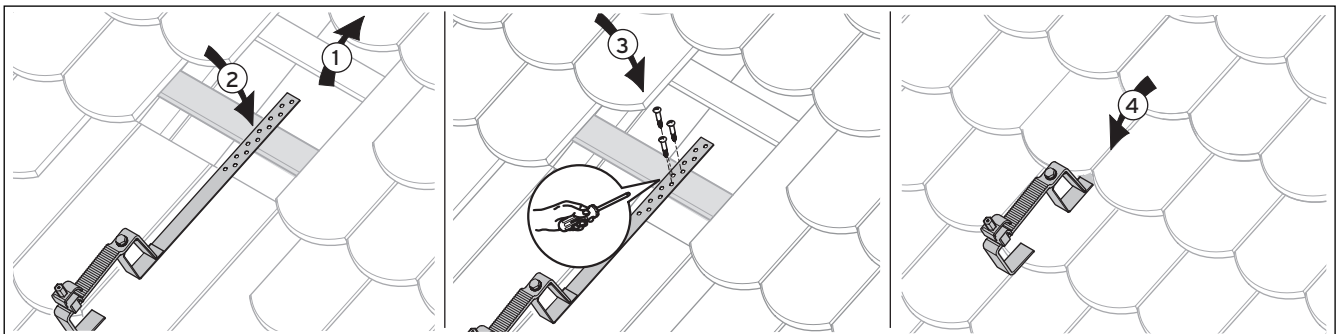
Abb. 6.6 Befestigung Dachanker Typ S
