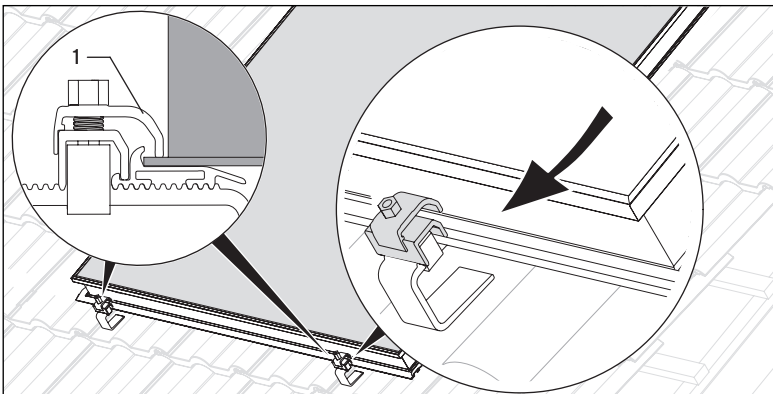
Abb. 6.10 Kollektor einhängen
