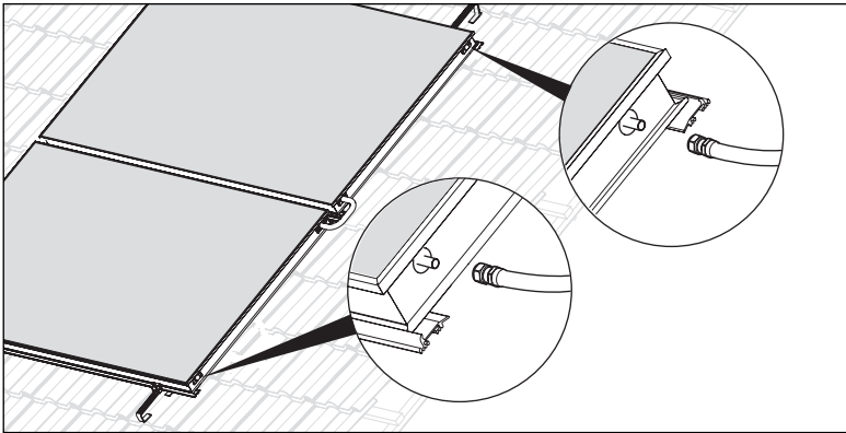
Abb. 6.21 Hydraulischer Anschluss bei Drainback-Kollektoren
