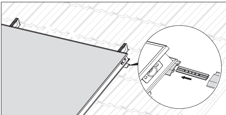
Abb. 6.13 Bei Feldanordnung nebeneinander Montageschienen verbinden
