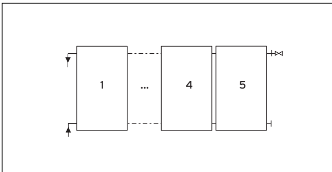
Abb. 4.3 Feldanordnung nebeneinander für 1 - 5 Kollektoren
