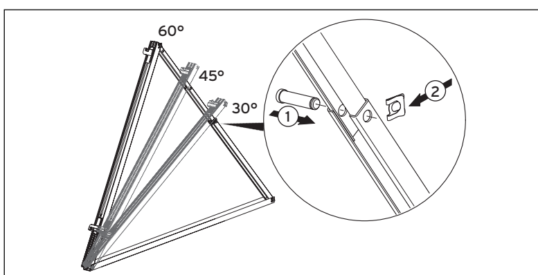
Abb. 5.4 Gestelle montieren
