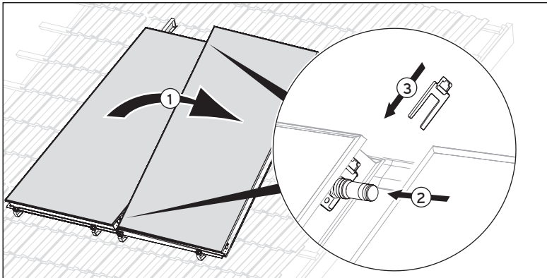
Abb. 6.15 Bei Feldanordnung nebeneinander weitere Kollektoren montieren
