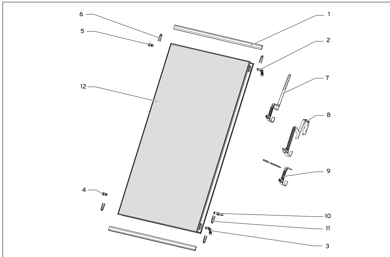
Abb. 4.1 Einbauset Aufdachmontage (hier: Vertikaler Kollektor)
