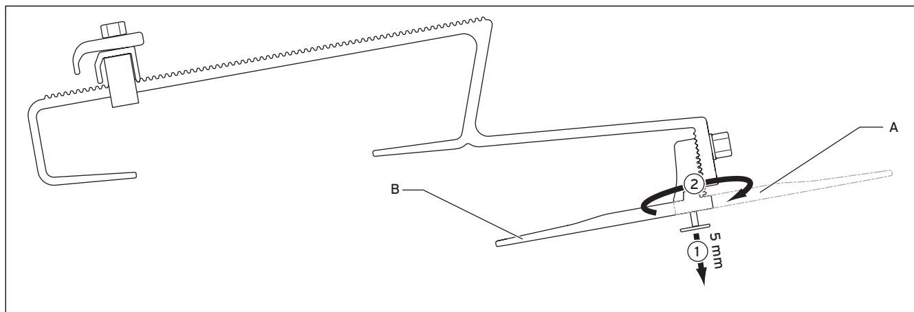
Abb. 6.3 Dachanker Typ P
