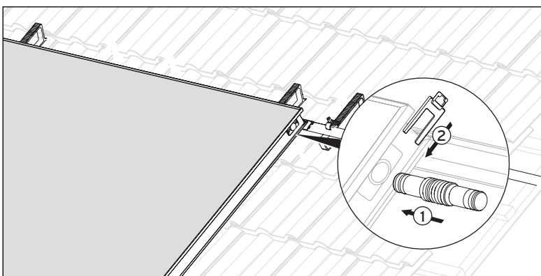
Abb. 6.14 Bei Feldanordnung nebeneinander Verbindungsstücke anbringen
