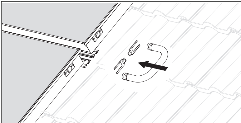
Abb. 6.18 Verbindung der Kollektoren untereinander
