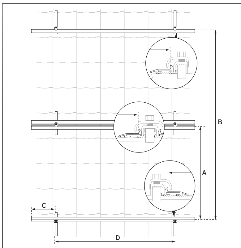
Abb. 6.2 Montageschienen bei Feldanordnung übereinander
