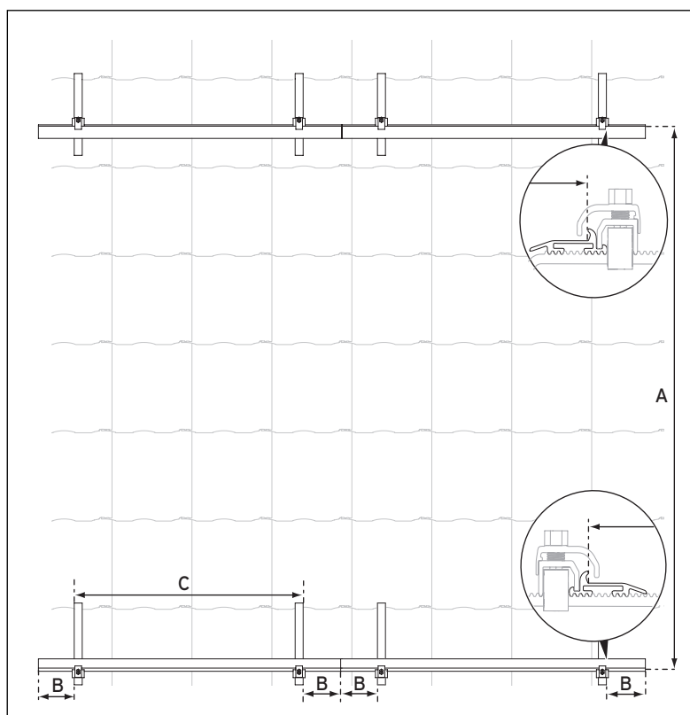
Abb. 6.1 Montageschienen bei Feldanordnung nebeneinander
