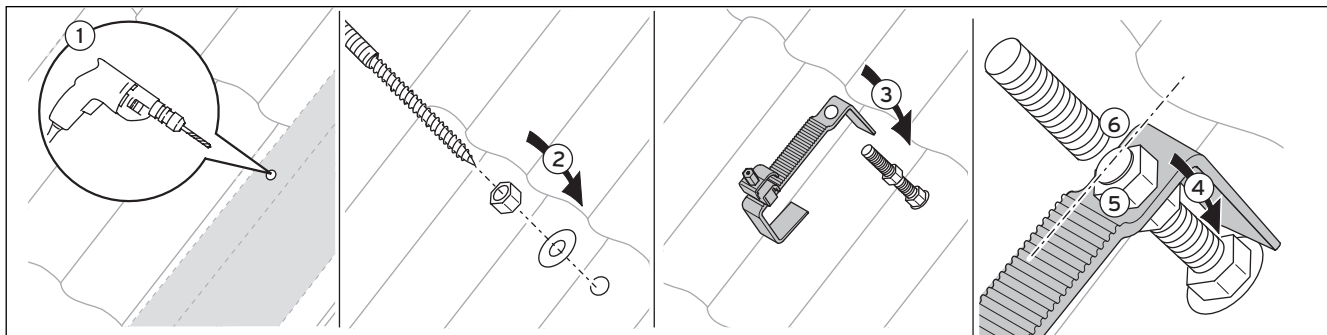
Abb. 6.7 Befestigung mit Stockschaube
