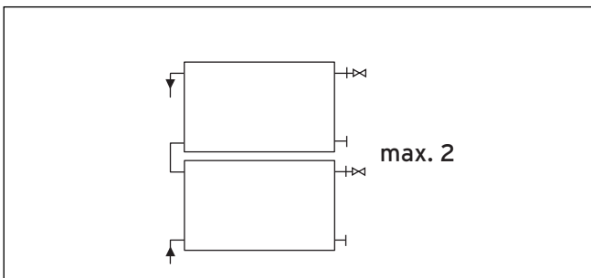
Abb 4.5 Feldanordnung übereinander
