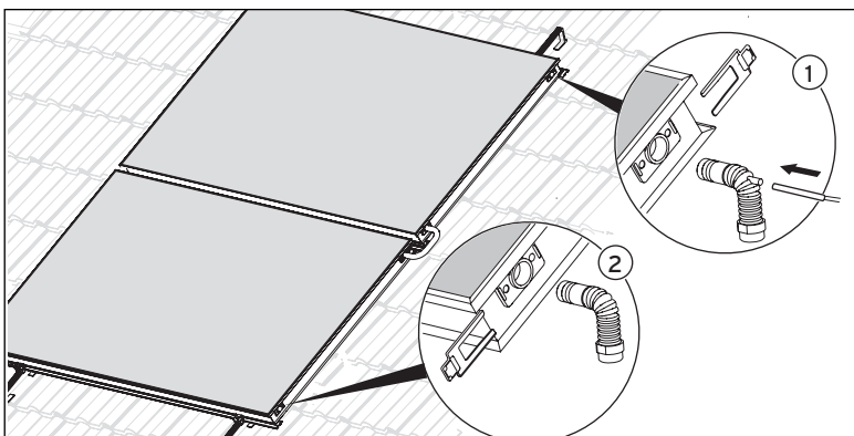
Abb. 6.19 Hydraulischer Anschluss bei Feldanordnung übereinander
