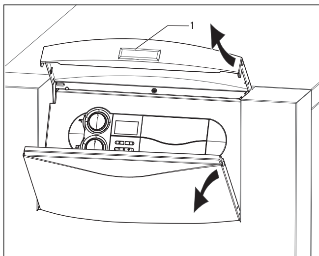
Abb. 5.1 Frontklappe öffnen
