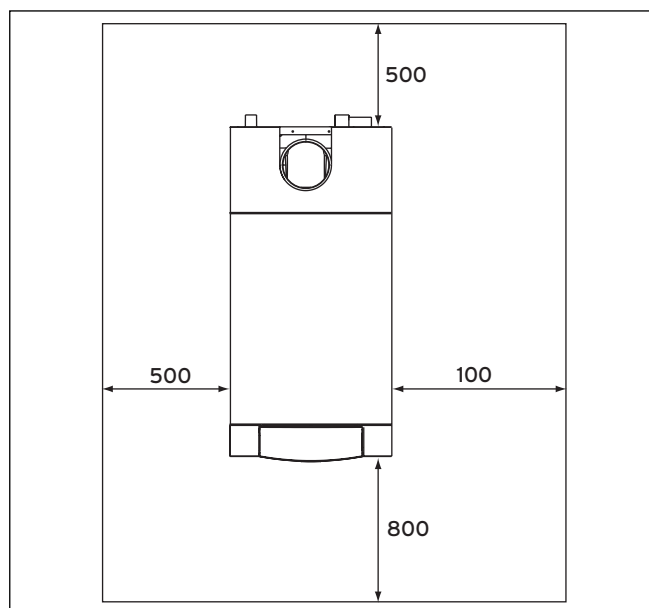
Abb. 4.2 Empfohlene Abstände bei der Aufstellung (in mm)
