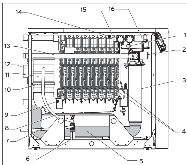
Abb. 2.4 Ansicht von links
