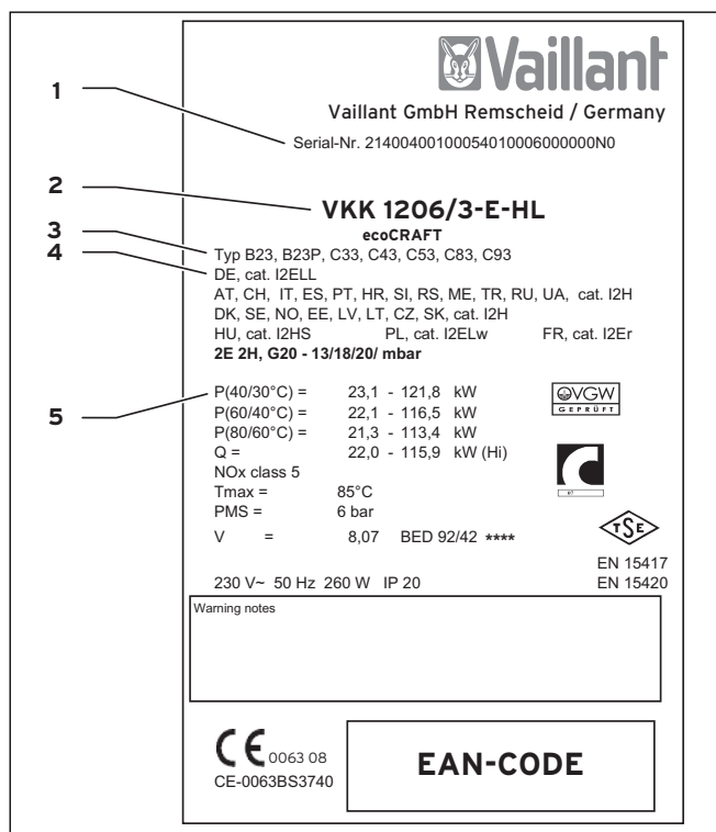
Abb. 2.1 Typenschild
