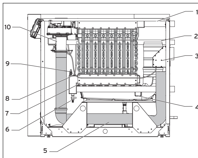
Abb. 2.3 Ansicht von rechts
