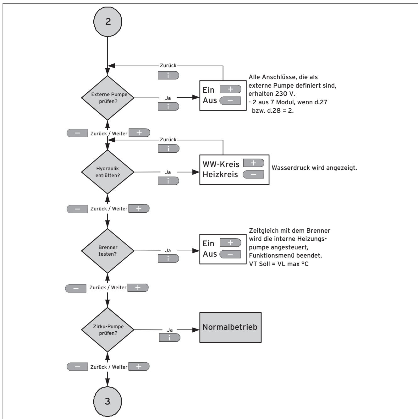
Abb. 6.1 Funktionsmenü (Fortsetzung)
