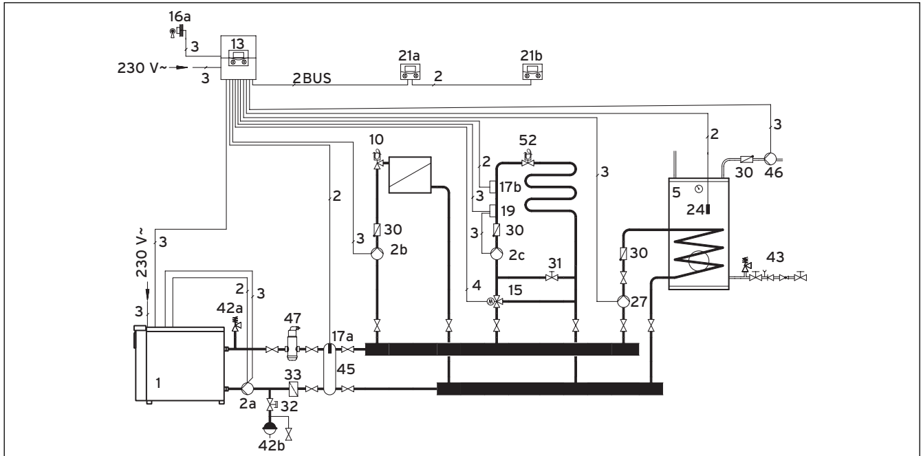
Abb. 5.5 Hydraulikschema mit hydraulischer Weiche
