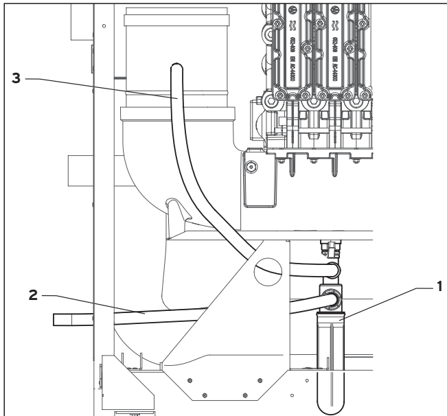
Abb. 5.6 Siphon
