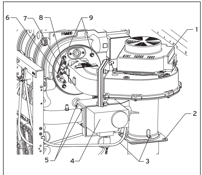
Abb. 8.6 Brenner ausbauen
