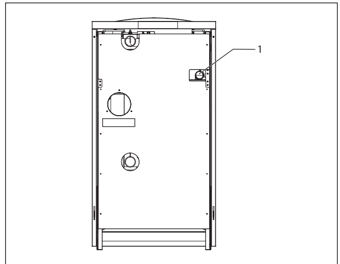
Abb. 5.3 Gasanschluss (Rückseite des Gas-Brennwertkessels)
