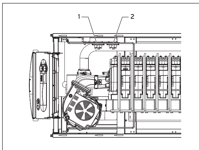
Abb. 8.4 Abgasdruckwächter überprüfen
