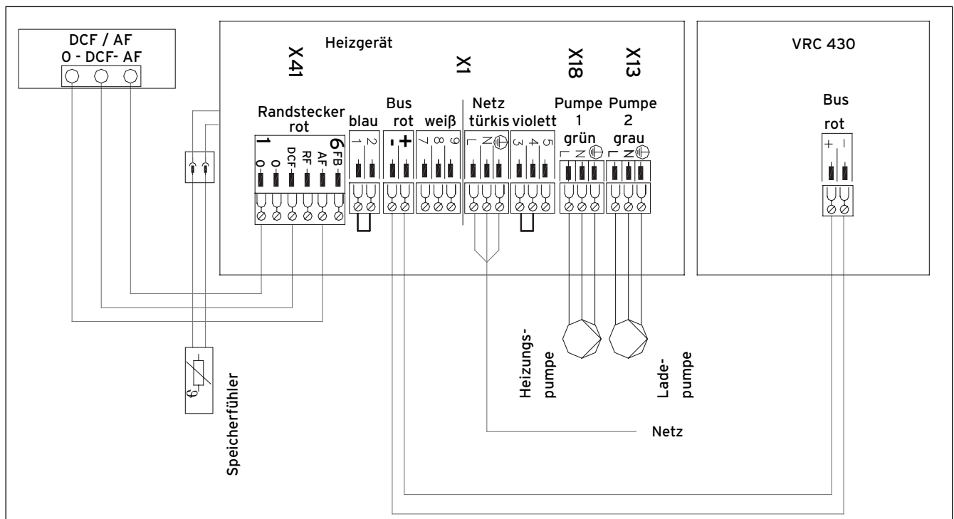
Abb. 5.9 Anschluss Regelgerät VRC 430
