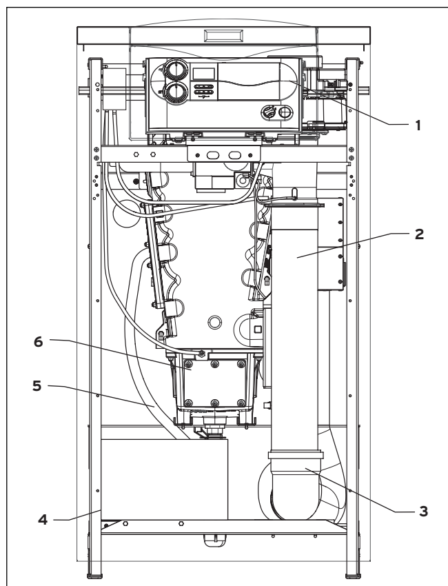
Abb. 2.6 Vorderansicht
