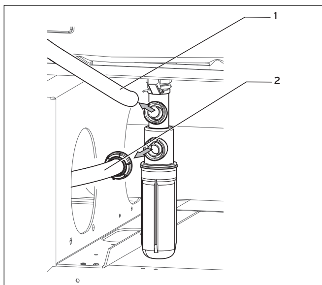
Abb. 8.2 Schläuche entfernen
