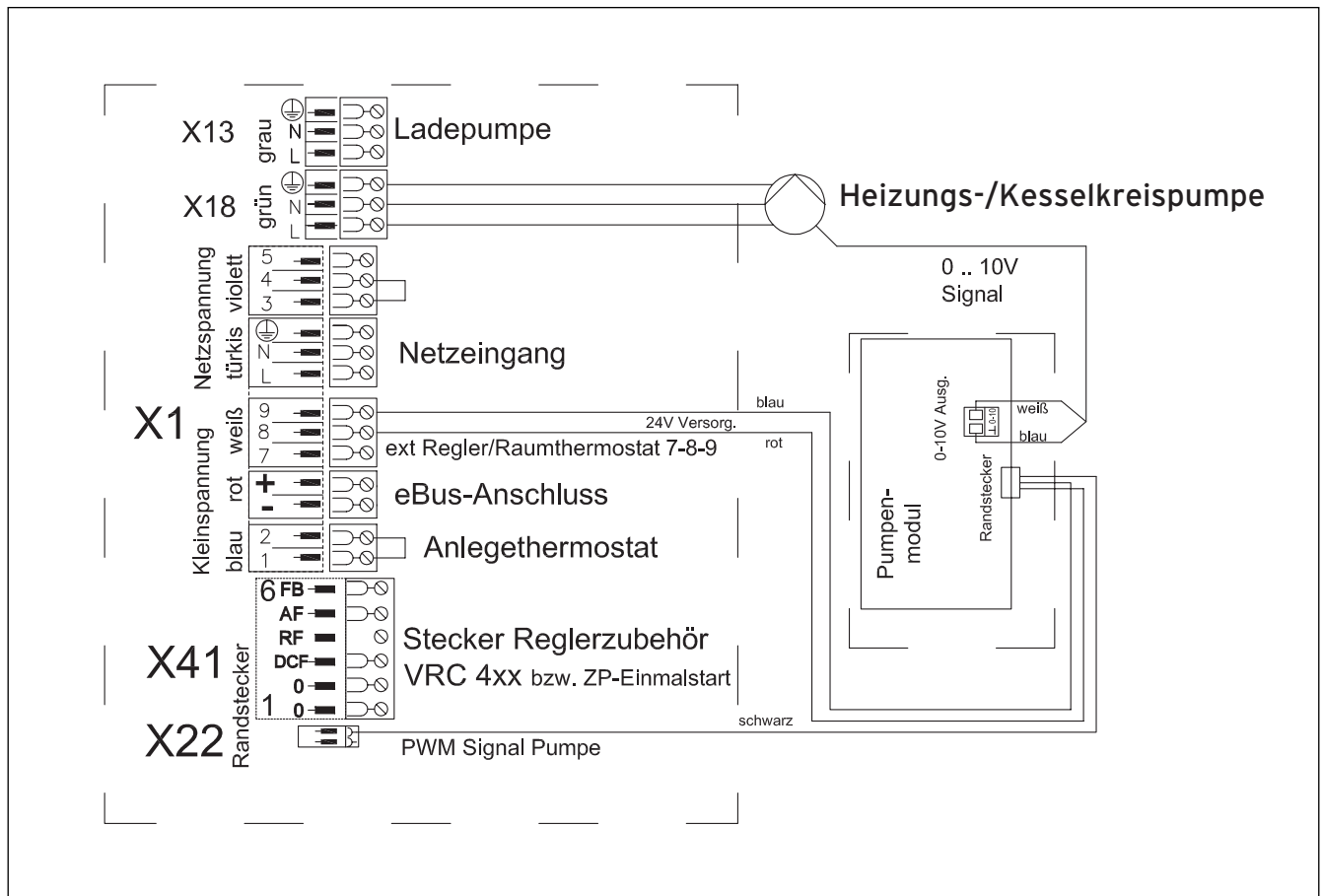
Abb. 5.8 Elektrischer Anschlussplan VKK 806/3-E-HL bis VKK 2806/3-E-HL
