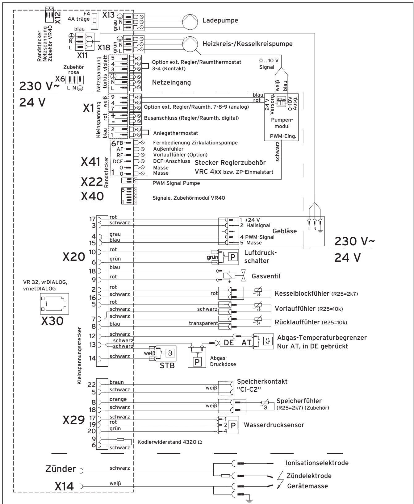
Abb. 5.7 Anschluss elektrischer Zubehöre und interne Verdrahtung
