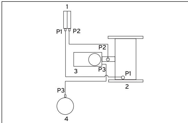
Abb. 8.5 Anschluss des Verbrennungsluftdruckwächters
