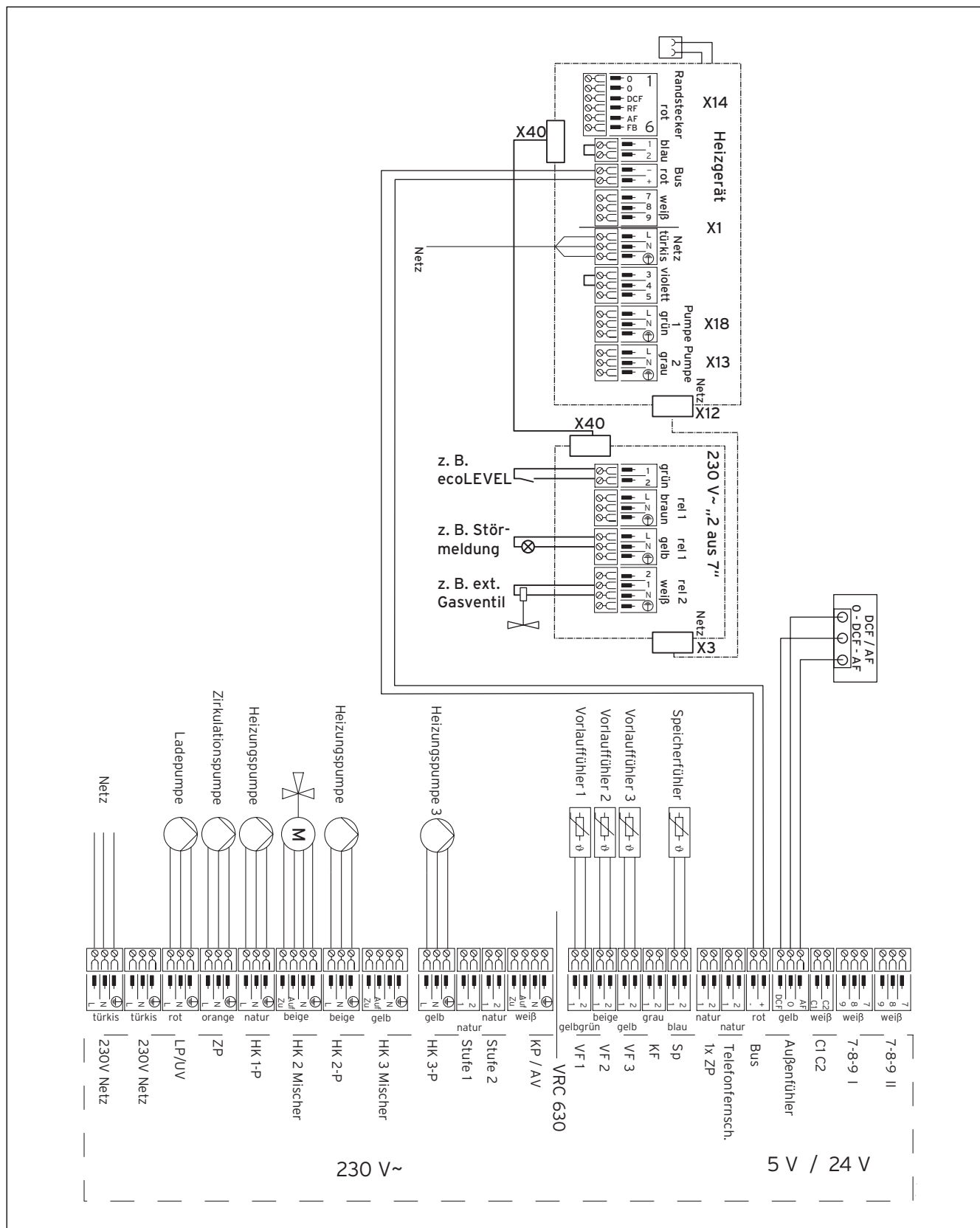
Abb. 5.10 Anschluss Regelgerät VRS 620, VRC 630
