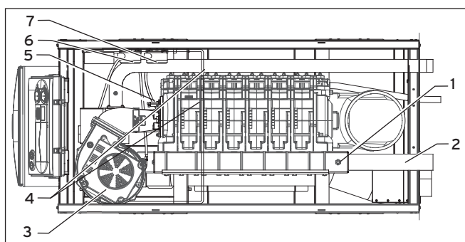
Abb. 2.5 Draufsicht
