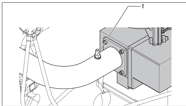
Abb. 6.2 Gasfließdruck prüfen
