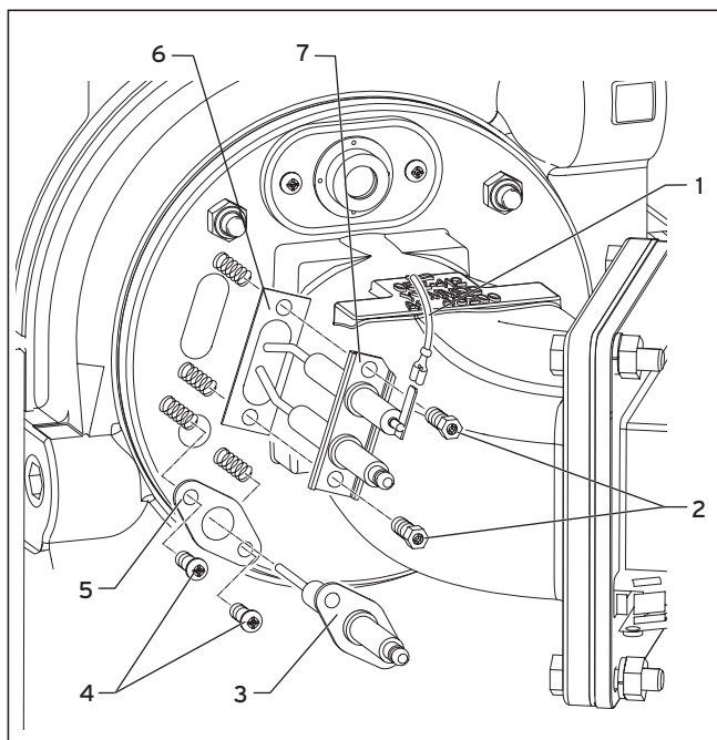
Abb. 8.9 Ausbau der Zünd- und Ionisations-/Überwachungselektrode
