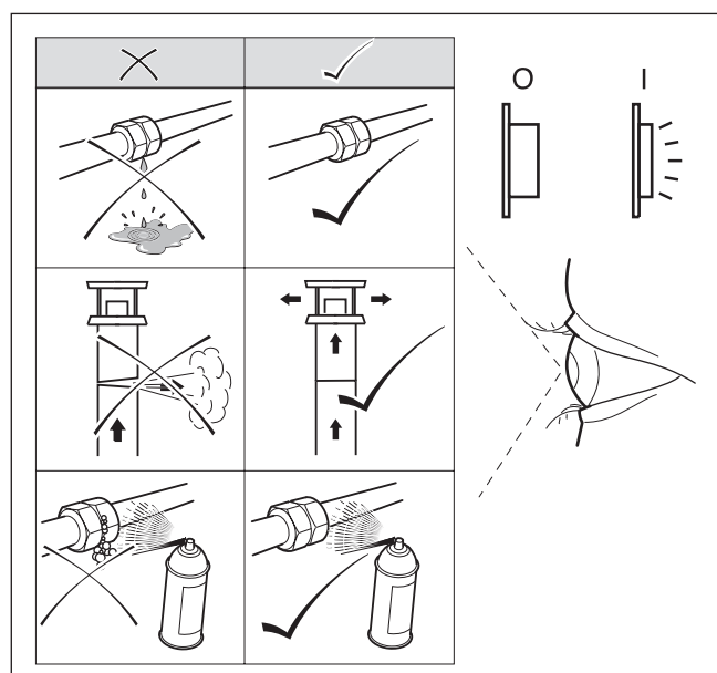
Abb. 6.5 Sicht- und Dichtepfung des Gerätes und der Anlage
