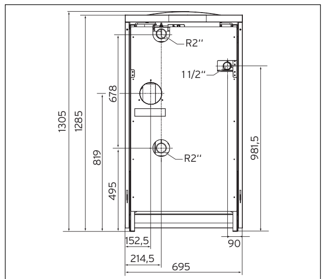
Abb. 4.3 Rohranschlussmaße (in mm)
