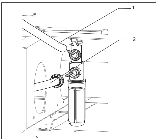
Abb. 8.2 Schläuche entfernen
