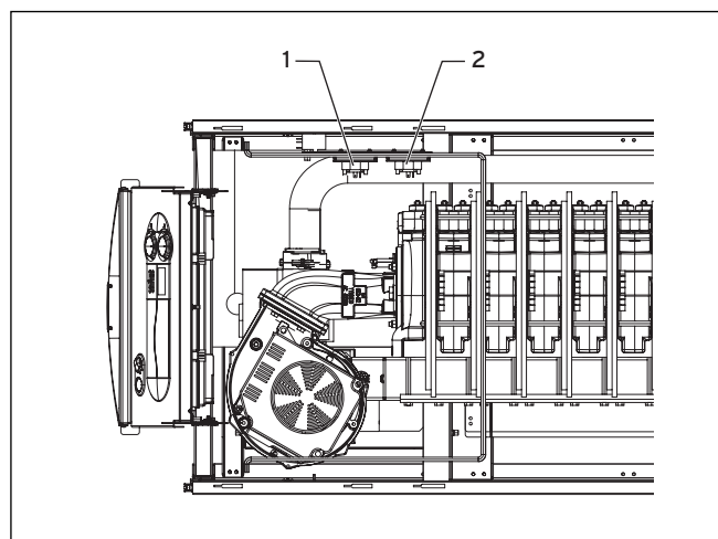
Abb. 8.4 Abgasdruckwächter überprüfen
