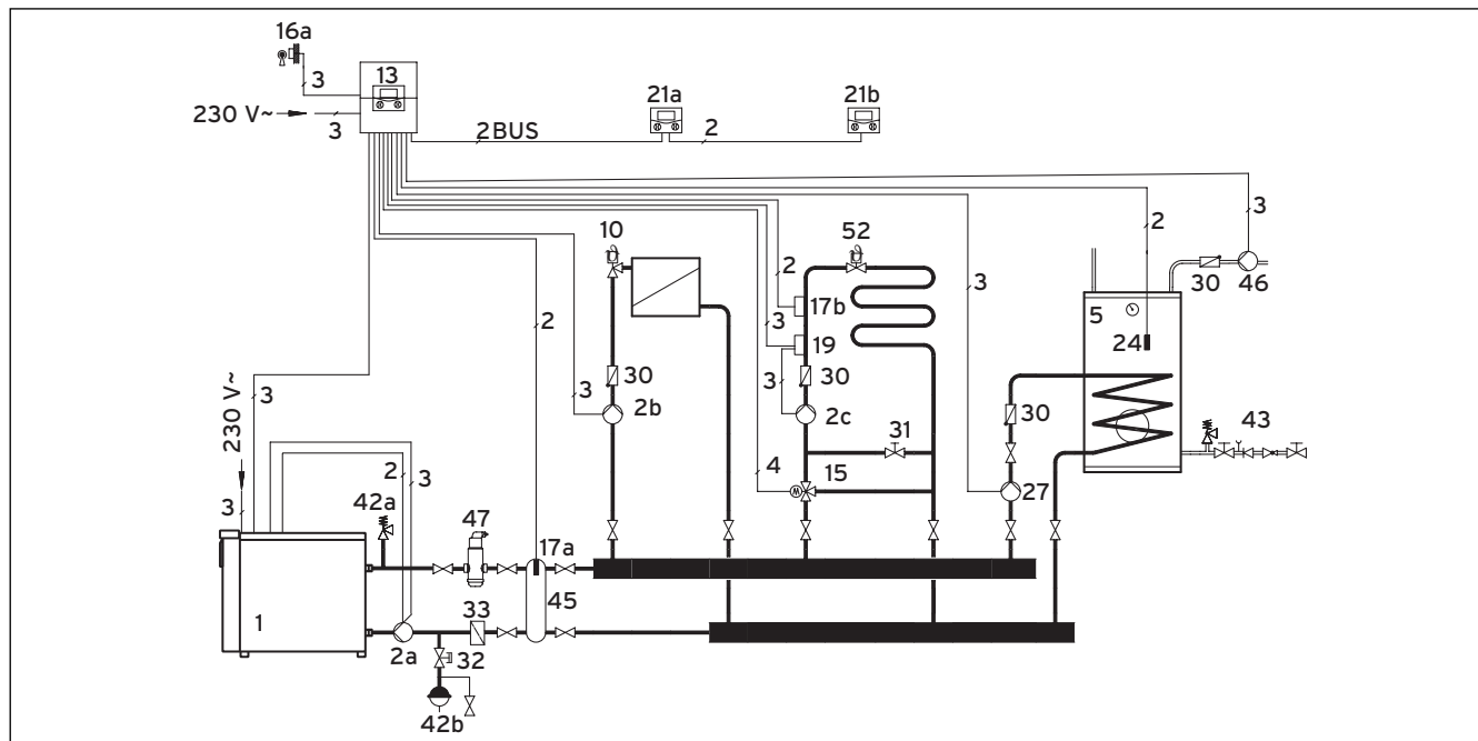
Abb. 5.5 Hydraulikschema mit hydraulischer Weiche
