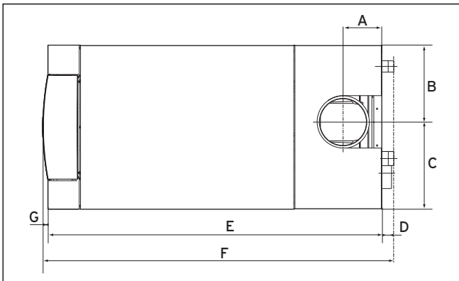
Abb. 4.4 Gerätemaße
