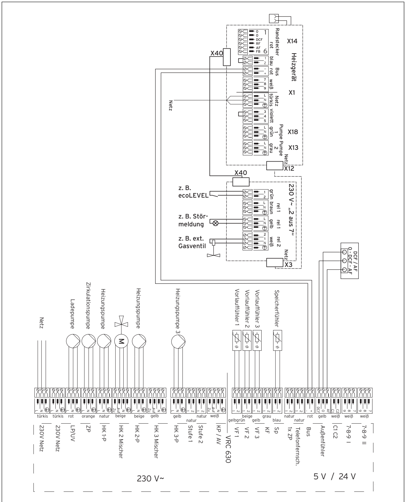
Abb. 5.10 Anschluss Regelgerät VRS 620, VRC 630
