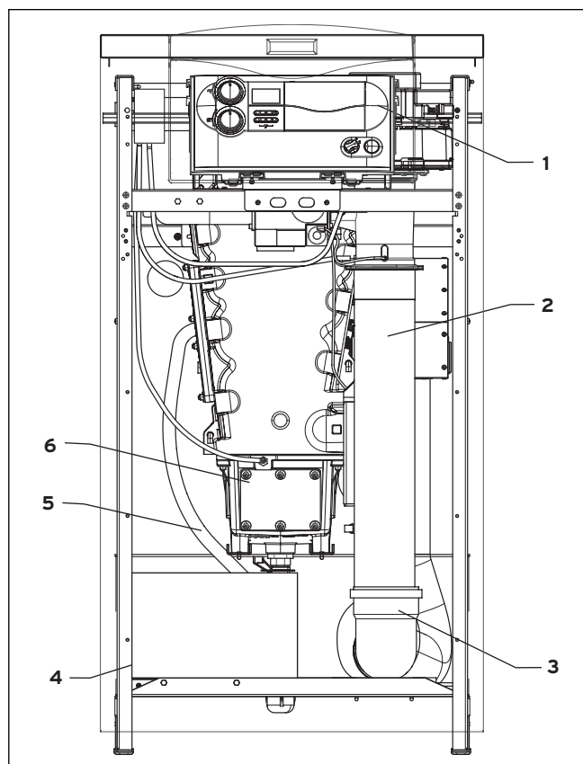
Abb. 2.6 Vorderansicht
