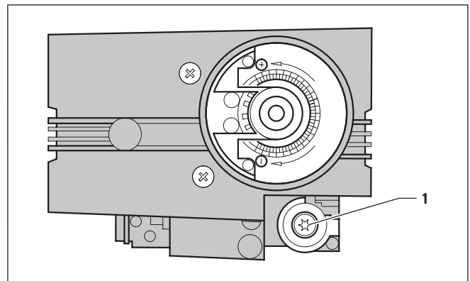
Abb. 6.4 Nullpunktschraube
