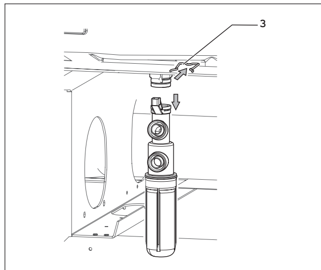
Abb. 8.3 Bügel abziehen
