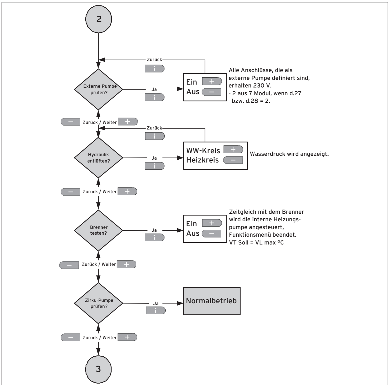
Abb. 6.1 Funktionsmenü (Fortsetzung)
