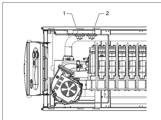
Abb. 8.4 Abgasdruckwächter überprüfen
