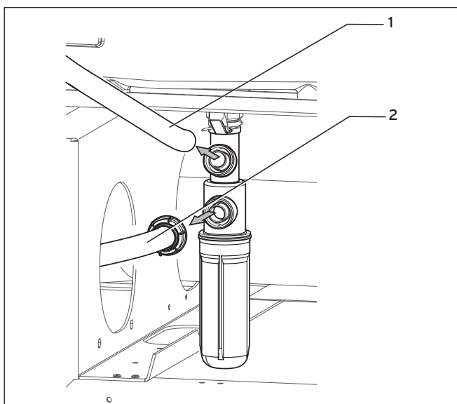
Abb. 8.2 Schläuche entfernen
