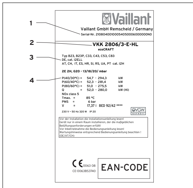
Abb. 2.1 Typenschild
