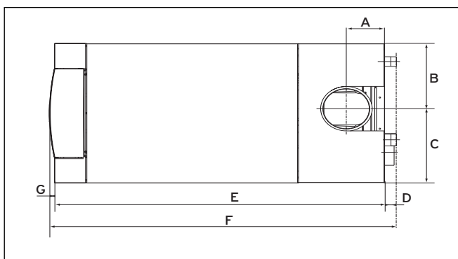
Abb. 4.4 Gerätemaße
