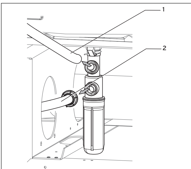
Abb. 8.2 Schläuche entfernen
