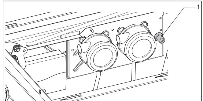
Abb. 8.9 Entriegelungstaste
