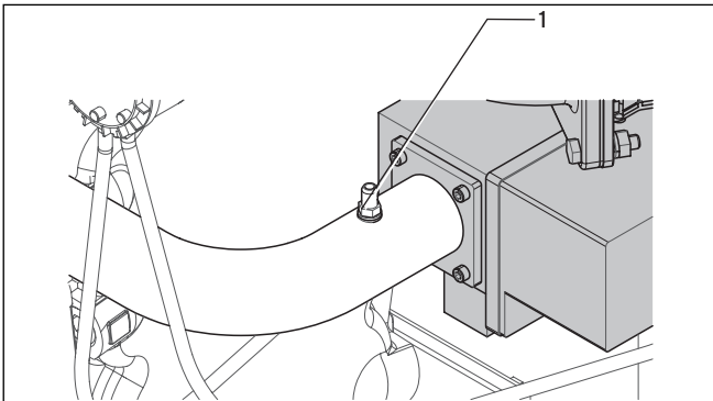
Abb. 6.2 Gasfließdruck prüfen
