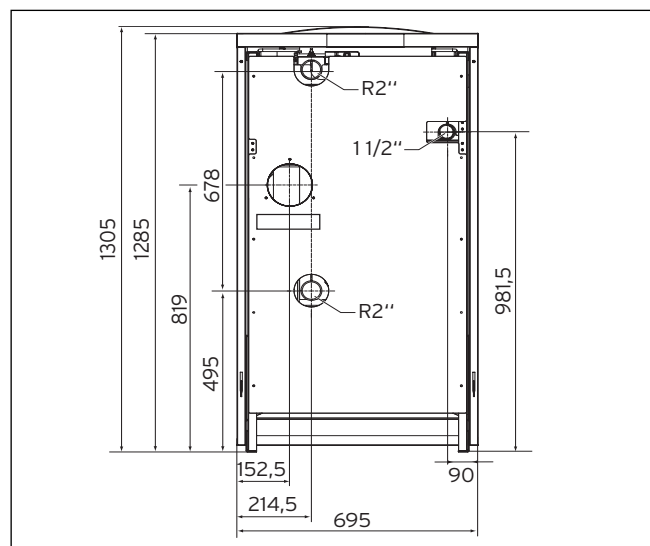
Abb. 4.3 Rohranschlussmaße
