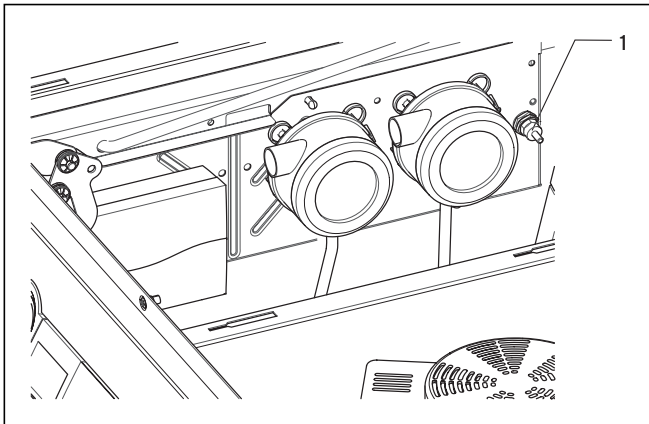
Abb. 9.1 Entriegelung nach STB Abschaltung
