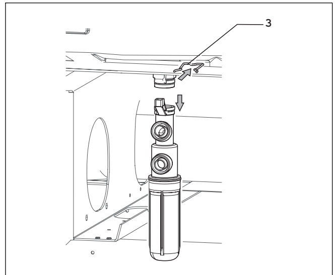
Abb. 8.3 Bügel abziehen
