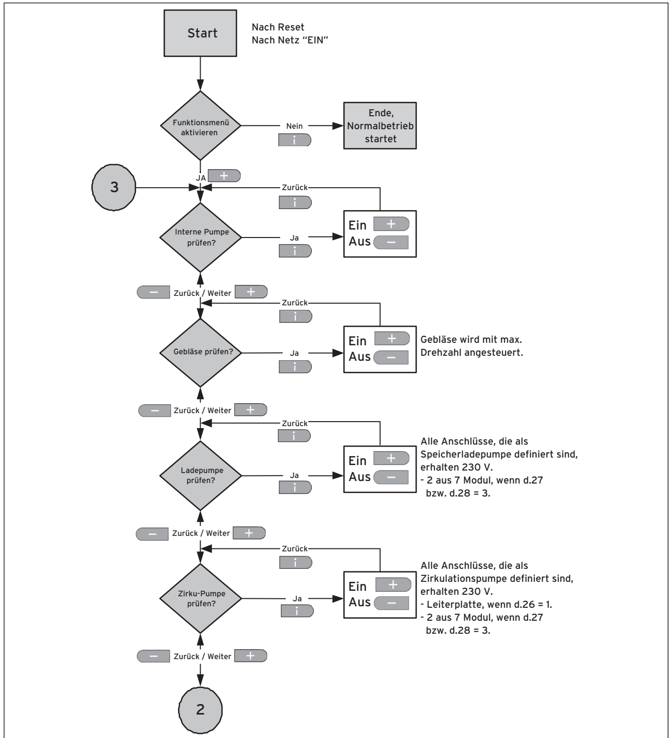
Abb. 6.1 Funktionsmenü (Forts. nächste Seite)
