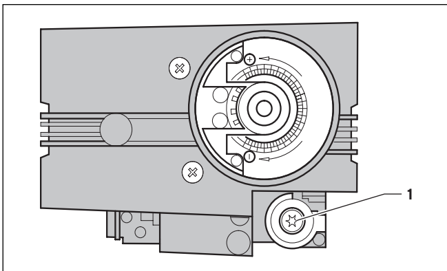
Abb. 6.4 Nullpunktschraube
