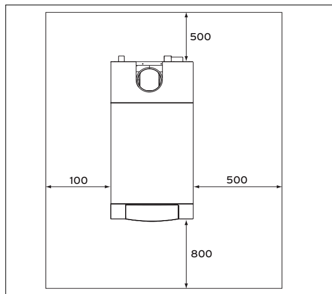
Abb. 4.2 Empfohlene Abstände bei der Aufstellung
