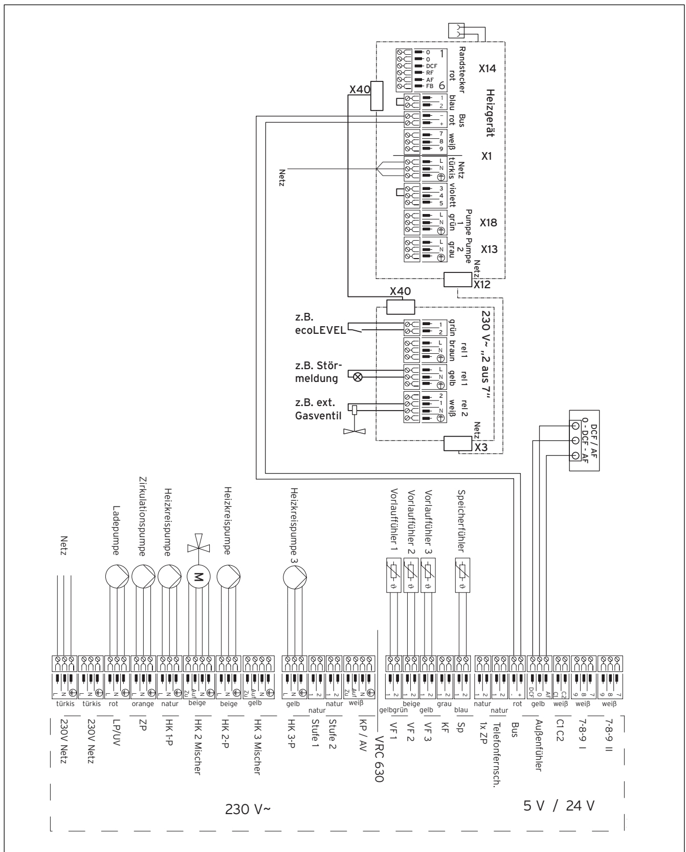
Abb. 5.9 Anschluss Regelgerät VRC 630
