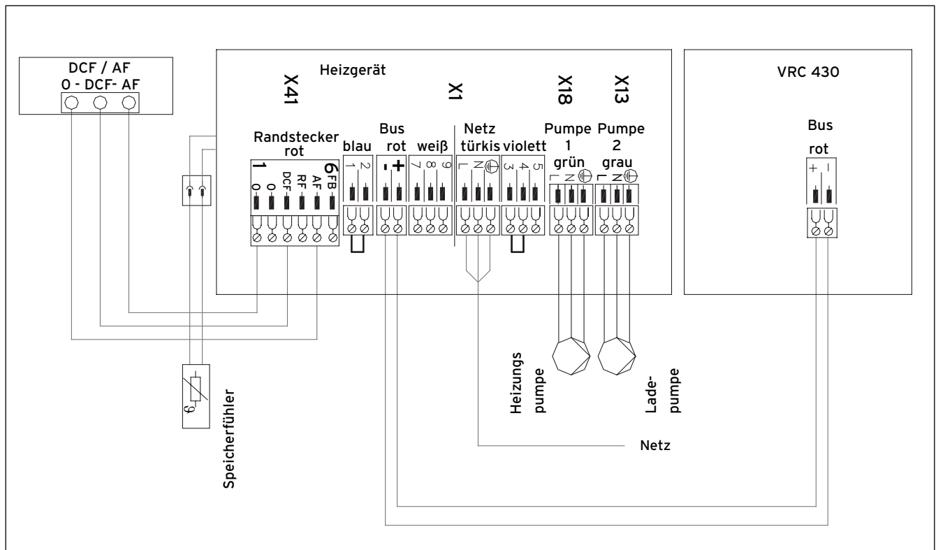
Abb. 5.8 Anschluss Regelgerät VRC 430
