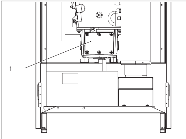
Abb. 8.1 Kondenswassersammler reinigen
