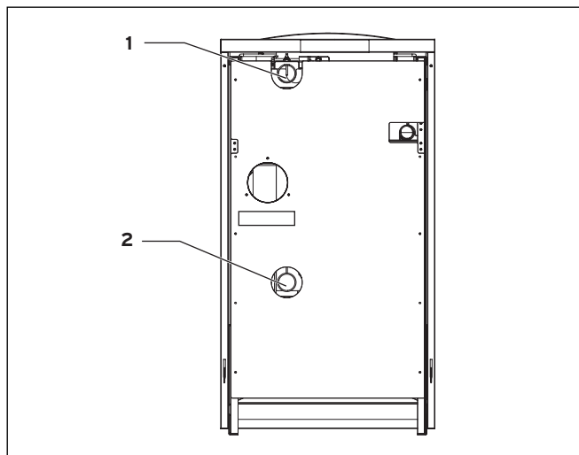
Abb. 5.4 Heizungsseitiger Anschluss (Rückseite des Kessels)
