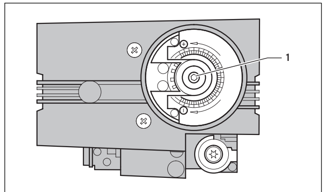
Abb. 6.3 Gasdurchflussschraube
