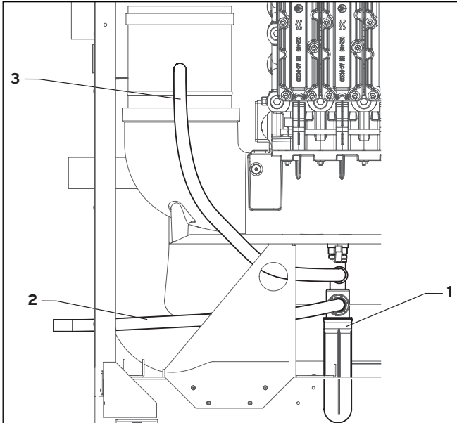
Abb. 5.6 Siphon
