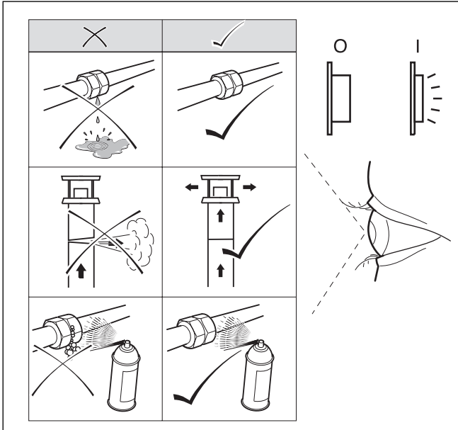
Abb. 6.5 Sichtprüfung des Gerätes und der Anlage
