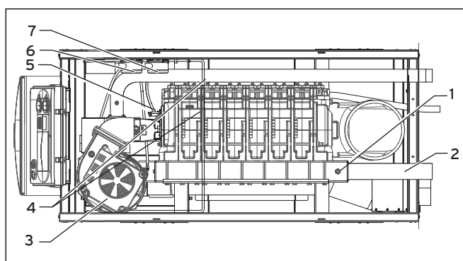
Abb. 2.5 Draufsicht
