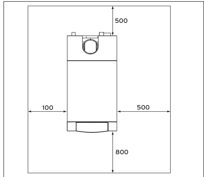
Abb. 4.2 Empfohlene Abstände bei der Aufstellung
