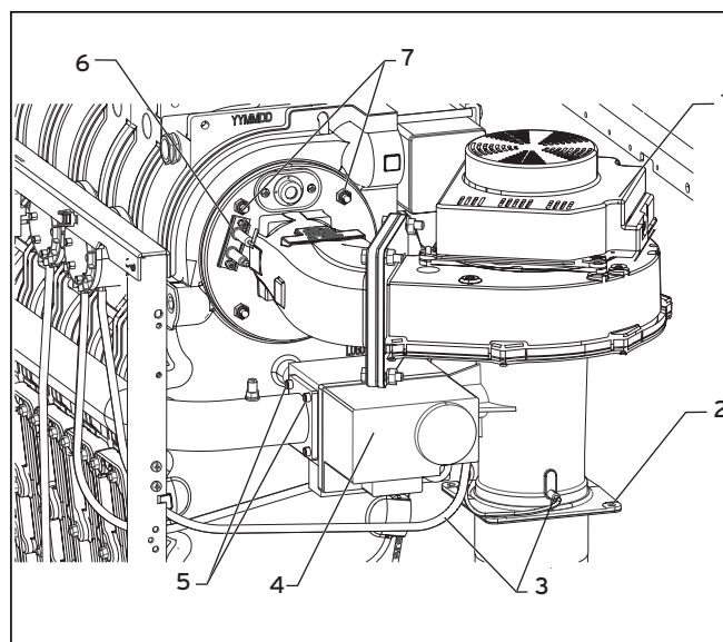
Abb. 8.6 Brenner ausbauen
