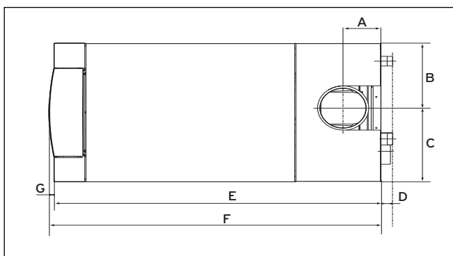
Abb. 4.4 Gerätemaße
