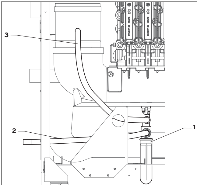
Abb. 5.6 Siphon
