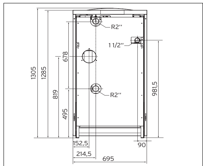
Abb. 4.3 Rohranschlussmaße
