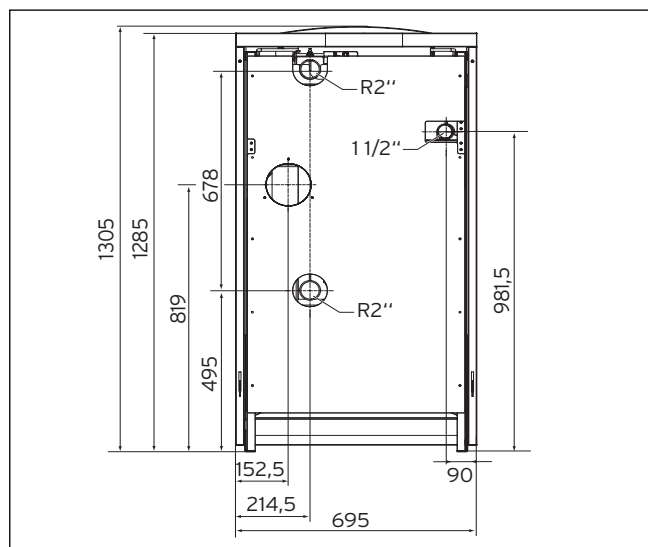
Abb. 4.3 Rohranschlussmaße
