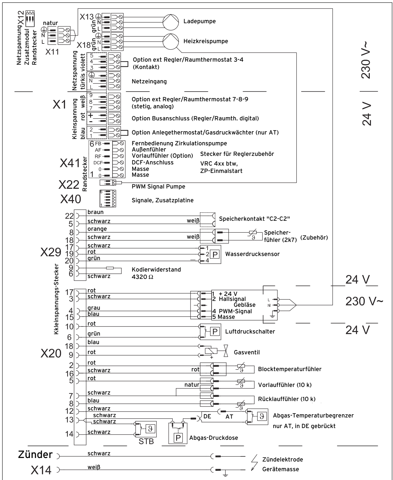
Abb. 5.4 Anschluss elektrischer Zubehöre und interne Verdrahtung
