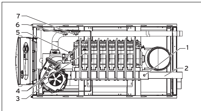
Abb. 2.4 Draufsicht
