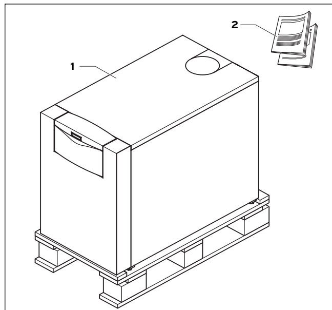
Abb. 4.1 Lieferumfang
