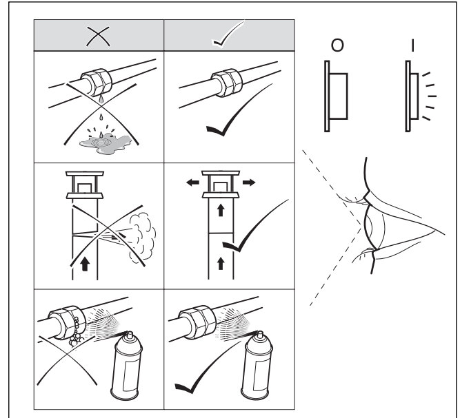
Abb. 6.4 Sichtprüfung des Gerätes und der Anlage
