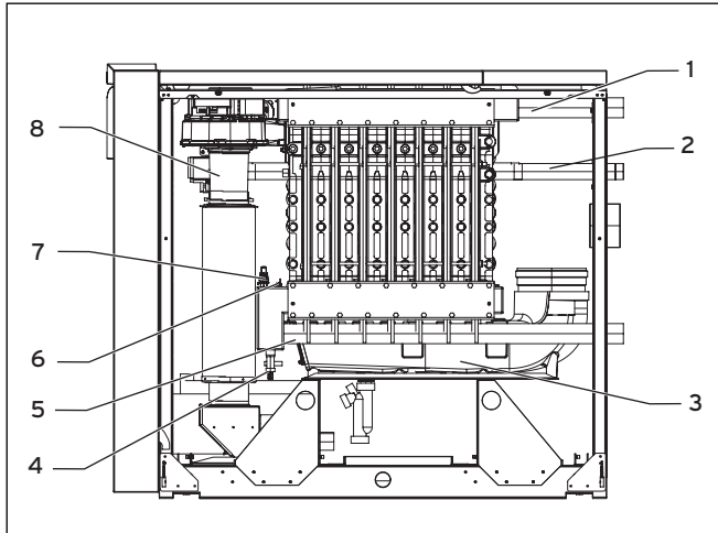
Abb. 2.2 Ansicht von rechts
