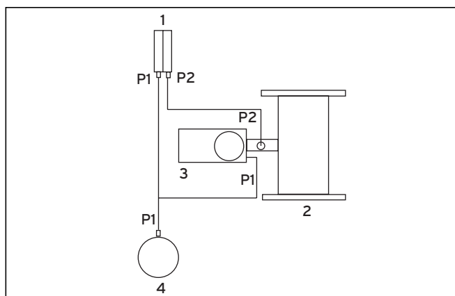
Abb. 8.4 Anschluss des Verbrennungsluftdruckwächters
