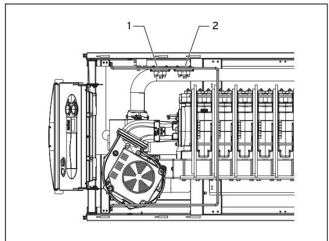
Abb. 8.3 Abgasdruckwächter überprüfen
