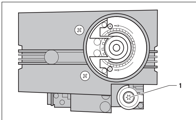
Abb. 6.3 Nullpunktschraube
