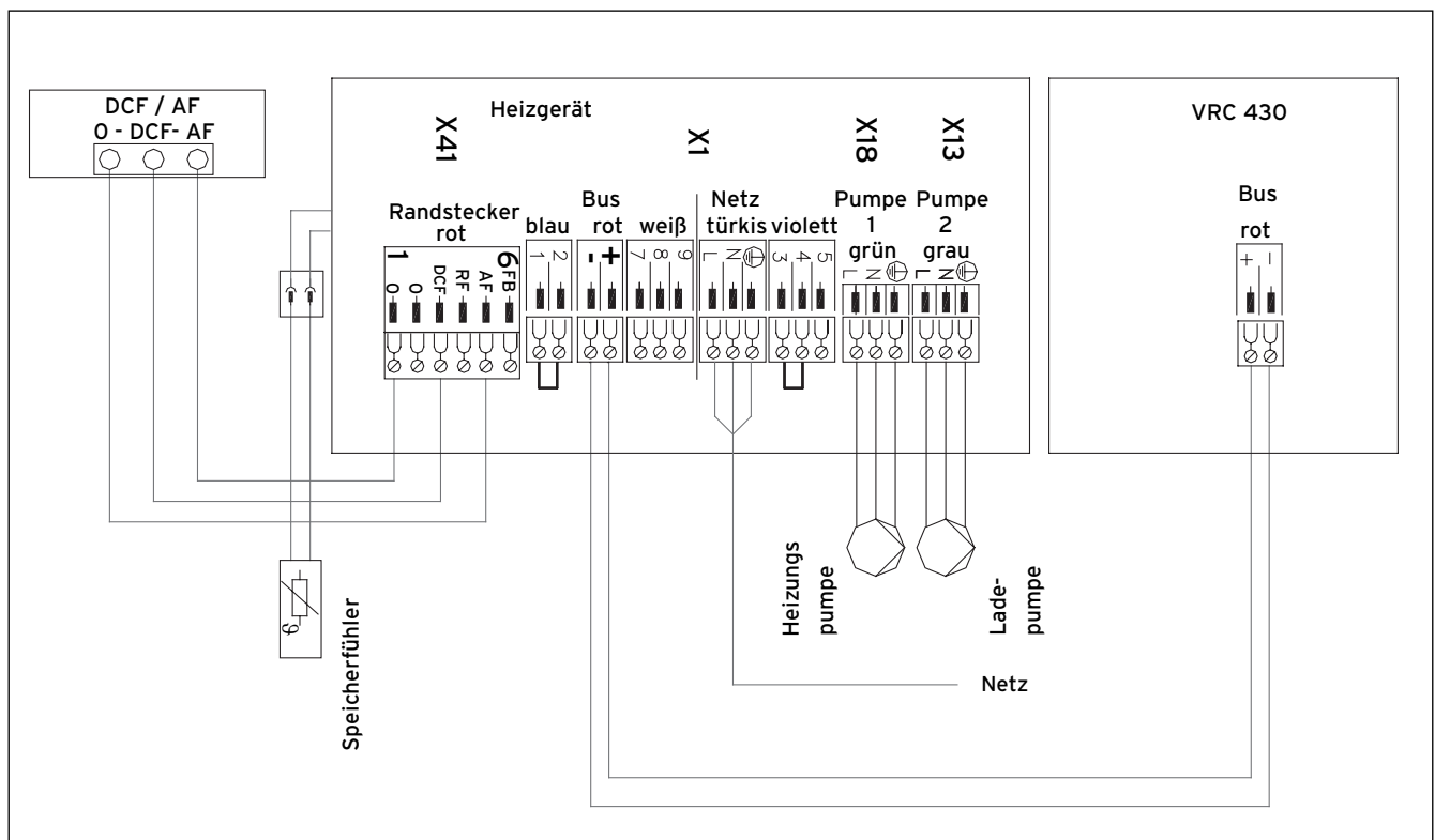
Abb. 5.5 Anschluss Regelgerät VRC 430
