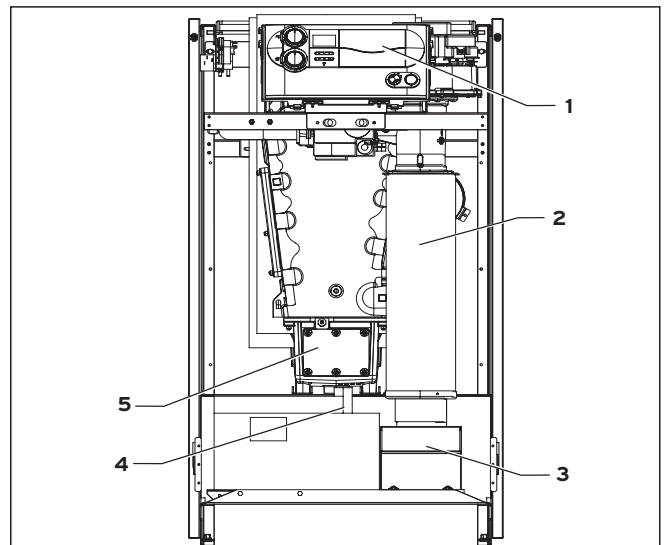
Abb. 2.5 Vorderansicht
