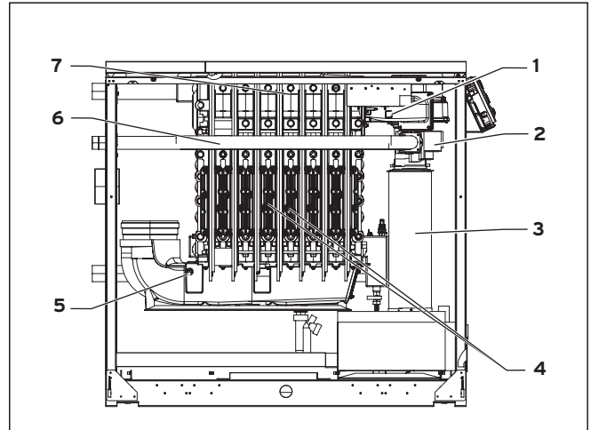
Abb. 2.3 Ansicht von links
