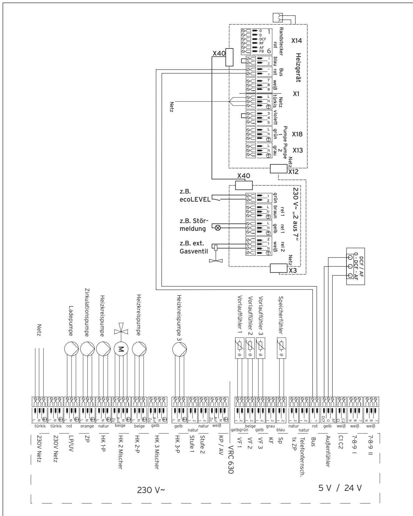
Abb. 5.6 Anschluss Regelgerät VRC 630
