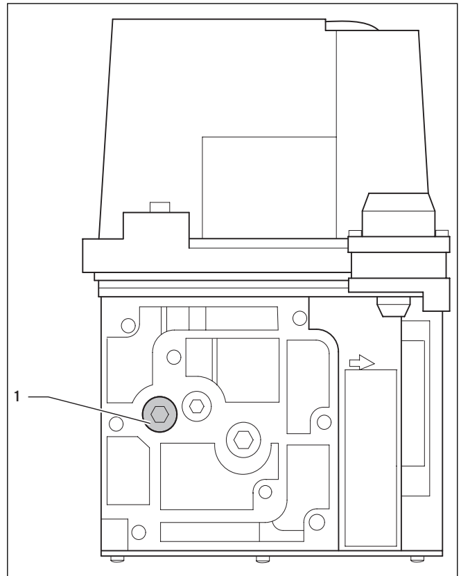
Abb. 6.1 Gasfließdruck prüfen
