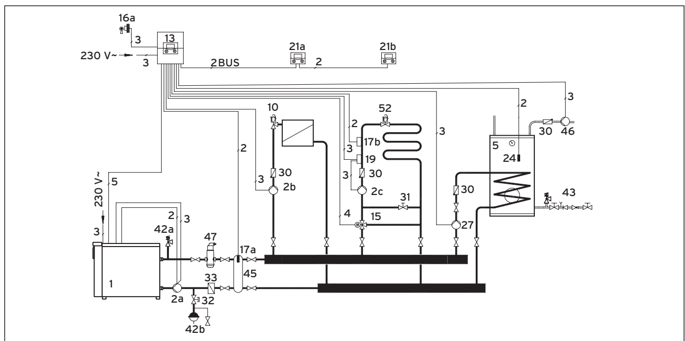
Abb. 5.3 Hydraulikschema mit hydraulischer Weiche
