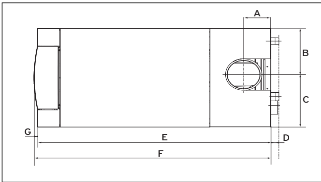
Abb. 4.4 Gerätemaße
