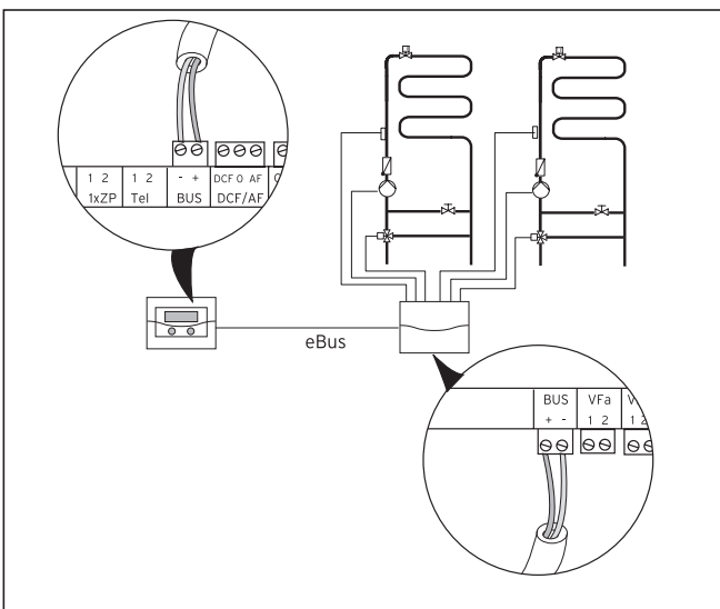
Abb. 5.16 Weitere Mischerkreise anschließen
