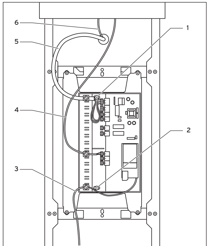
Abb. 5.18 vrnetDIALOG installieren
