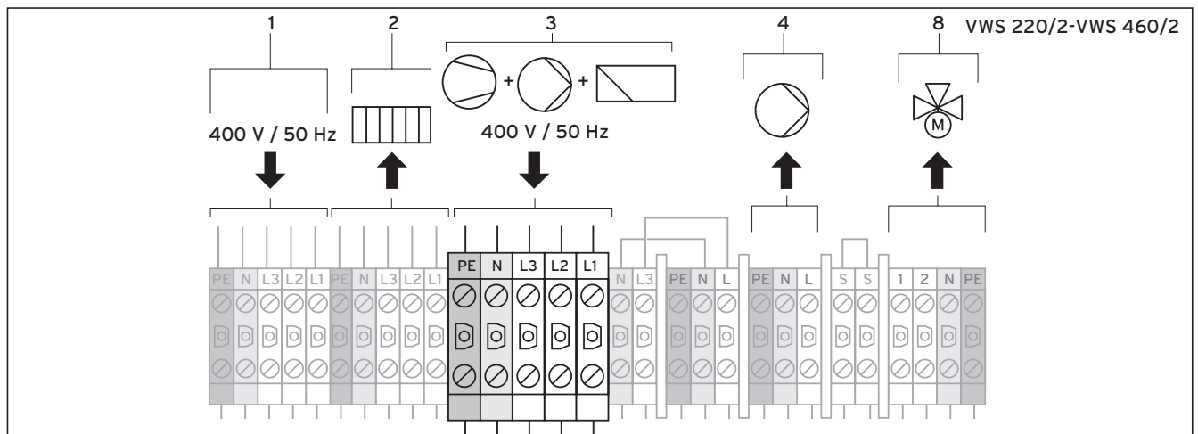
Abb. 5.2 Ungesperrte Netzeinspeisung (Lieferzustand) VWS
