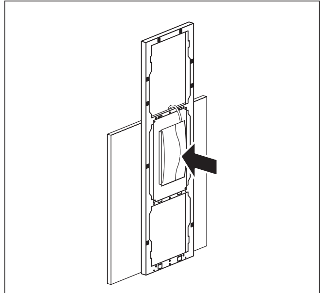
Abb. 5.17 vrnetDIALOG montieren
