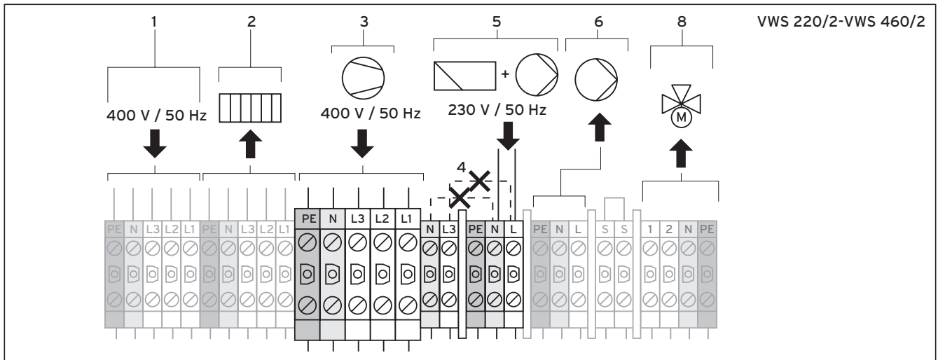
Abb. 5.4 Zweikreis-Einspeisung VWS
