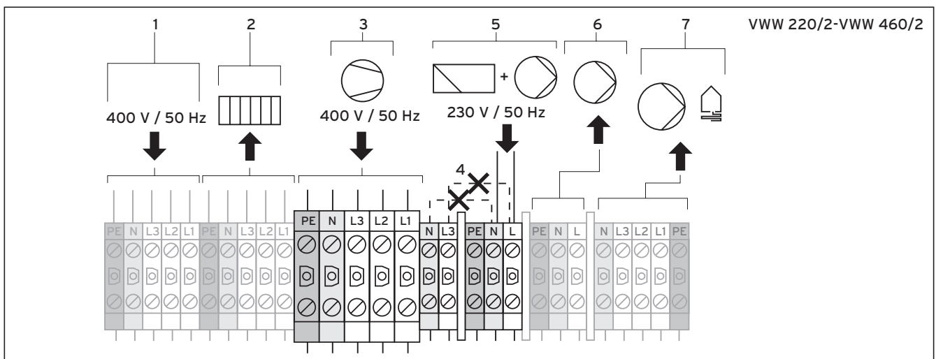
Abb. 5.5 Zweikreis-Einspeisung VWW
