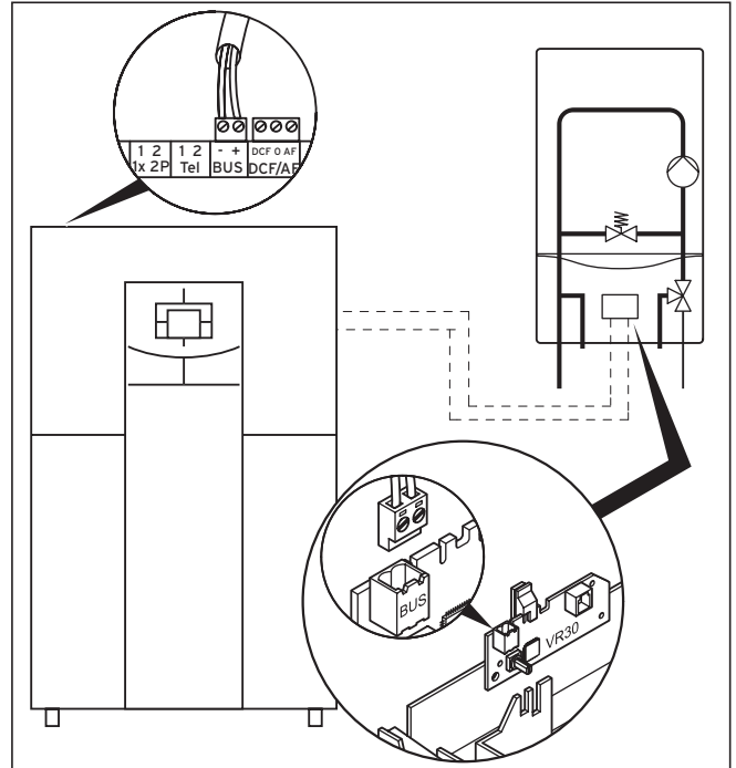
Abb. 5.19 Heizgerät mit eBUS-Schnittstelle anschließen
