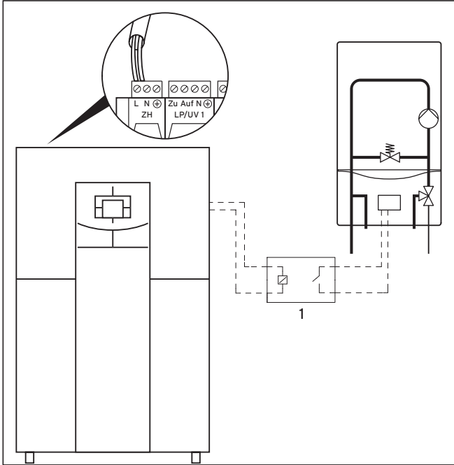
Abb. 5.20 Heizgerät ohne eBUS-Schnittstelle anschließen
