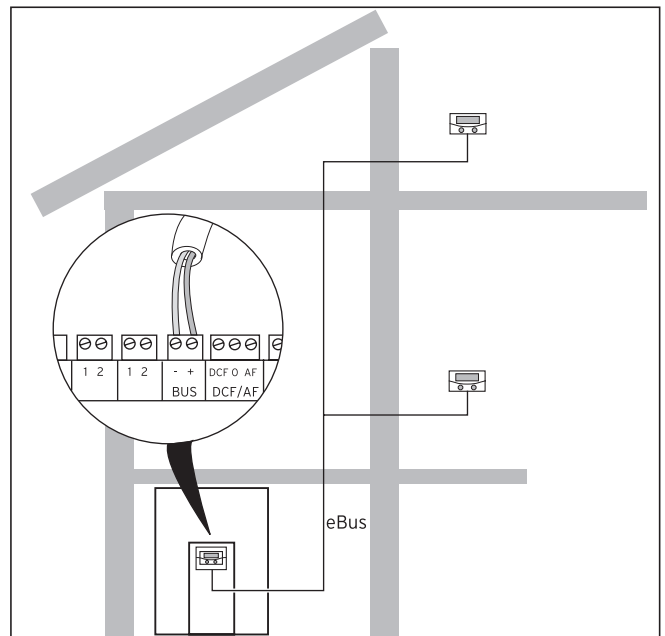
Abb. 5.14 Fernbediengeräte anschließen
