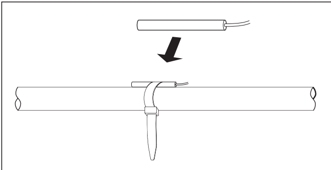
Abb. 5.7 Standardfühler VR 10
