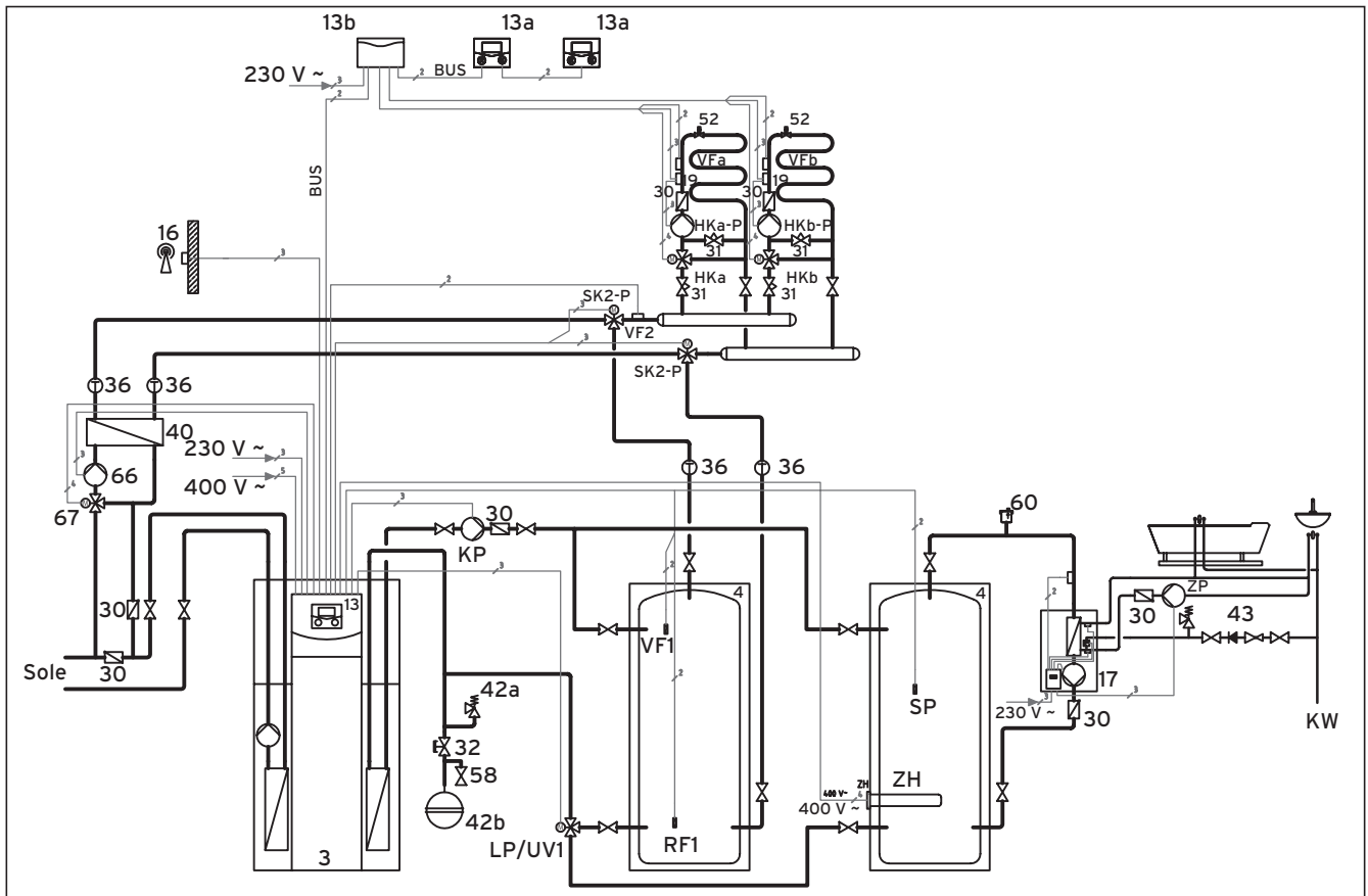
Abb. 5.12 Hydraulikplan 10
