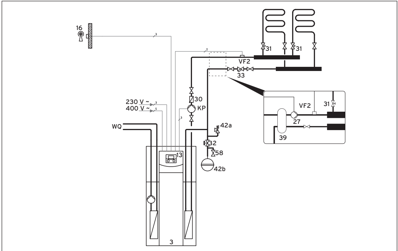
Abb. 5.8 Hydraulikplan 1
