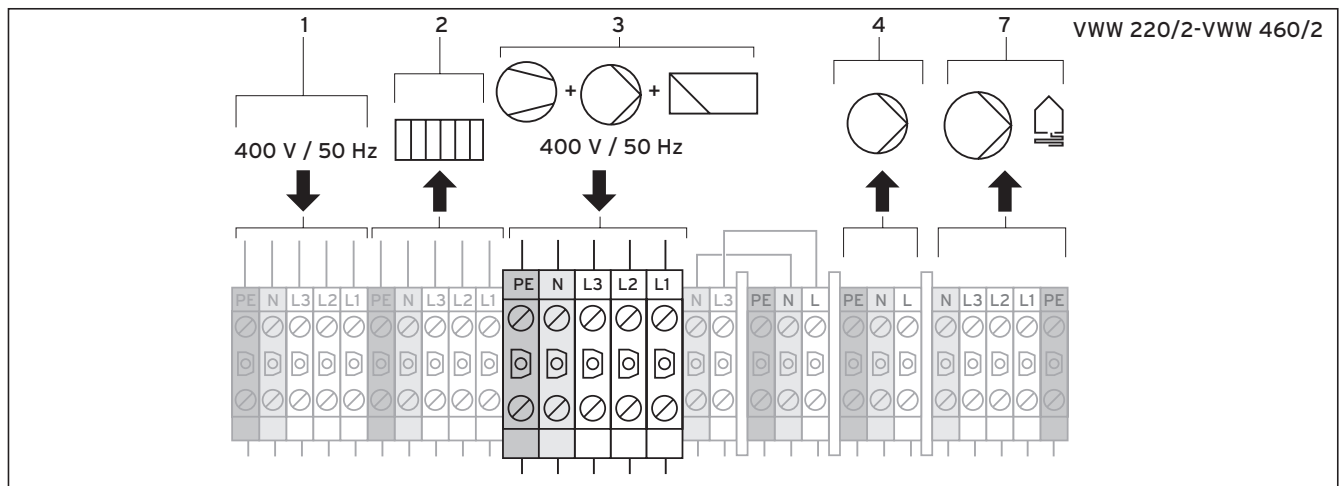
Abb. 5.3 Ungesperrte Netzeinspeisung (Lieferzustand) VWV
