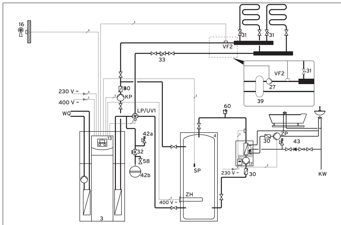
Abb. 5.10 Hydraulikplan 3
