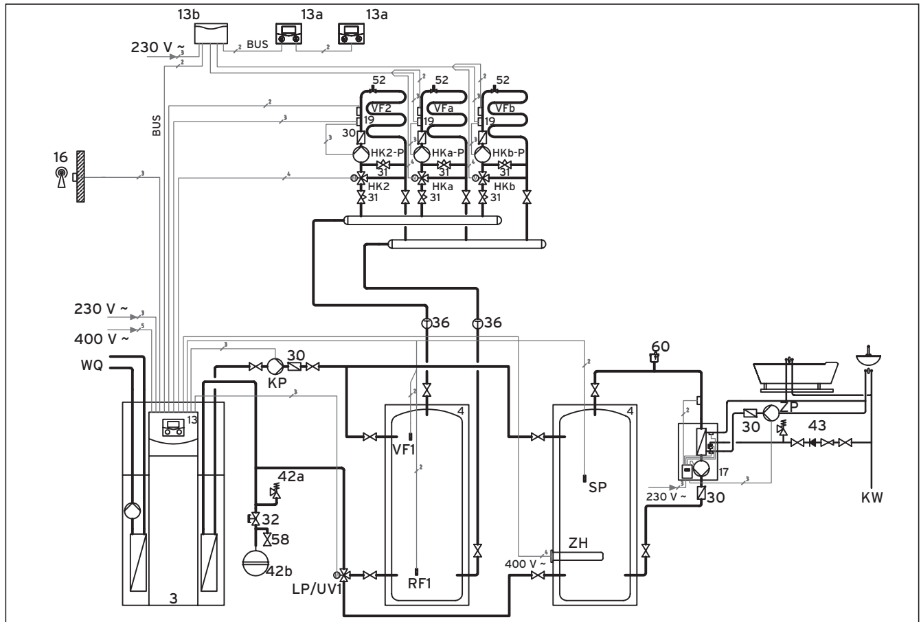
Abb. 5.11 Hydraulikplan 4
