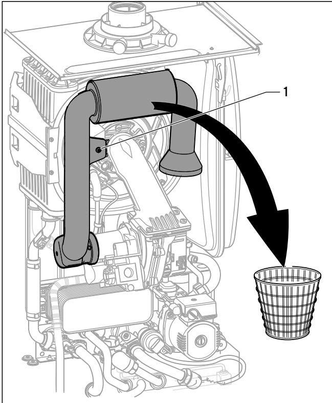
Abb. 2.1 Luftansaugrohr entfernen
