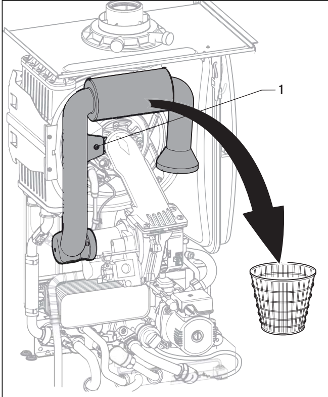
Abb. 2.1 Luftansaugrohr entfernen
