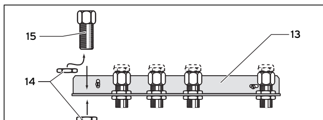
Sl. 4.6 Konzola kod ocjevljenja odozgo
