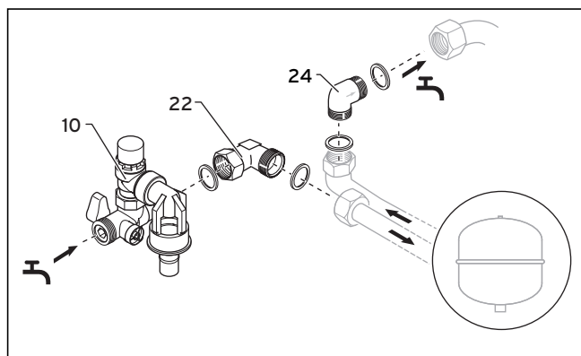
Sl. 4.12 Priključak ekspanzijske posude za toplu vodu
