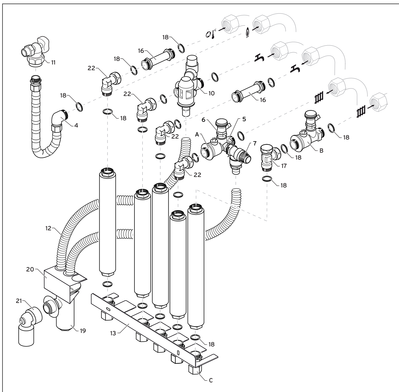
SI. 4.14: Pregled priključaka uređaja (ovdje: ocjevljenje odozdo)
