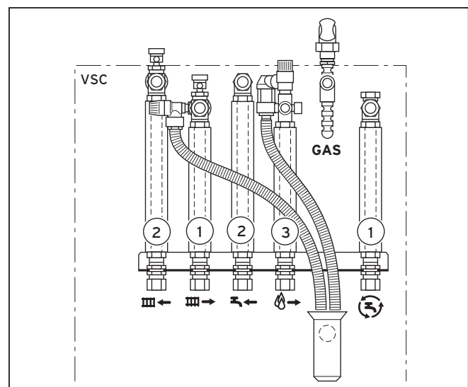
Abb. 4.8 Verrohrung von unten
