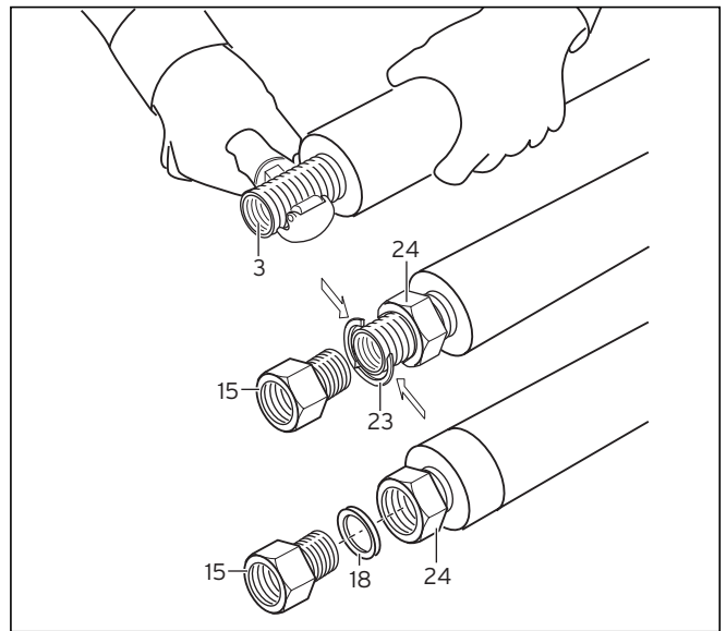
Abb. 4.10 Edelstahl-Wellrohr einkürzen
