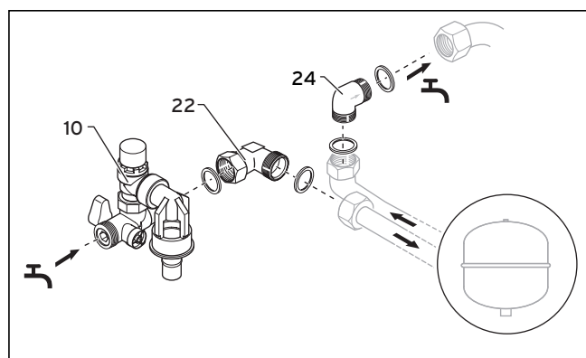
Sl. 4.12 Priključitev raztezne posode za toplo vodo
