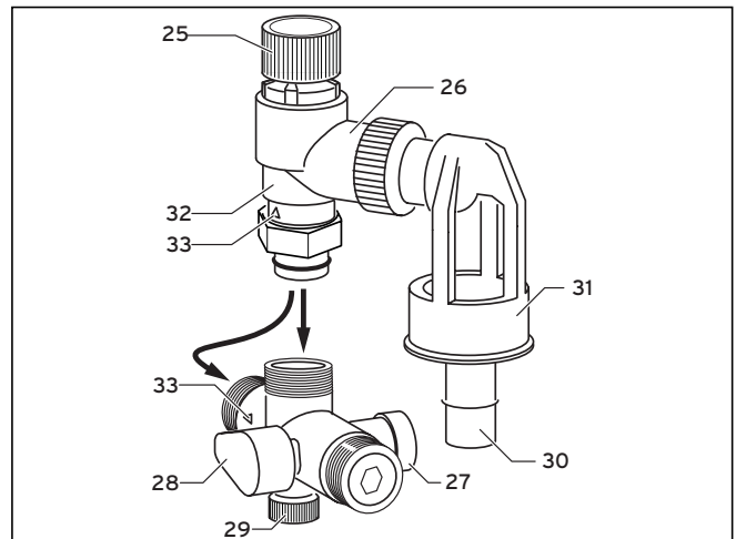
Abb. 4.13 Sicherheitsgruppe
