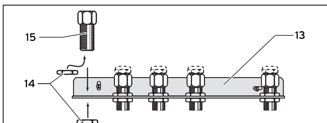
Abb. 4.6 Konsole bei Verrohrung von oben
