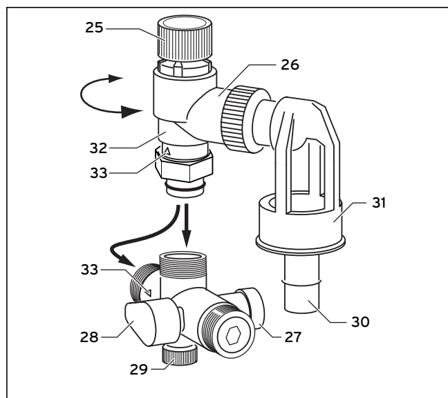
Abb. 4.11 Sicherheitsgruppe
