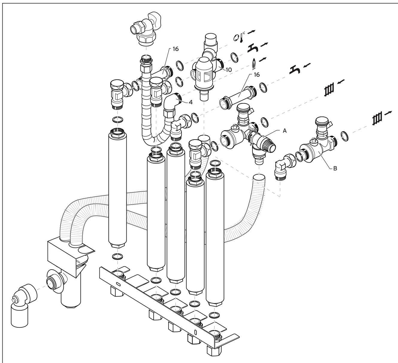
Abb. 4.7: Übersicht Geräteanschlüsse
