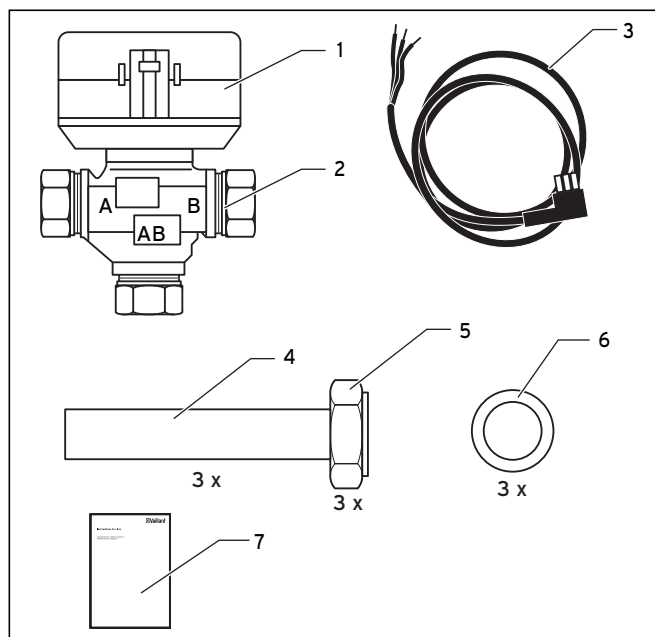
Fig. 3.1 Contenu de la livraison soupape à 3 voies externe
