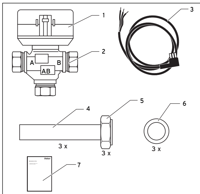
3.1. ábra: Külső 3-utas szelep szállítási terjedelem
