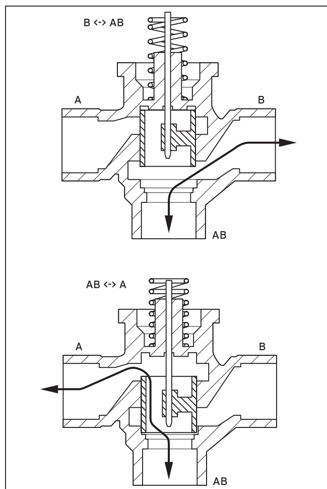
Rys. 4.1 Montaż w funkcji rozdzielacza w dopływie grzewczym wytwornicy ciepła
