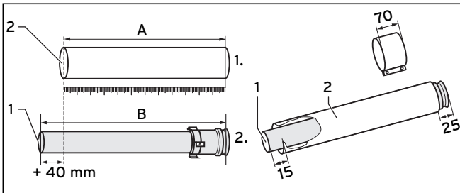
Abb. 6.79 Rohre kürzen
