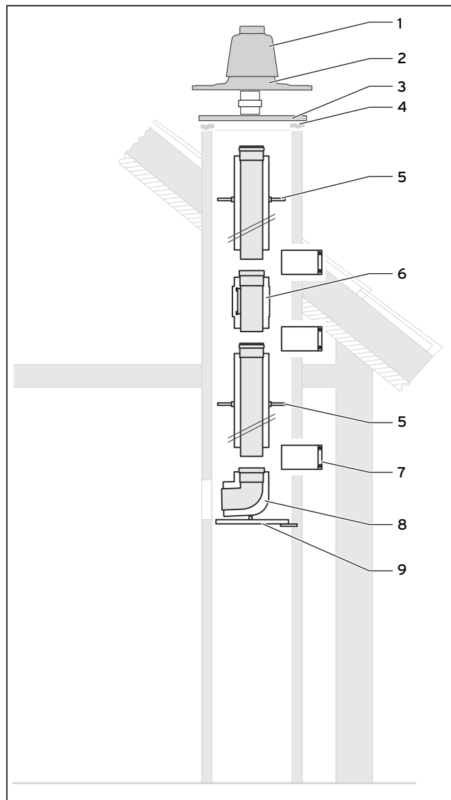
Abb. 6.72 Montagebeispiel raumluftunabhängig
