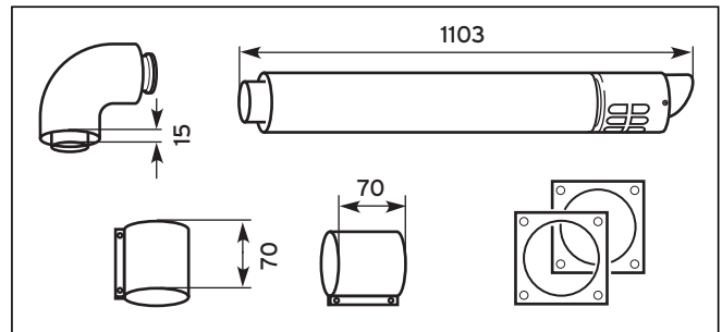
Abb. 6.5 Lieferumfang Art.-Nr. 303 209
