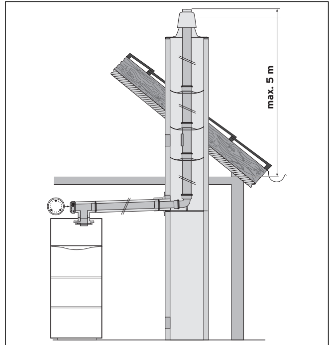
Abb. 6.18 Montagebeispiel raumluftunabhängig
