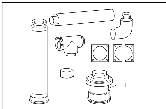
Abb. 6.67 Lieferumfang Art.-Nr. 303 230
