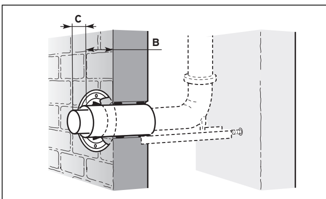
Abb. 3.3 Raumluftunabhängiger Betrieb
