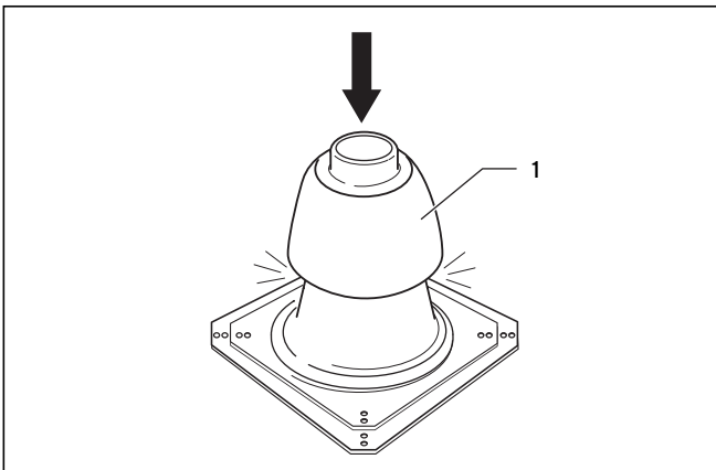
Abb. 6.43 Die Haube muss hörbar einrasten
