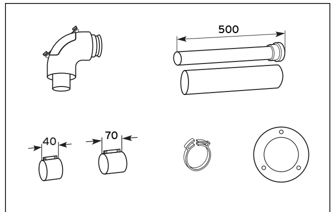
Abb. 5.18 Lieferumfang (Art.-Nr. 303 923)
