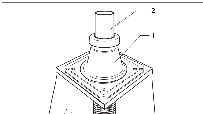
Abb. 6.63 Schachtabdeckung montieren
