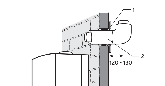
Abb. 6.68 Außenwanddurchführung montieren
