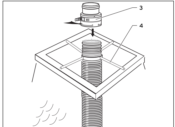
Abb. 6.45 Verbindungsstück montieren
