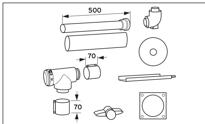
Abb. 6.71 Lieferumfang Art.-Nr. 303 220
