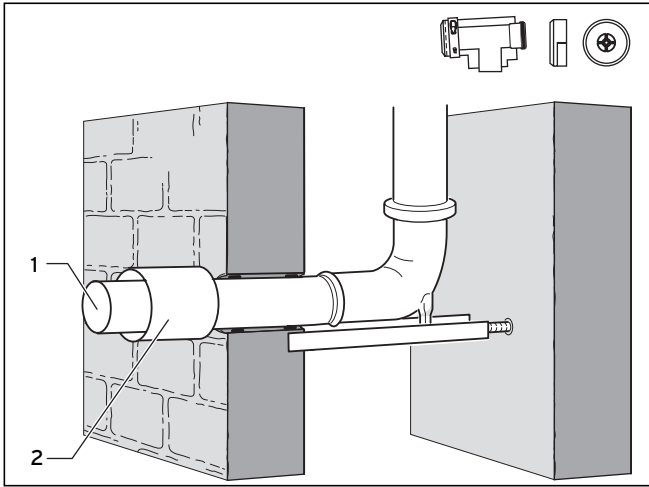
Abb. 6.24 Raumluftabhängiger Betrieb
