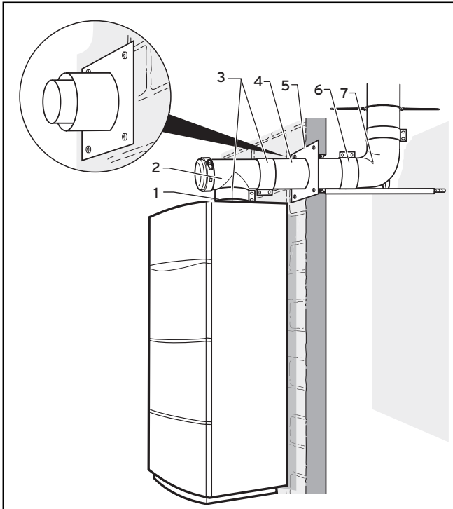
Abb. 6.76 Direktinstallation
