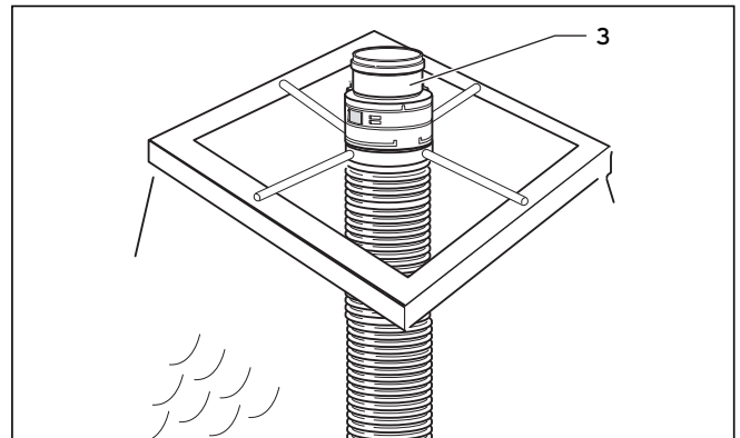
Abb. 6.46 Verbindungsstück mit flexibler Abgasleitung
