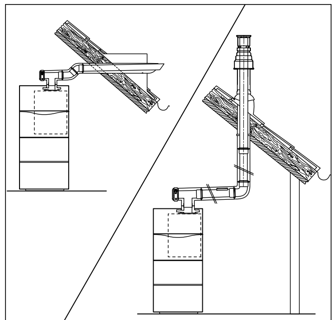
Abb. 5.3 Luft-/Abgasführung mit Vaillant Zubehör (Beispiele)
