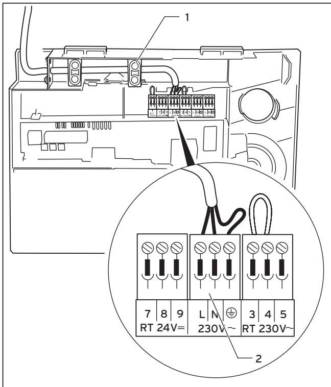
Abb. 5.6 Anschluss der Netzzuleitung
