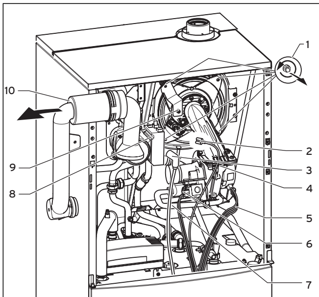
Abb. 8.2 Brennermodul ausbauen
