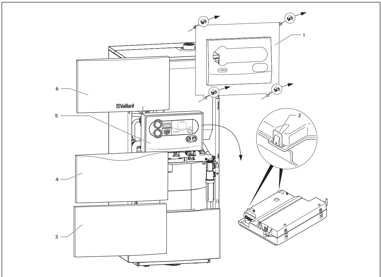
Abb. 5.5 Geräteverkleidung abnehmen
