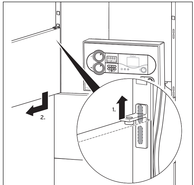
Abb. 4.10 Tür entfernen
