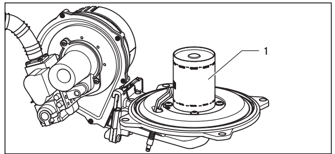
Abb. 8.5 Brenner prüfen
