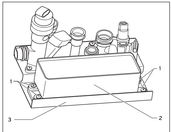
Abb. 8.12 Sekundär-Wärmetauscher entkalken
