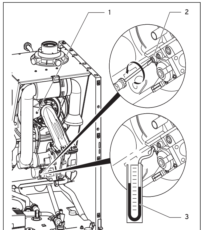
Abb. 7.5 Anschlussdruck (Gasfließdruck) messen
