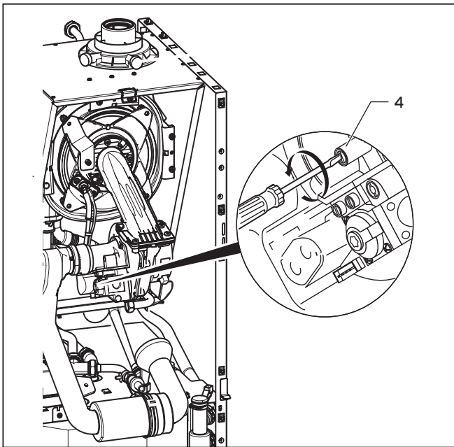
Abb. 7.6 Luftzahl einstellen
