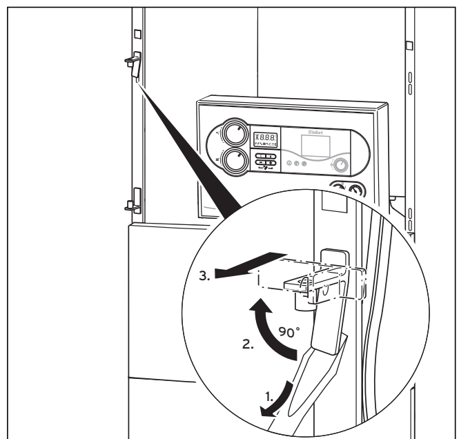
Abb. 4.11 Türanschlag wechseln
