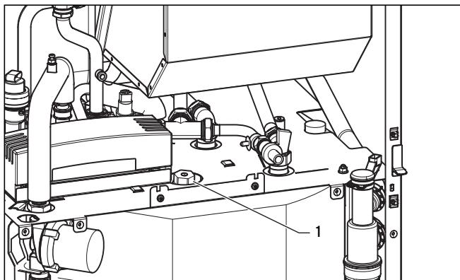
Abb. 8.13 Magnesium-Schutzanode warten
