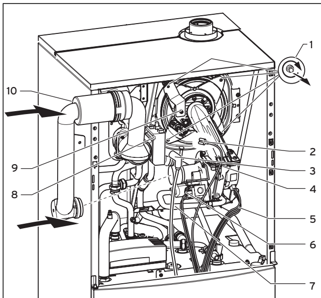
Abb. 8.7 Brennermodul einbauen
