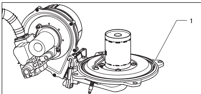
Abb. 8.6 Brenntürdichtung ersetzen
