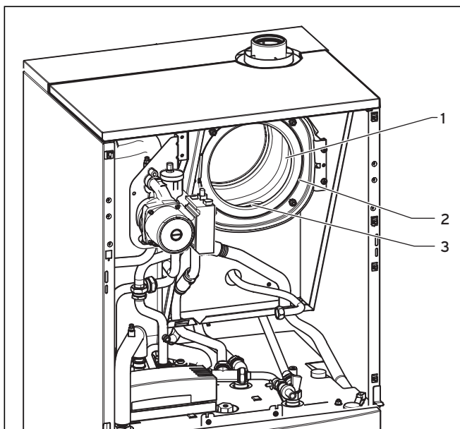
Abb. 8.4 Integral-Kondensations-Wärmetauscher reinigen
