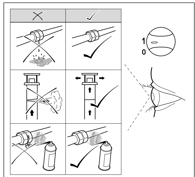
Abb. 6.6 Funktionsprüfung
