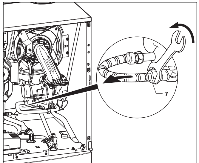
Abb. 8.3 Gaszuleitung trennen
