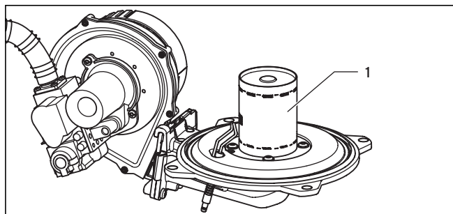
Abb. 8.5 Brenner prüfen
