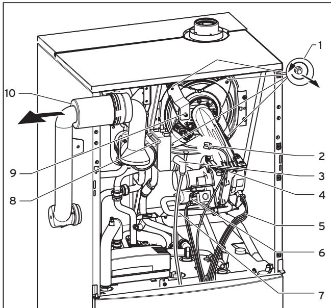
Abb. 8.2 Brennermodul ausbauen
