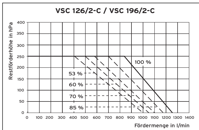
Abb. 7.2 Pumpenkennlinie VSC 126/2-C und 196/2-C
