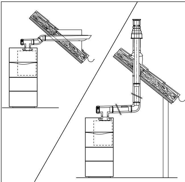
Abb. 5.4 Luft-/Abgasführung mit Vaillant Zubehör (Beispiele)
