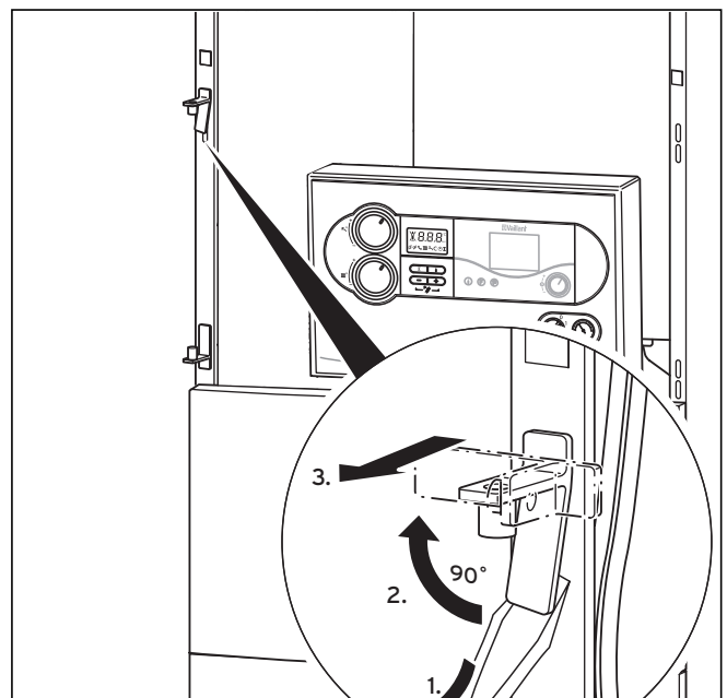
Abb. 4.11 Türanschlag wechseln
