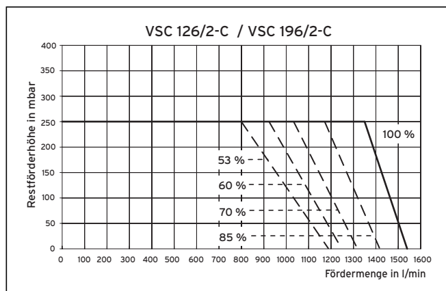
Abb. 7.2 Pumpenkennlinie VSC 126/2-C / VSC 196/2-C
