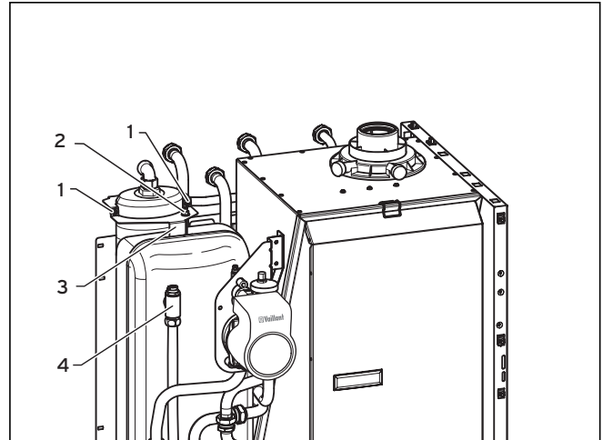
Abb. 9.5 Austauschen des Ausdehnungsgefäßes
