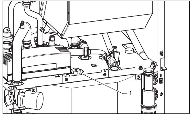
Abb. 8.13 Magnesium-Schutzanode warten
