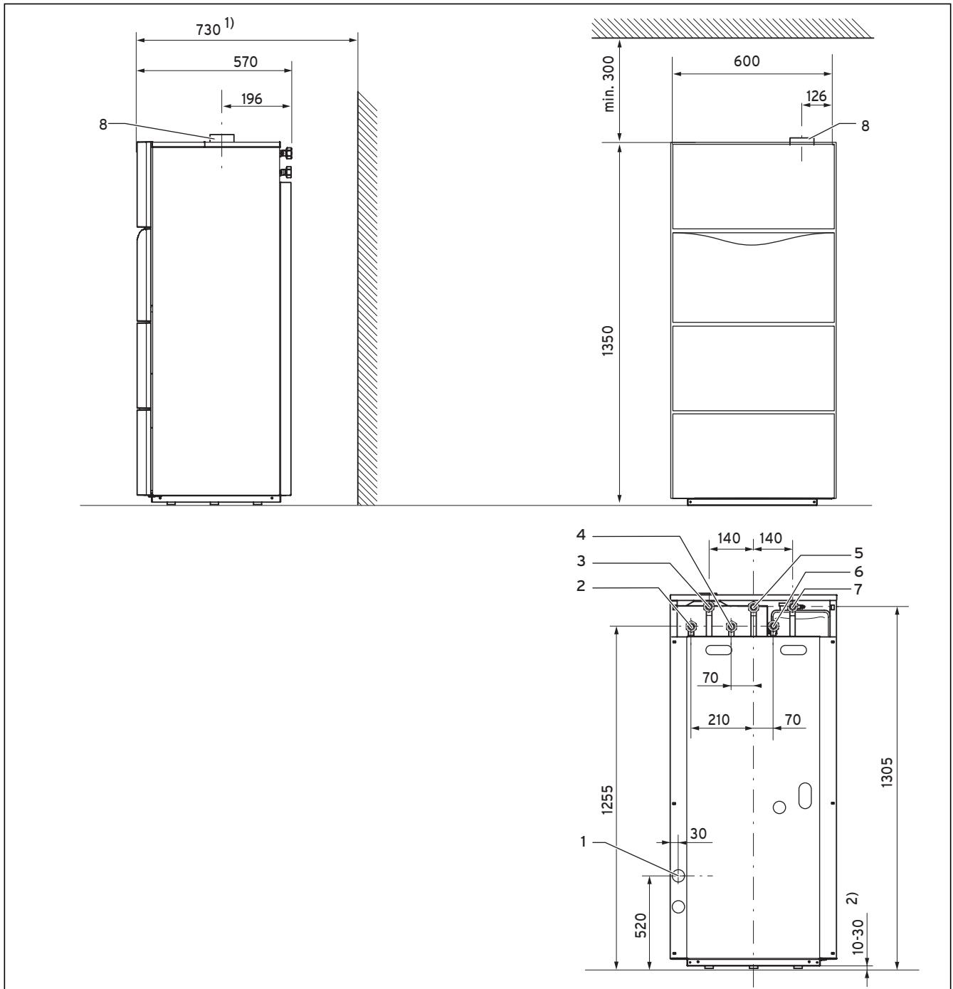
Abb. 4.7 Abmessungen in mm VSC 126/2-C 140, VSC 196/2-C 150
