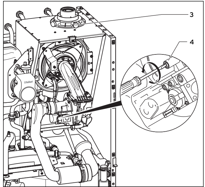
Abb. 6.5 CO 2 -Prüfung
