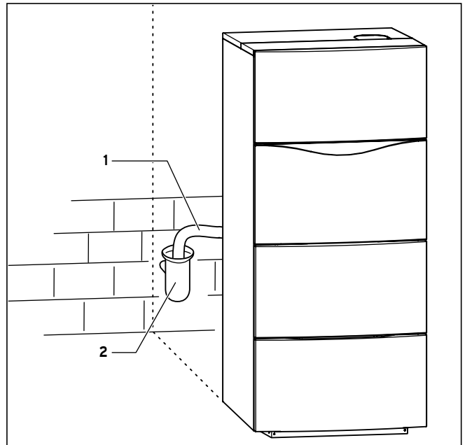
Abb. 5.5 Kondenswasser-Ablaufschlauch installieren
