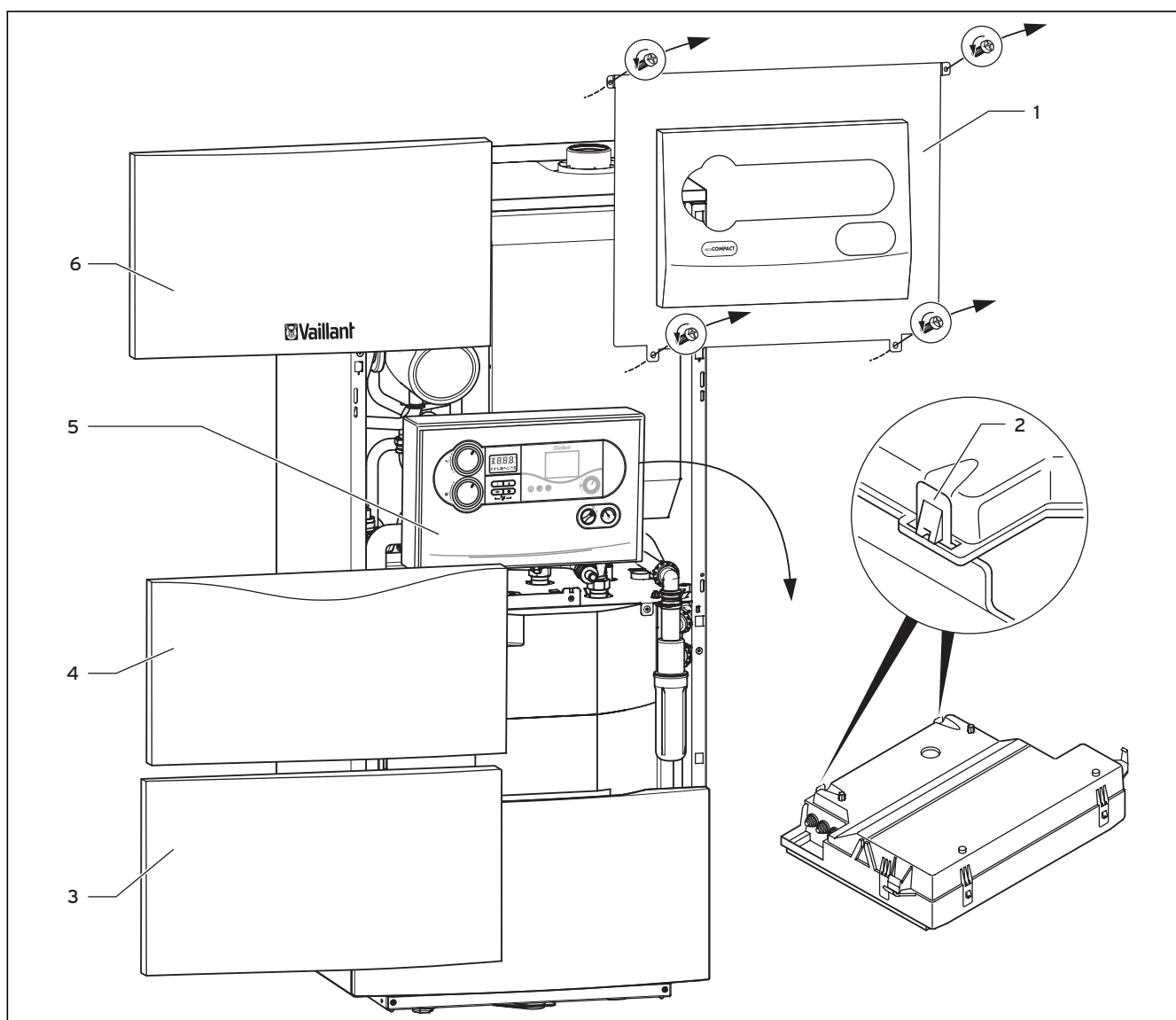
Abb. 5.6 Geräteverkleidung abnehmen
