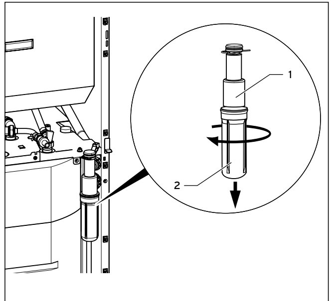
Abb. 8.8 Siphon reinigen
