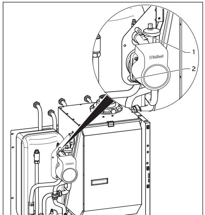
Abb. 8.11 Pumpe ausbauen
