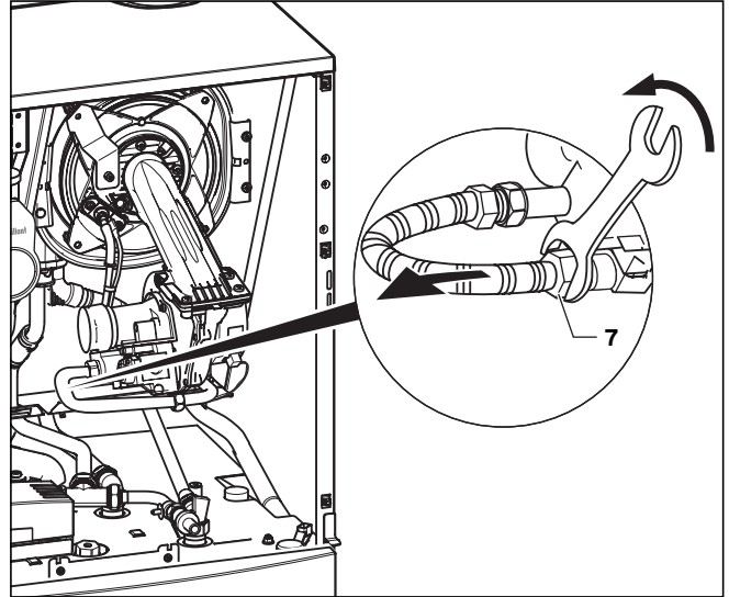
Abb. 8.3 Gaszuleitung trennen
