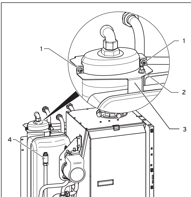
Abb. 5.3 Warmwasser-Ausdehnungsgefäß Ein-/Ausbau
