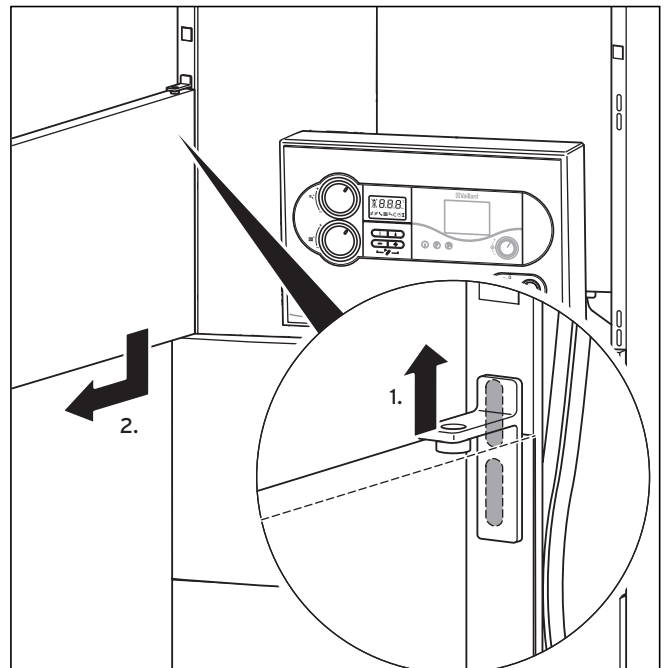
Abb. 4.10 Tür entfernen
