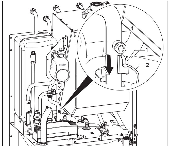
Abb. 9.7 Anschluss-Stutzen für Kapillarrohr
