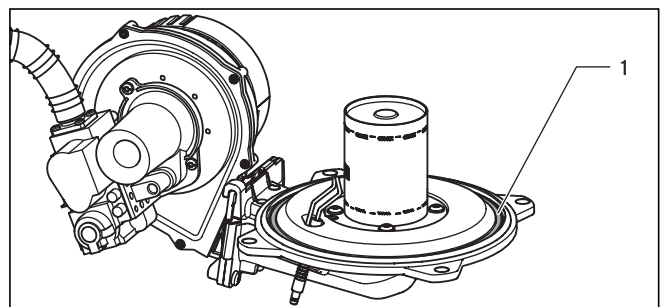
Abb. 8.6 Brennertürdichtung ersetzen
