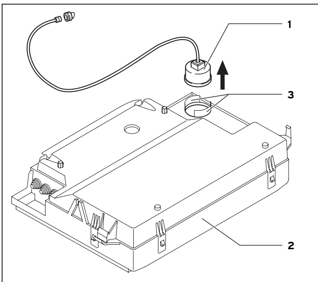
Abb. 9.6 Manometer austauschen
