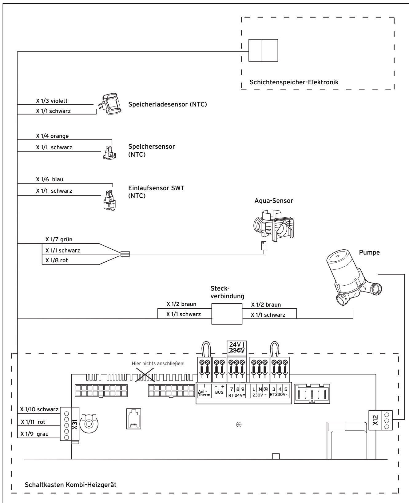
Abb. 5.13 Verdrahtungsplan Schichtenspeicher
