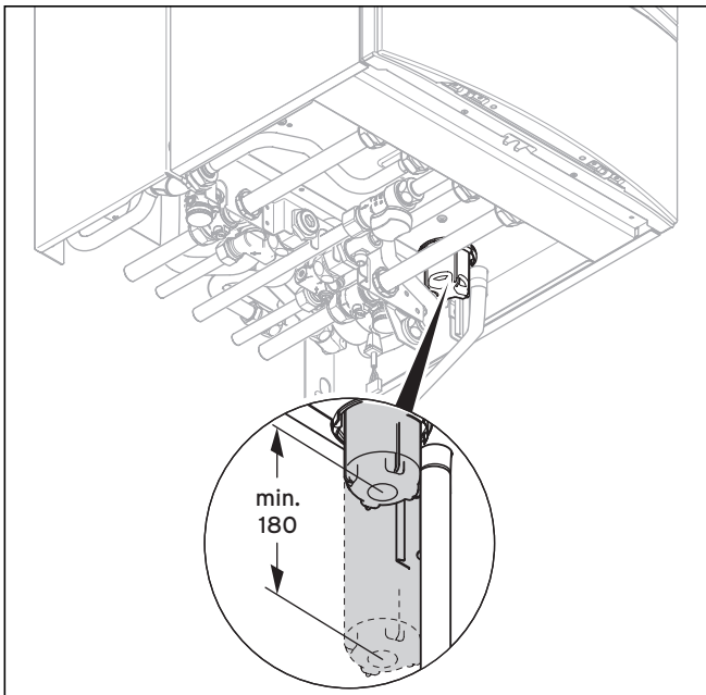
Abb. 5.7 Montageraum Kondenswassersiphon
