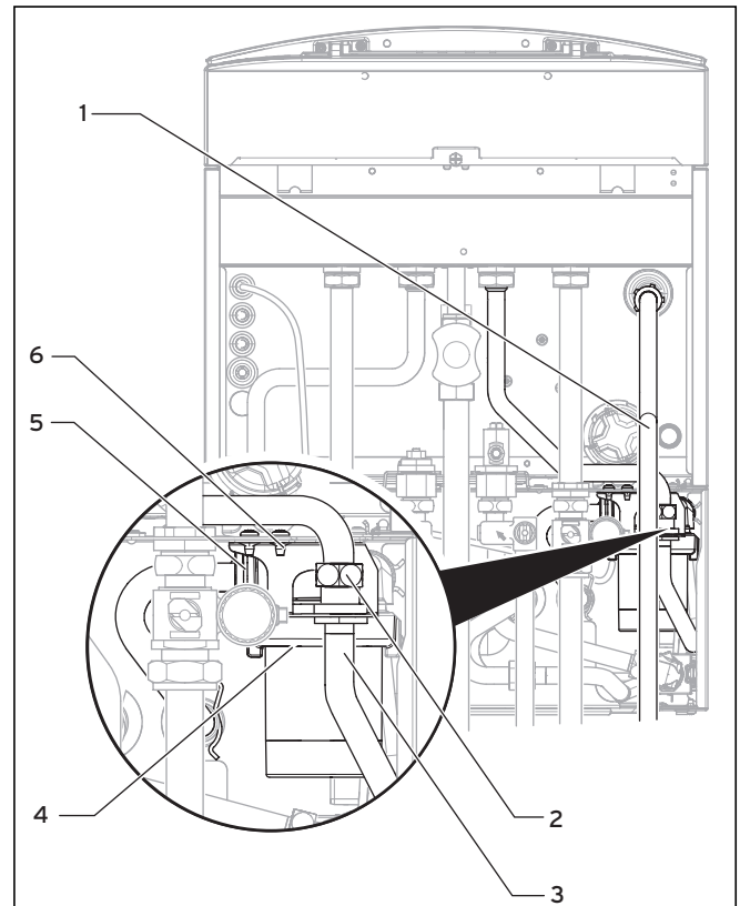
Abb. 10.1 Speicherladepumpe austauschen
