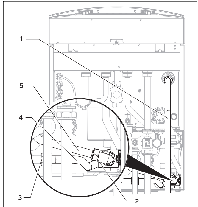
Abb. 10.2 Aqua-Sensor austauschen
