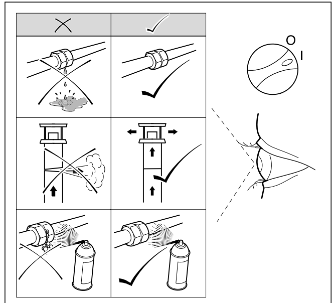
Abb. 8.3 Funktionsprüfung
