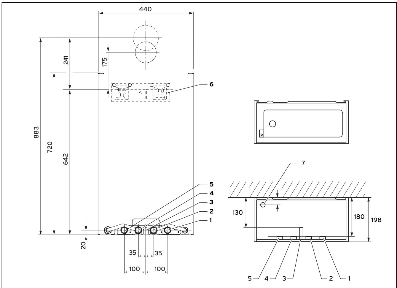
Abb. 4.2 Abmessungen Schichtenspeicher
