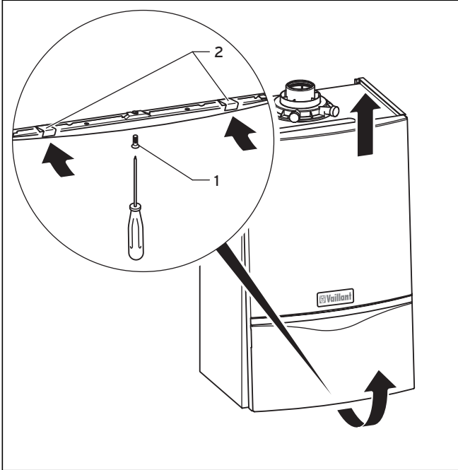
Abb. 4.6 Frontverkleidung abnehmen
