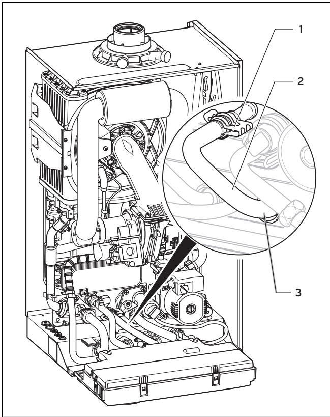
Abb. 4.8 Rohrleitungsbogen einbauen
