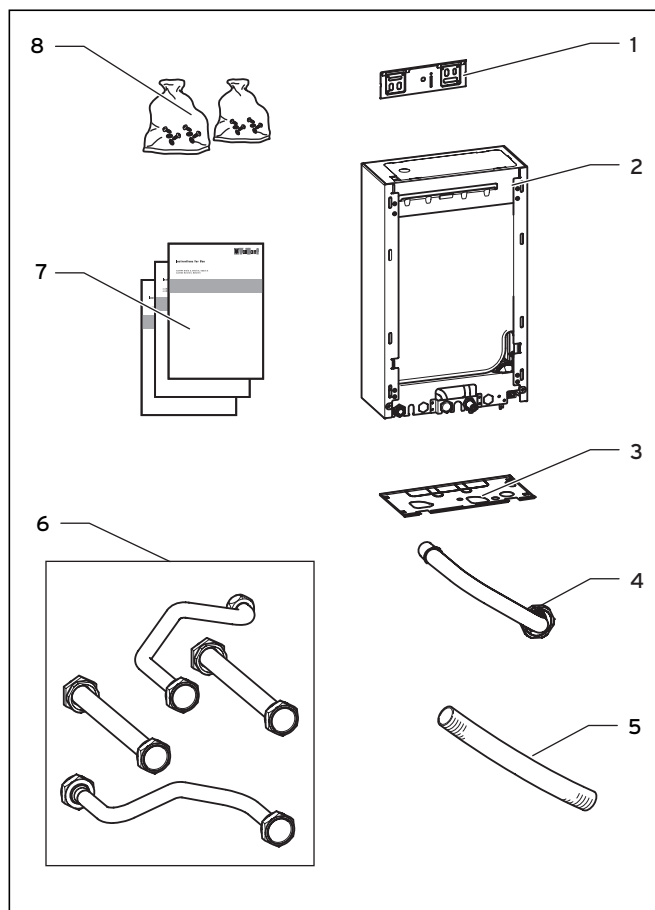
Abb. 4.1 Lieferumfang
