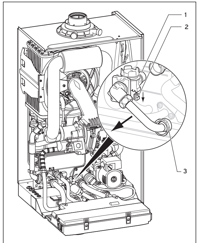
Abb. 4.7 Aqua-Sensor ausbauen
