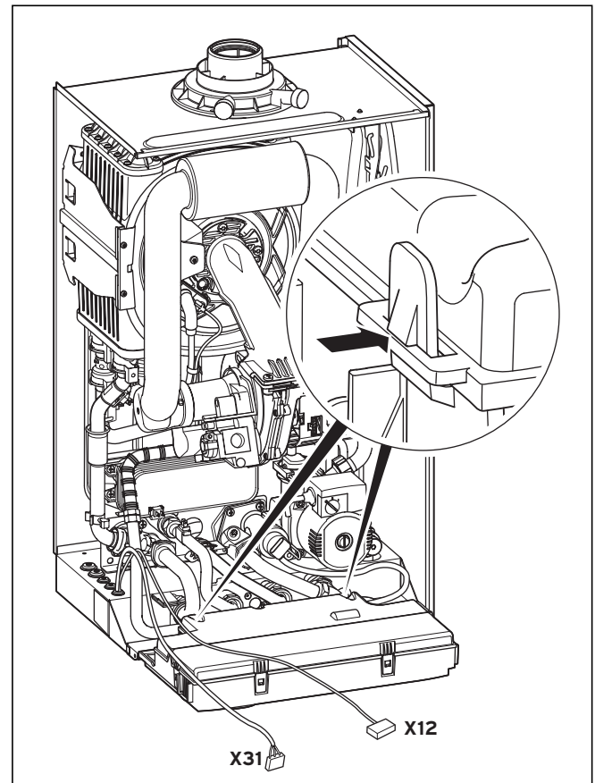
Abb. 5.10 Schaltkastenrückwand öffnen
