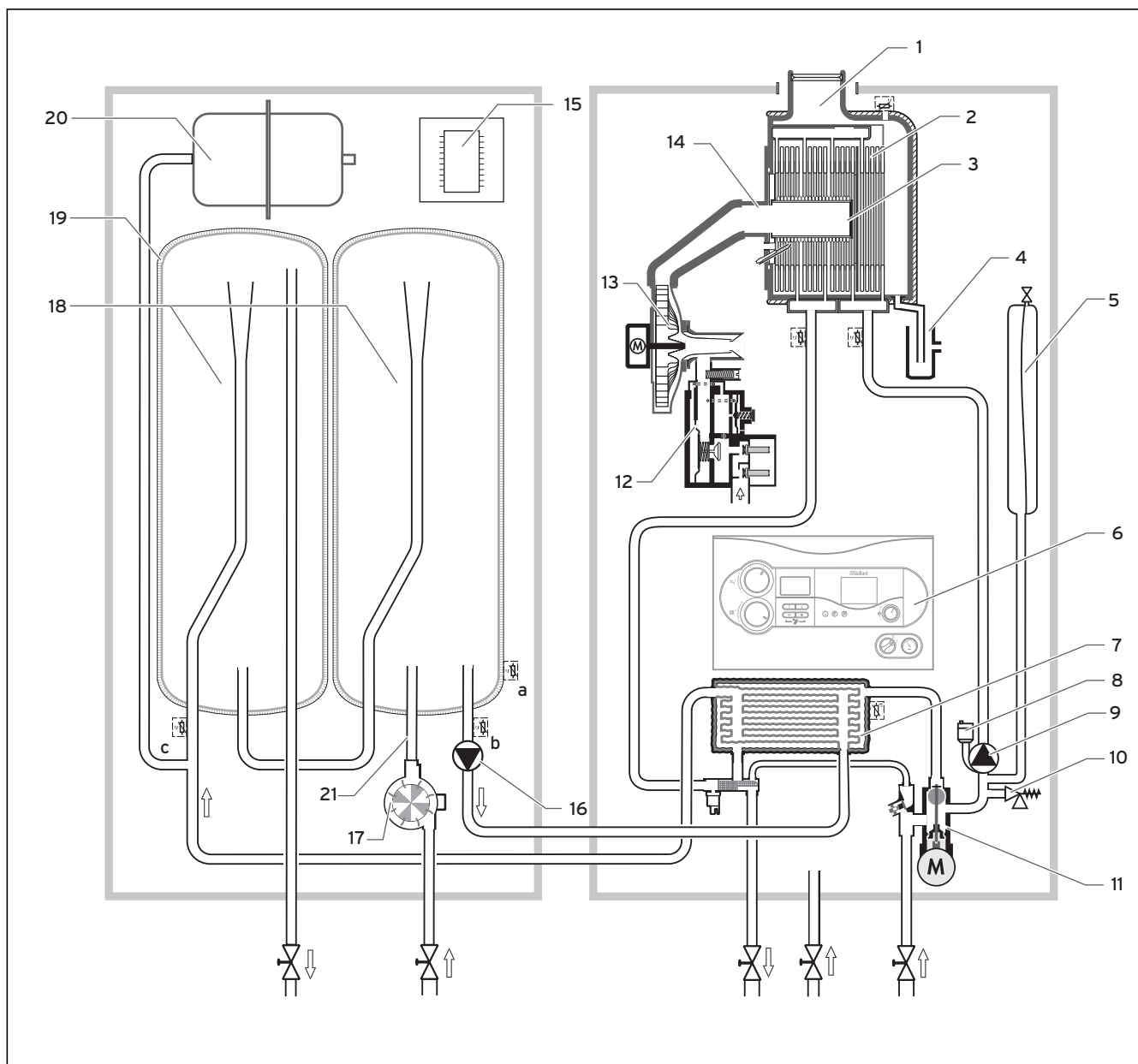
Abb. 2.2 Ablaufschema
