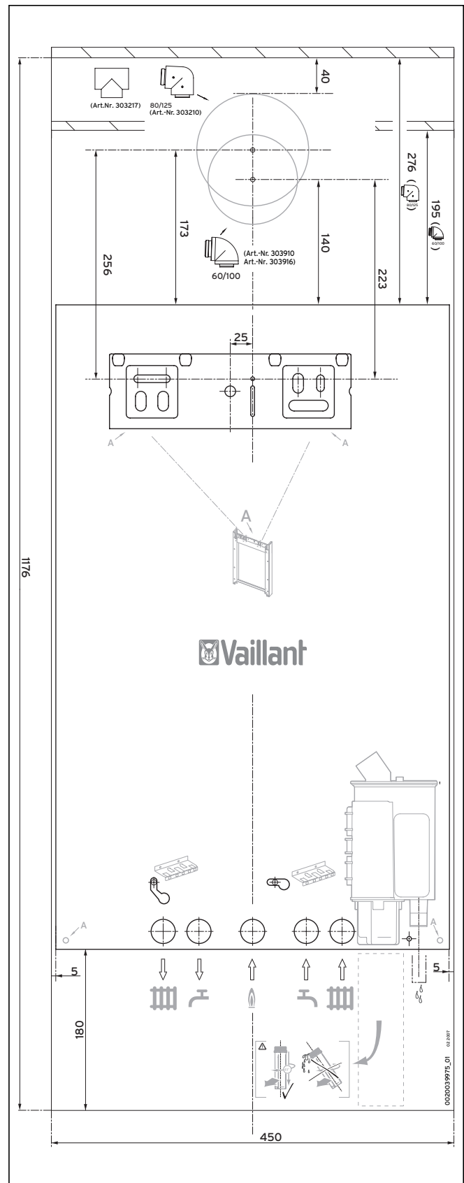
Abb. 4.3 Montageschablone/Montagefreiräume
