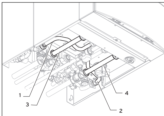
Abb. 5.3 Rohrverbindungen zwischen actoSTOR VIH CL 20 S und ecoTEC plus montieren
