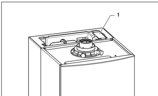
Abb. 10.3 Elektronik austauschen
