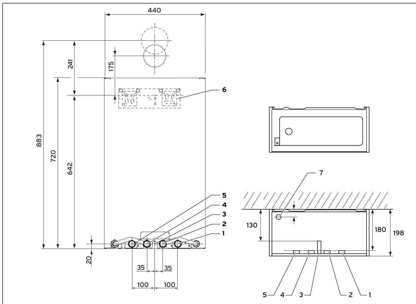
Abb. 4.2 Abmessungen Schichtenspeicher
