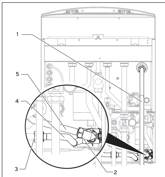
Abb. 10.2 Aqua-Sensor austauschen
