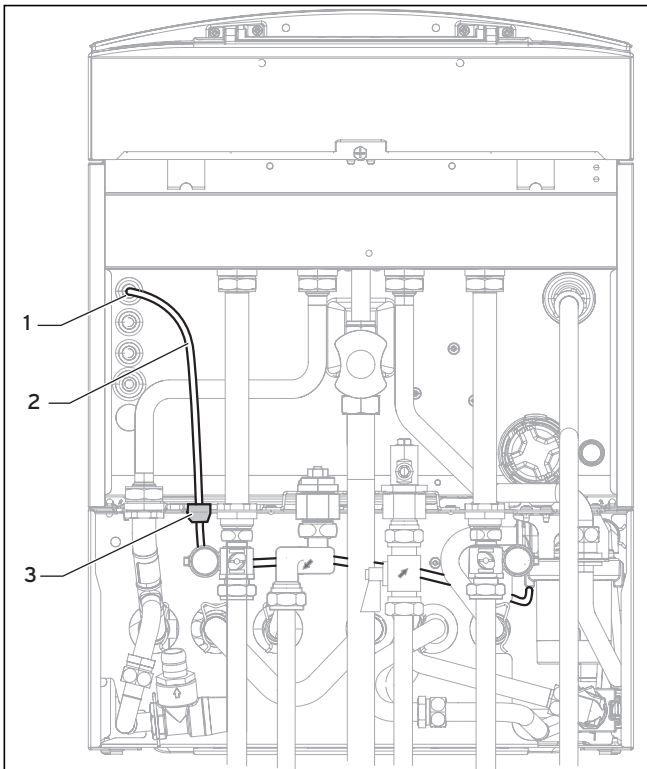
Abb. 5.11 Kabelführung an der Geräteunterseite
