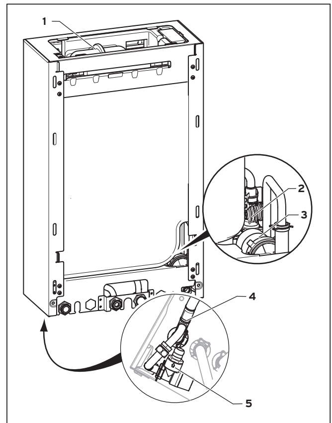
Abb. 2.1 Funktionselemente Schichtenspeicher actoSTOR VIH CL 20 S
