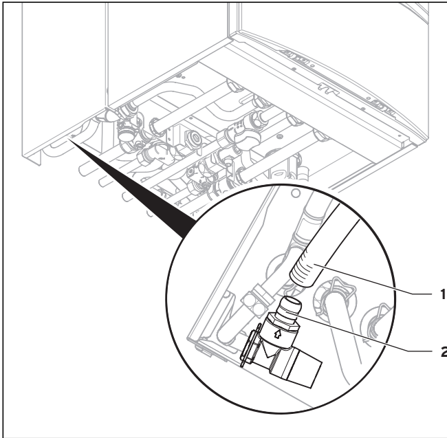
Abb. 5.9 Anschluss Ablaufleitung Warmwasser-Sicherheitsventil
