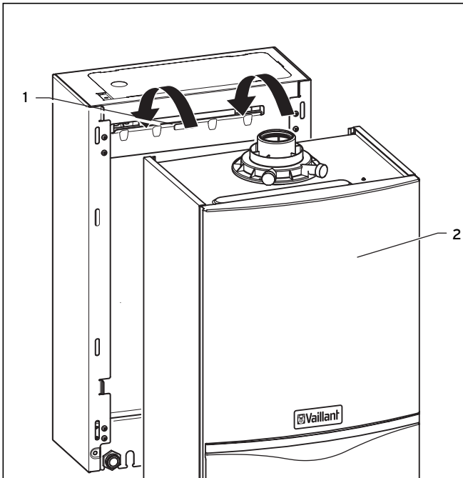
Abb. 4.5 Montage ecoTEC plus an actoSTOR VIH CL 20 S
