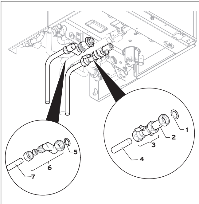
Abb. 5.2 Installieren des Kalt- und Warmwasseranschlusses
