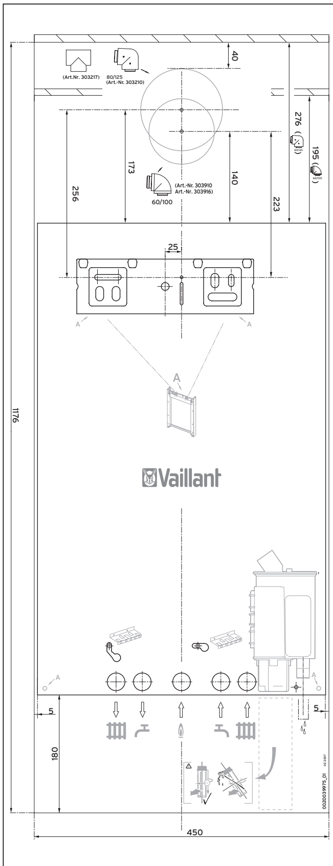
Abb. 4.3 Montageschablone/Montagefreiräume
