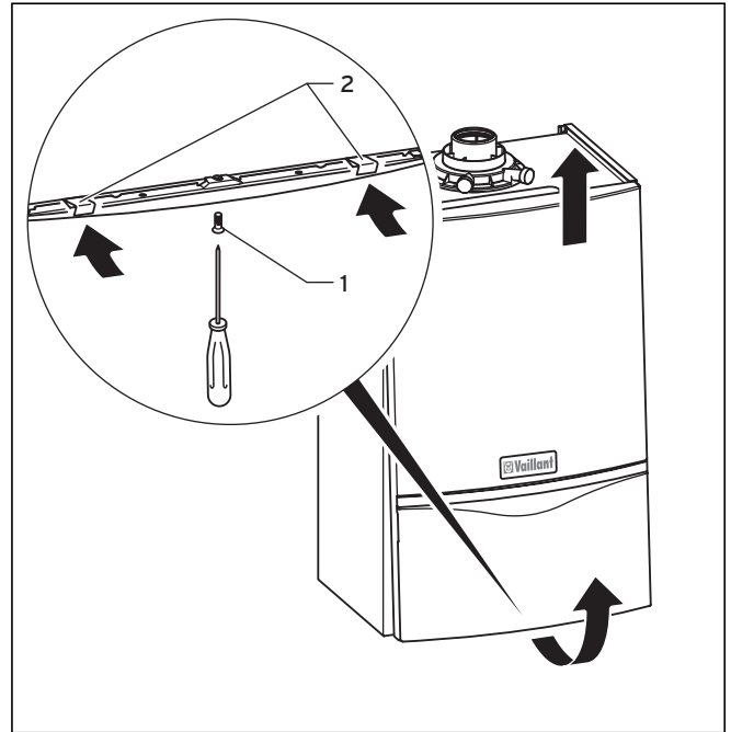
Abb. 4.6 Frontverkleidung abnehmen
