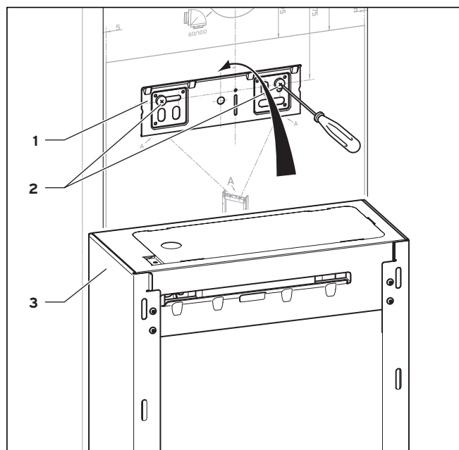
Abb. 4.4 actoSTOR VIH CL 20 S mit Gerätehalter
