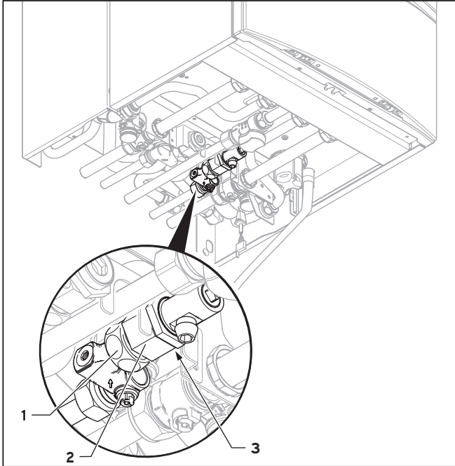
Abb. 8.1 Ausbau des Siebs im Kaltwassereingang
