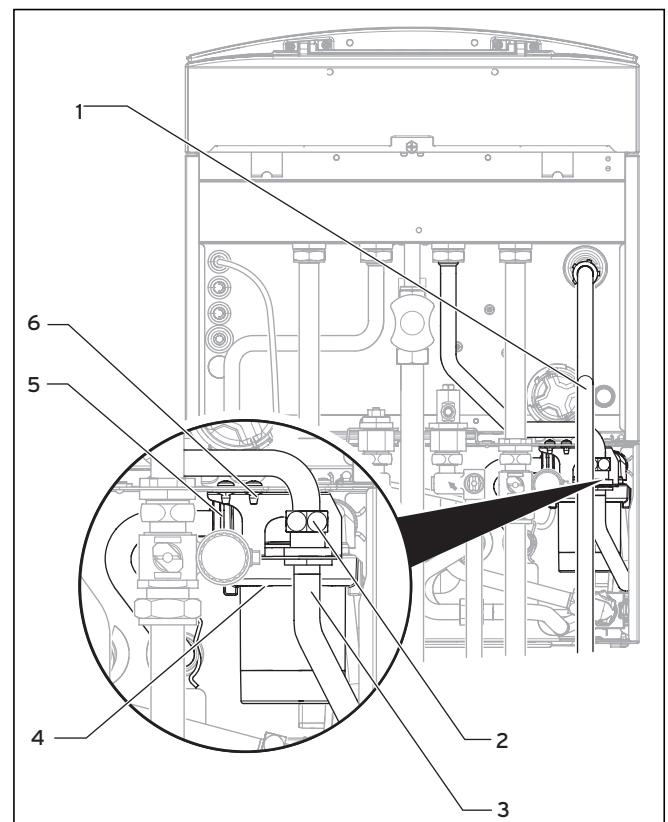
Abb. 10.1 Speicherladepumpe austauschen
