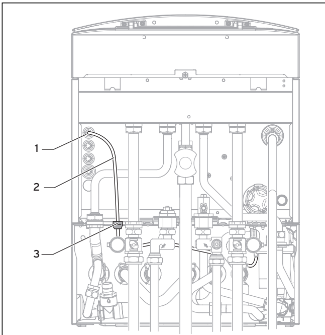
Abb. 5.11 Kabelführung an der Geräteunterseite
